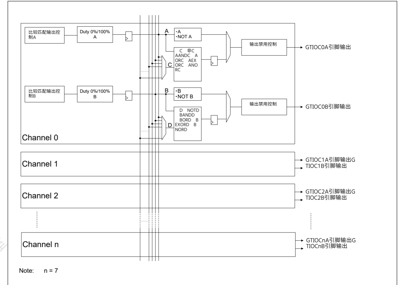
Figure 21.61 通道间逻辑操作框图
