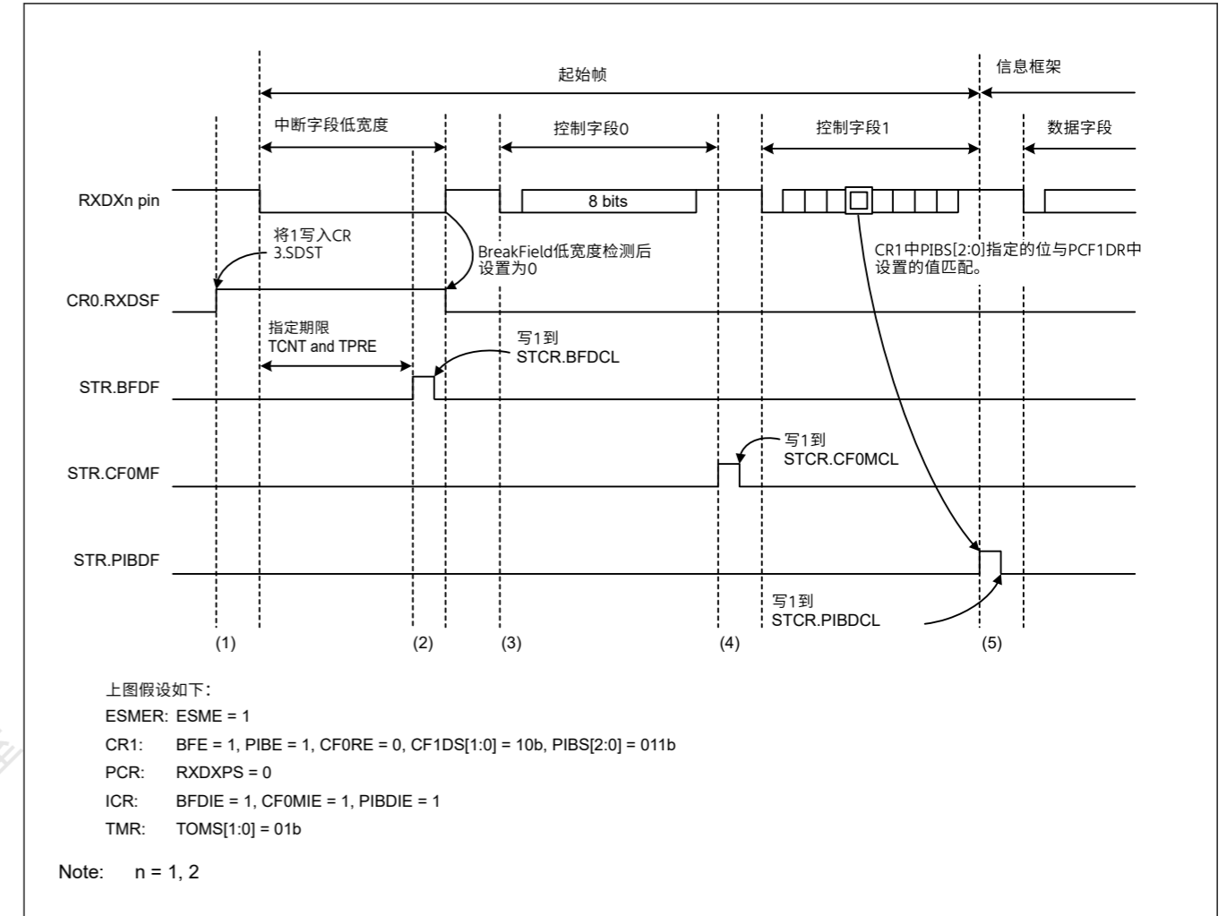
图27.110 CR1.PIBE位为1时接收起始帧时的操作示例
