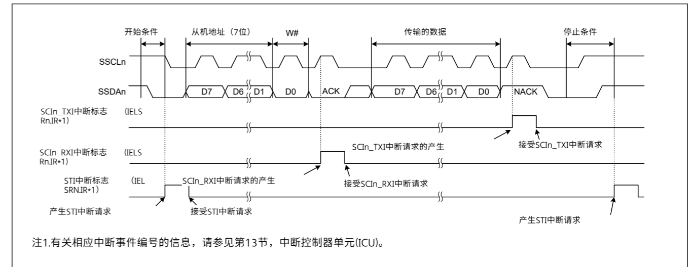
Figure 27.94 使用7位从机地址、ACK中断和NACK中断的简单IIC模式下主机传输操作示例2
