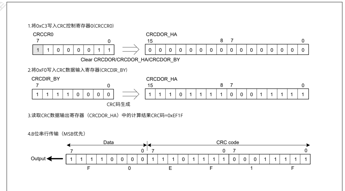
Figure 34.3 MSB优先数据传输
