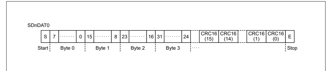
Figure 33.2 SDnDAT在1位宽模式下
