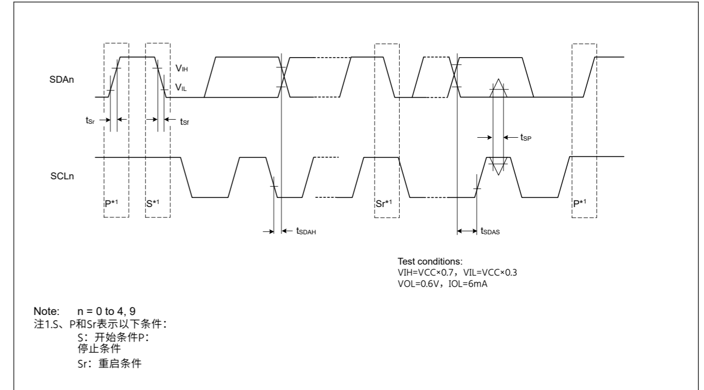
Figure 47.33 SCI简单IIC模式时序
