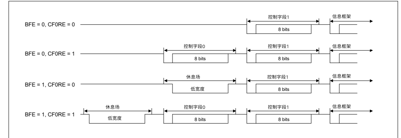
图27.105起始帧的结构
