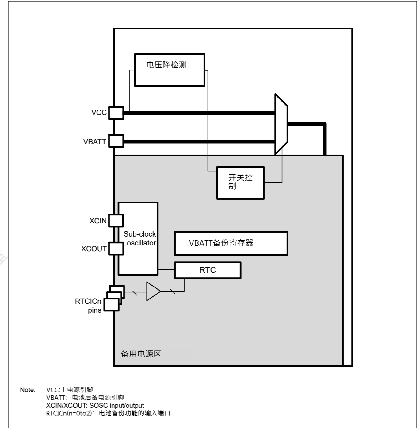
Figure 11.1 电池备份功能的配置
