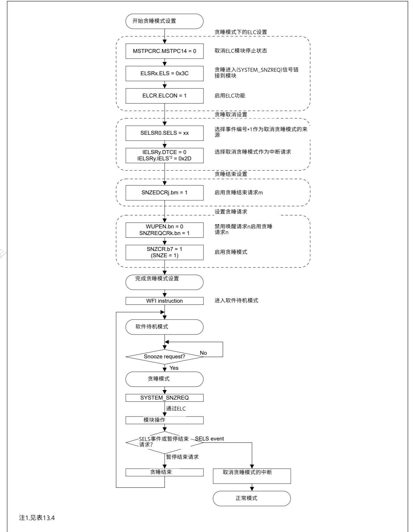
Figure 10.6 在贪睡模式下使用ELC的设置示例
