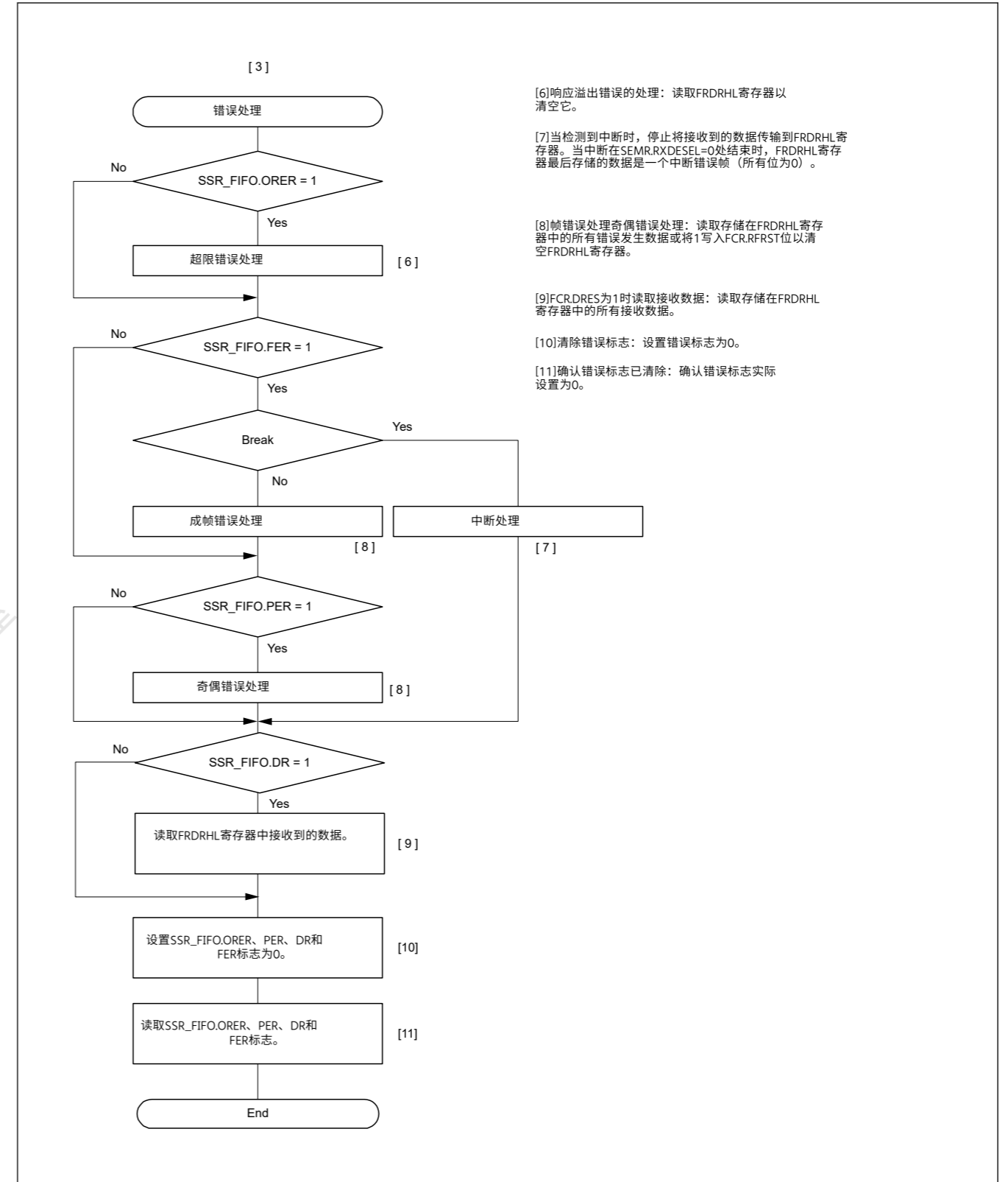
Figure 27.30 异步模式下串行接收的示例流程图（FIFO选择和地址匹配使能）(3)
