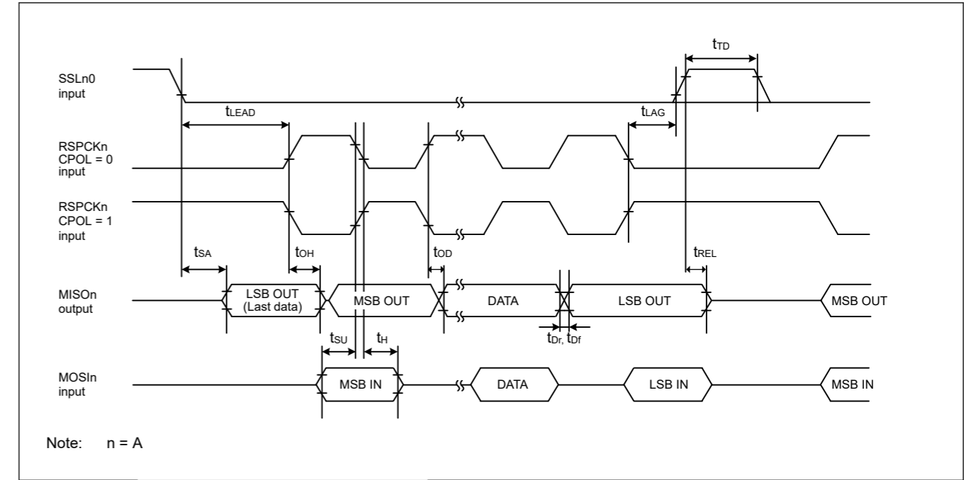
Figure 47.40 CPHA=1时从机的SPI时序
