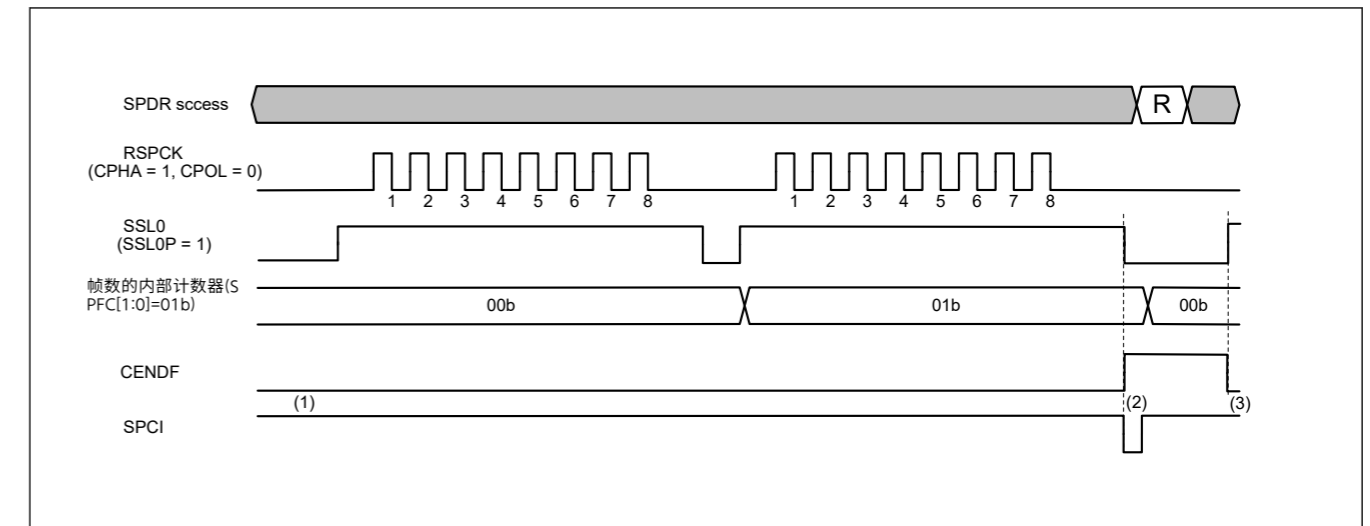
Figure 30.33 通信结束中断操作示例 (SPI上仅接收从模式 Operation)
