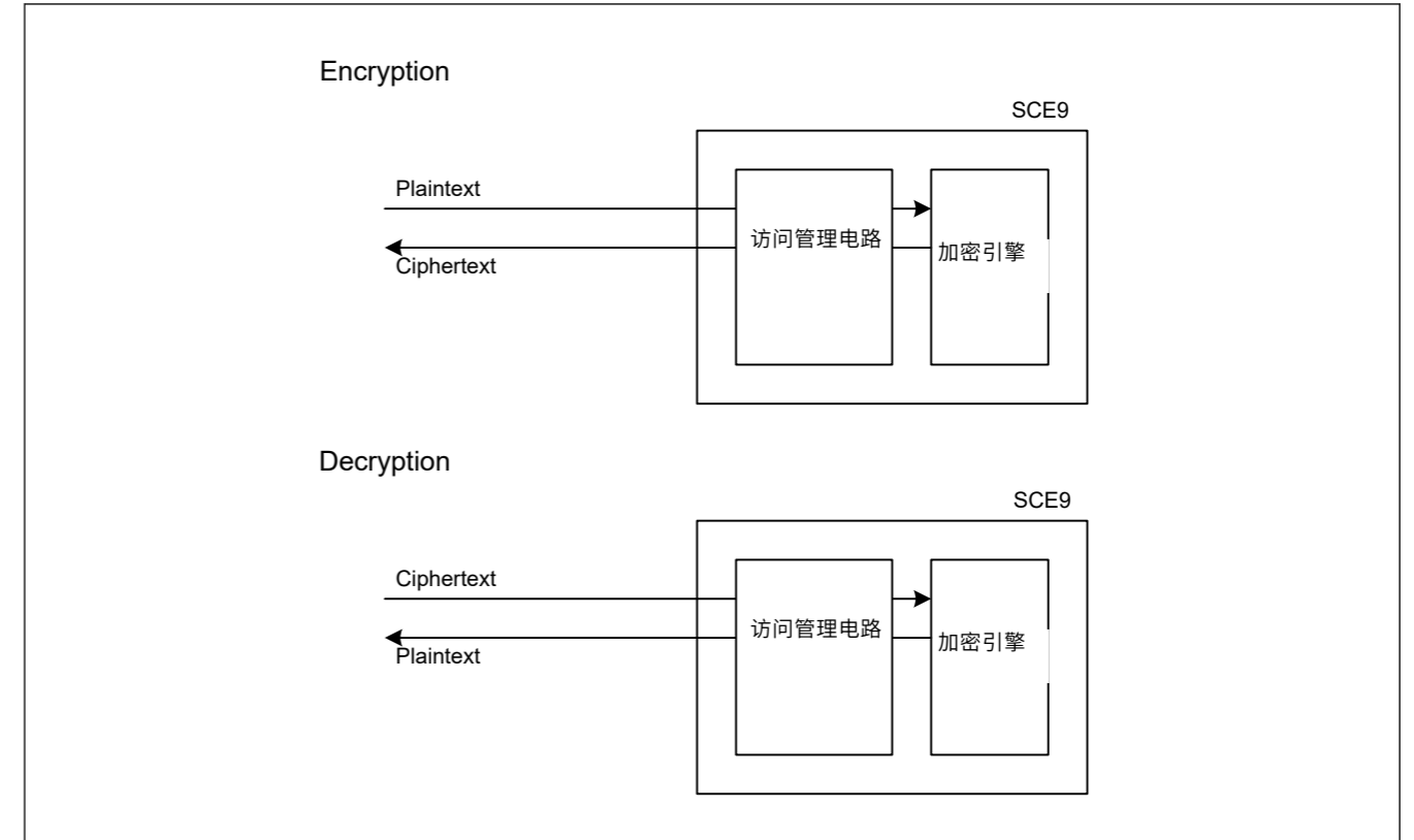
Figure 36.2 加密引擎的概念图
