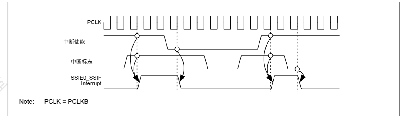
Figure 32.59 公共中断源的时序图, SSIE0_SSIF
