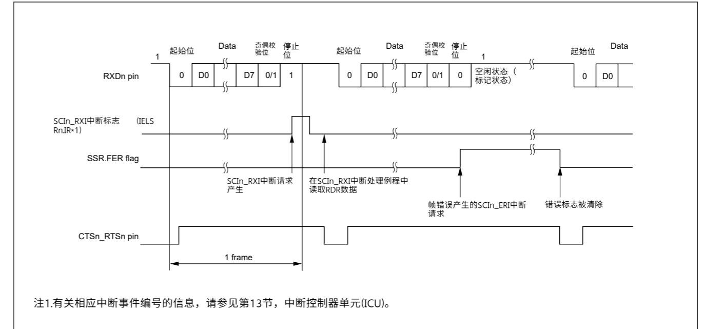
Figure 27.19 使用RTS功能,8位数据、奇偶校验位和1个停止位时,异步模式下串行接收的SCI操作示例(2)
