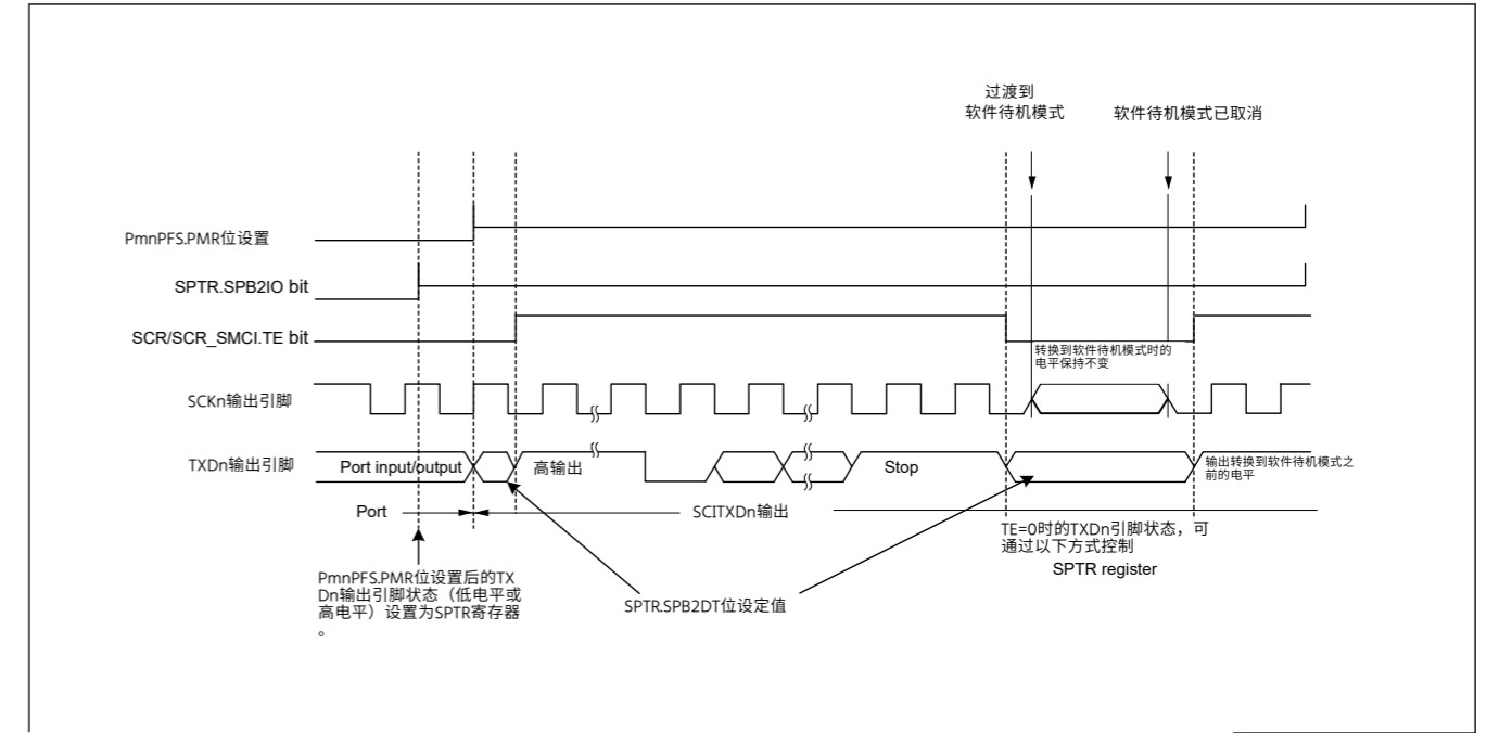
图27.119 转换到内部时钟和异步传输的软件待机模式期间的端口引脚状态
