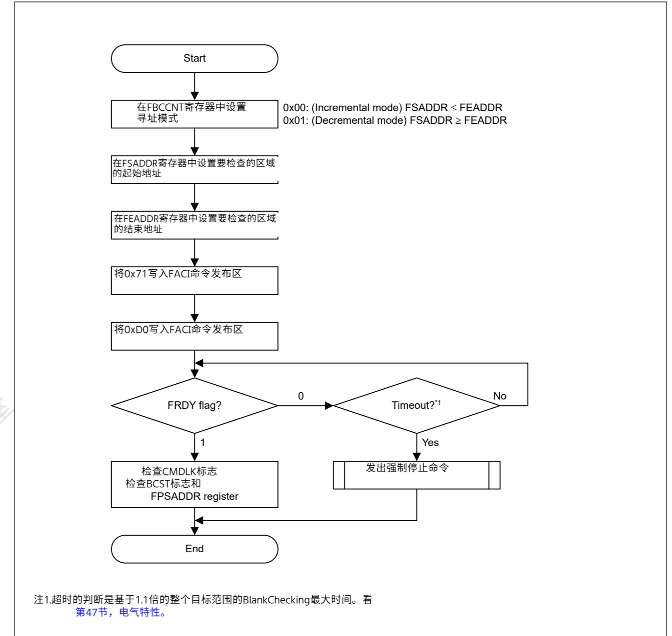
Figure 44.23 空白检查命令的使用流程
