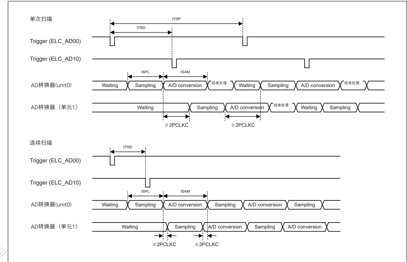
Figure 37.24 交错操作中的触发输入时序
