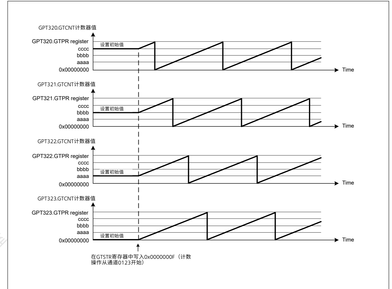
Figure 21.37 以相同计数周期开始的软件阶段示例 (GTPR寄存器值)
