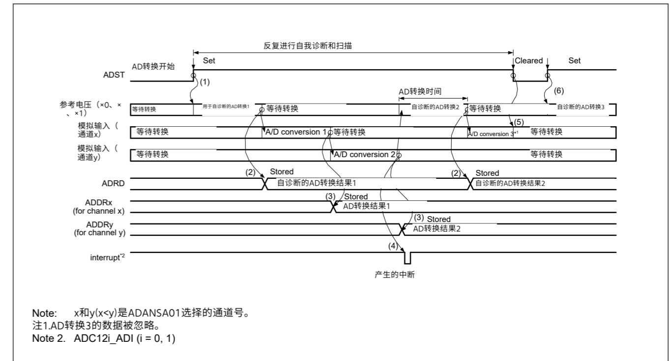
Figure 37.14 使用自诊断选择模拟输入（通道x和y）时连续扫描模式下的基本操作示例
