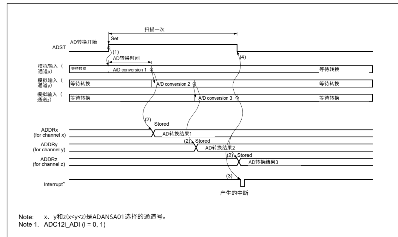
Figure 37.8 选择模拟输入（通道x至z）时单次扫描模式下的基本操作示例
