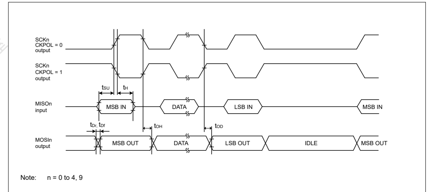
Figure 47.29 CKPH=1时主机的SCI简单SPI模式时序
