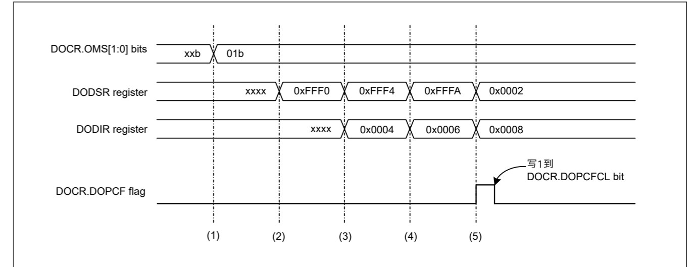
Figure 41.3 数据添加模式中的操作示例
