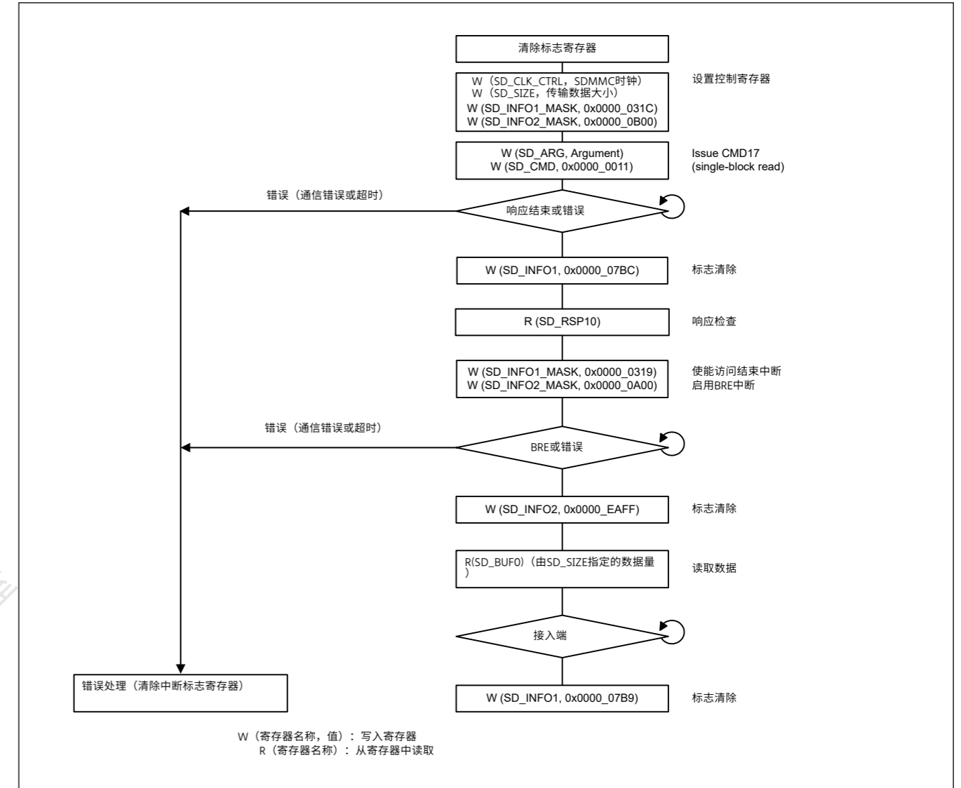
Figure 33.11 单块读操作示例流程
