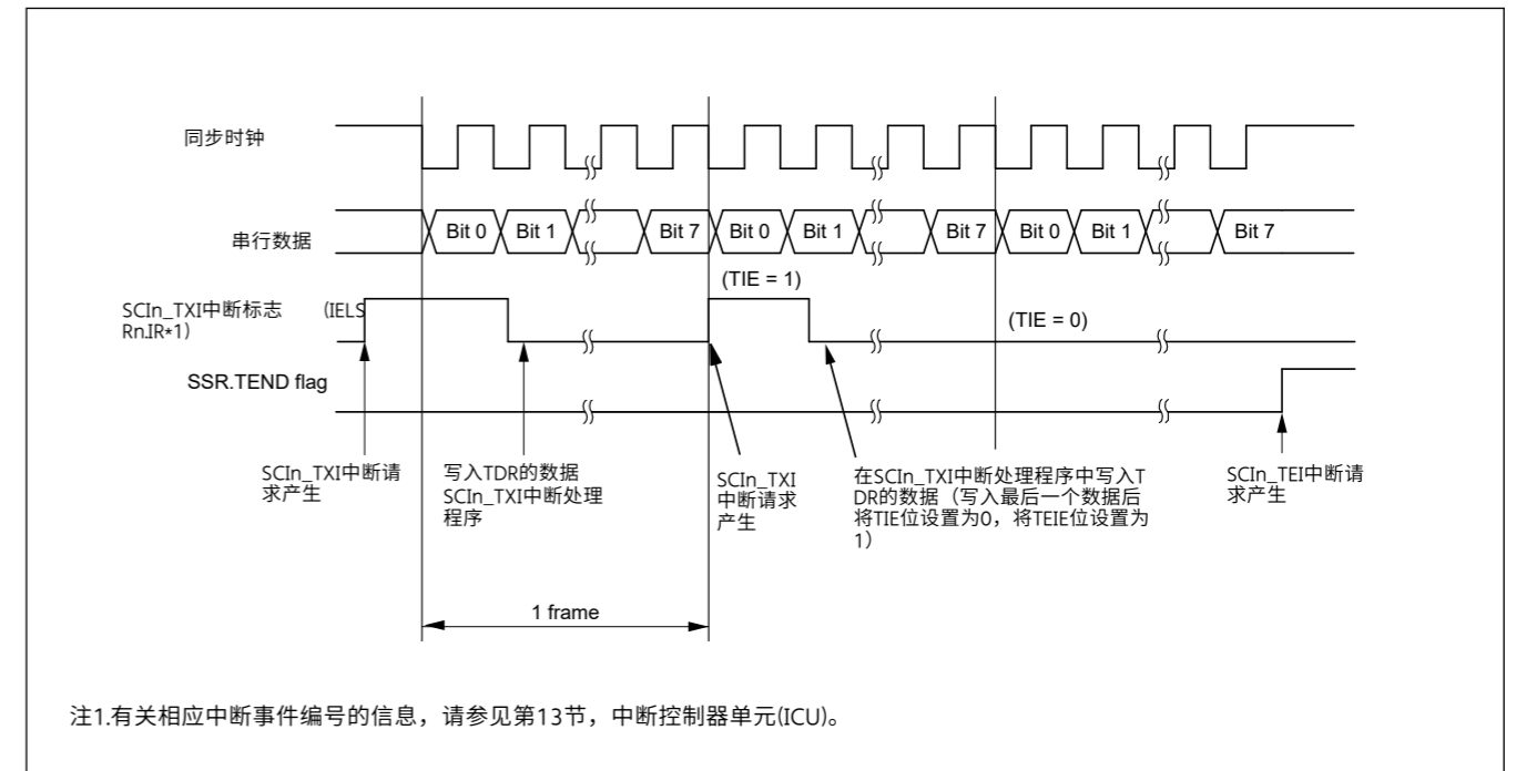
Figure 27.68 从传输中间到传输完成的时钟同步模式下的串行数据传输示例
