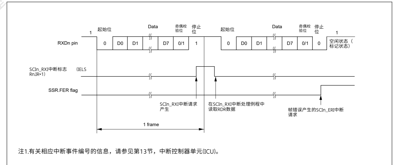
Figure 27.18 异步模式下串行接收的SCI操作示例(1)不使用RTS功能时，具有8位数据、奇偶校验位和1个停止位
