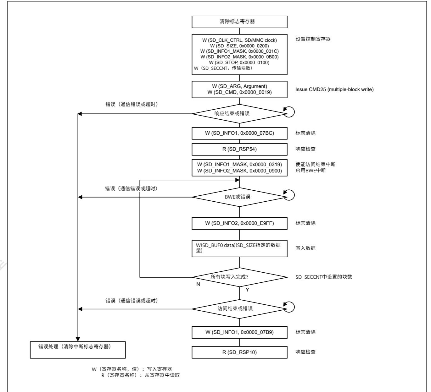
Figure 33.14 使用内部定时器的多块写入操作示例
