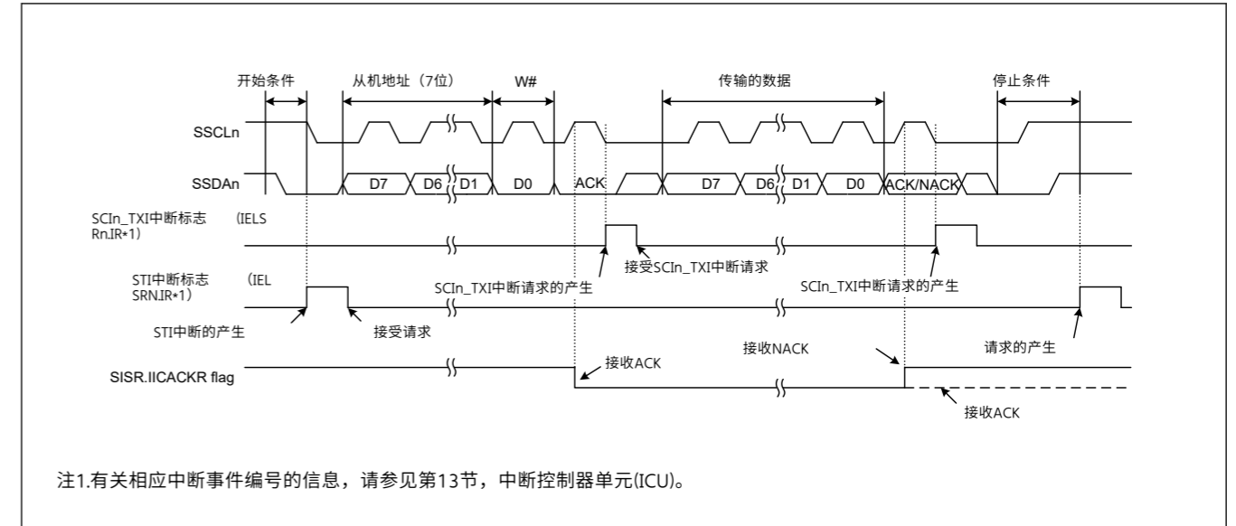
Figure 27.93 简单IIC模式下主机发送操作示例1，具有7位从机地址、发送中断和接收中断
