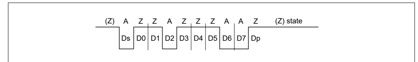
Figure 27.79 与SCMR=0中的SDIR、SCMR=0中的SINV和SMR_SMCI=0中的PM的直接约定
