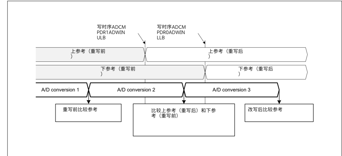
Figure 37.5 重写前后上下引用的比较
