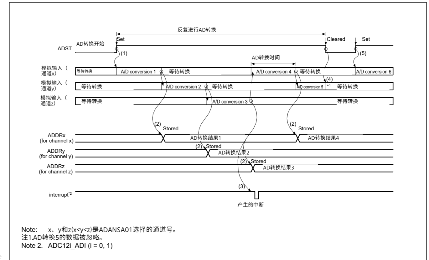
Figure 37.13 选择模拟输入（通道x至z）时连续扫描模式下的基本操作示例
