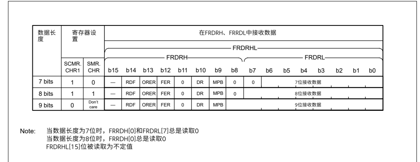
Figure 27.47 选择FIFO的多处理器模式下存储在FRDRH和FRDRL中的数据格式
