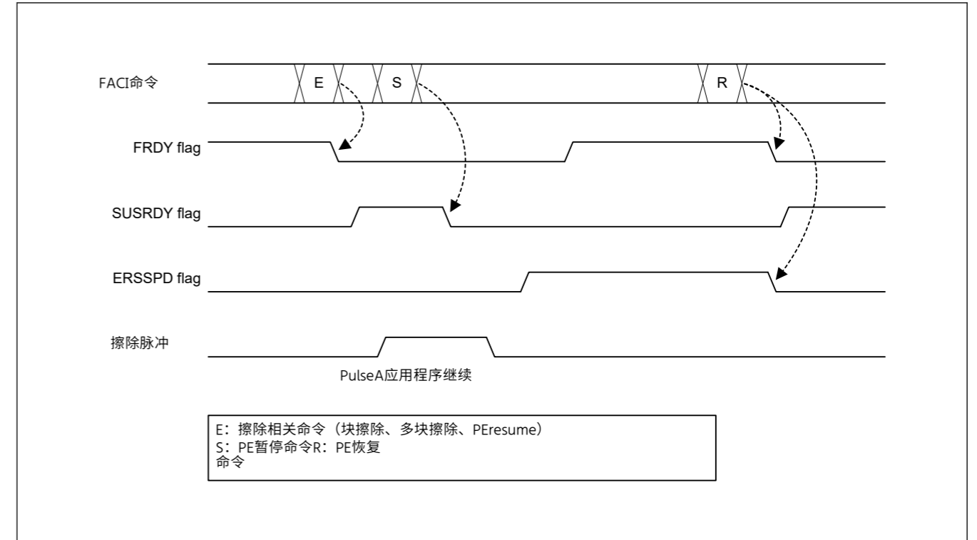
Figure 44.19 擦除期间暂停 (擦除优先模式)
