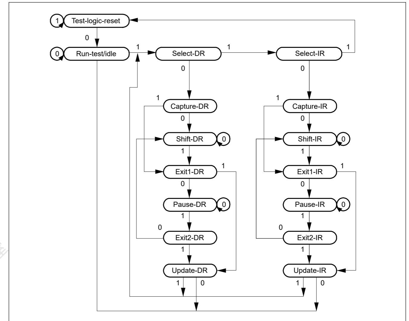
Figure 35.2 TAP控制器的状态转移图
