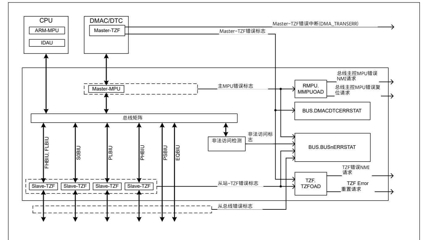
Figure 14.3 总线从每次错误检测到用户通知的操作
