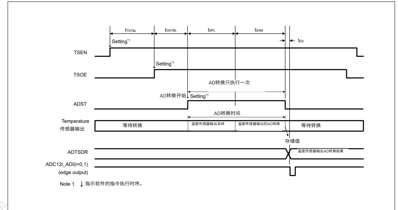
Figure 39.3 从温度传感器操作开始到AD转换完成的时间
