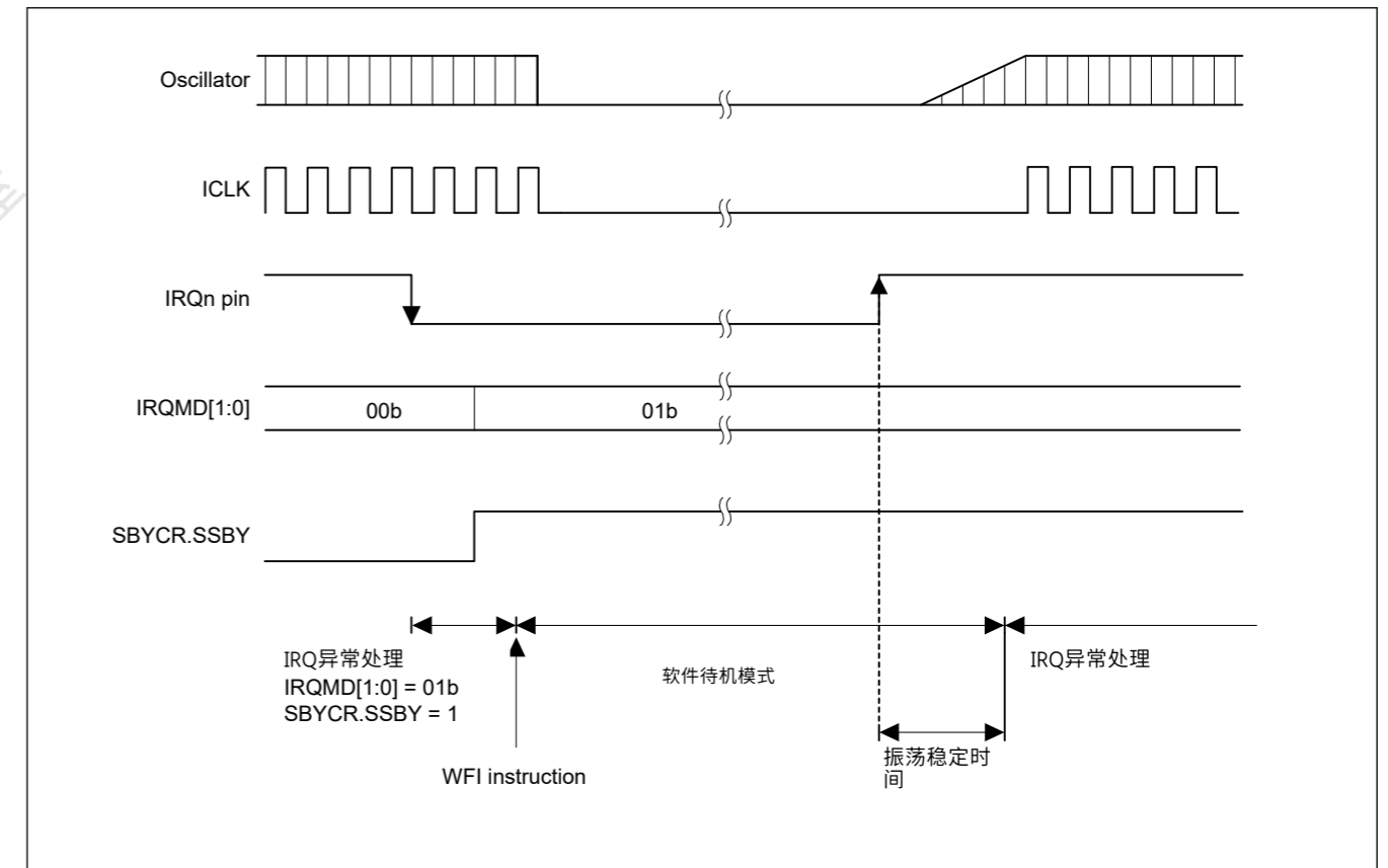
Figure 10.2 软件待机模式应用示例
