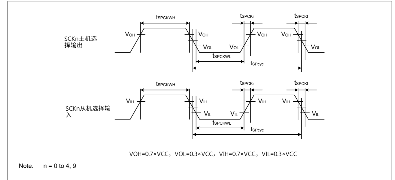
Figure 47.28 SCI简单SPI模式时钟时序
