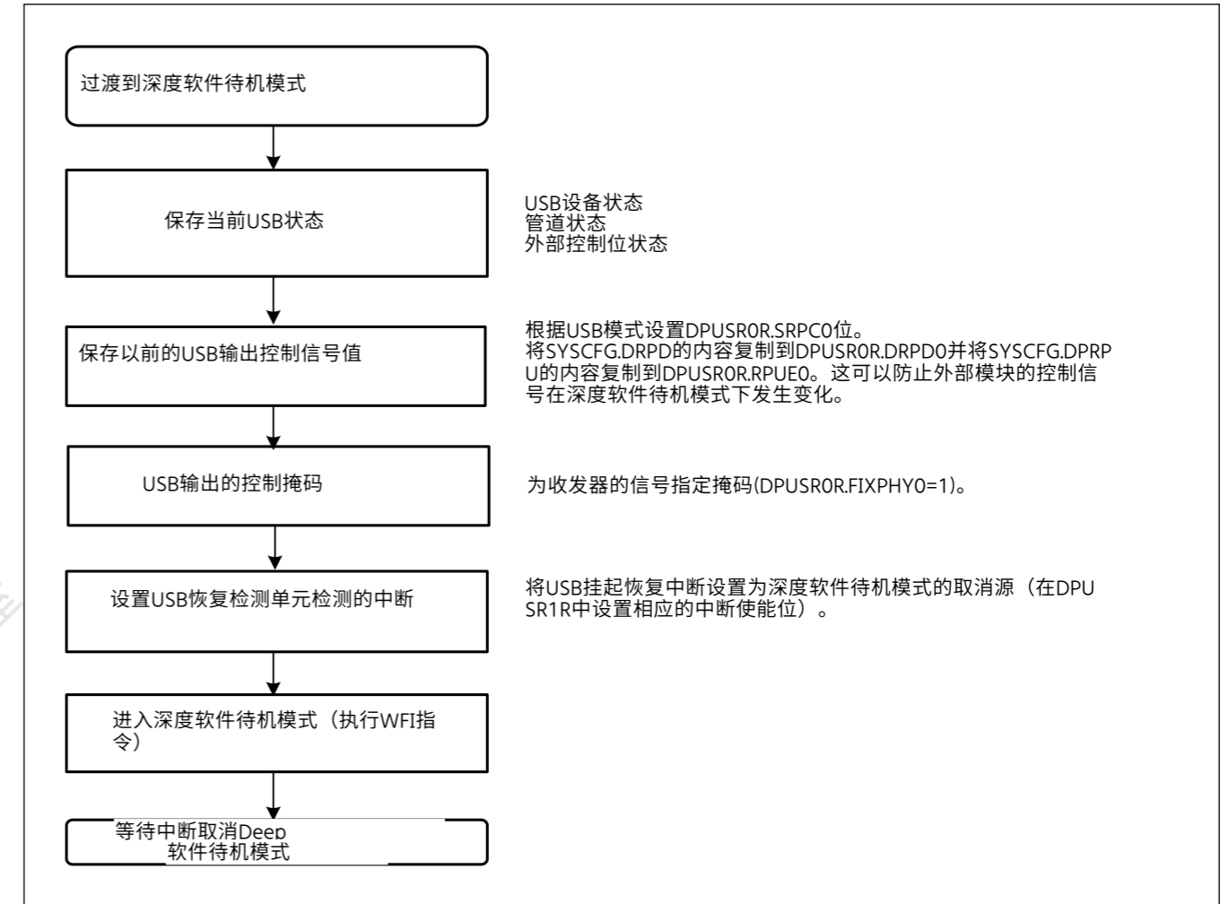
Figure 26.8 作为主机或设备控制器转换到深度软件待机模式的USBFS设置流程
