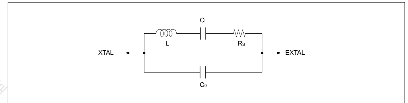
Figure 8.3 晶体谐振器的等效电路
