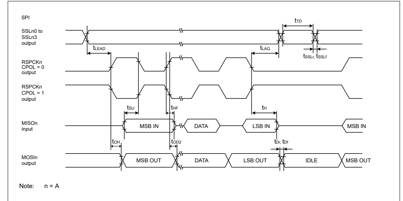
Figure 47.38 当CPHA=1且比特率设置为PCLKA/2时, 主机的RSPi时序
