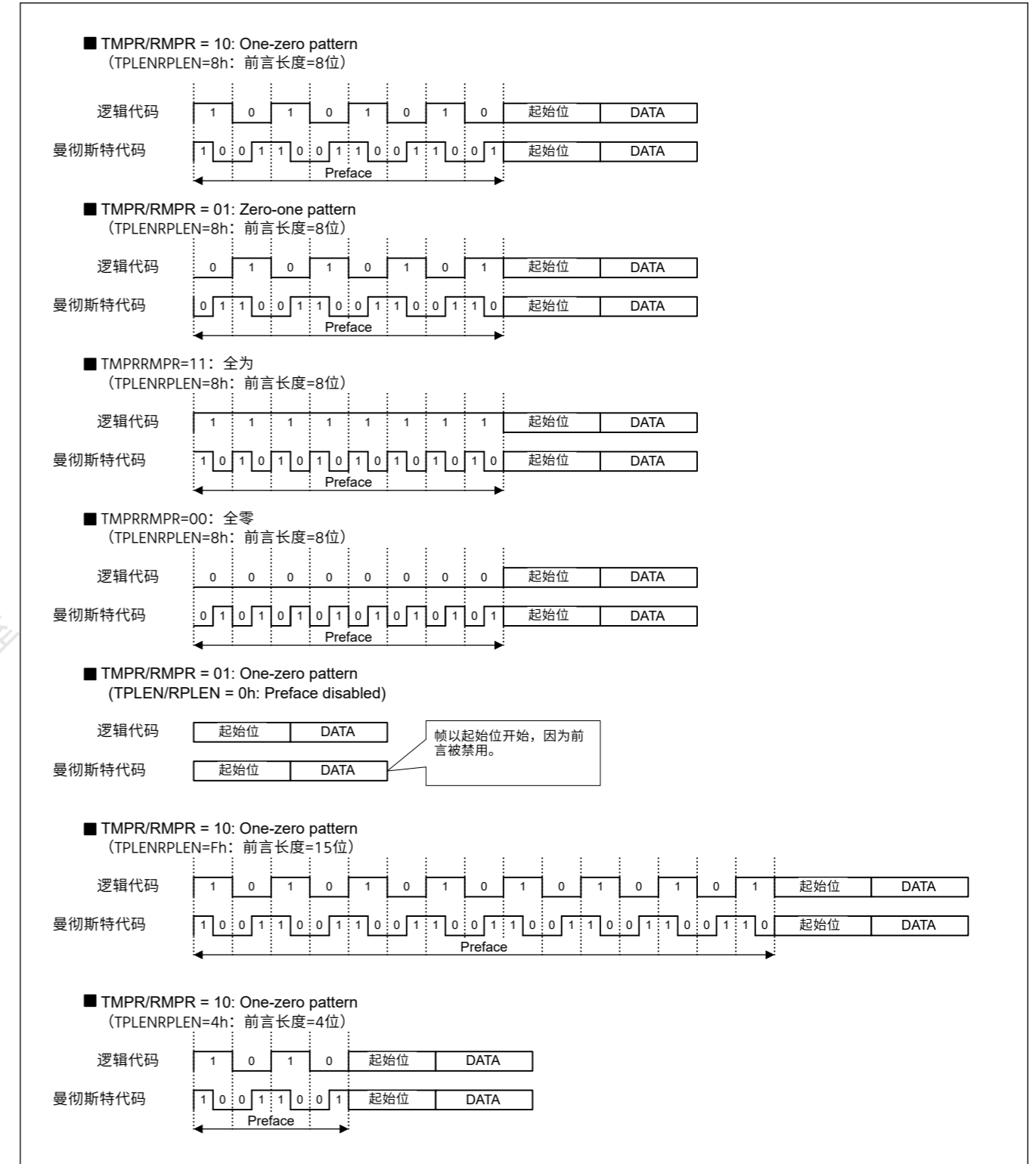
Figure 27.51 前言模式设置示例
