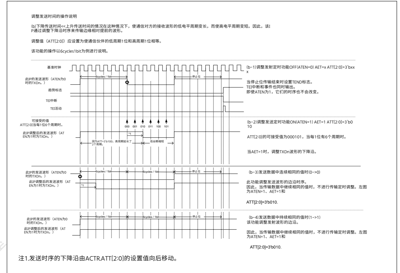
Figure 27.39 AET为1时发射时序调整操作说明
