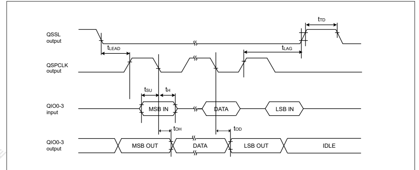
Figure 47.42 发送和接收时序
