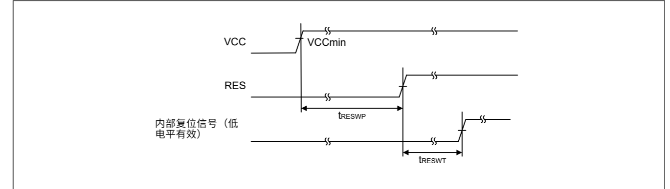
Figure 47.12 VCC超过V POR 电压阈值条件下的RES引脚输入时序
