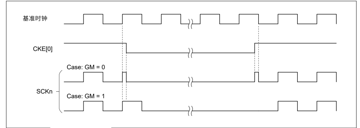
Figure 27.87 时钟输出时序
