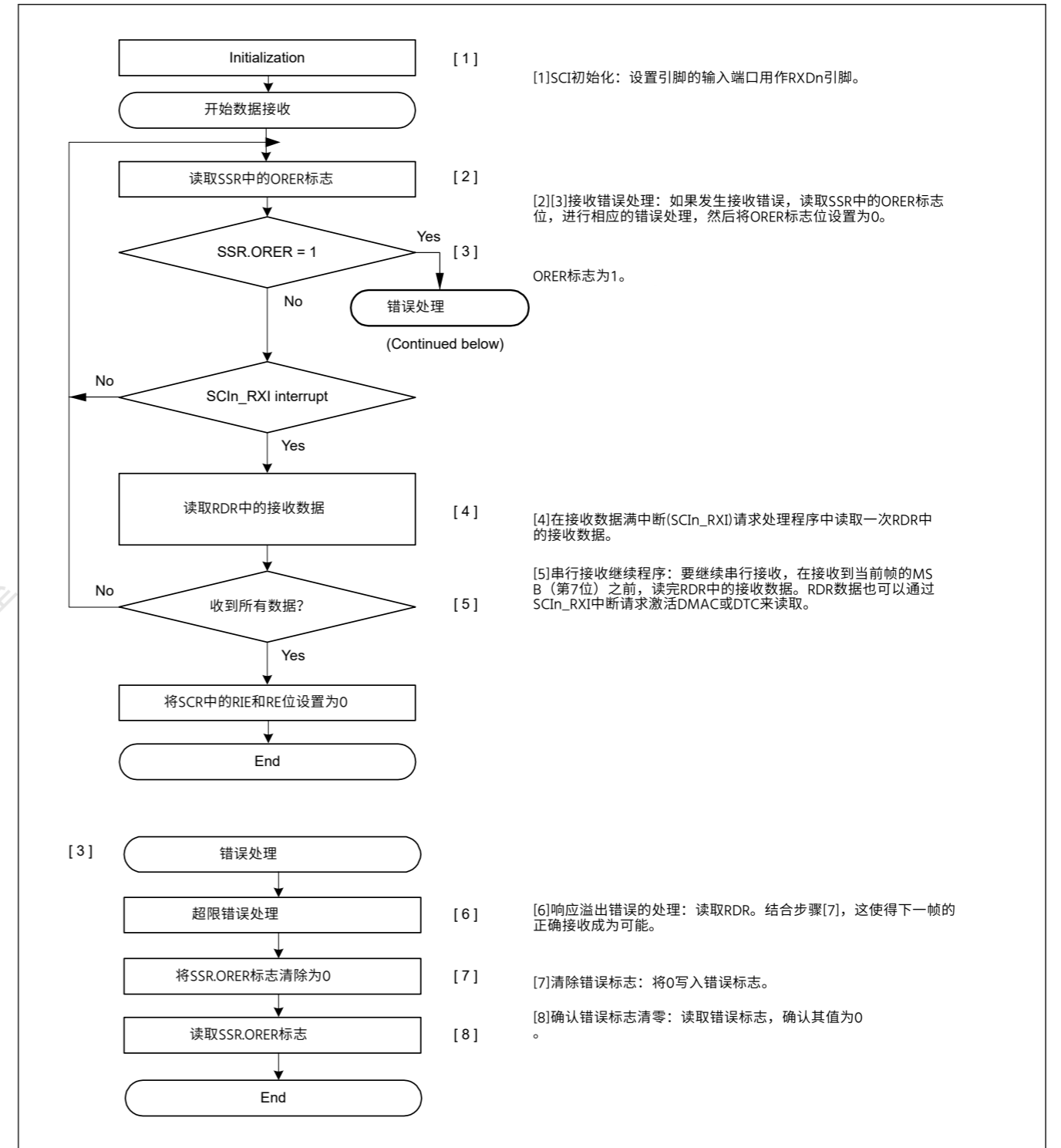
Figure 27.73 选择非FIFO的时钟同步模式下的串行接收示例流程
