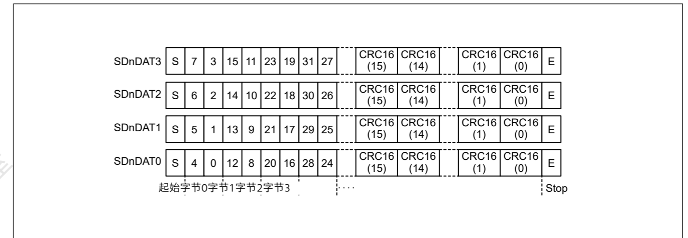
Figure 33.3 SDnDAT在4位宽模式下
