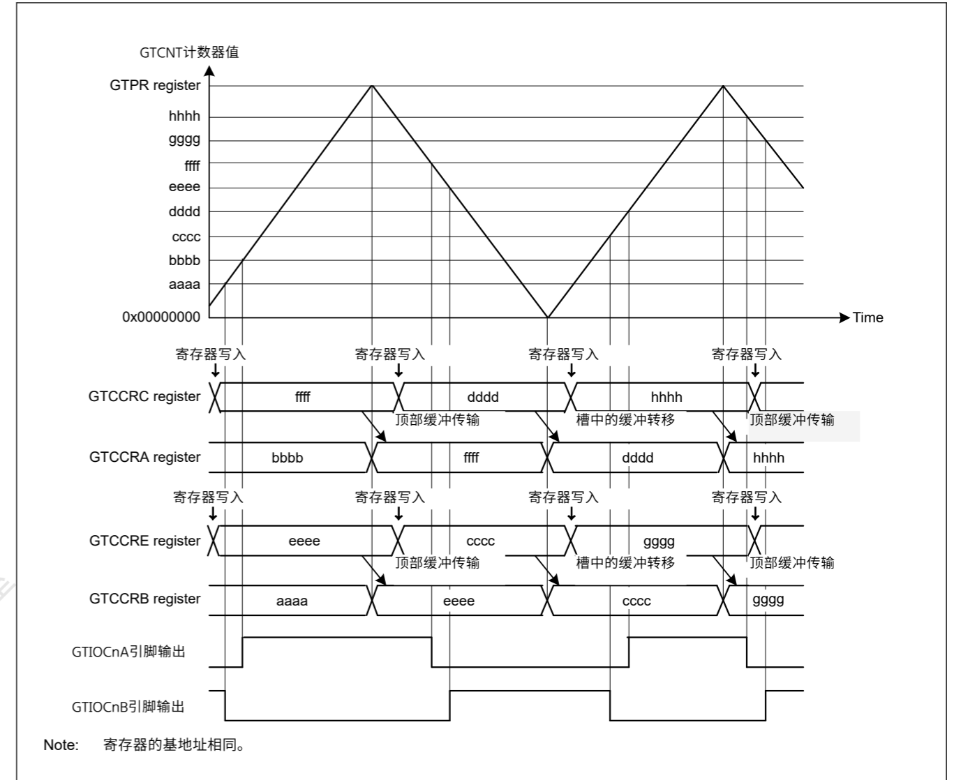
Figure 21.22 带缓冲操作的三角波PWM模式2操作示例，从GTIOCnA引脚和GTIOCnB引脚在计数开始时的高电平输出，输出在GTCCRA/GTCCRB比较匹配，并在循环结束时保留输出
