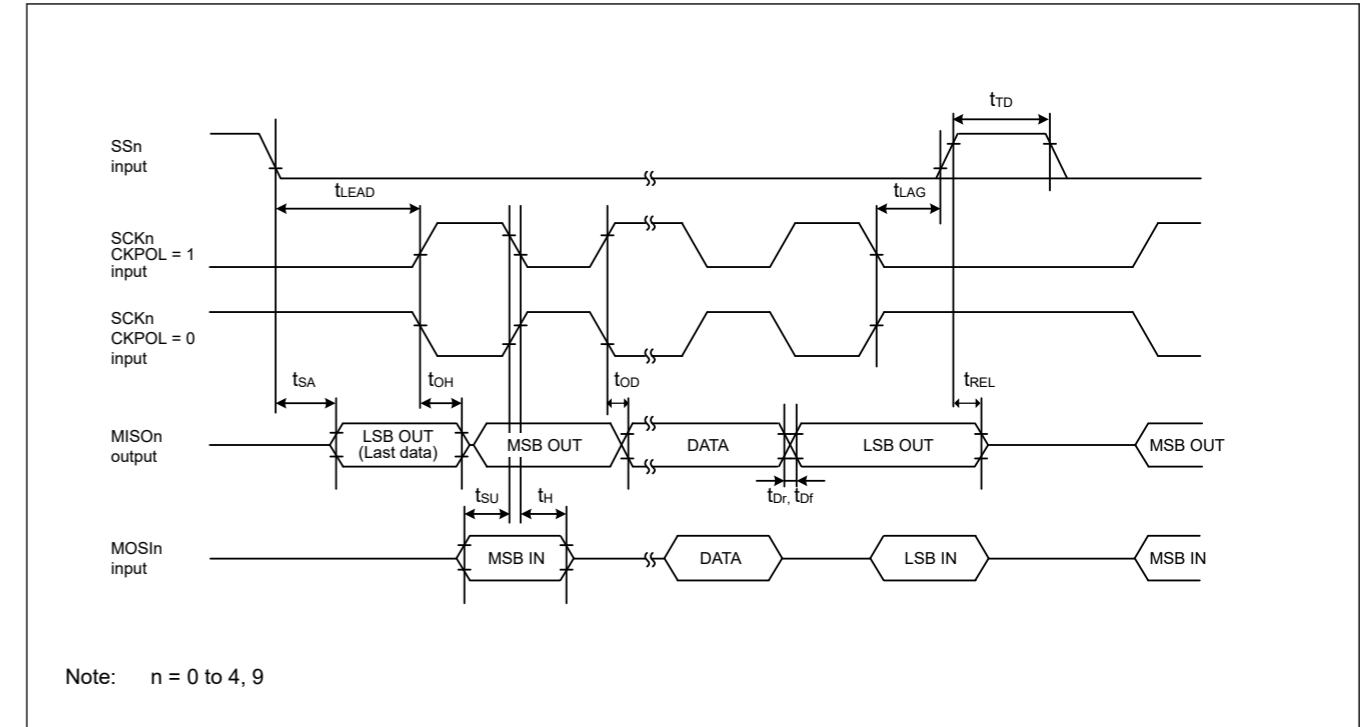
Figure 47.32 CKPH=0时从机的SCI简单SPI模式时序
