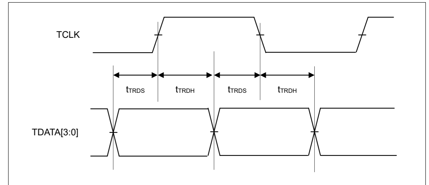
Figure 47.71 ETM输出时序
