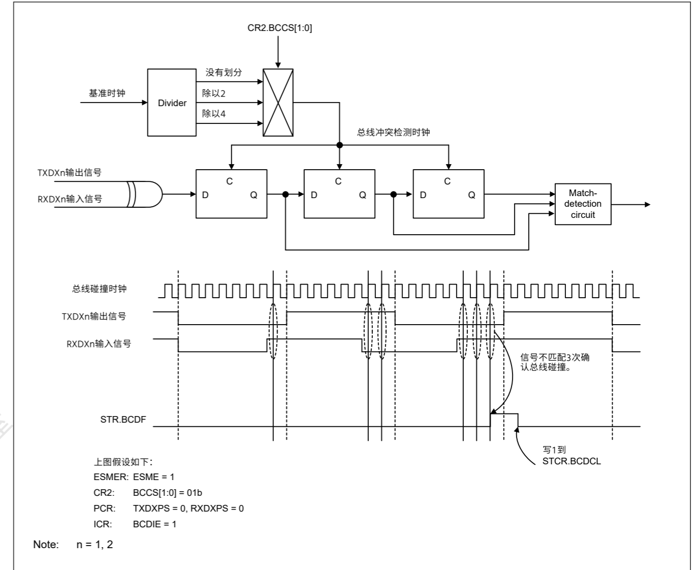
图27.111 带有总线冲突检测的操作示例
