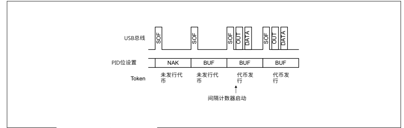
Figure 26.17 IITV=0时的代币发行
