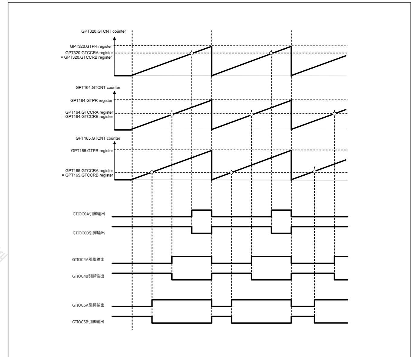
Figure 21.40 三相锯齿波互补PWM输出示例
