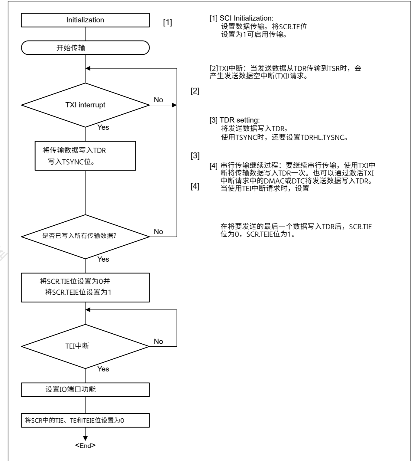
Figure 27.55 曼彻斯特模式下的串行传输流程图示例
