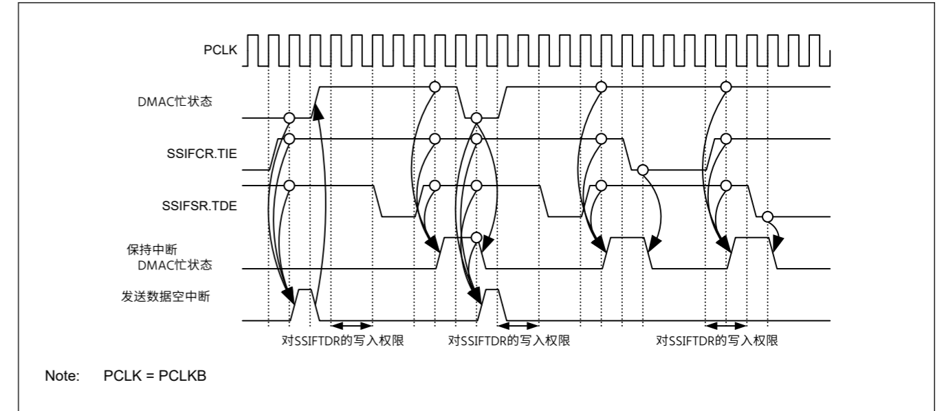
Figure 32.23 发送数据空中断的时序
