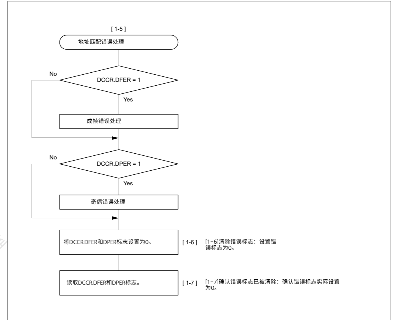
Figure 27.29 异步模式下串行接收的示例流程图 (FIFO选择和地址 Matching Enabled) (2)
