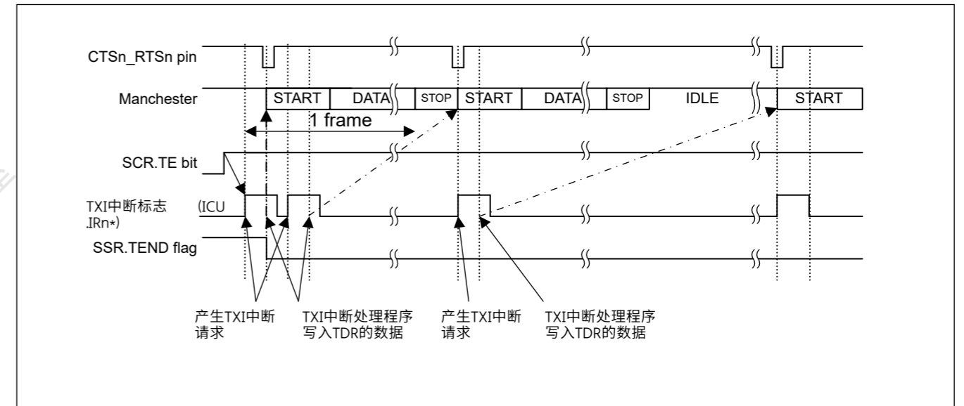
Figure 27.57 曼彻斯特模式下串行传输的传输开始操作示例 (无序但具有CTS功能)
