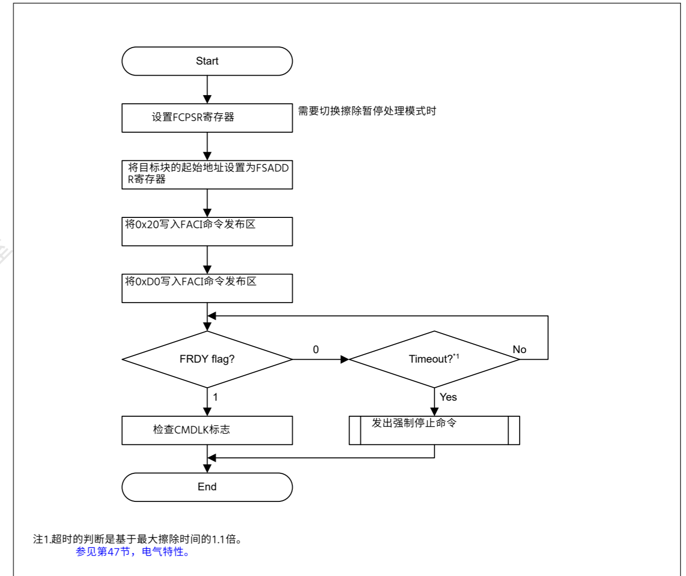
Figure 44.14 块擦除命令的使用流程
