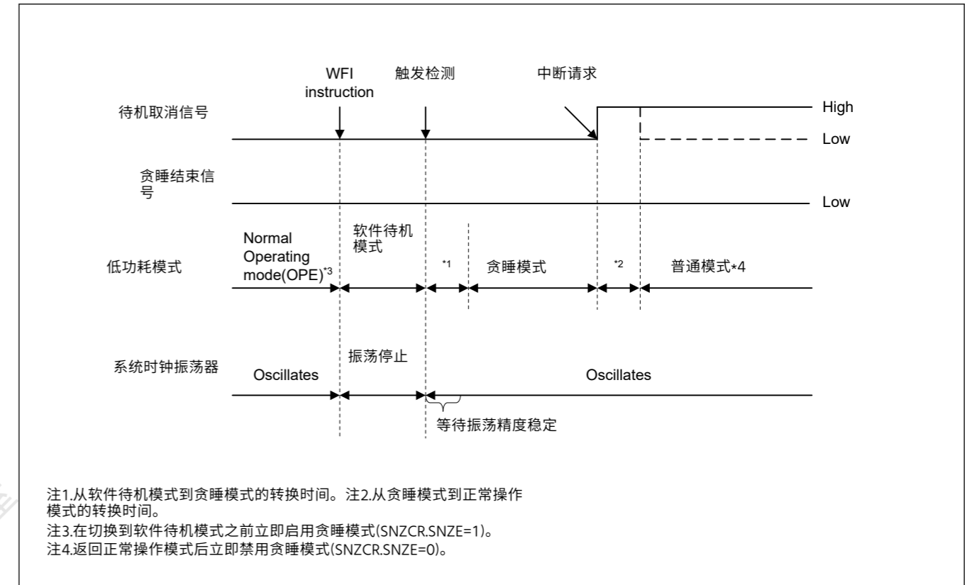
Figure 10.4 产生中断请求信号时取消贪睡模式
