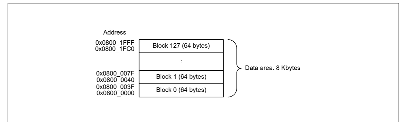
Figure 44.3 数据闪存映射
