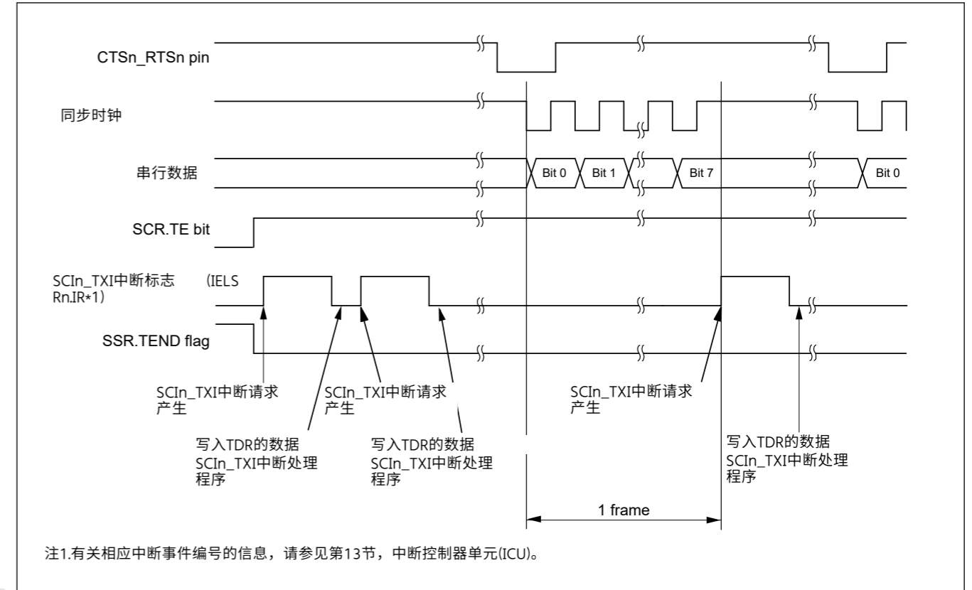
Figure 27.67 传输开始时使用CTS功能时时钟同步模式下的串行数据传输示例
