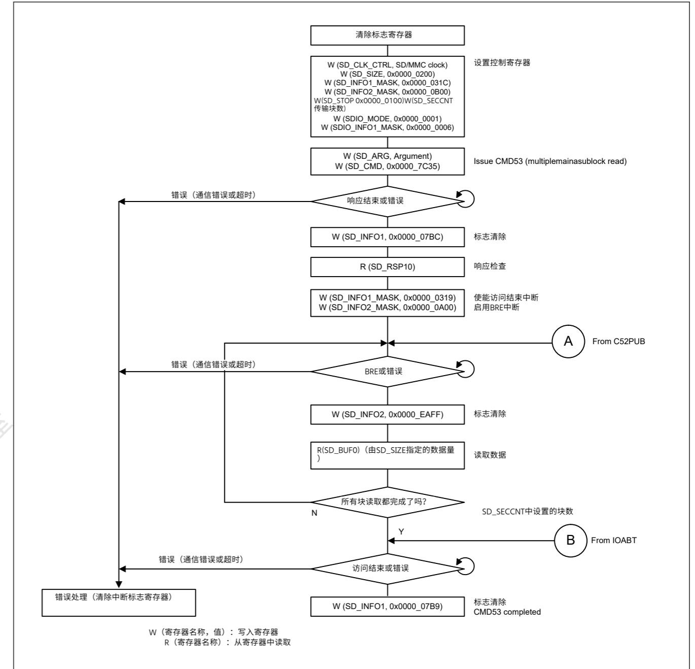
Figure 33.17 用于多块读取操作的IO_RW_EXTENDED命令(CMD53)示例
