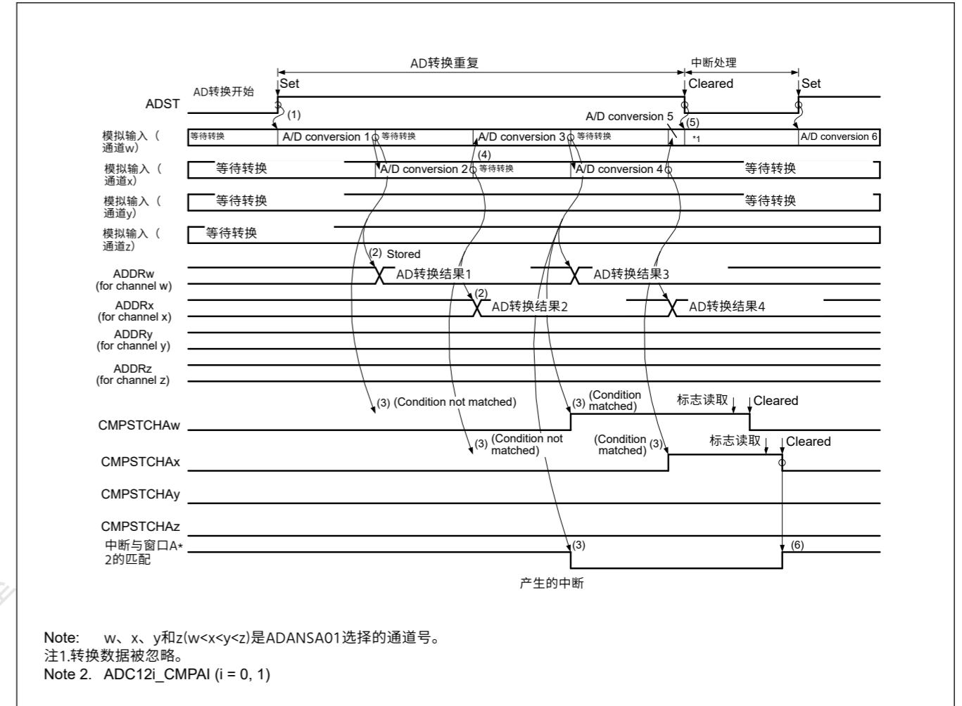
Figure 37.28 比较功能操作示例，比较模拟输入（通道w到z）时
