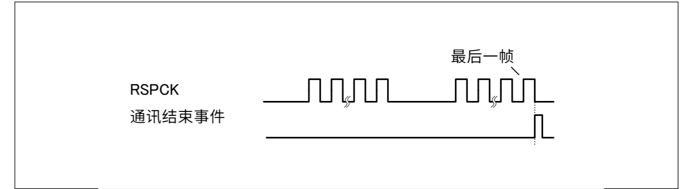
Figure 30.66 通信结束事件输出时序 (仅接收从机模式, 时钟同步 Operation)
