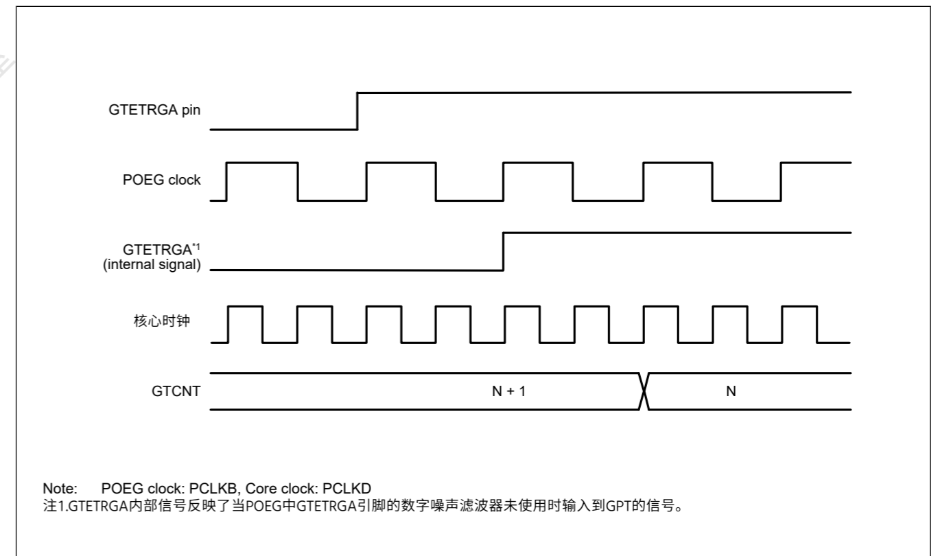
Figure 21.6 使用硬件源递减计数中的事件计数操作示例
