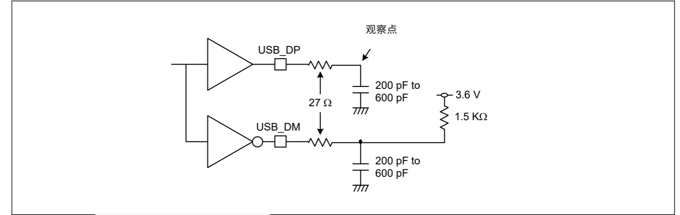
Figure 47.51 低速模式下的测试电路
