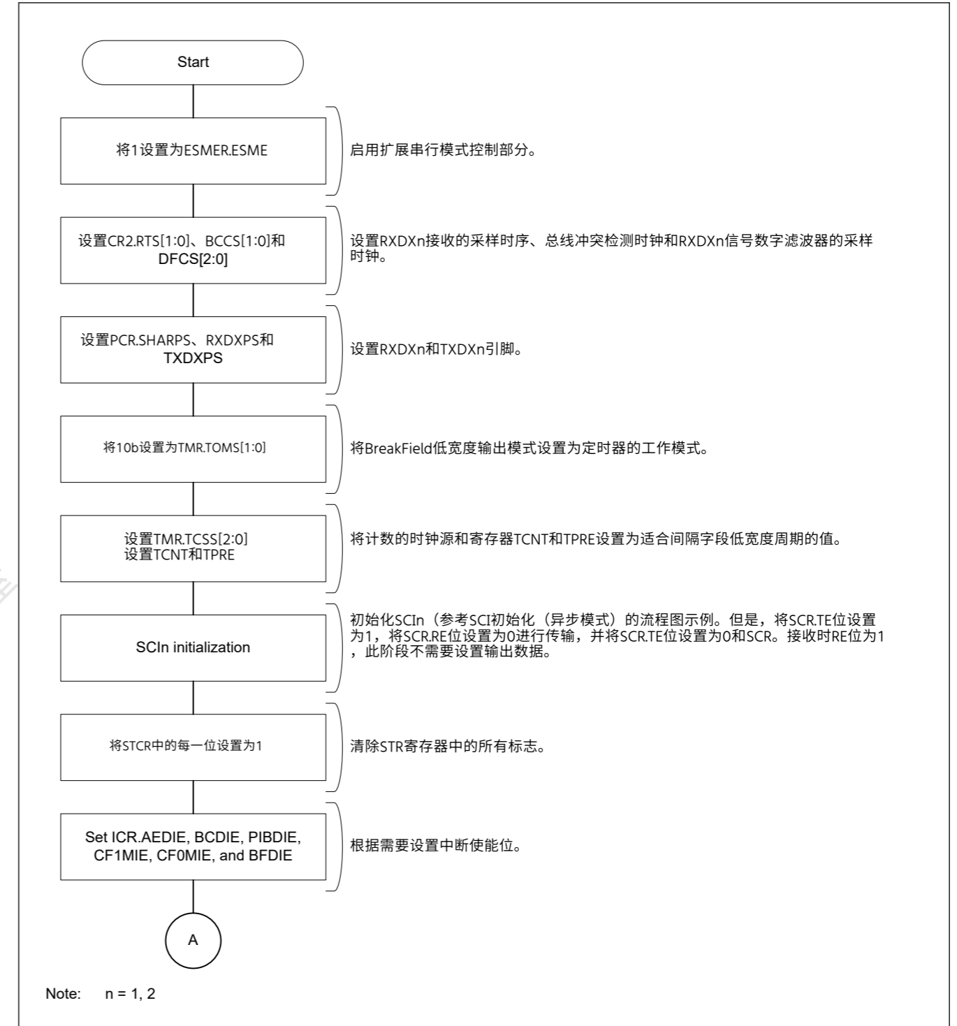
图27.103起始帧传输示例(1/2)
