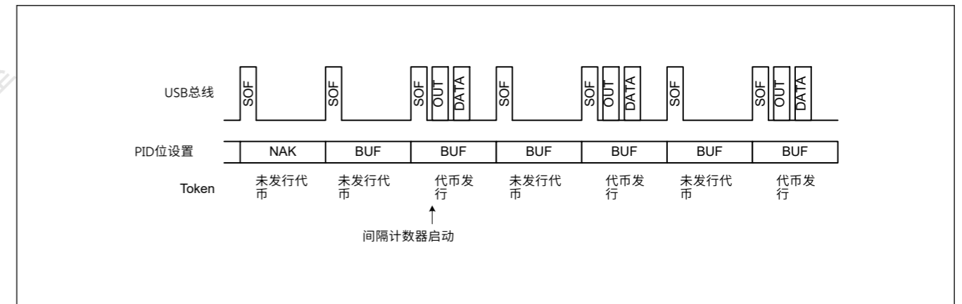
Figure 26.18 IITV=1时的代币发行
