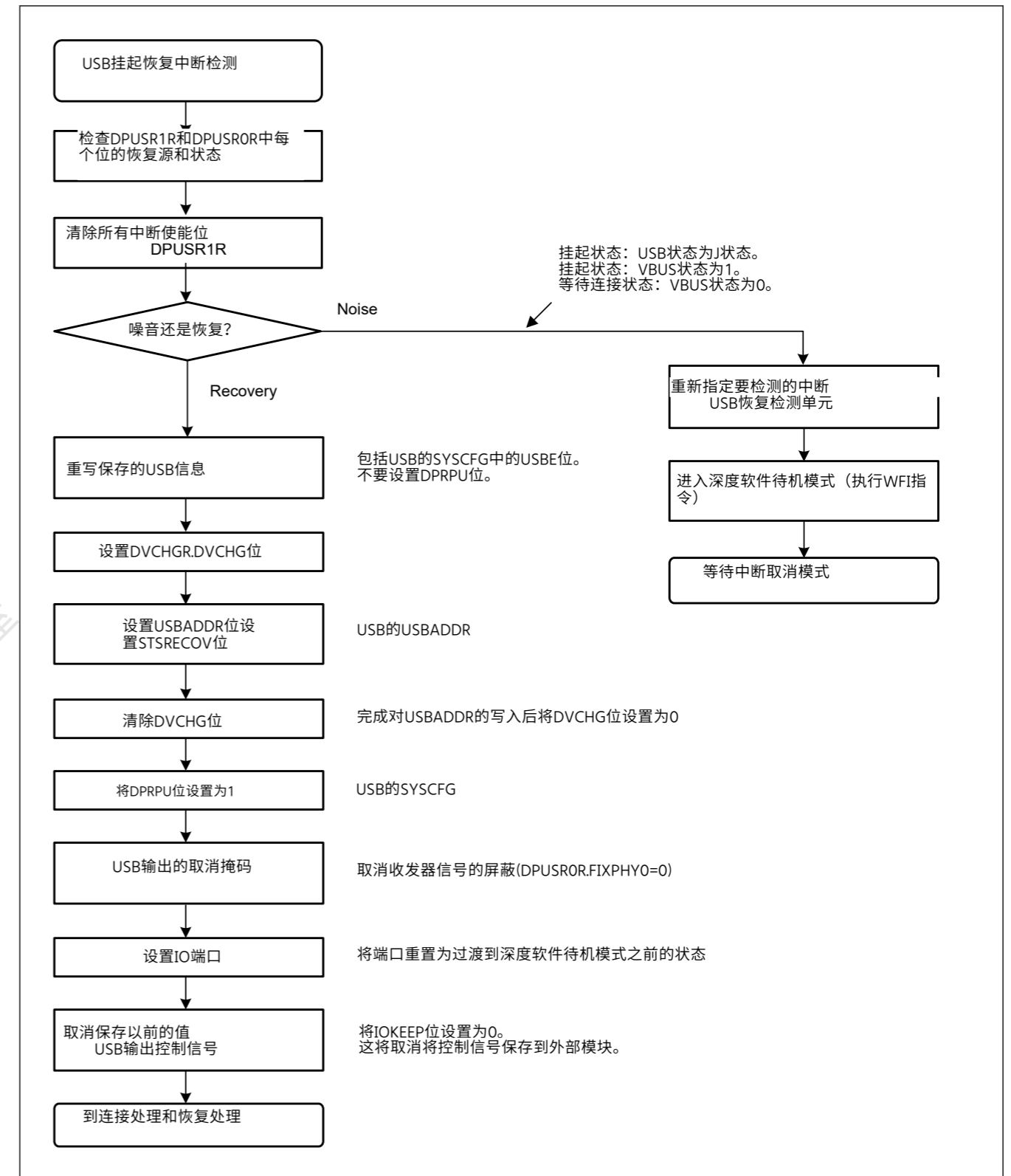
Figure 26.10 用于取消作为设备控制器的深度软件待机模式的USBFS设置流程
