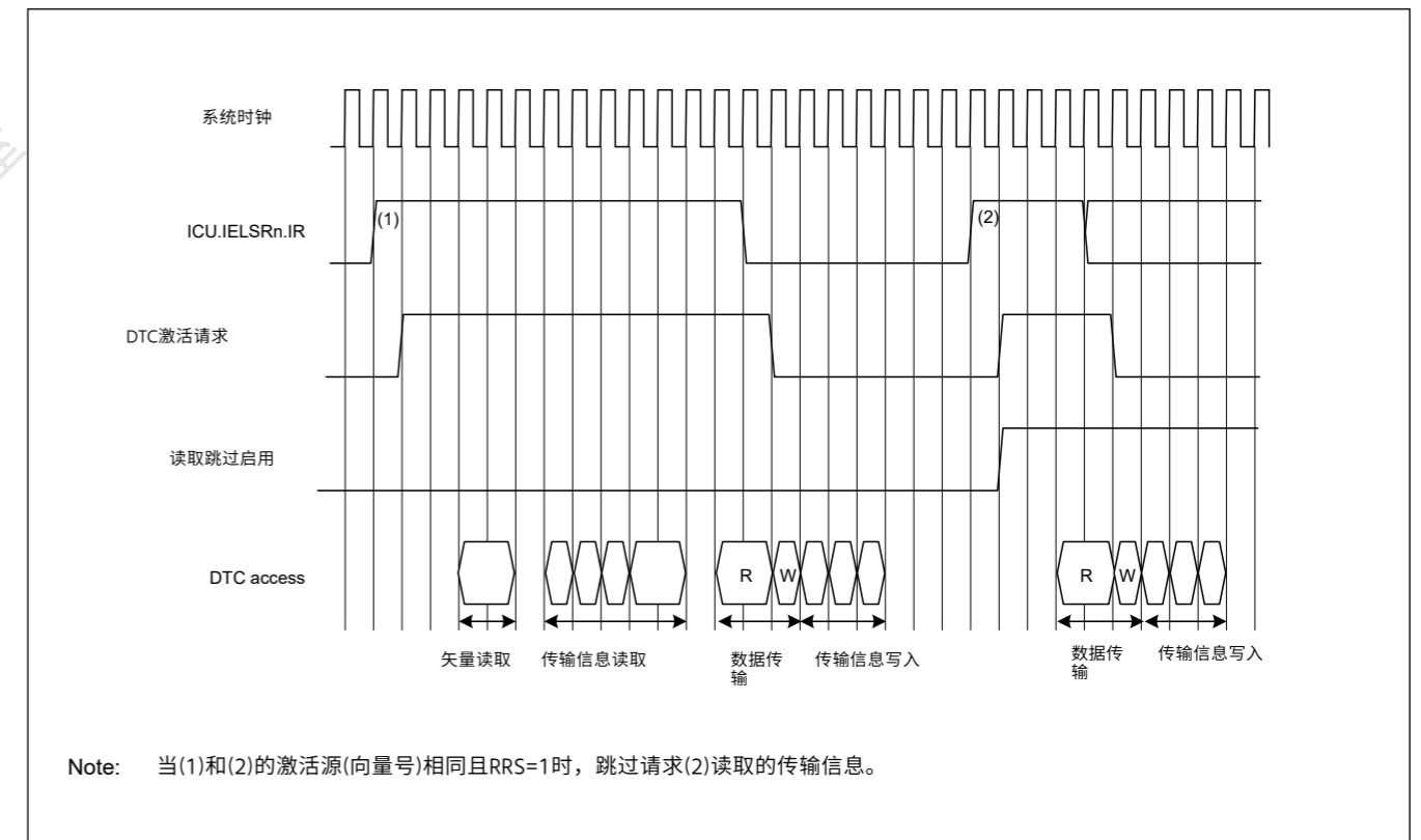
Figure 17.12 使用SRAM上的向量、传输信息和传输目标数据以及外围模块上的传输源数据跳过传输信息读取时的操作示例
