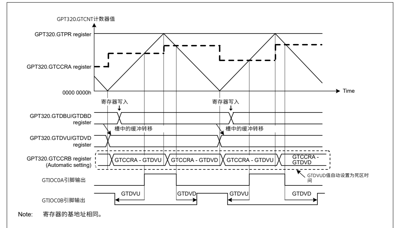
Figure 21.27 三角波中带死区时间的自动比较匹配值设置功能示例 PWM模式2或3, 高电平有效
