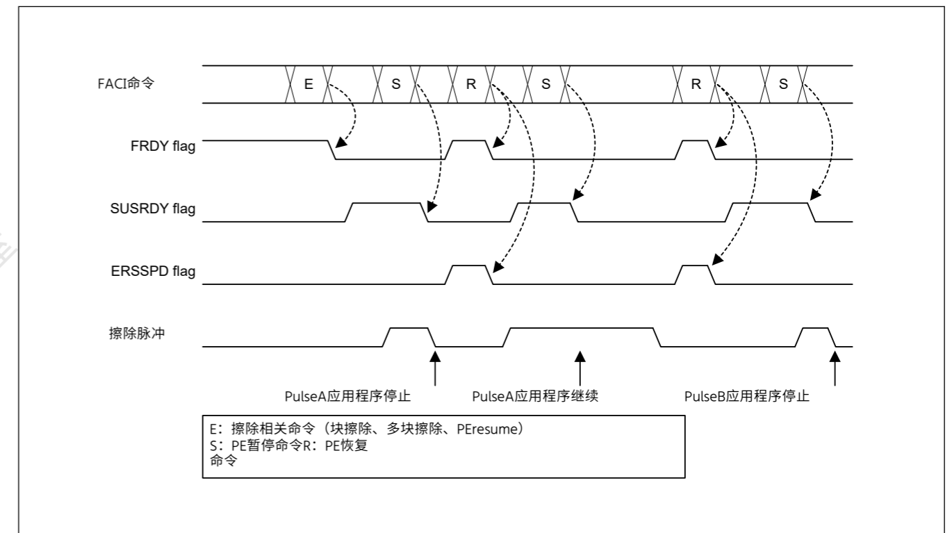
Figure 44.18 擦除期间暂停（暂停优先模式）
