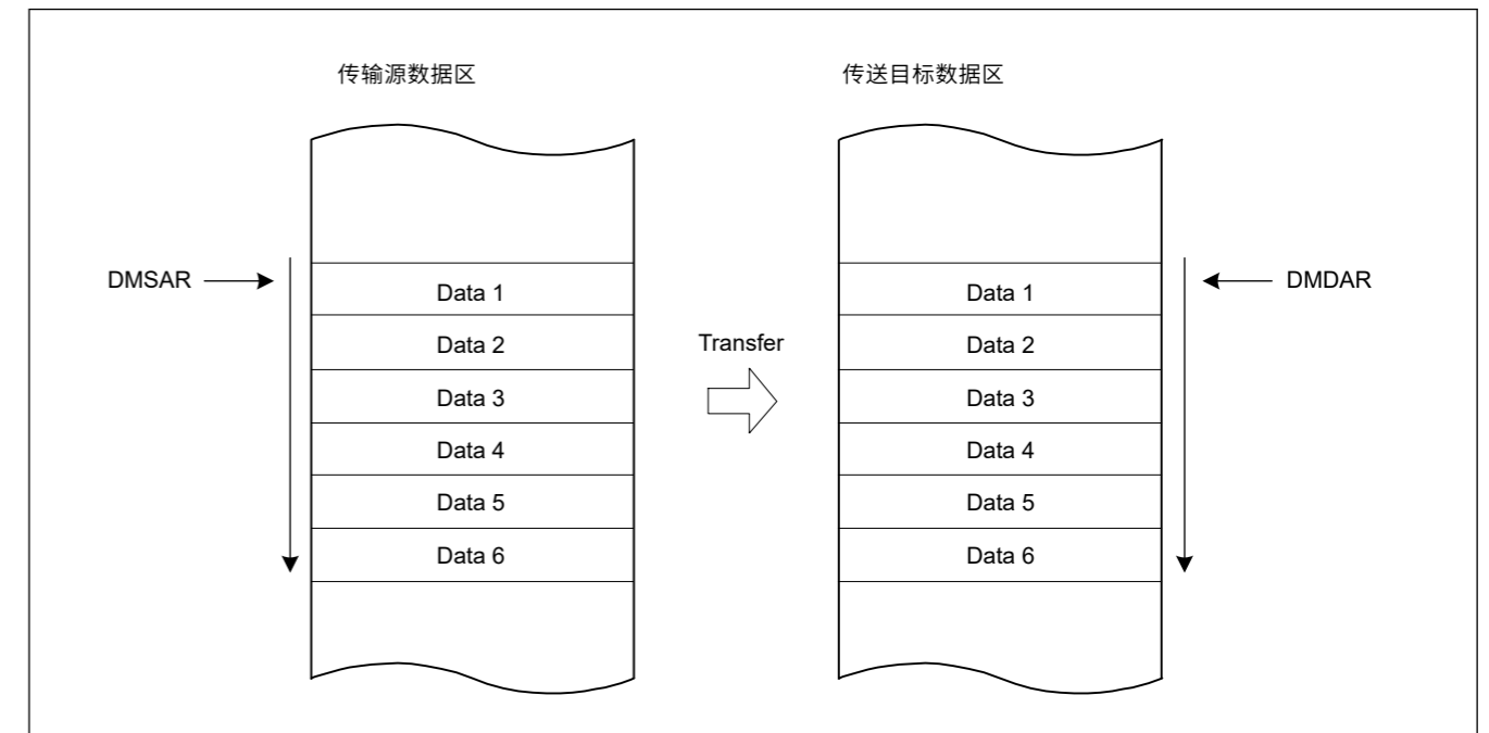
Figure 16.2 正常传输模式下的操作
