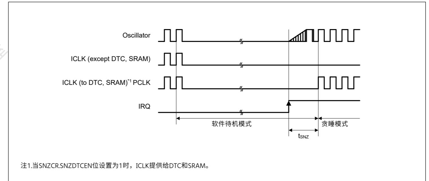
Figure 47.16 从软件待机模式到贪睡模式的恢复时间
