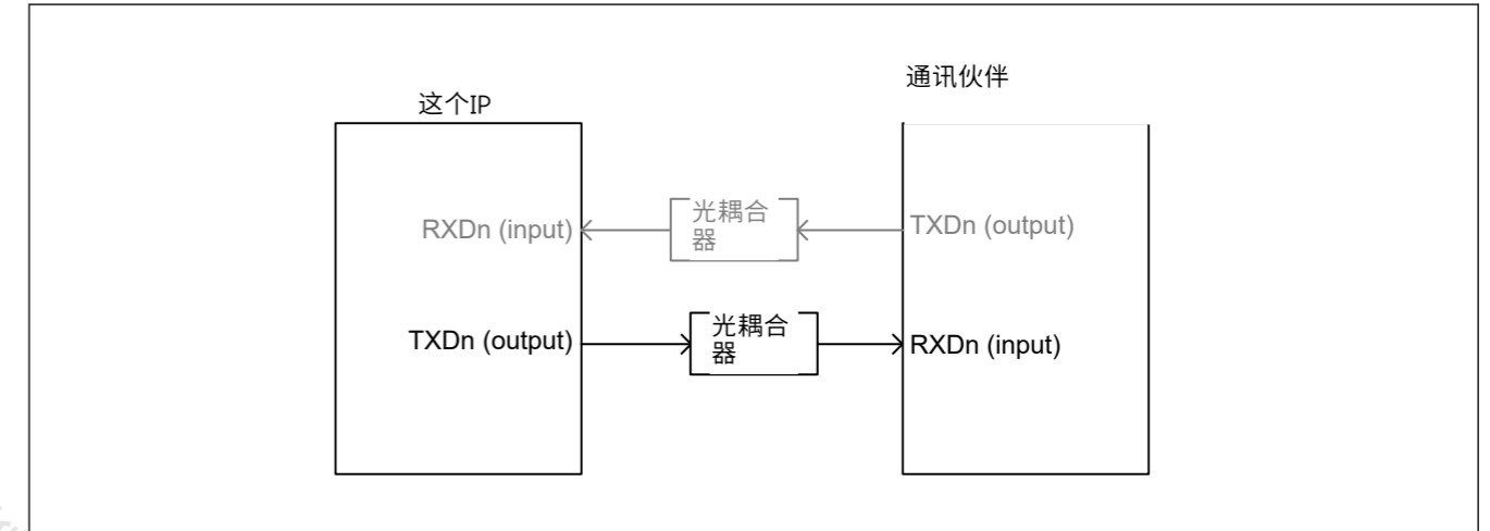
Figure 27.35 通过光耦合器传输的框图图像
