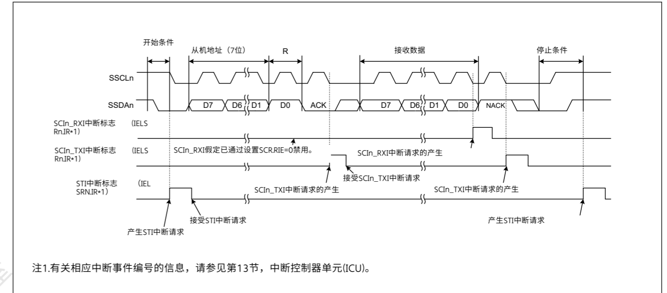
Figure 27.96 使用7位从地址、发送中断和接收中断的简单IIC模式下的主机接收示例操作
