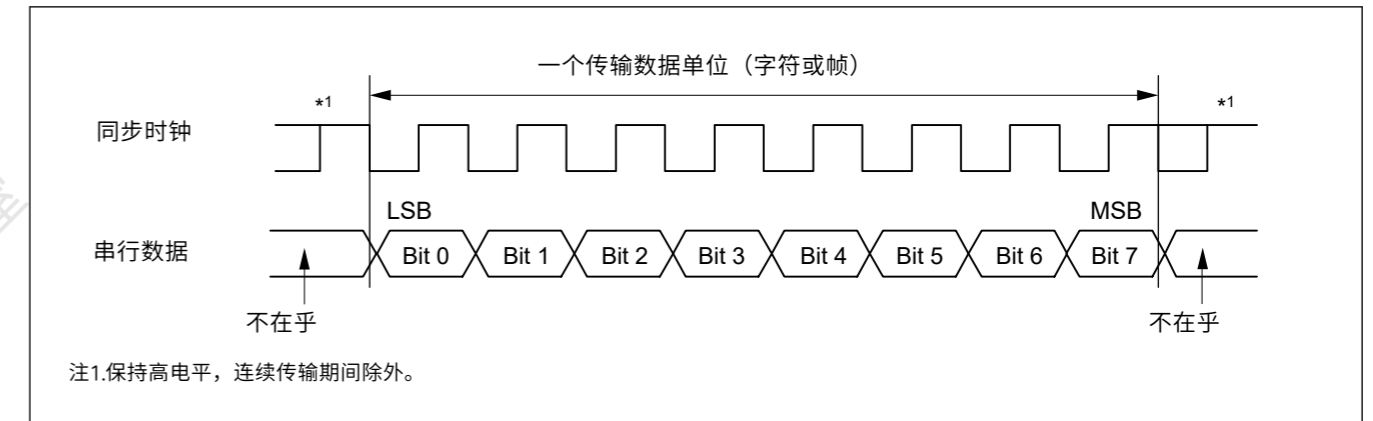
Figure 27.65 具有LSB优先顺序的时钟同步串行通信中的数据格式
