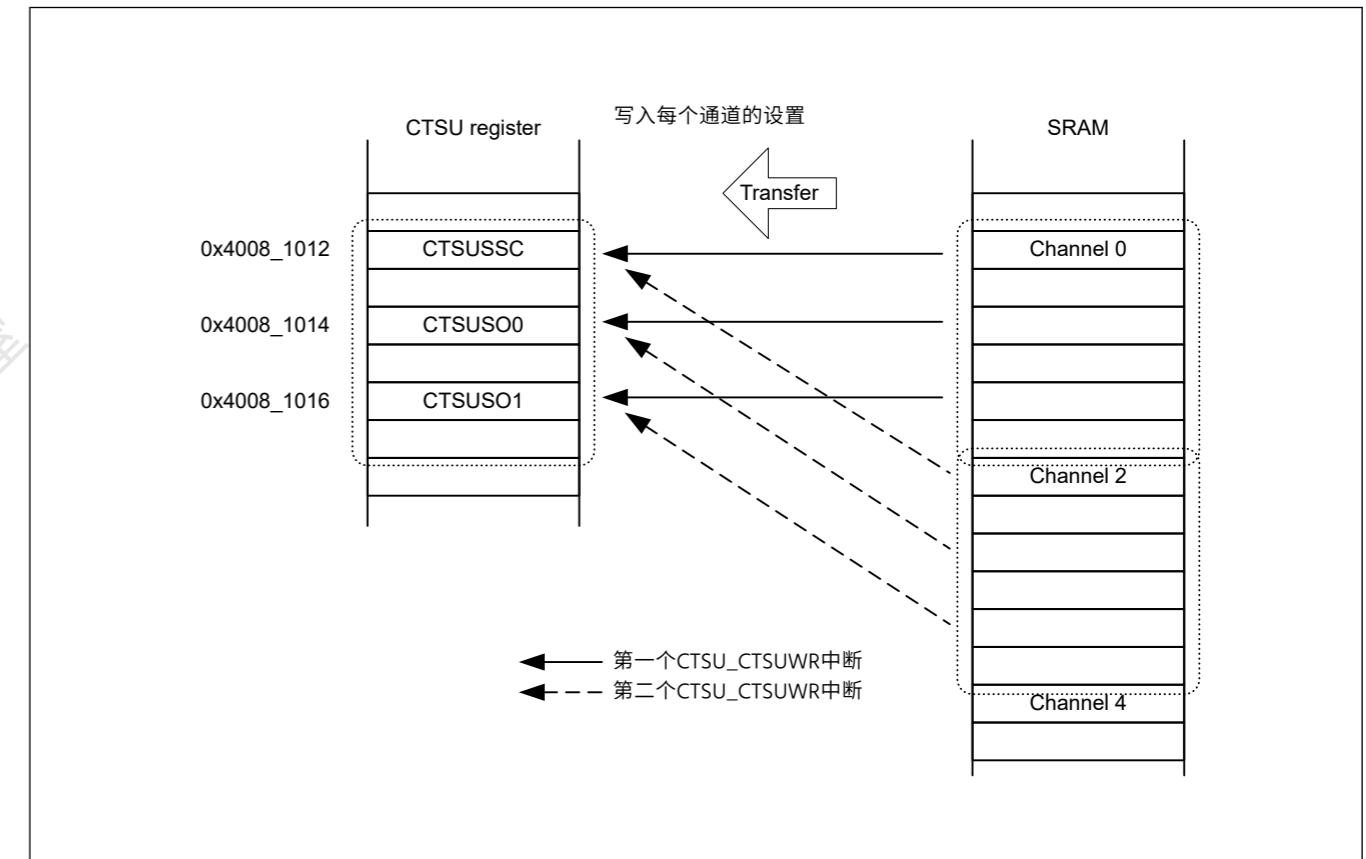
Figure 40.19 使用CTSUSUWR中断的DTC传输操作示例
