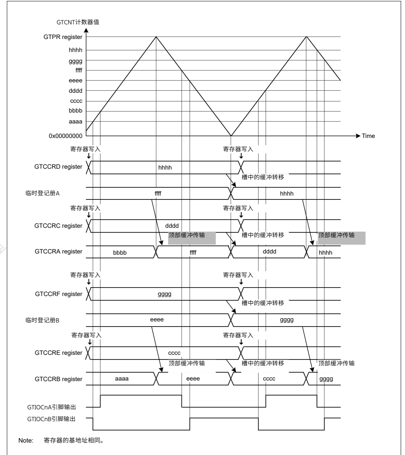
Figure 21.23 三角波PWM模式3操作示例，计数开始时GTIOCnA引脚输出低电平，GTIOCnB引脚输出高电平，在GTCCRAGTCRBB比较匹配时切换输出，并在周期结束时保持输出
