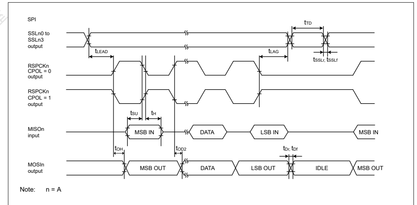
Figure 47.37 CPHA=1时主机的SPI时序
