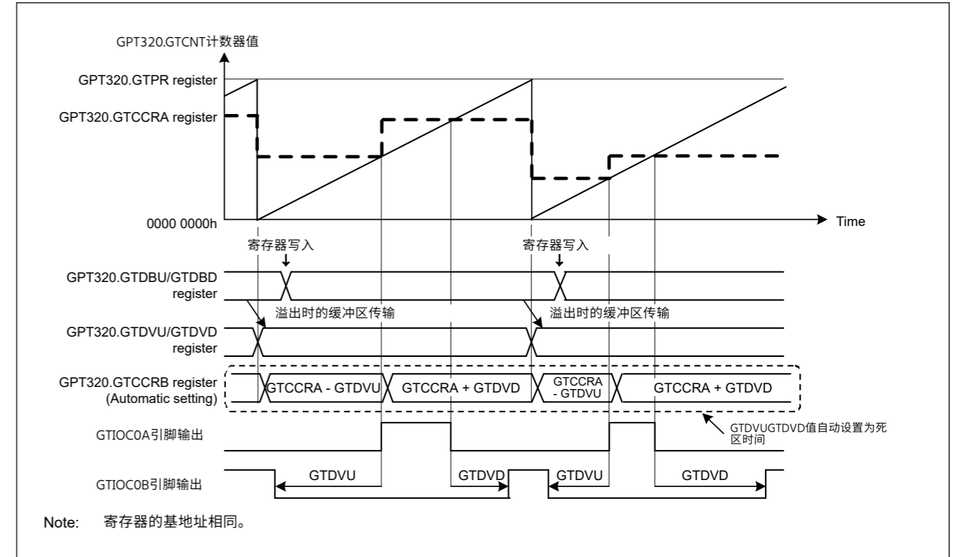
Figure 21.24 锯齿波单发脉冲模式、递增计数和高电平有效的自动死区时间设置功能操作示例
