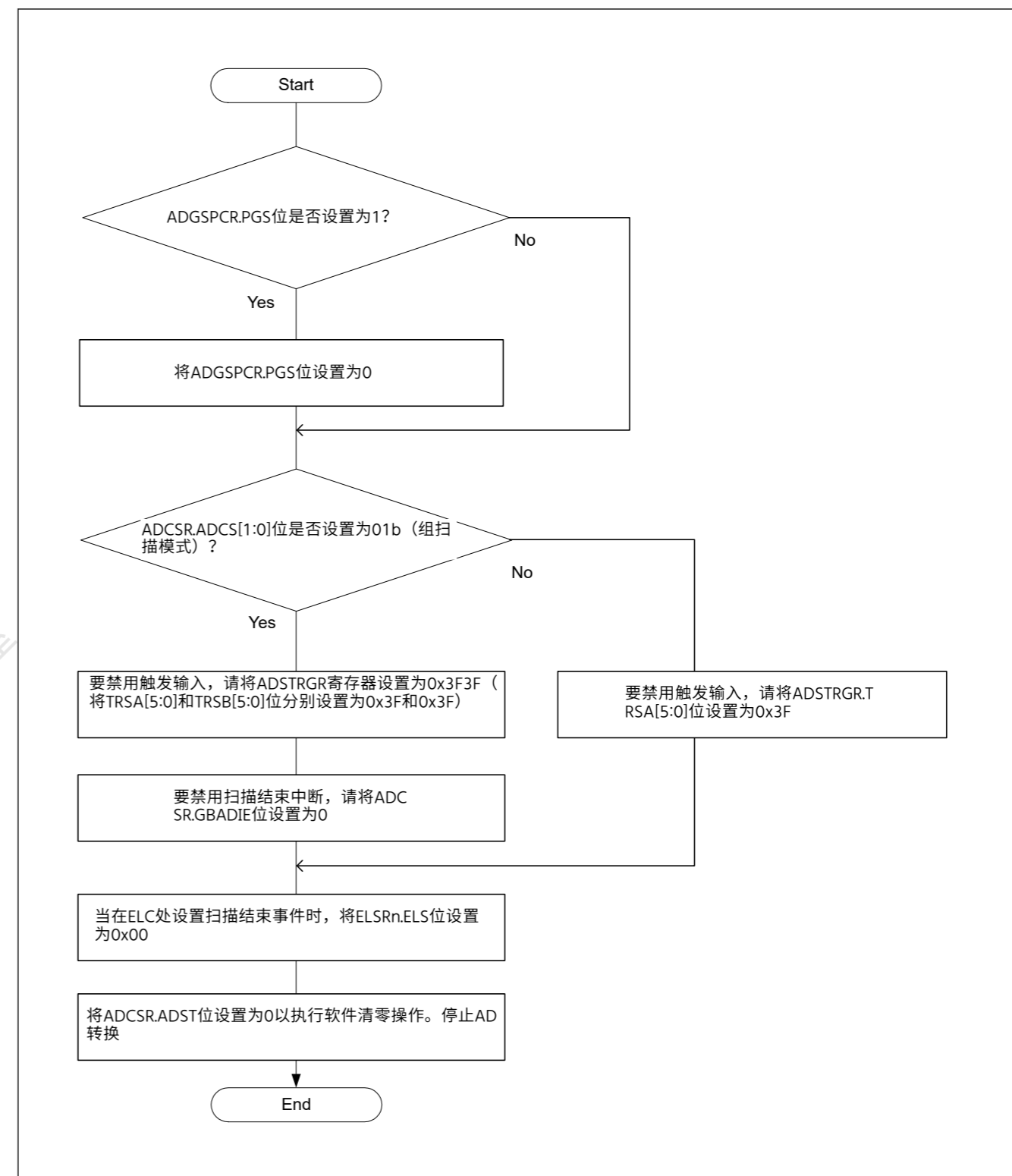
Figure 37.38 通过软件清除ADCSR.ADST位的程序
