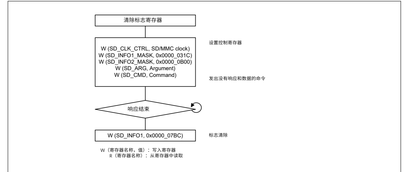
Figure 33.9 没有响应或数据的命令流示例
