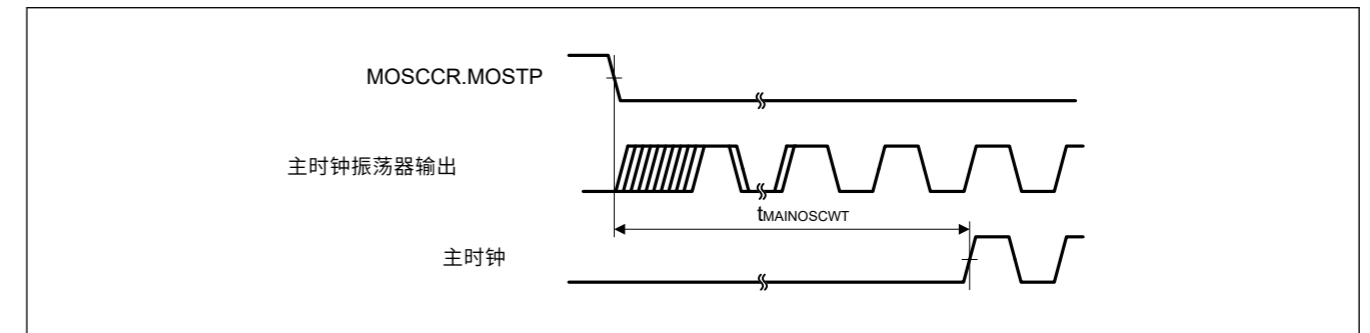
Figure 47.8 主时钟振荡开始时序
