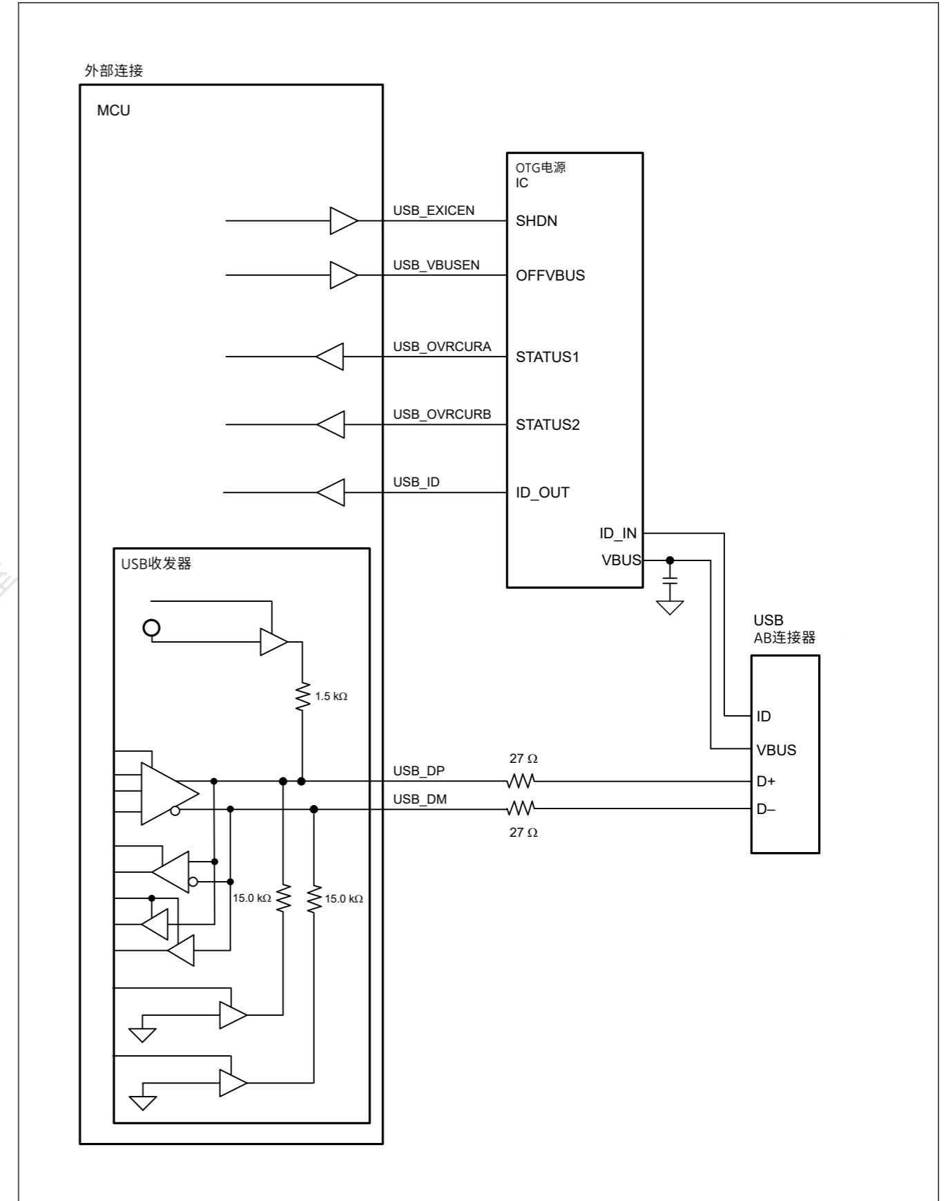
Figure 26.2 自供电系统中的示例OTG连接
