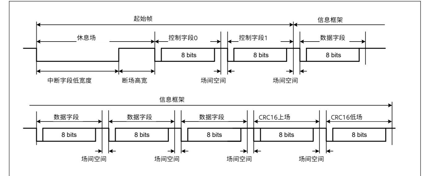
图27.101扩展串行模式控制部分的串行传输协议
