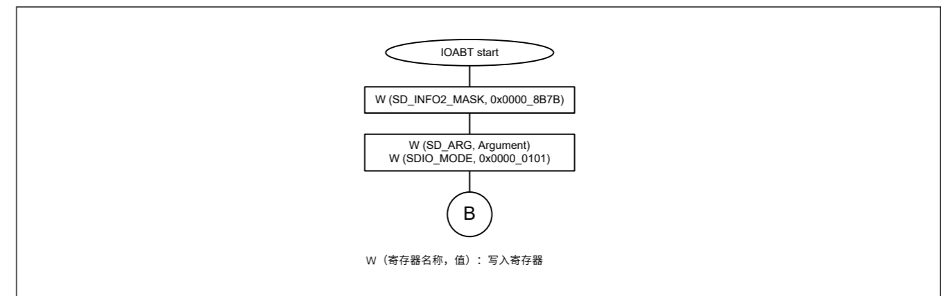
Figure 33.21 在CMD53多块写入期间发出CMD52 (SDIO中止) 时的流程
