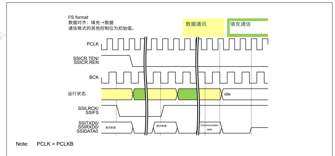
Figure 32.50 停止数据通信 (使用填充位)
