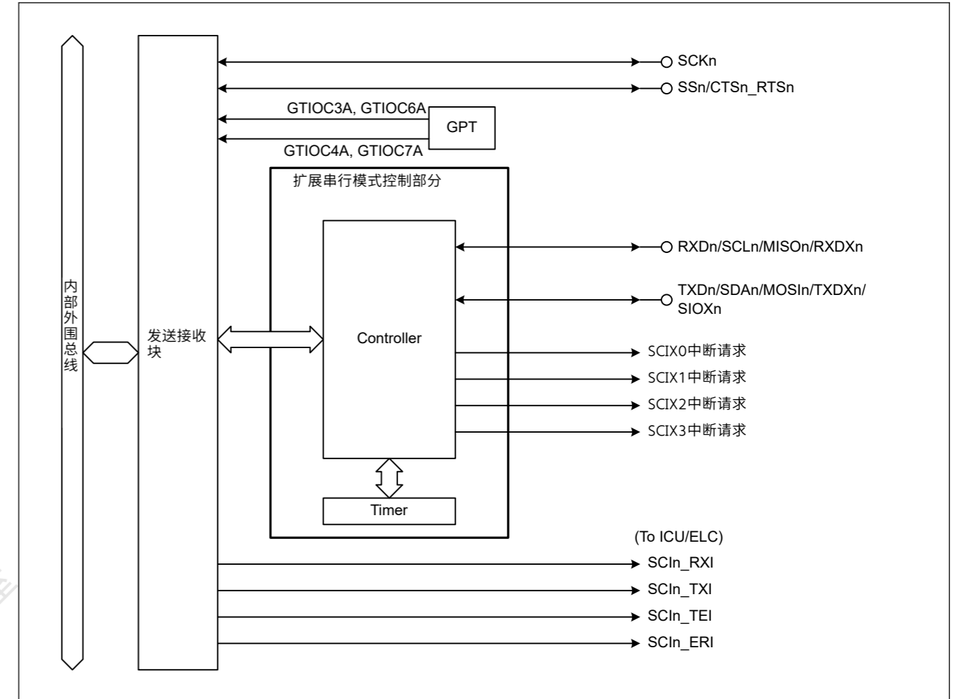
Figure 27.2 SCIn(n=1 2)扩展串行模式控制器框图
