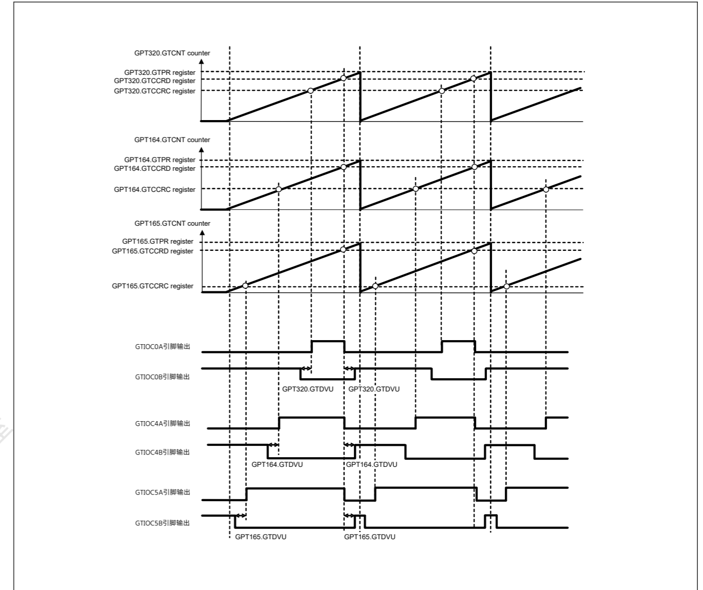
Figure 21.41 具有自动死区时间设置的三相锯齿波互补PWM输出示例
