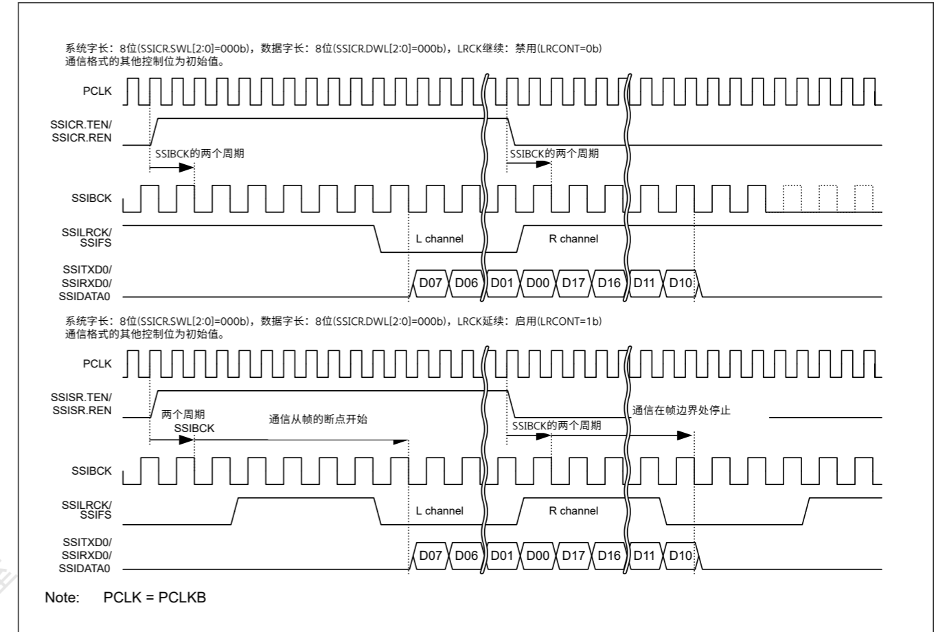
Figure 32.33 LR时钟帧同步继续操作示例
