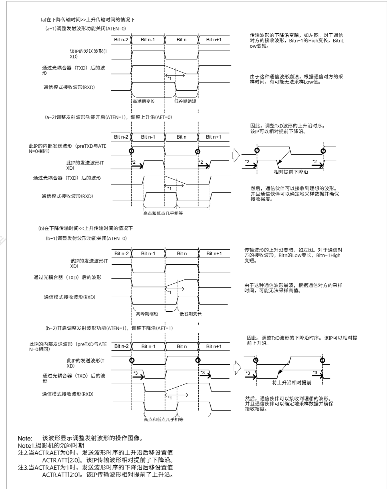
Figure 27.36 通过光电耦合器进行通信的传输运动图像图形
