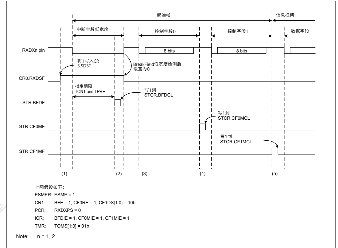
图27.106开始帧接收时的操作示例
