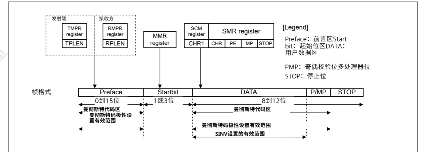
Figure 27.50 曼彻斯特模式下的帧格式
