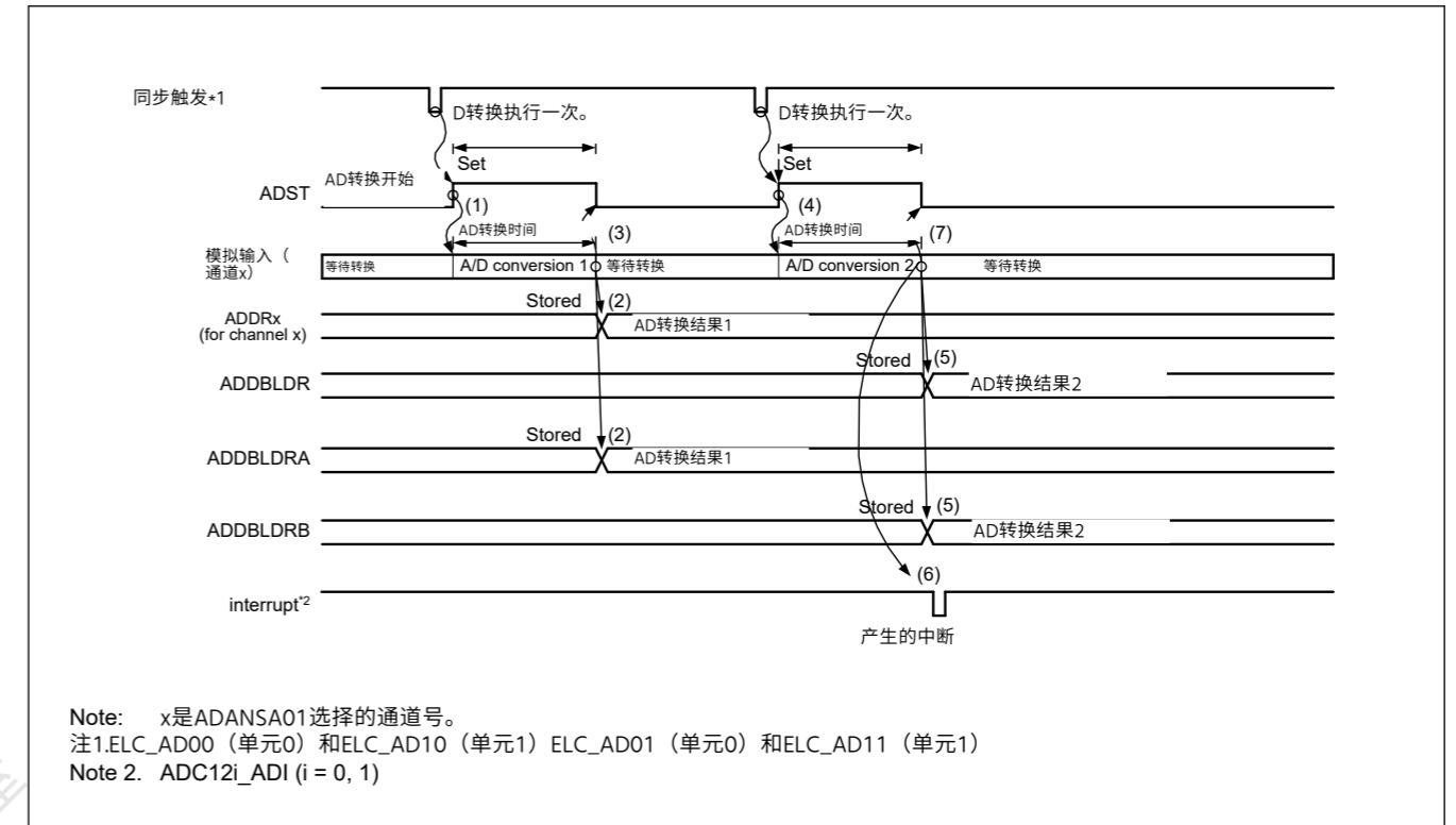
Figure 37.12 双触发模式下的扩展操作示例，为模拟输入（通道x）和ELC_AD00（单元0）和ELC_AD10（单元1）选择了重复ELC_AD01（单元0）和ELC_AD11（单元1）
