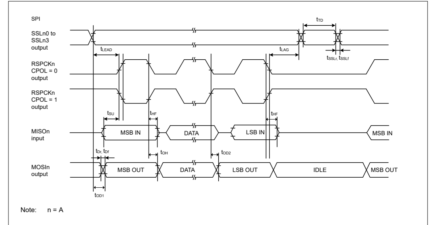
Figure 47.36 当CPHA=0且比特率设置为PCLKA/2时主设备的SPI时序
