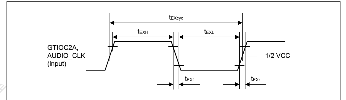
Figure 47.45 时钟输入时序
