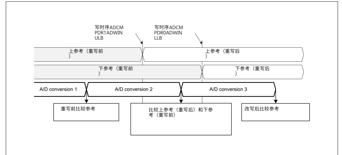
Figure 37.6 重写前后上下引用的比较
