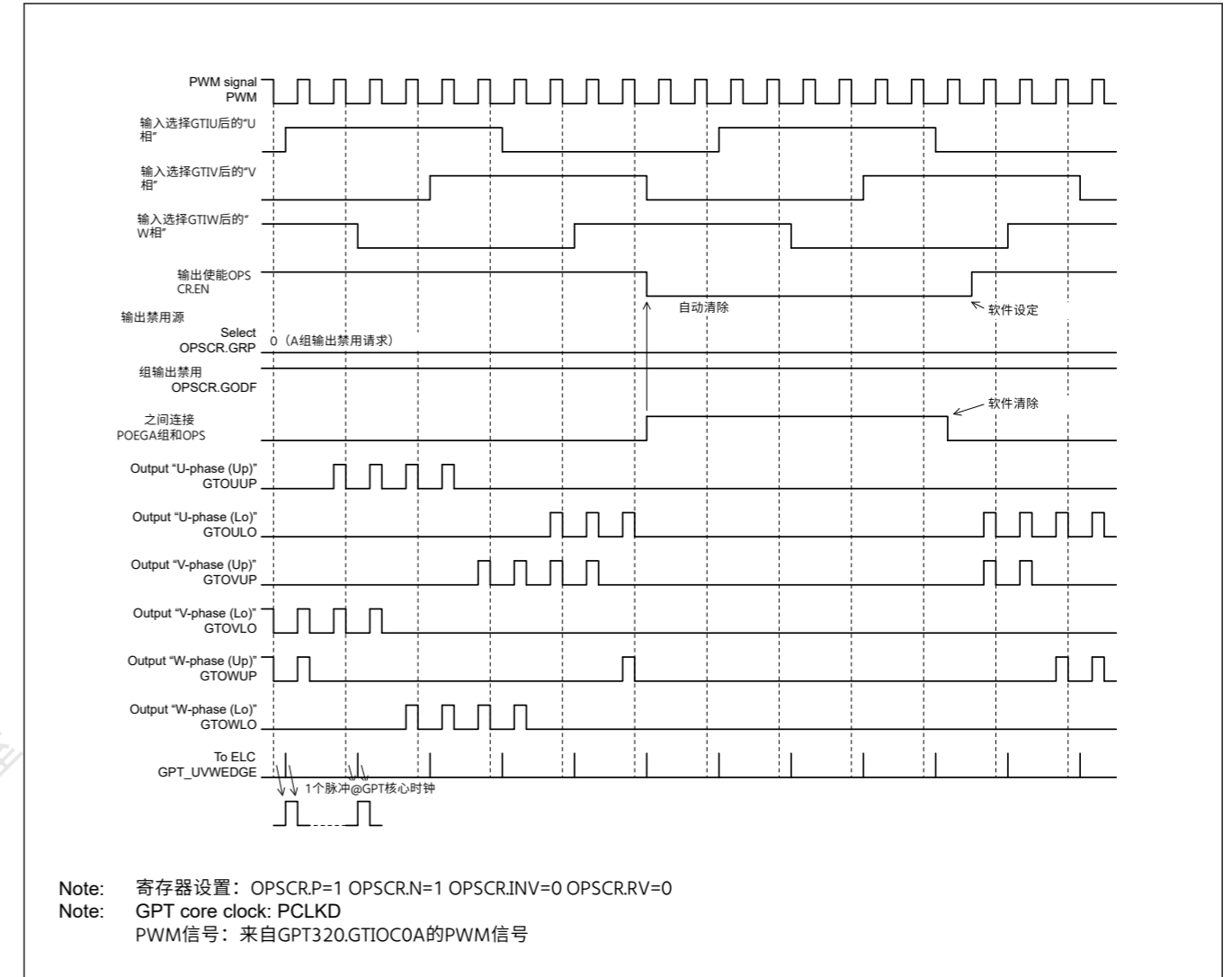
Figure 21.60 组输出禁用控制操作示例
