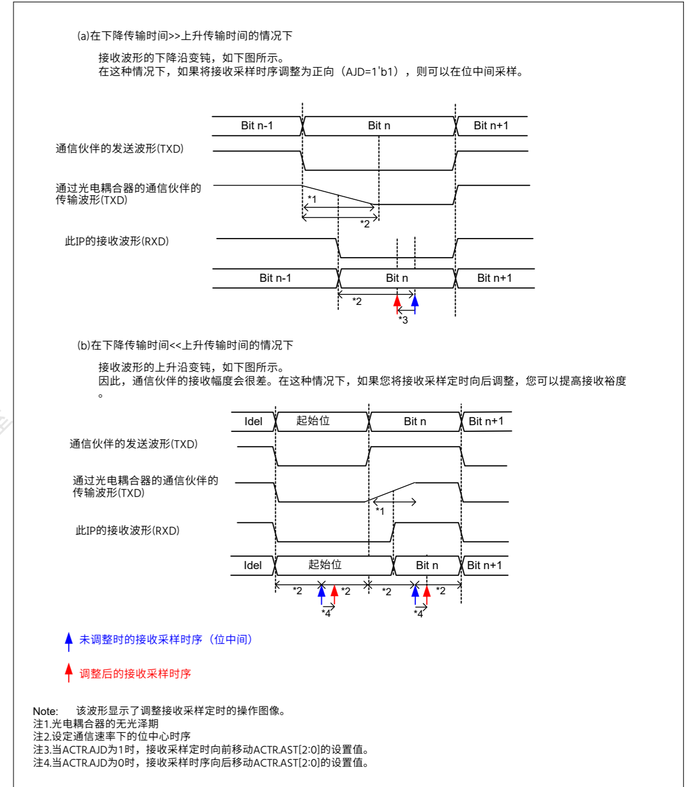
Figure 27.32 通过光电耦合器进行通信的接收运动图像图
