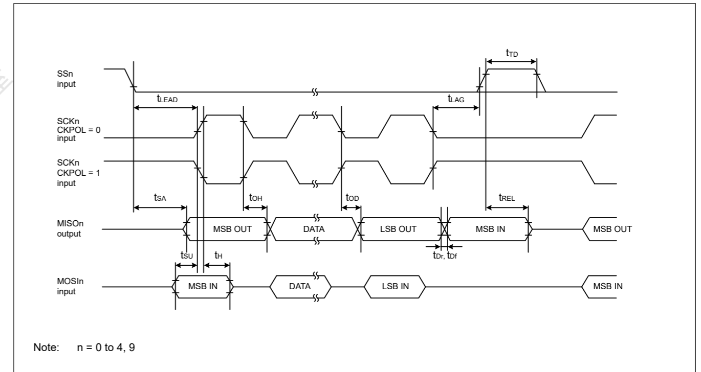
Figure 47.31 CKPH=1时从机的SCI简单SPI模式时序
