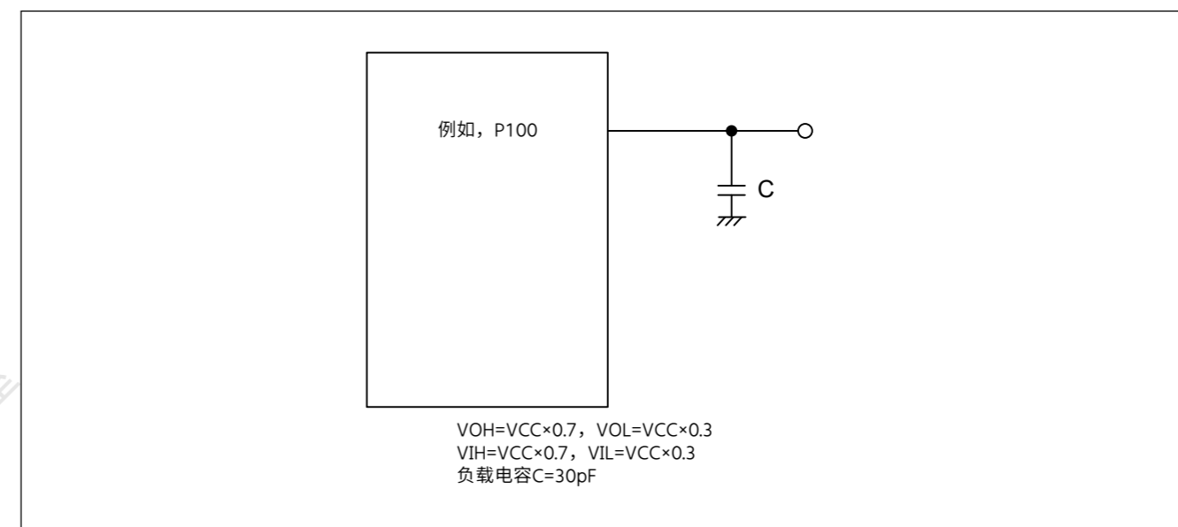
Figure 47.1 输入或输出定时测量条件
