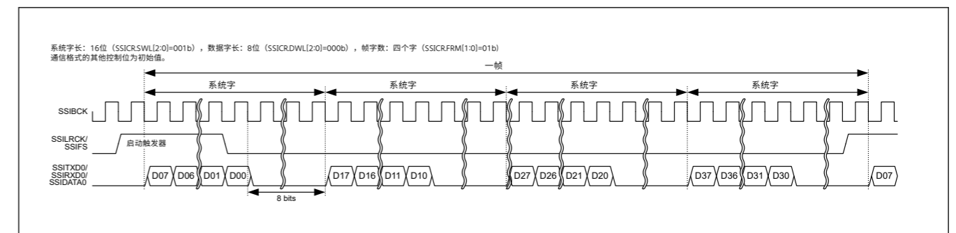
Figure 32.42 TDM格式 (带填充: 系统字长>数据字长)
