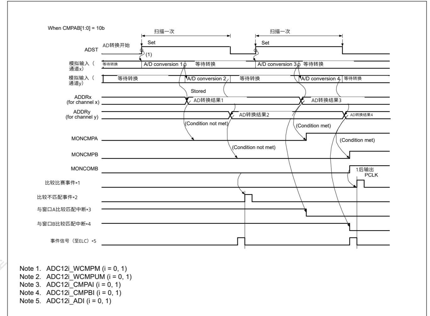
Figure 37.30 比较模拟输入（通道x和y）时比较功能事件输出的示例操作
