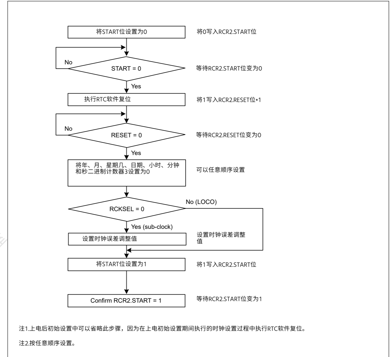
Figure 23.4 设定时间
