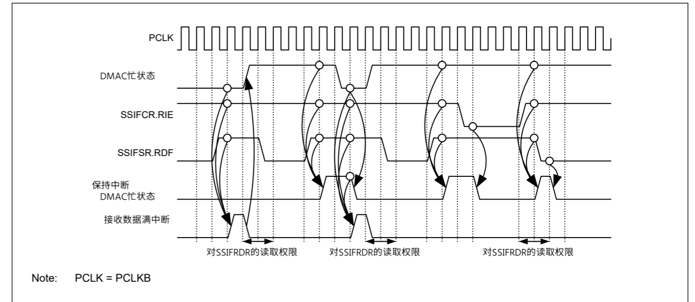
Figure 32.22 接收数据满中断的时序
