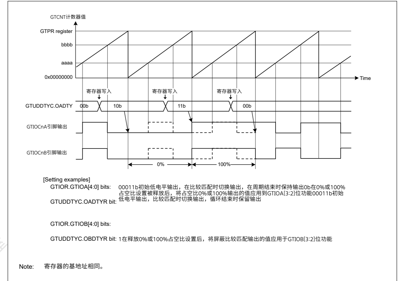
Figure 21.29 输出占空比0%和100%功能示例
