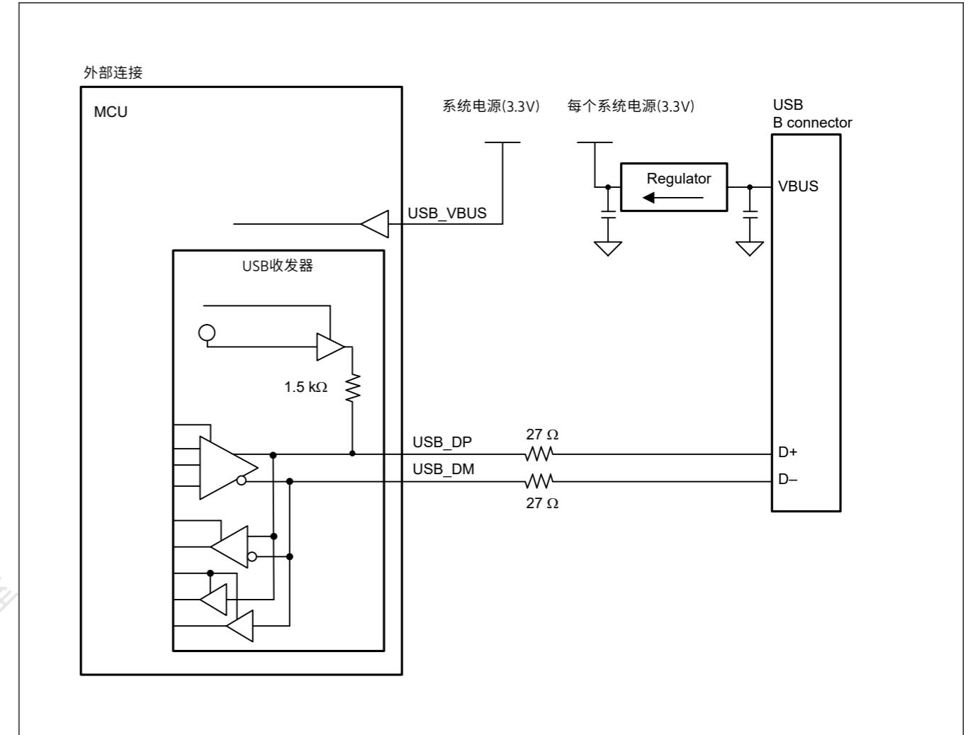
Figure 26.5 总线供电状态下的示例设备连接
