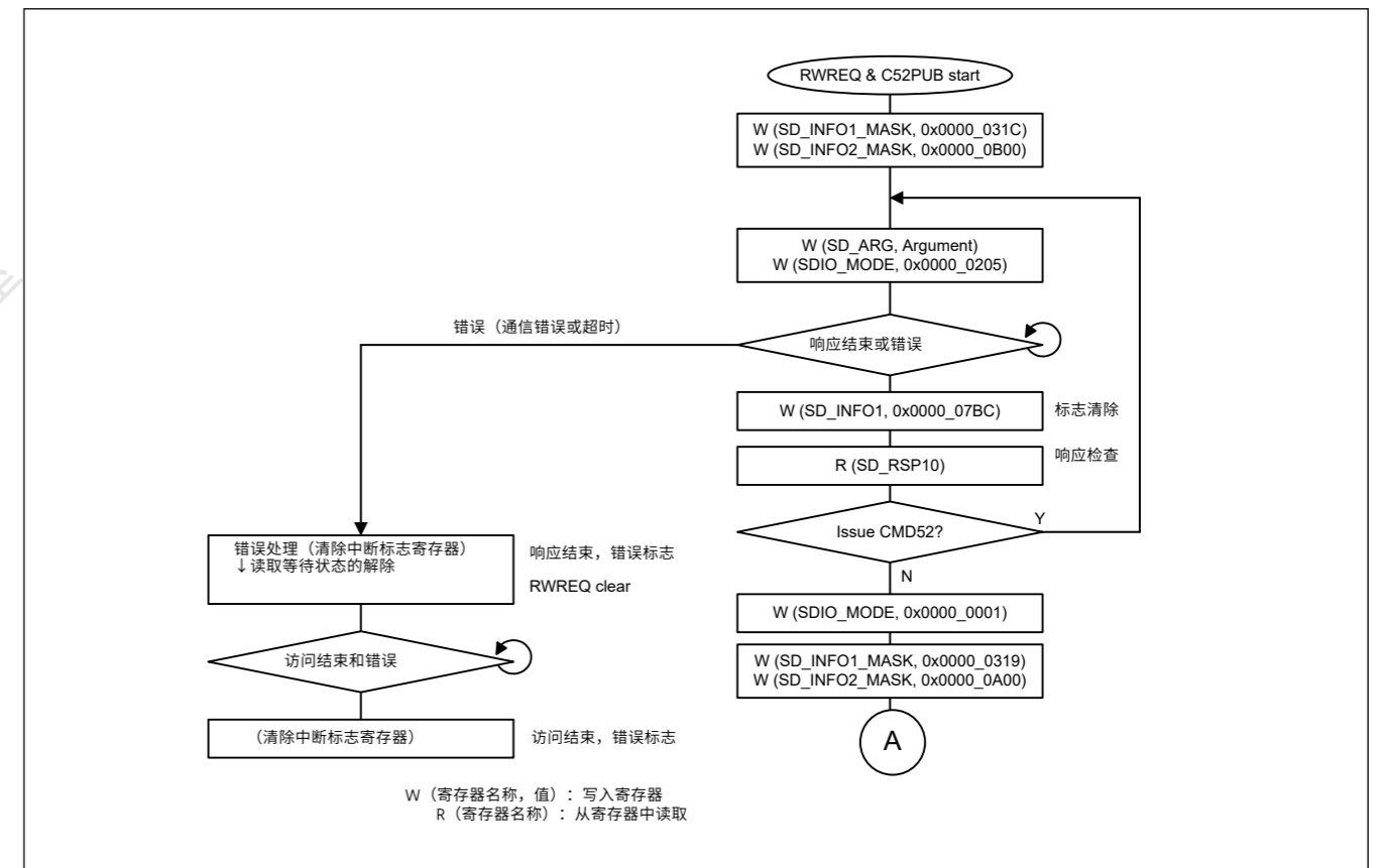
Figure 33.19 在CMD53多块读取期间发出CMD52 (SDIO无中止) 时的流程, 而SD主机接口处于读取等待状态
