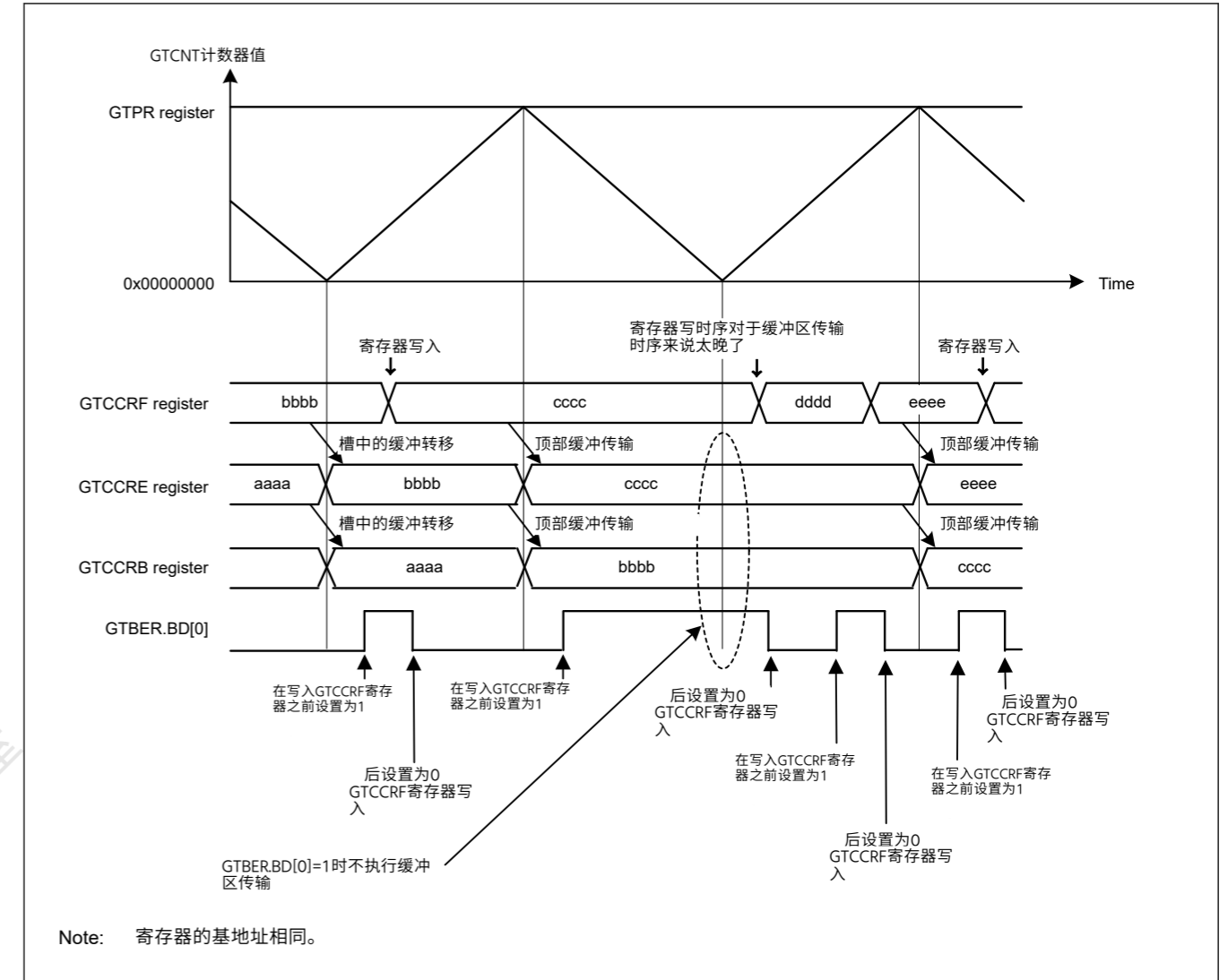
Figure 21.64 三角波缓冲操作、双缓冲操作、波谷和波峰缓冲转移的禁用操作示例
