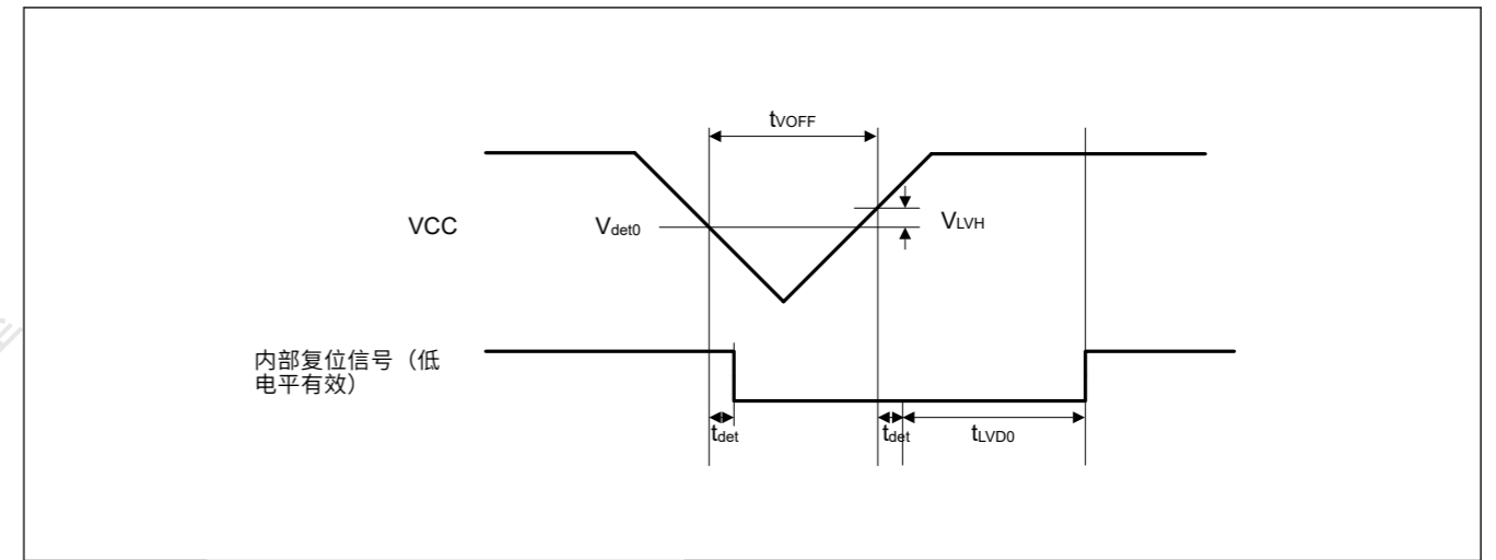
Figure 47.57 电压检测电路时序 ( V_{det0} )
