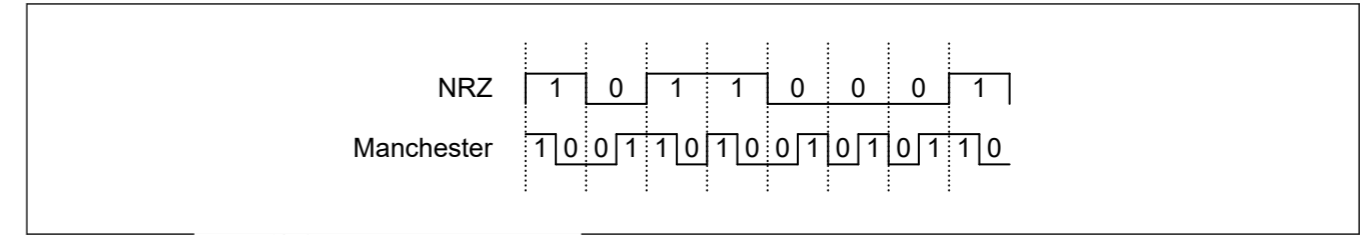
Figure 27.49 曼彻斯特编码示例
