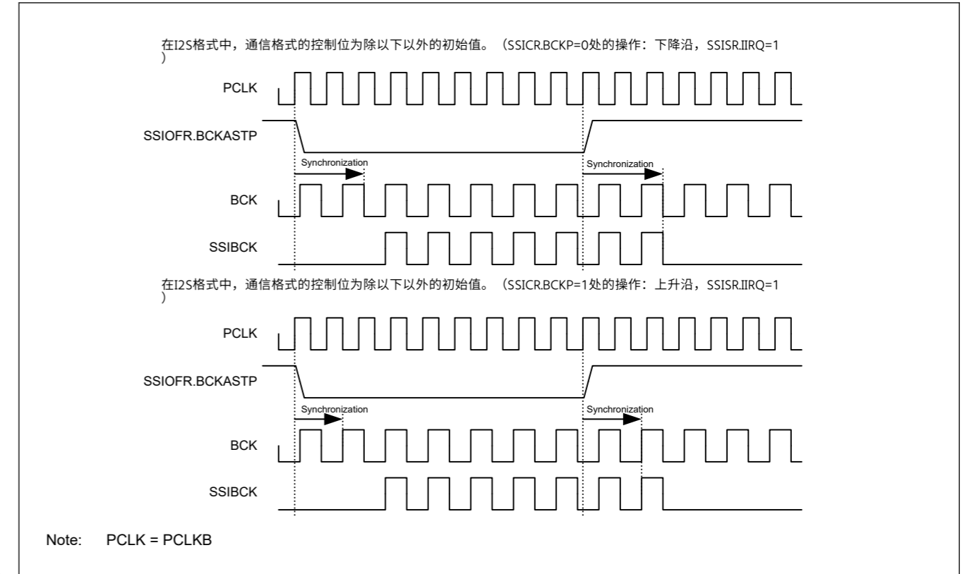
Figure 32.45 使用SSIOFR.BCKASTP停止SSIBCK的示例
