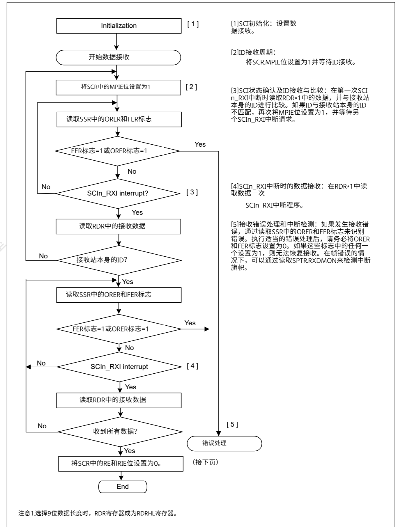
Figure 27.45 选择非FIFO的多处理器串行接收示例流程(1)
