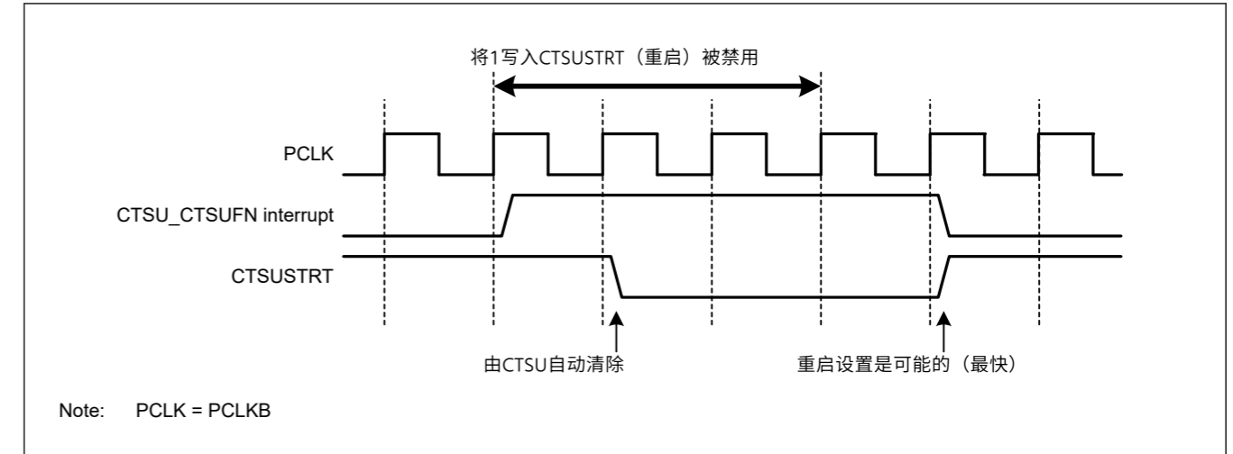
Figure 40.21 重新开始测量的注意事项
