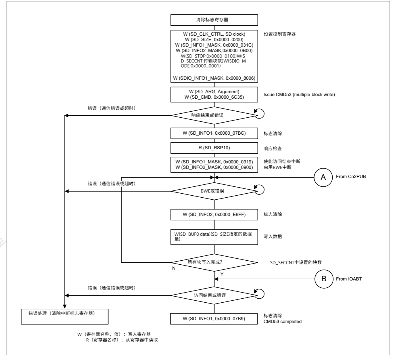
Figure 33.20 CMD53多块写入操作期间的IO_RW_EXTENDED命令示例
