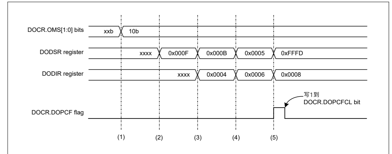
Figure 41.4 数据减法模式下的操作示例
