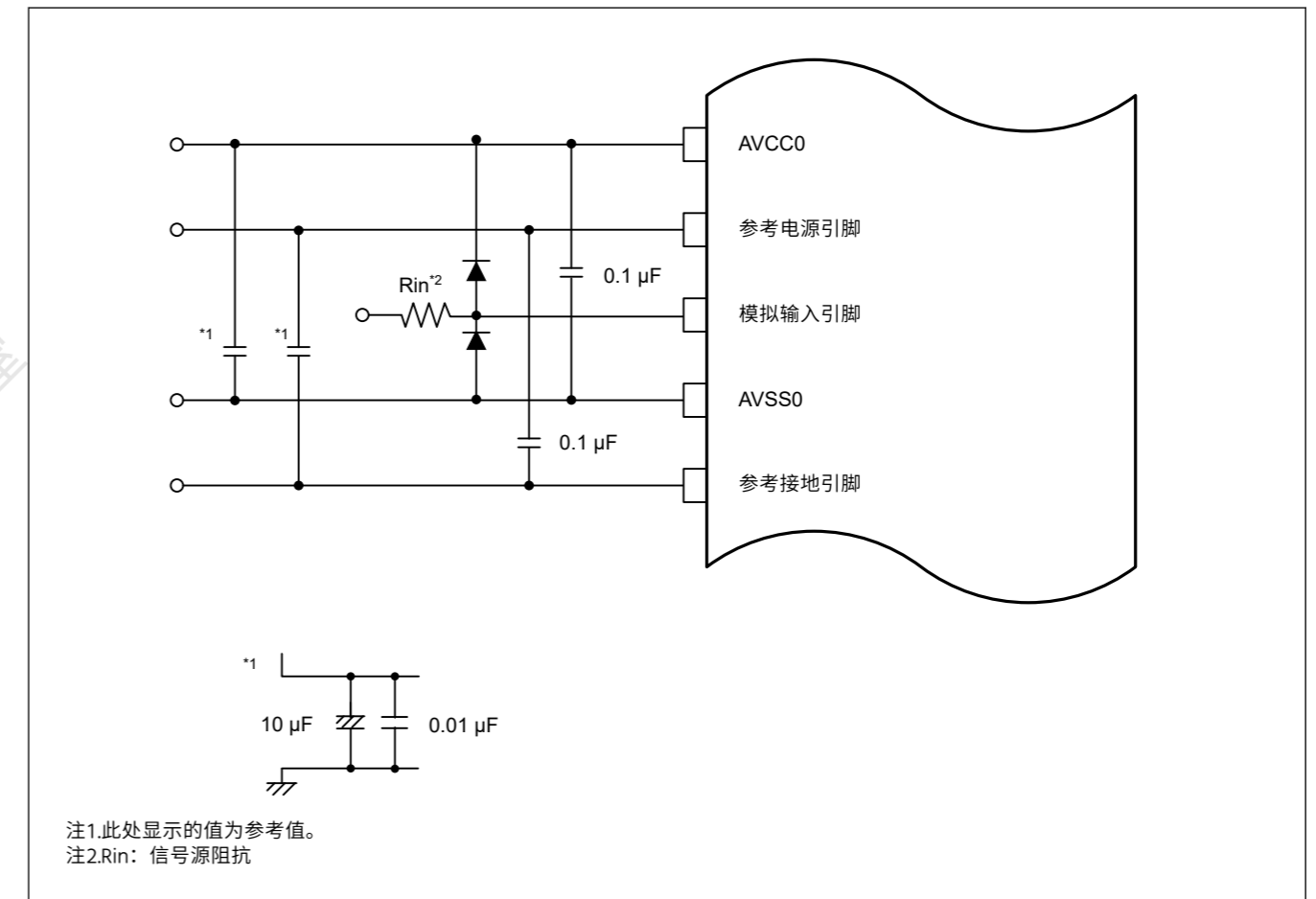
Figure 37.39 模拟输入保护电路示例
