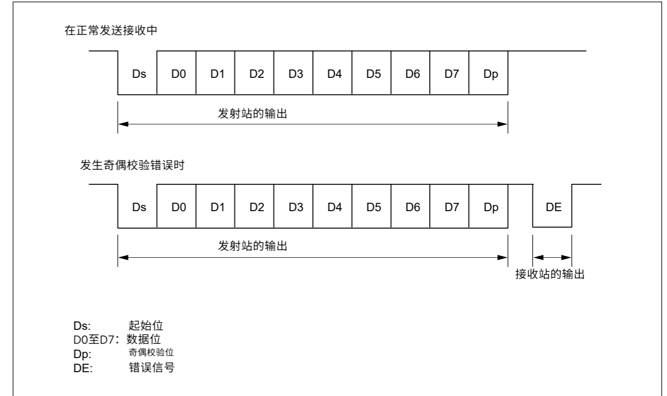
Figure 27.78 智能卡接口模式下的数据格式
