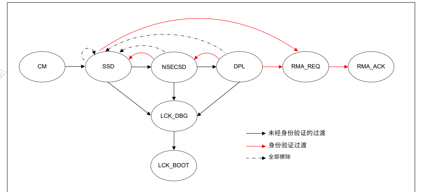
Figure 46.2 设备生命周期示意图
