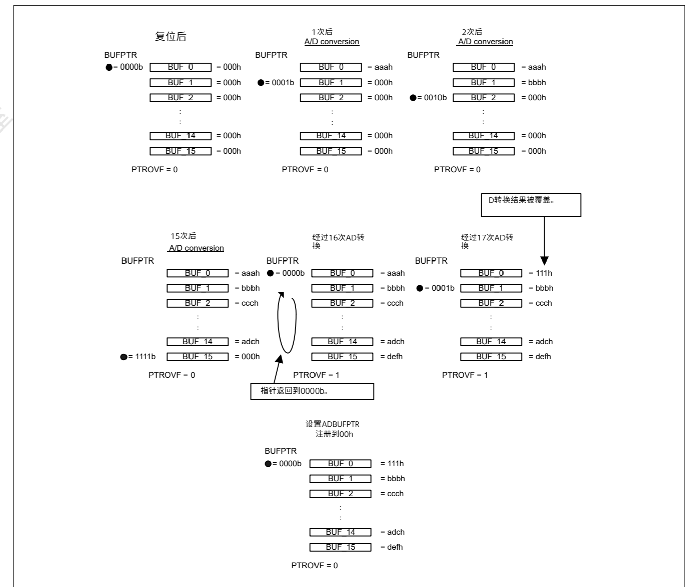
Figure 37.37 数据缓冲区、指针和溢出标志操作
