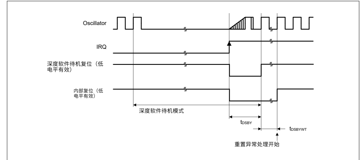
Figure 47.15 深度软件待机模式取消时序
