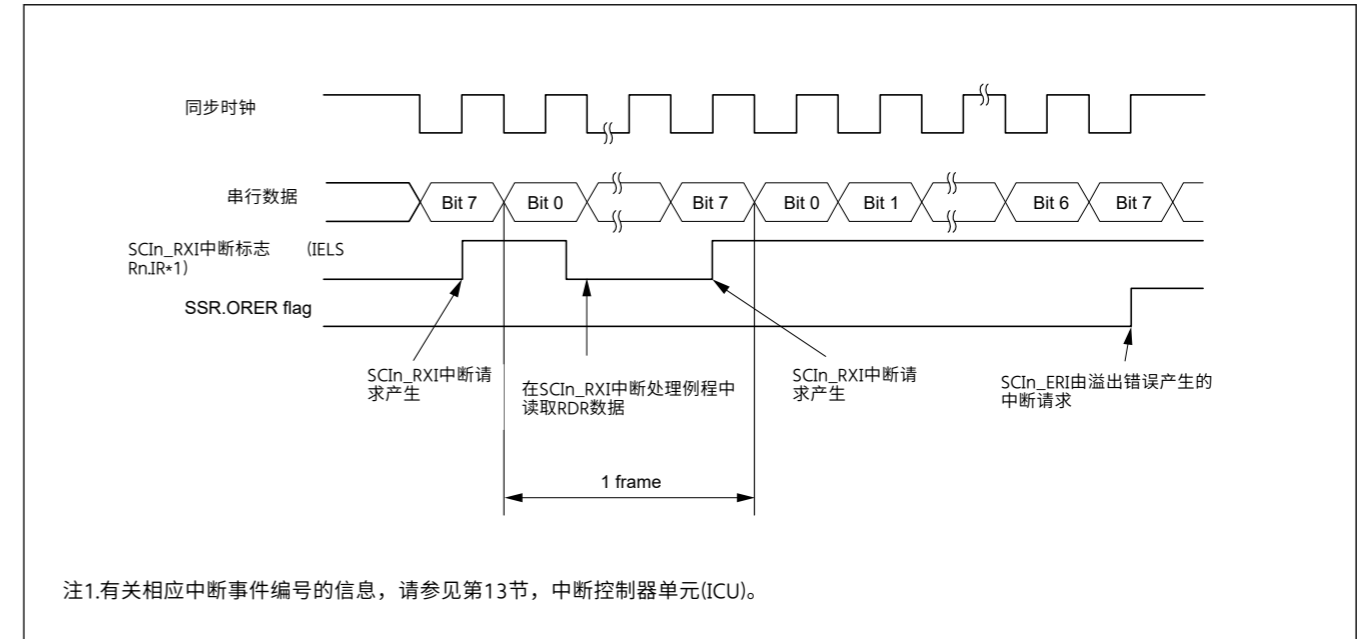
Figure 27.71 不使用RTS功能时时钟同步模式下串行接收的示例操作(1)
