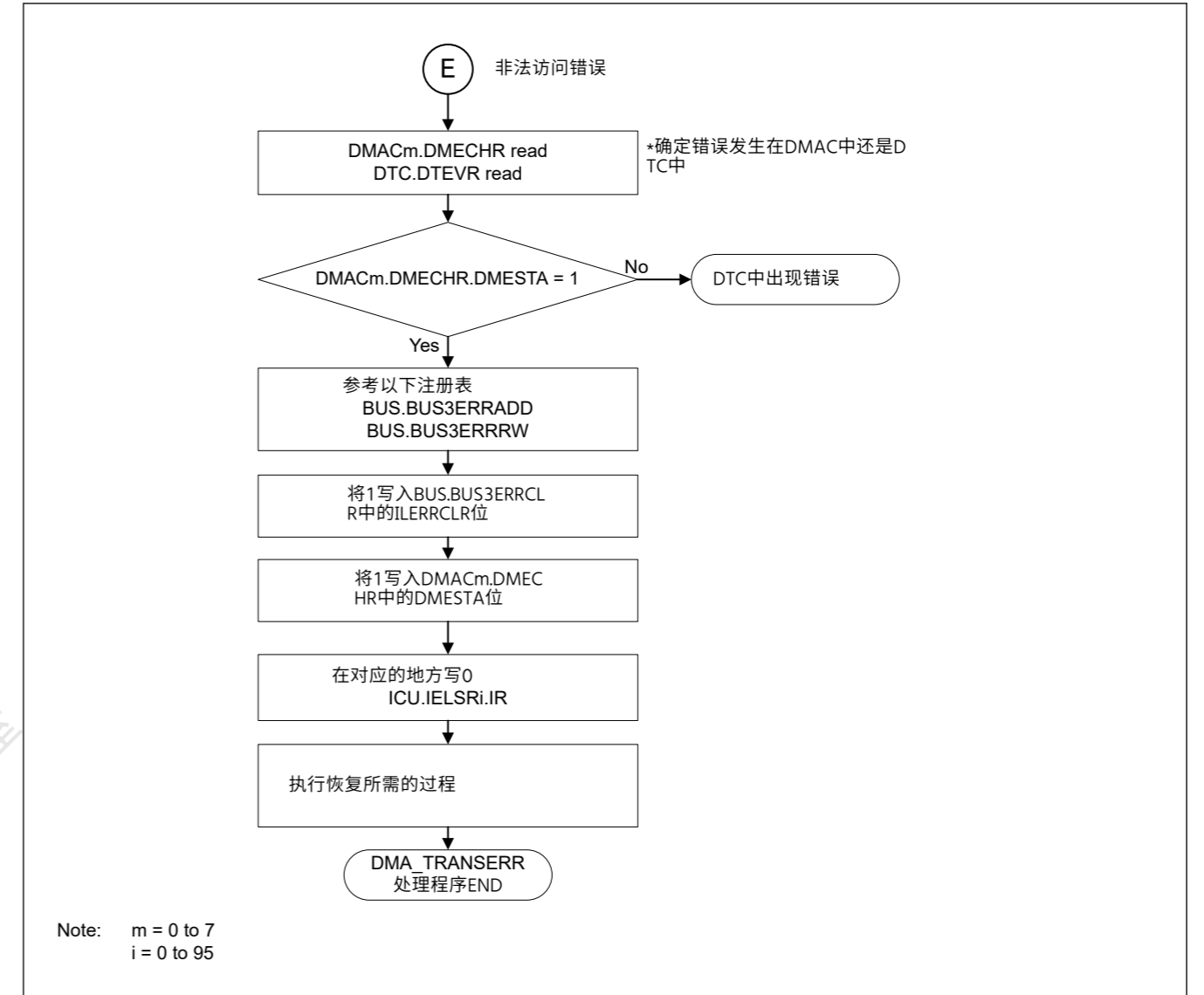
Figure 16.32 非法访问错误在DMA_TRANSERR处理程序中的处理
