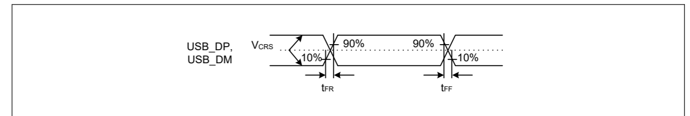
Figure 47.52 全速模式下的USB_DP和USB_DM输出时序
