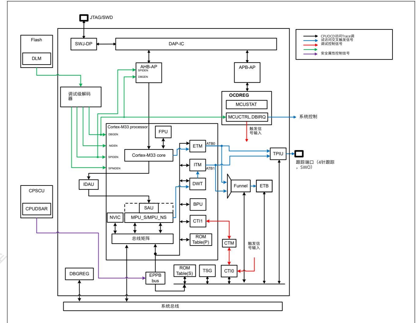
Figure 2.1 Cortex-M33框图
