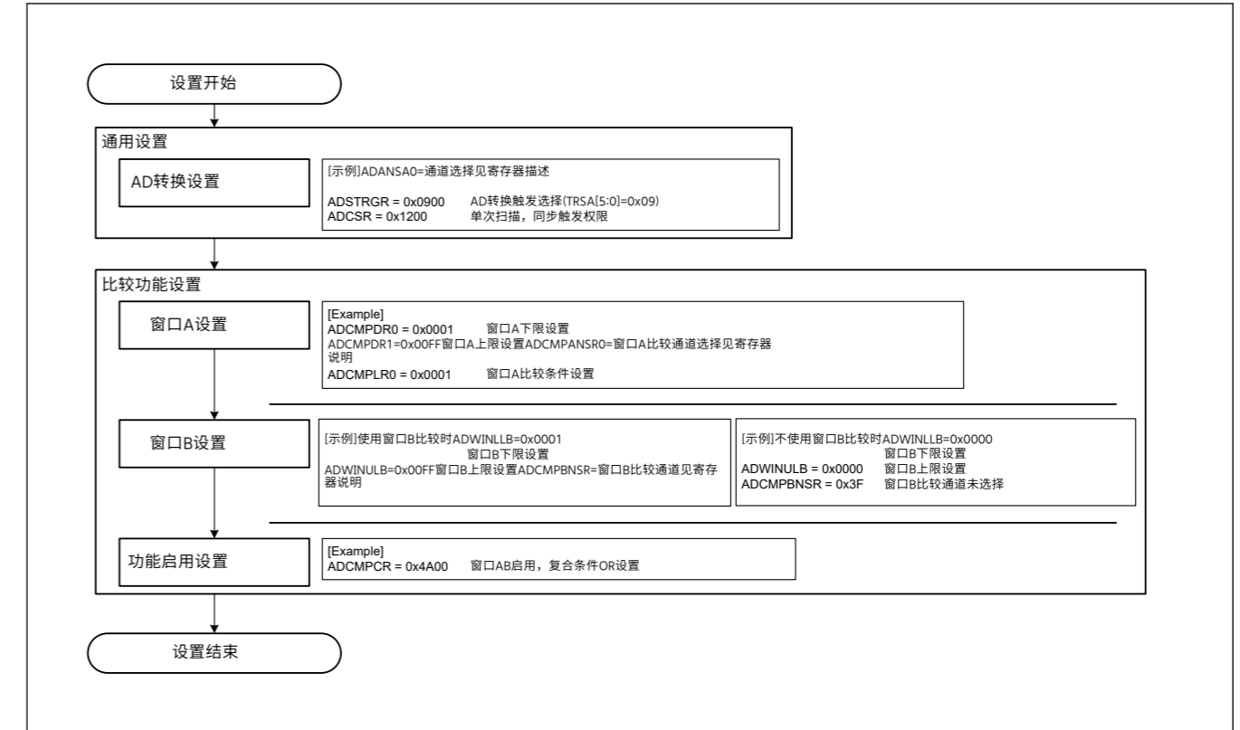
Figure 37.29 使用比较功能的事件输出时的设置示例
