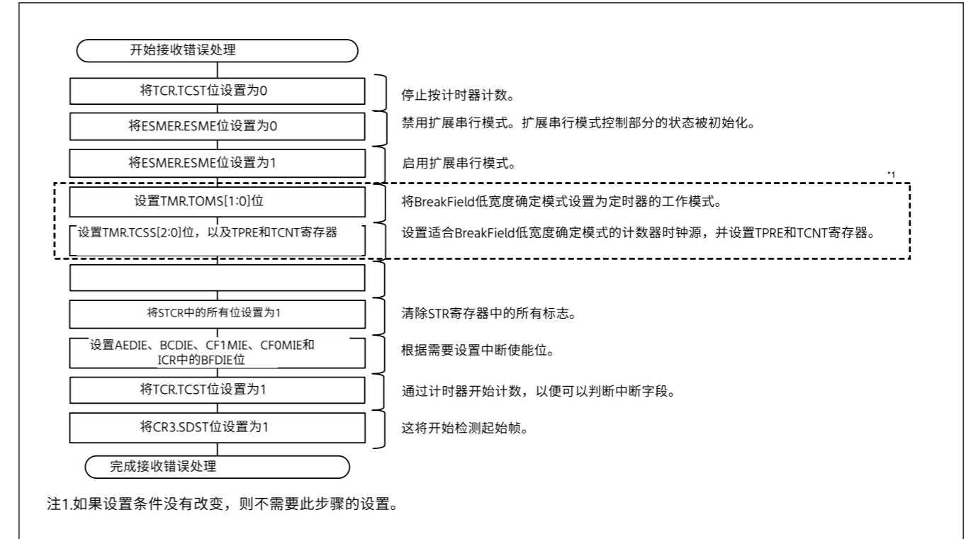
图27.125接收错误处理流程图示例 (接收起始帧期间)
