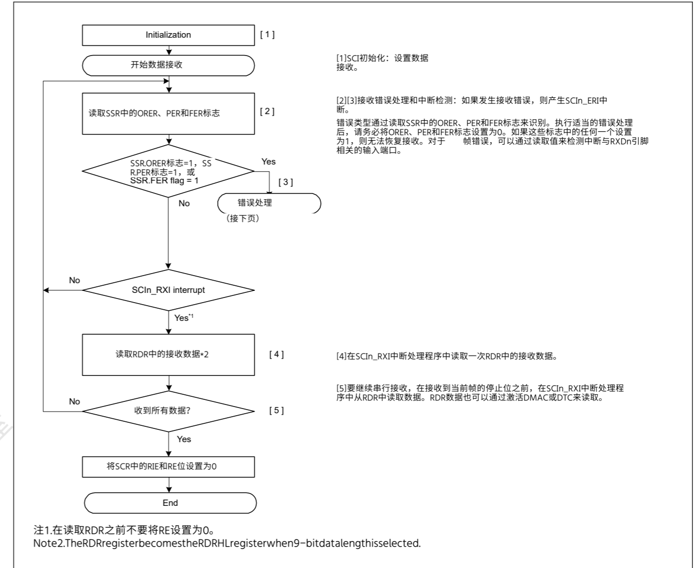
Figure 27.20 异步模式下串行接收的示例流程, 选择了非FIFO和地址匹配已禁用(1)
