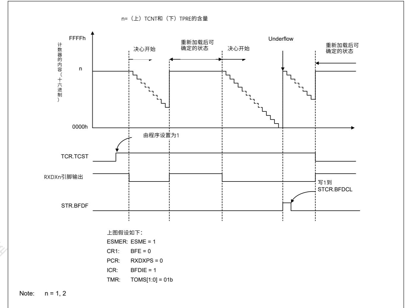
图27.116中断场低宽度确定模式下的操作示例
