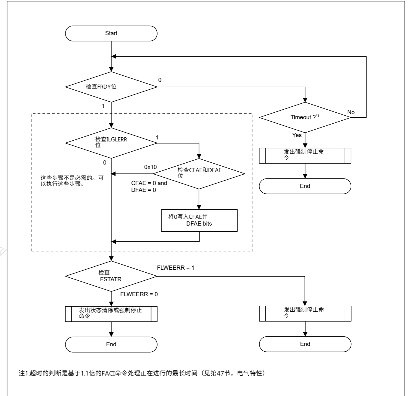
Figure 44.12 从命令锁定状态恢复流程
