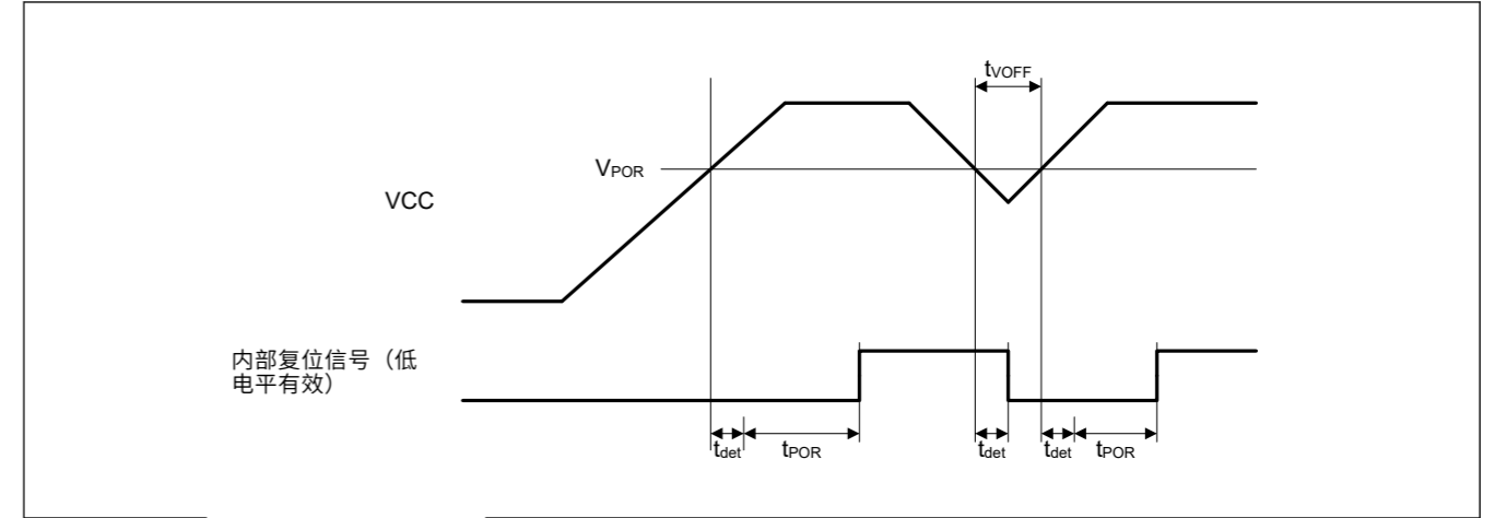
Figure 47.56 上电复位时序
