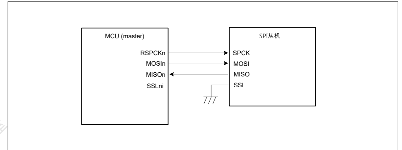
Figure 30.5 MCU为主的单主单从配置示例
