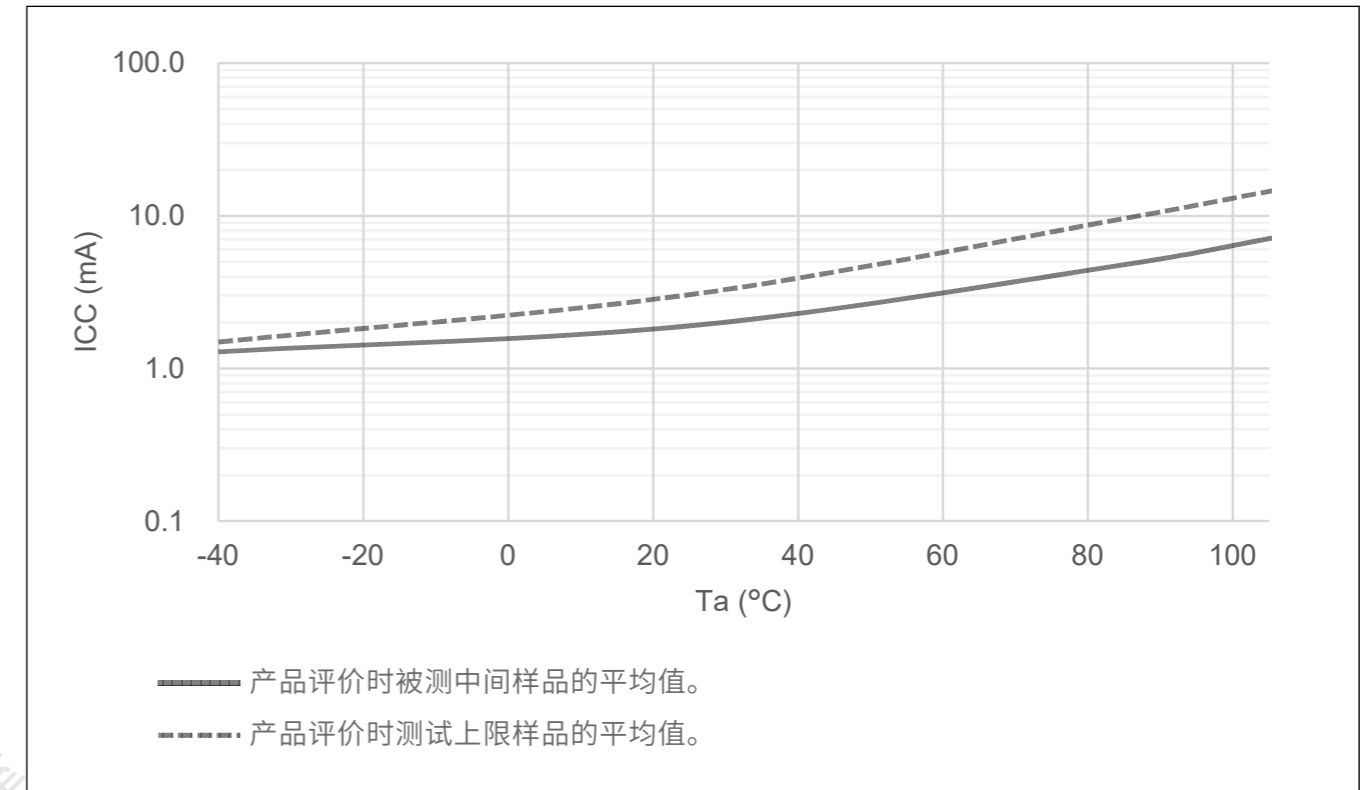
Figure 47.2 软件待机模式下的温度依赖性 (参考数据)
