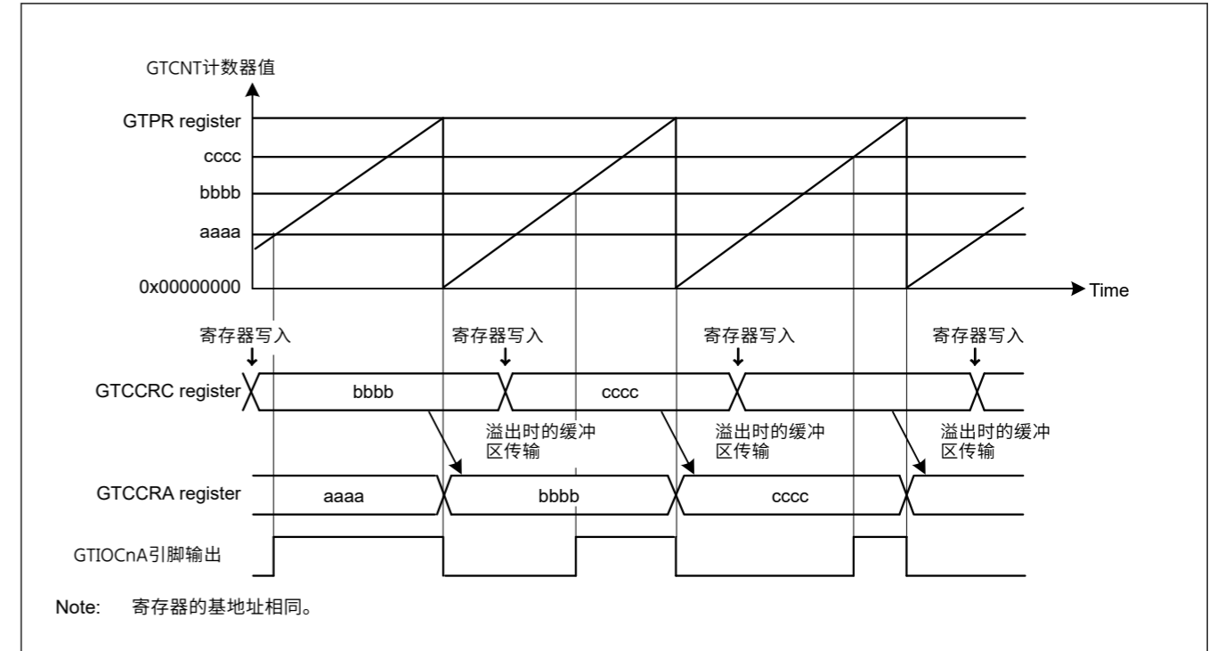
Figure 21.14 GTCCRA和GTCCRB缓冲器操作示例，输出比较、递增计数中的锯齿波、GTCCRA比较匹配时的高输出和周期结束时的低输出
