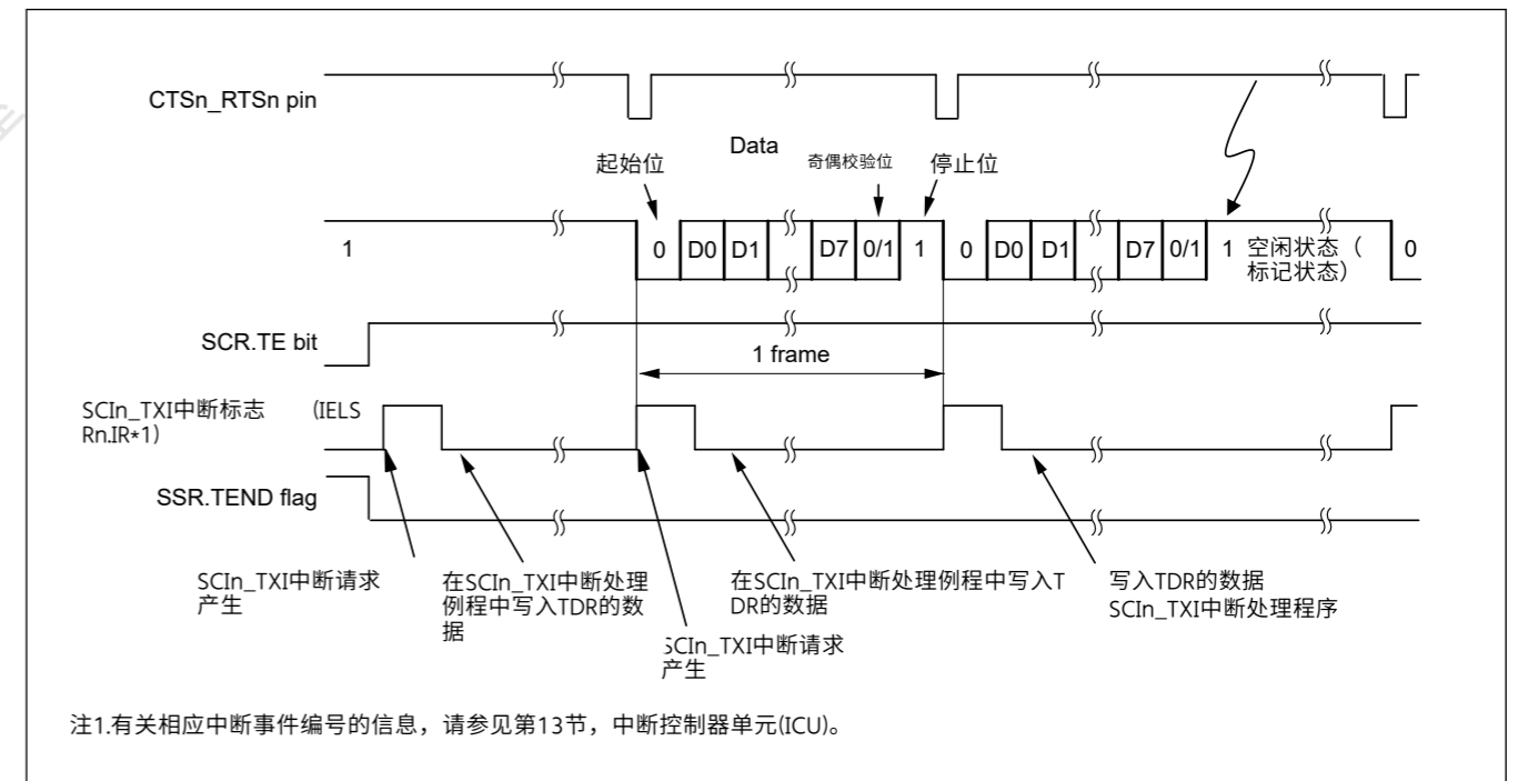
Figure 27.12 异步模式下串行传输的示例操作(2)使用8位数据、奇偶校验位、一个停止位、使用CTS功能以及在传输开始时
