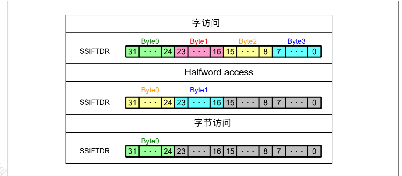
Figure 32.30 对发送FIFO数据寄存器的寄存器访问示例
