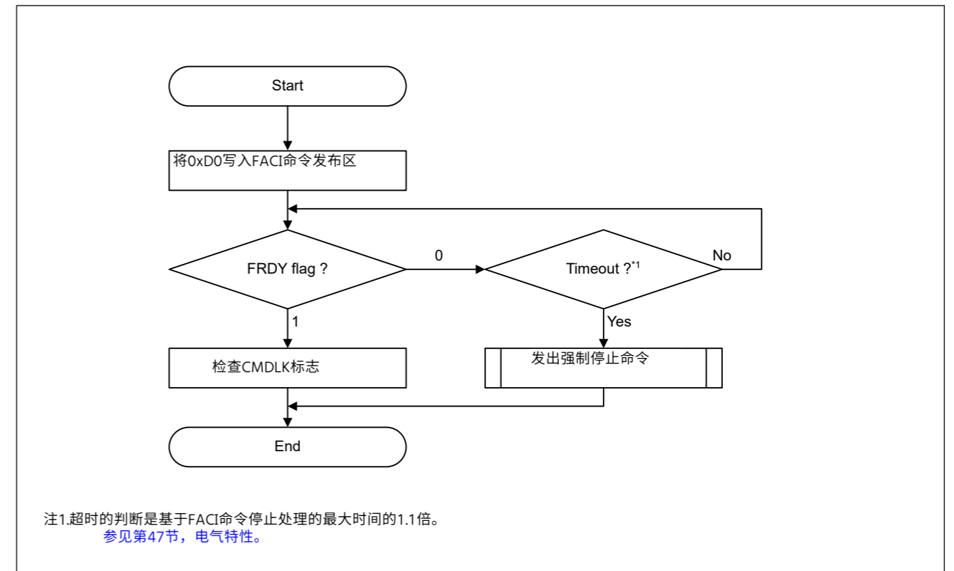
Figure 44.20 PEresume命令的使用流程
