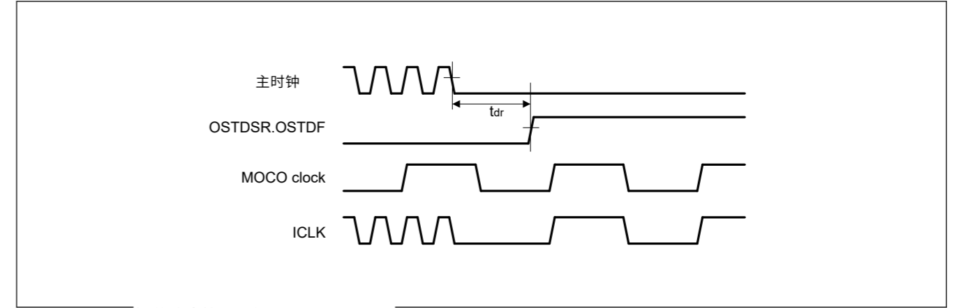
Figure 47.55 振荡停止检测时机
