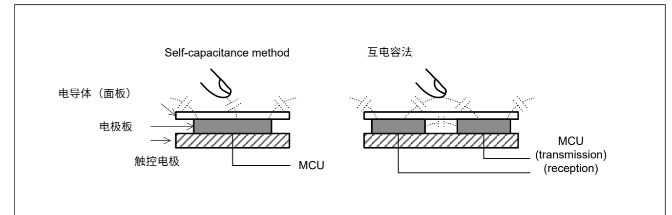
Figure 40.2 自电容和互电容方法
