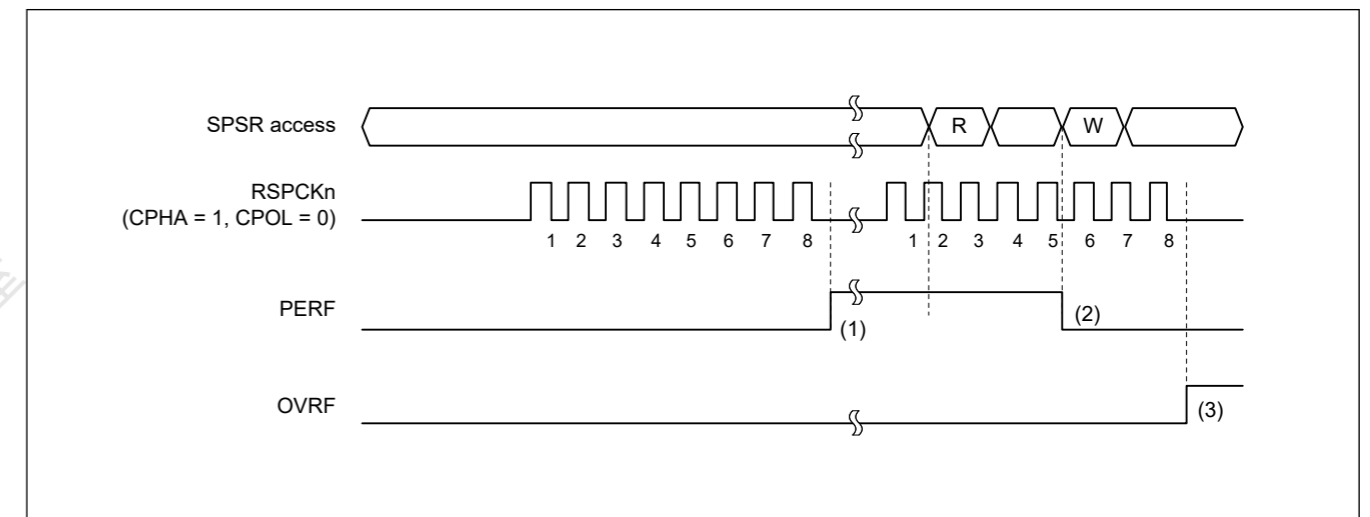
Figure 30.42 PERF标志的操作示例
