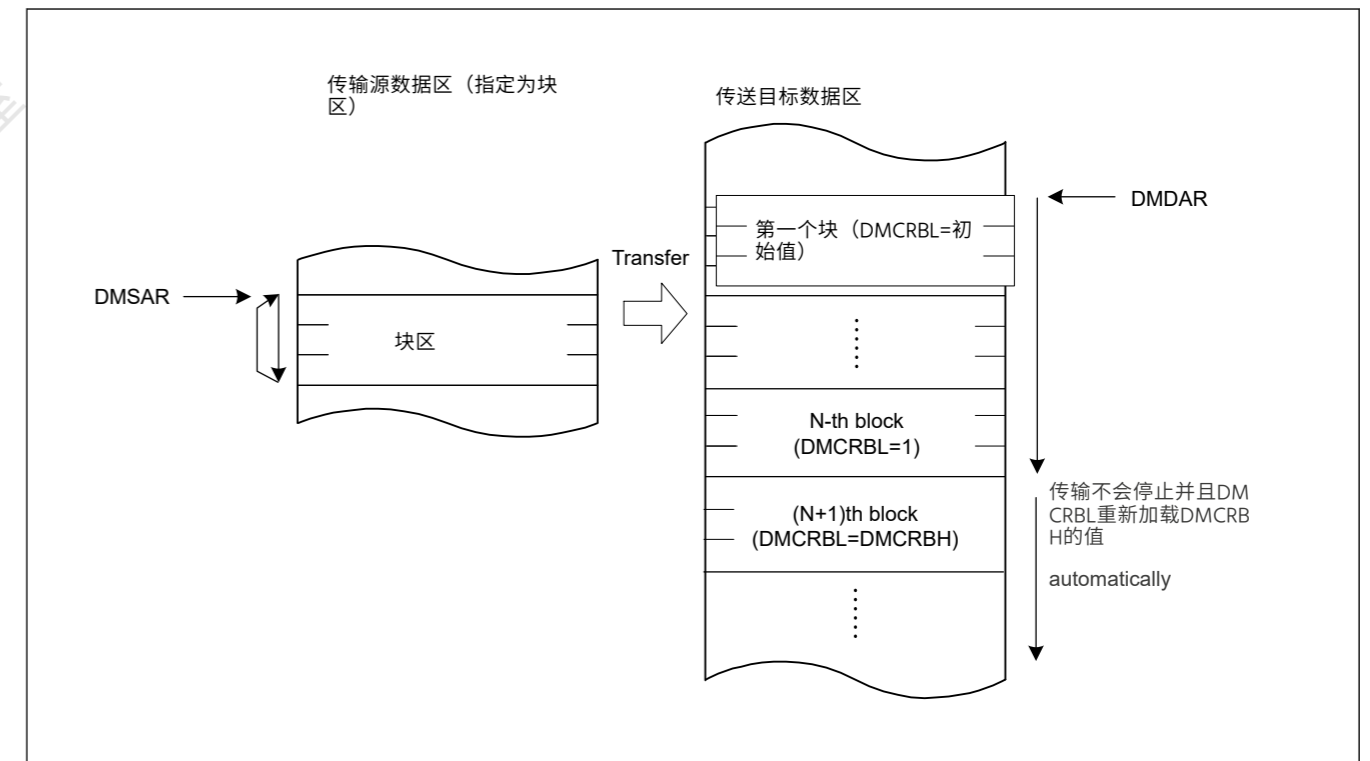
Figure 16.10 DMTMD.TKP位设置为1时块传输模式下的操作
