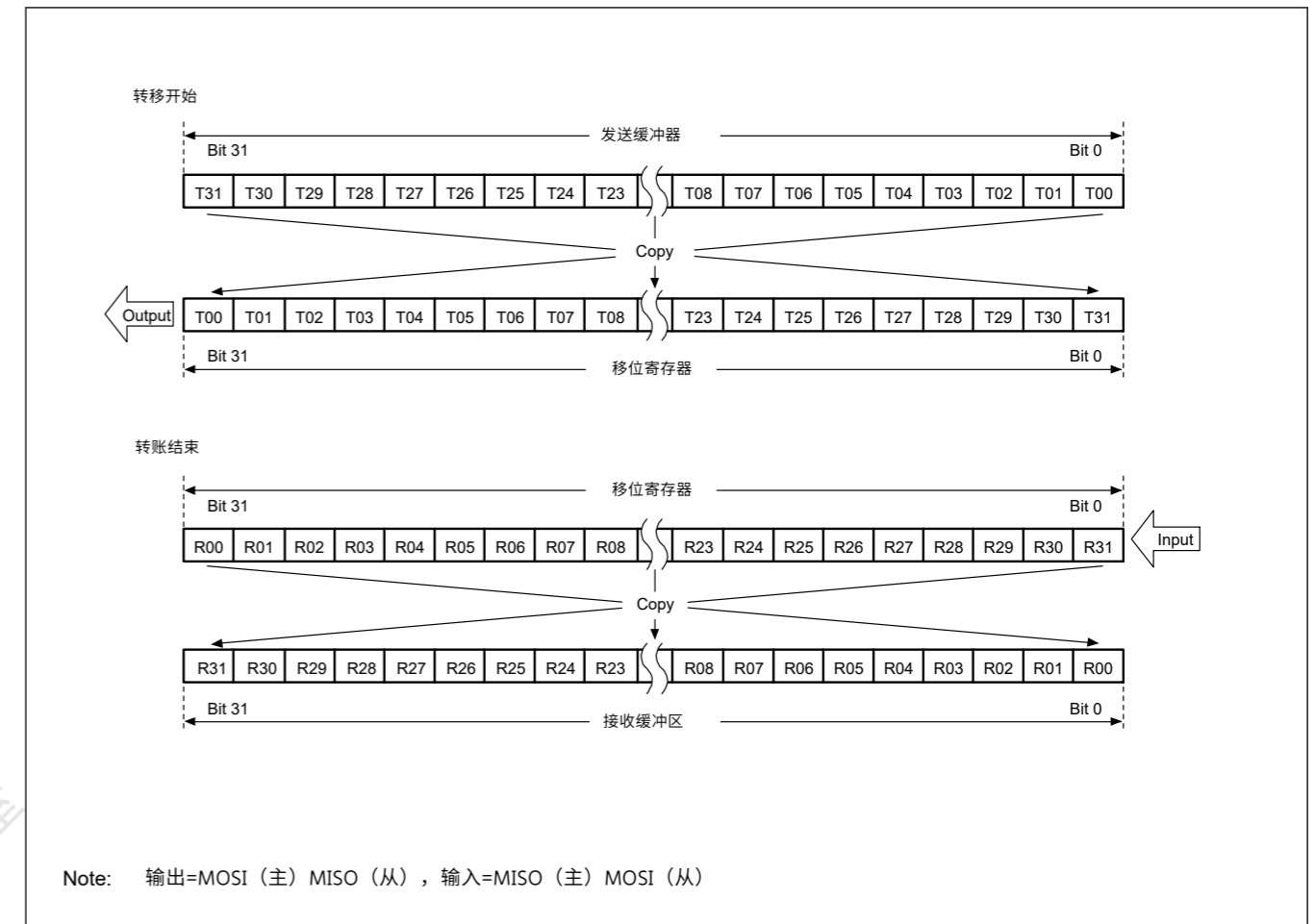
Figure 30.16 LSB优先传输，32位数据和奇偶校验禁用
