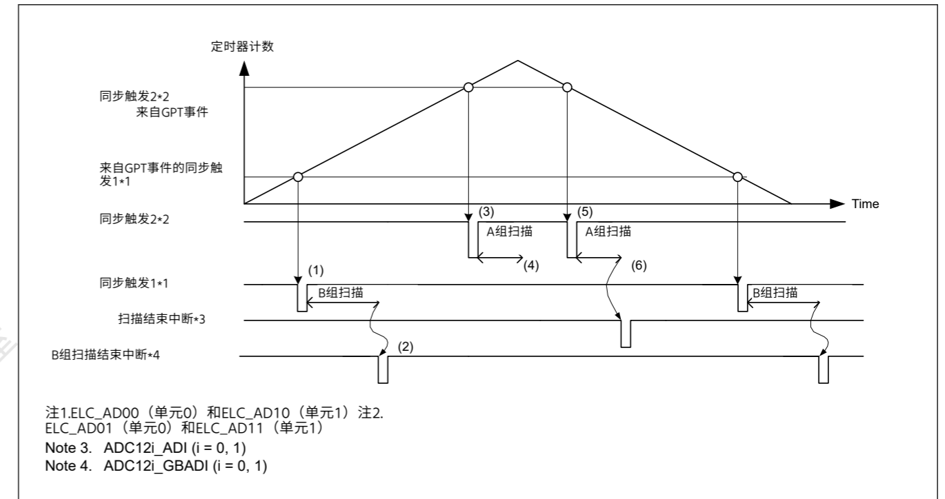
Figure 37.17 当使用来自ELC的同步触发时，具有双触发模式的组扫描模式下的基本操作示例
