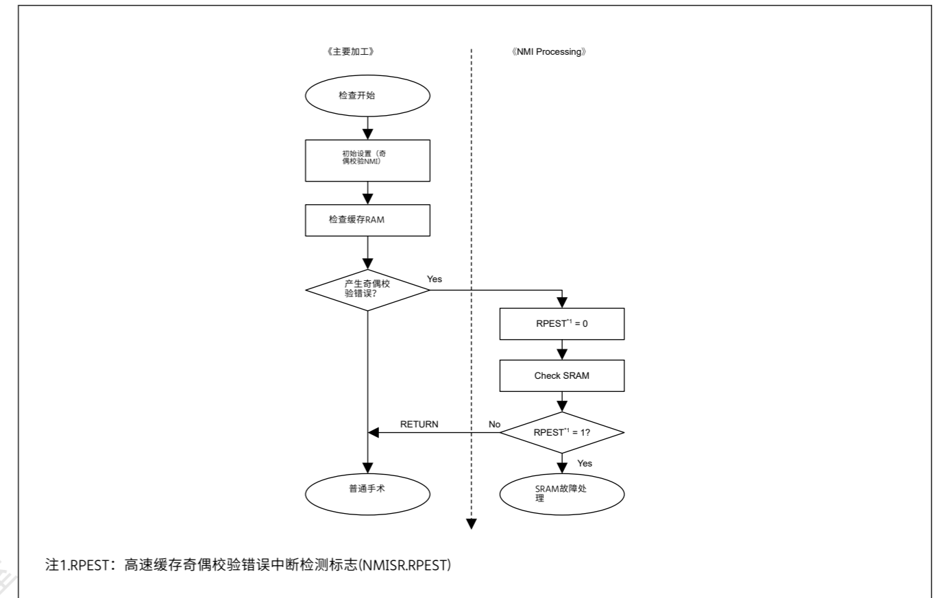
Figure 14.9 启用奇偶校验中断时的缓存奇偶校验流程
