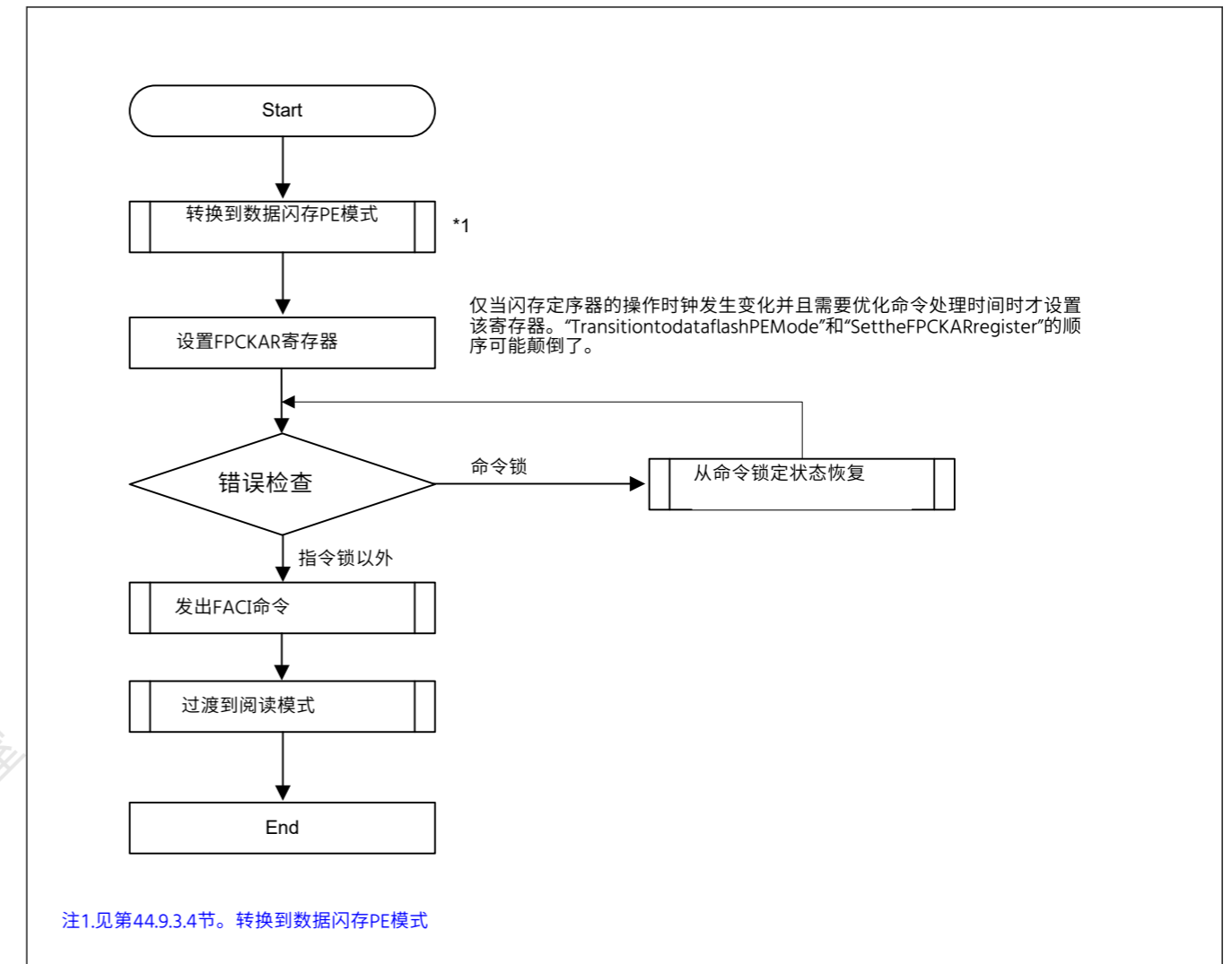
Figure 44.8 数据闪存PE模式下的命令使用概述
