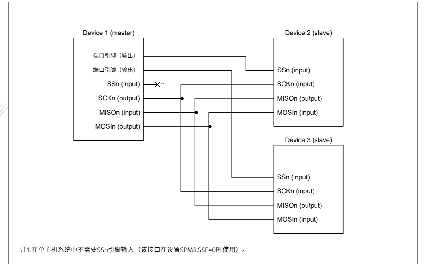
Figure 27.98 在SPMR.SSE位=0的单主模式下使用简单SPI模式的示例连接
