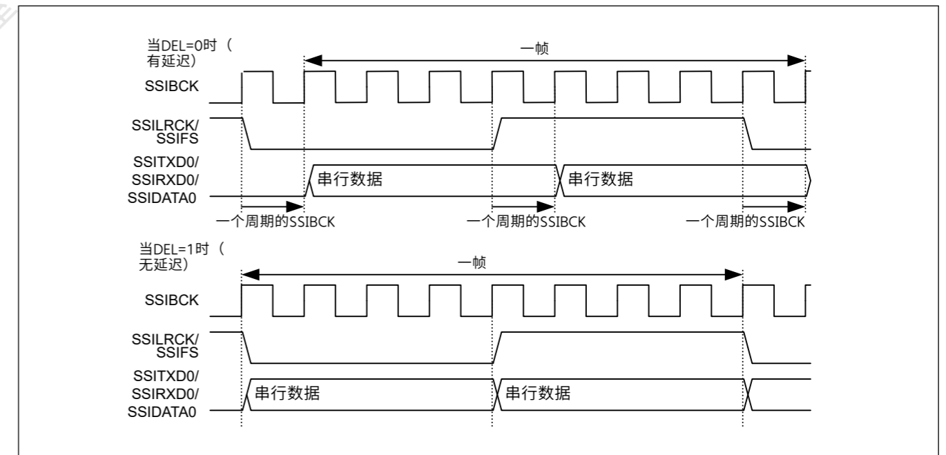
Figure 32.7 串行数据延迟设置
