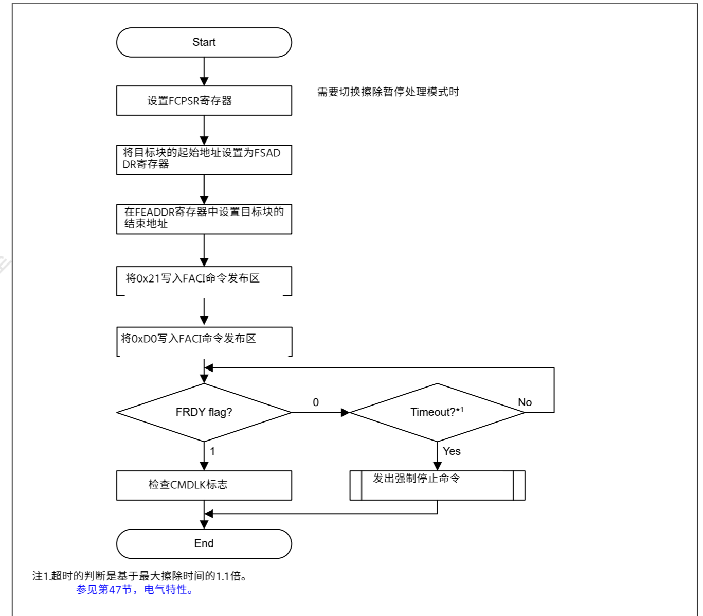
Figure 44.15 多块命令的使用流程
