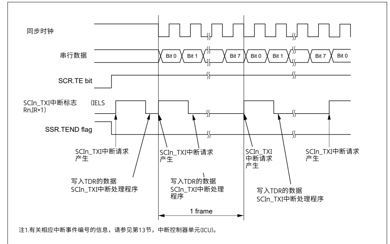
Figure 27.66 传输开始时未使用CTS功能时时钟同步模式下的串行数据传输示例
