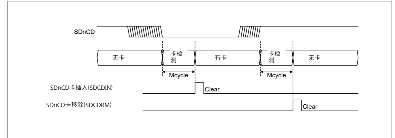
Figure 33.7 SDnCD卡检测示例
