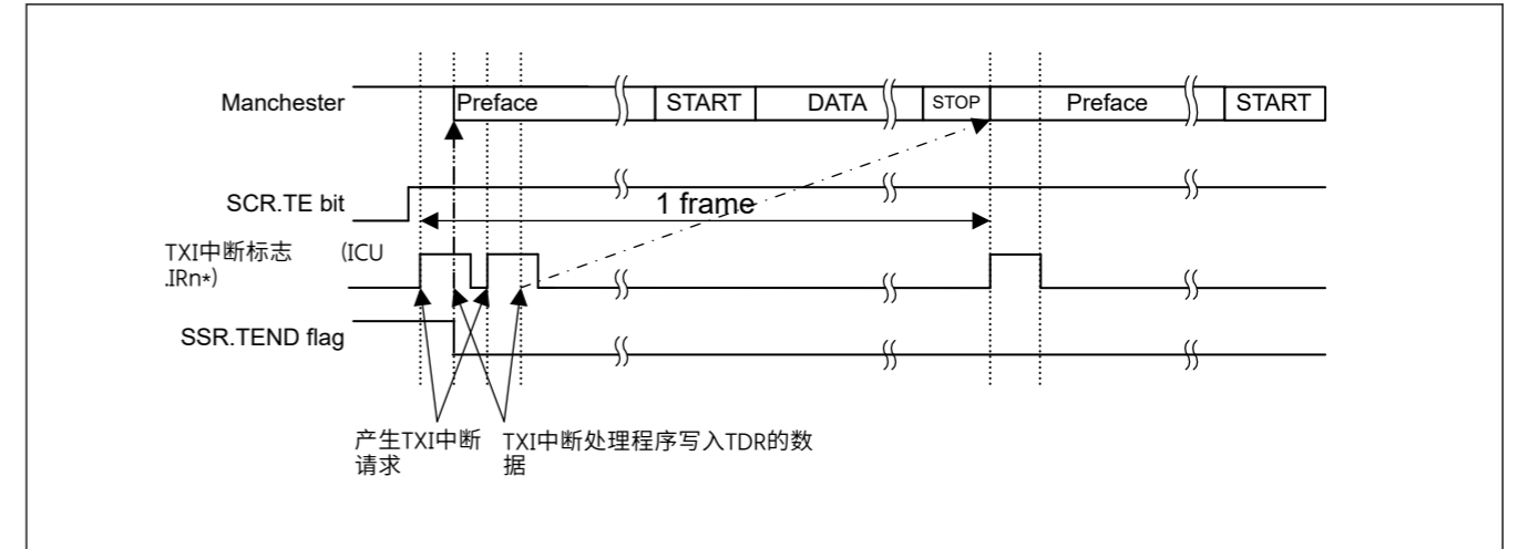
Figure 27.56 曼彻斯特模式下串行传输的传输开始操作示例 (使用前言但没有CTS功能)
