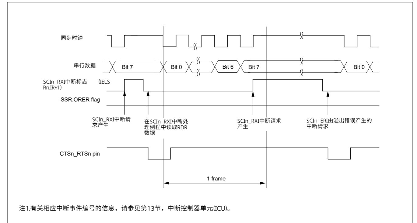
Figure 27.72 使用RTS功能时时钟同步模式下串行接收的示例操作(2)
