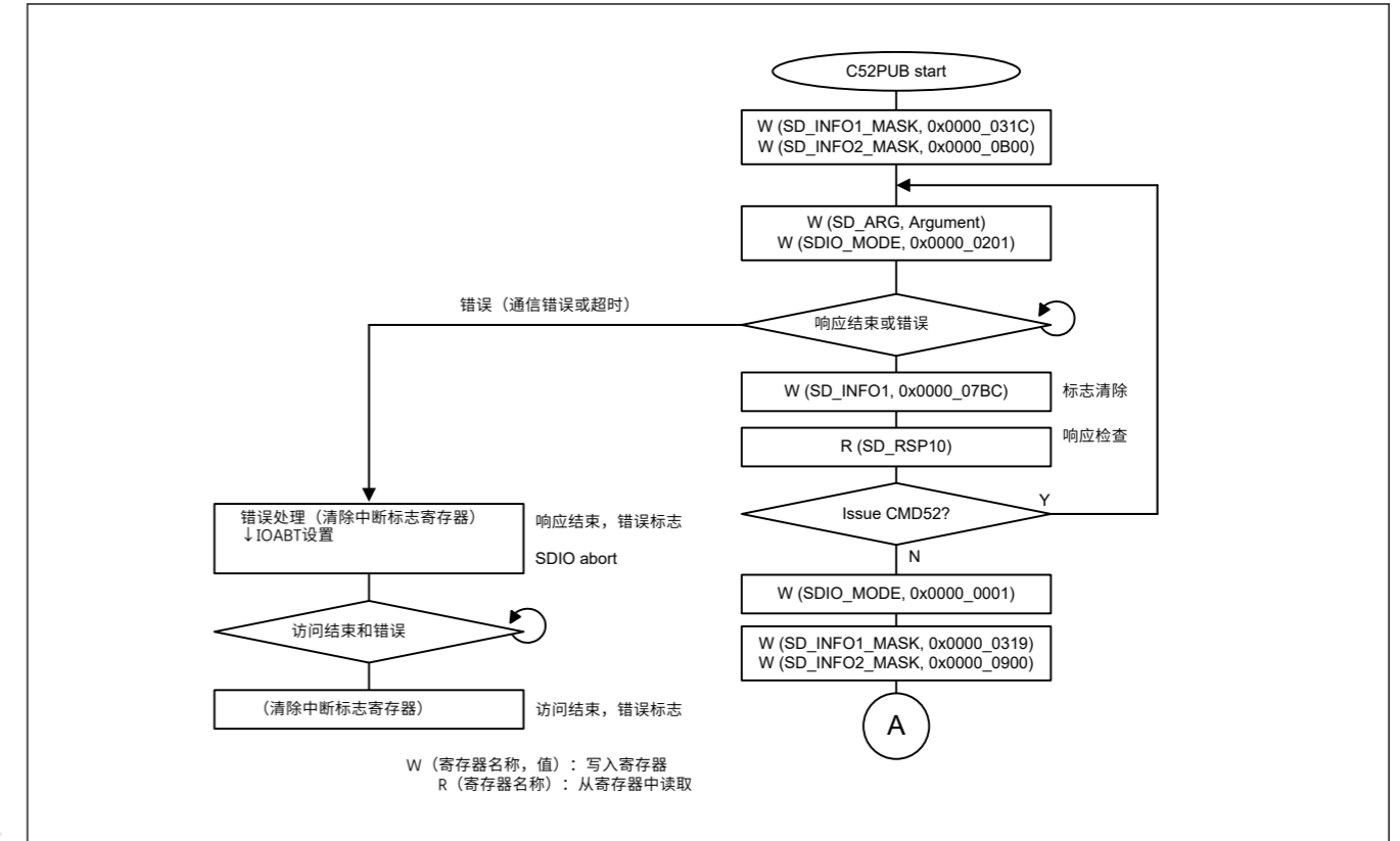
Figure 33.22 在CMD53多块写入期间发出CMD52 (SDIO无中止) 时的流程
