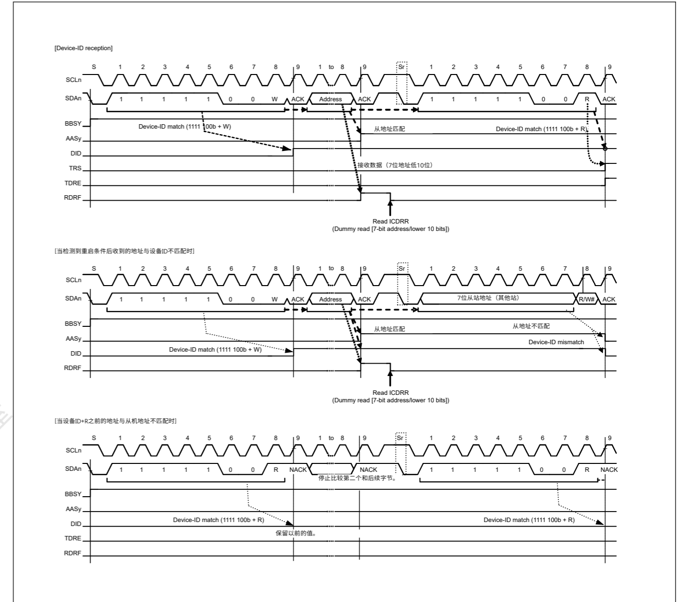
Figure 28.28 在接收设备ID期间设置AASy和DID标志并清除时序
