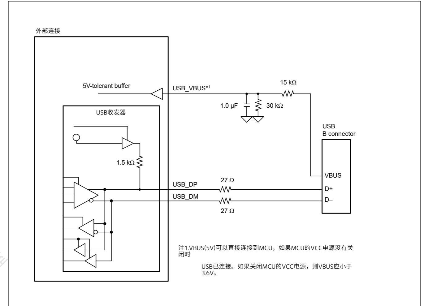
Figure 26.3 自供电系统中的示例设备连接
