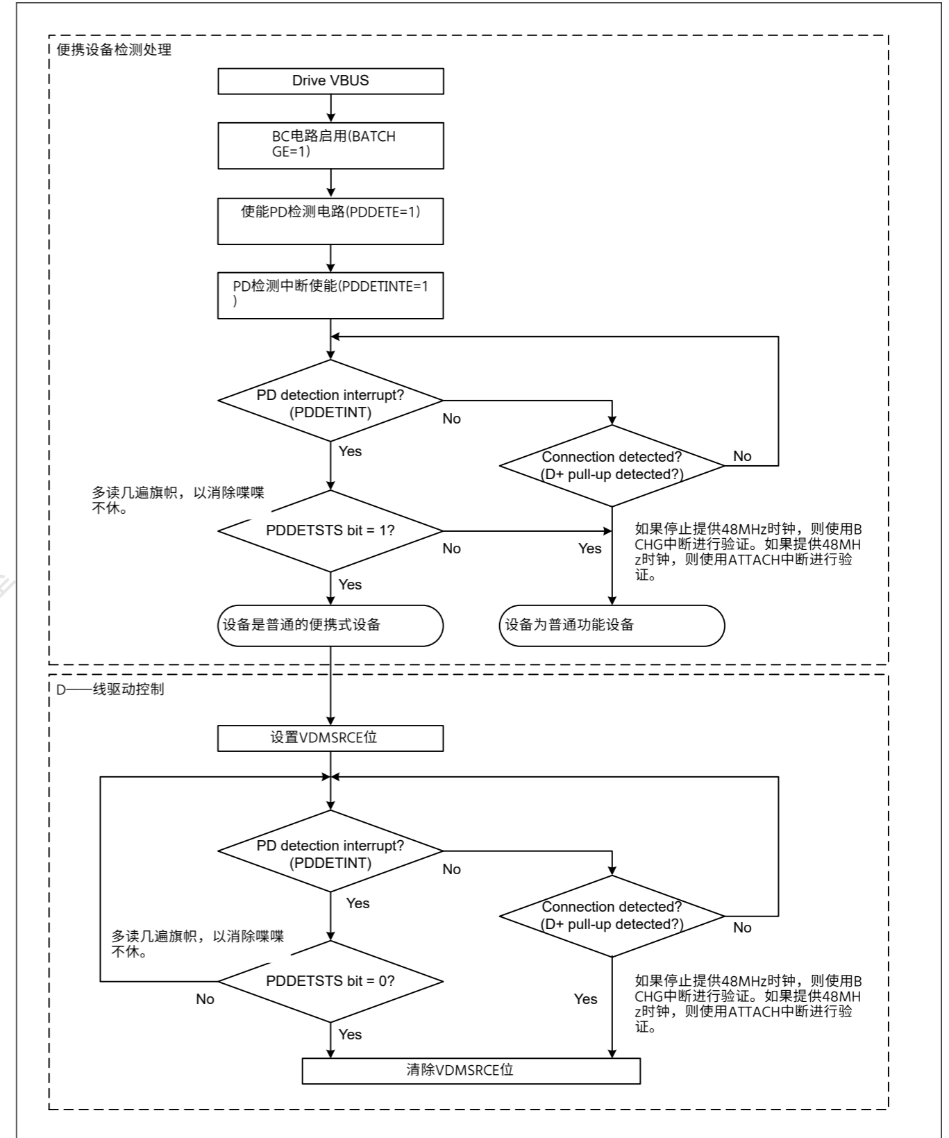
Figure 26.25 使用便携式设备检测功能时的处理流程 (步骤1.至4.)
