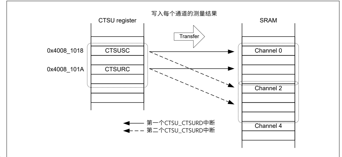
Figure 40.20 使用CTSUS_CTSURD中断的DTC传输操作示例
