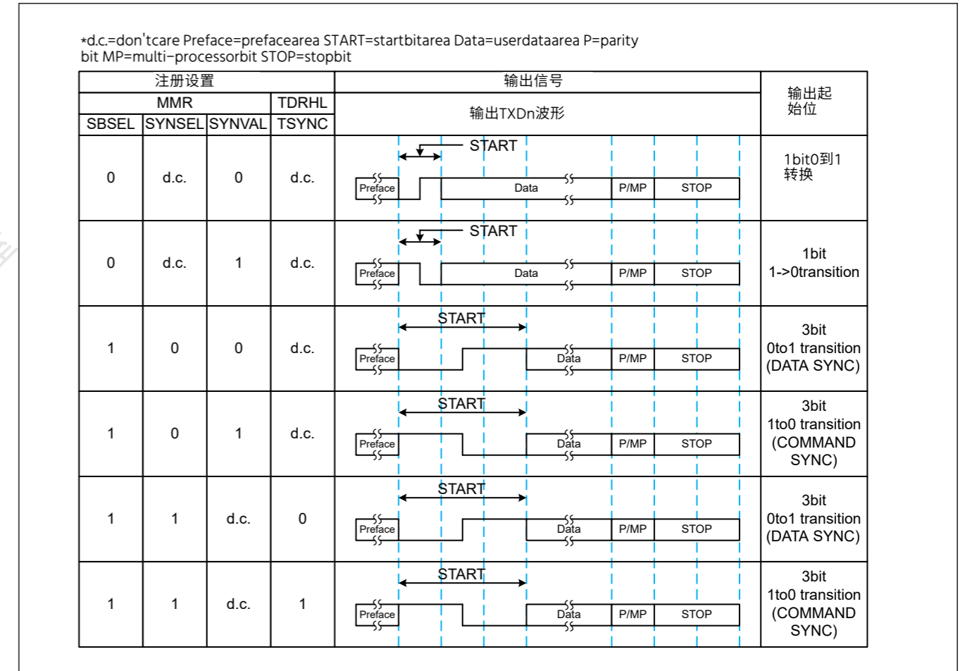
Figure 27.52 发送时起始位区域的相关设置和格式
