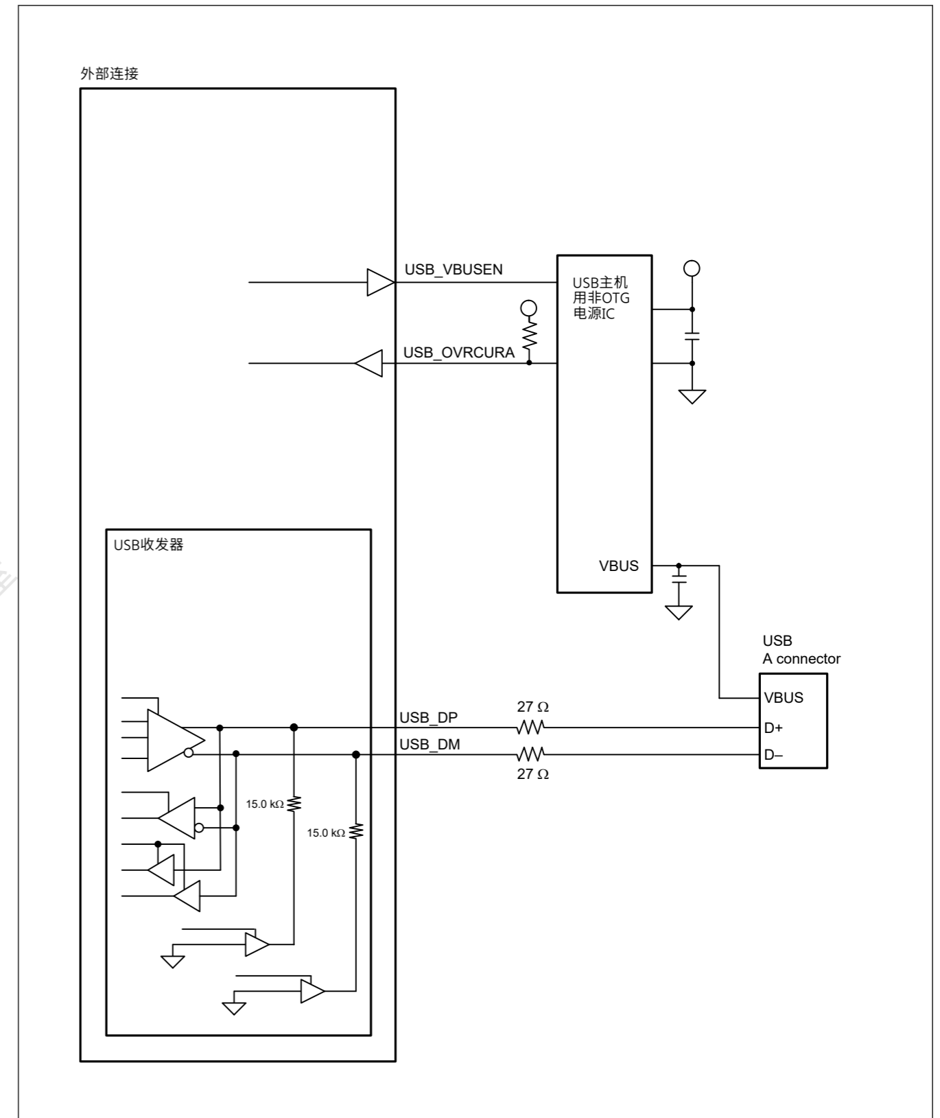
Figure 26.4 主机连接示例
