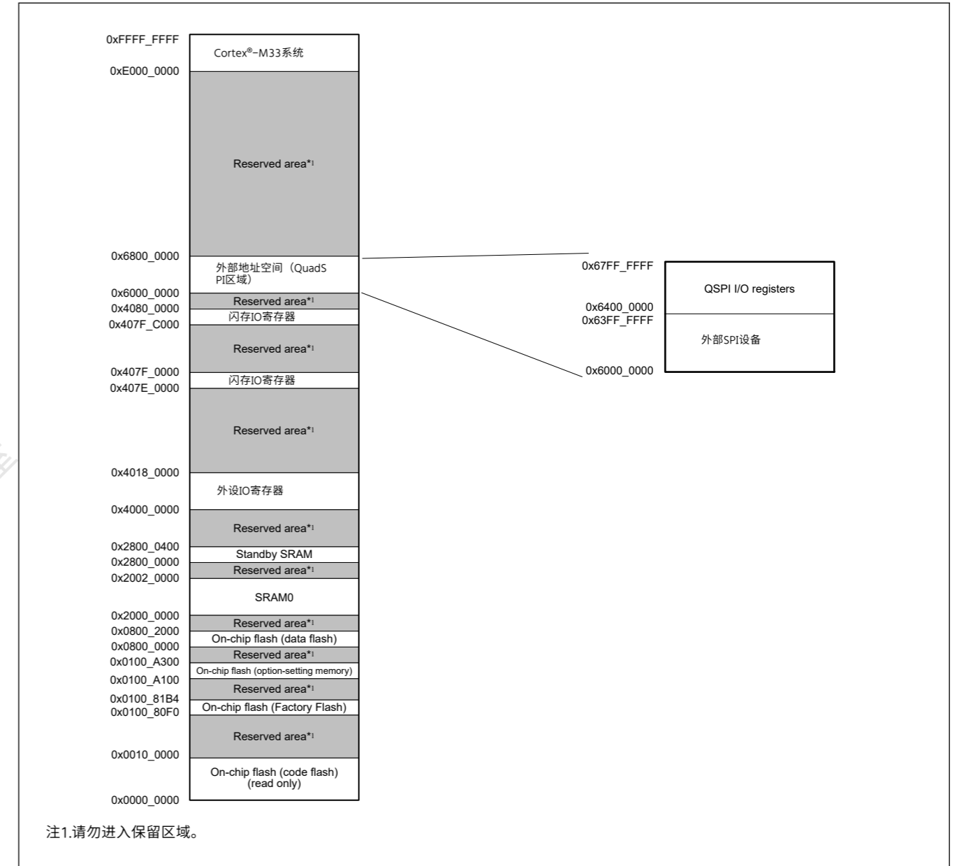
Figure 4.2 外部地址空间之间的关联
