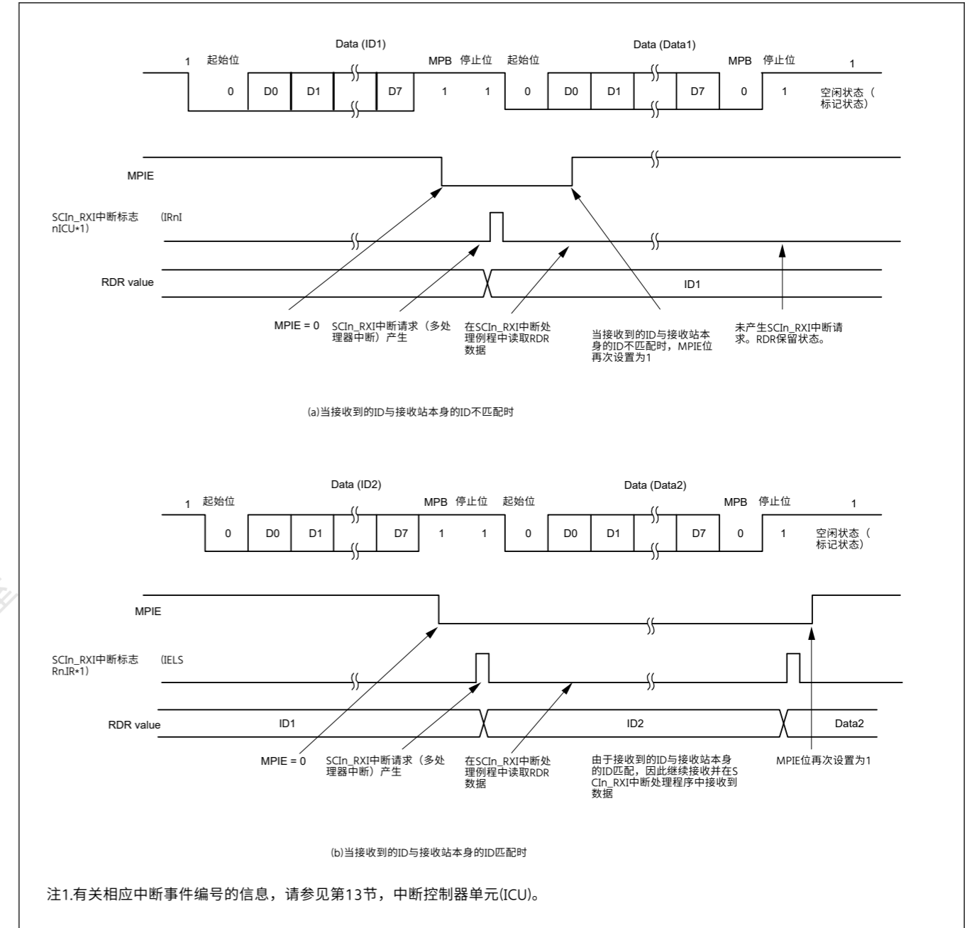
Figure 27.44 使用8位数据、多处理器位和1个停止位的SCI接收示例
