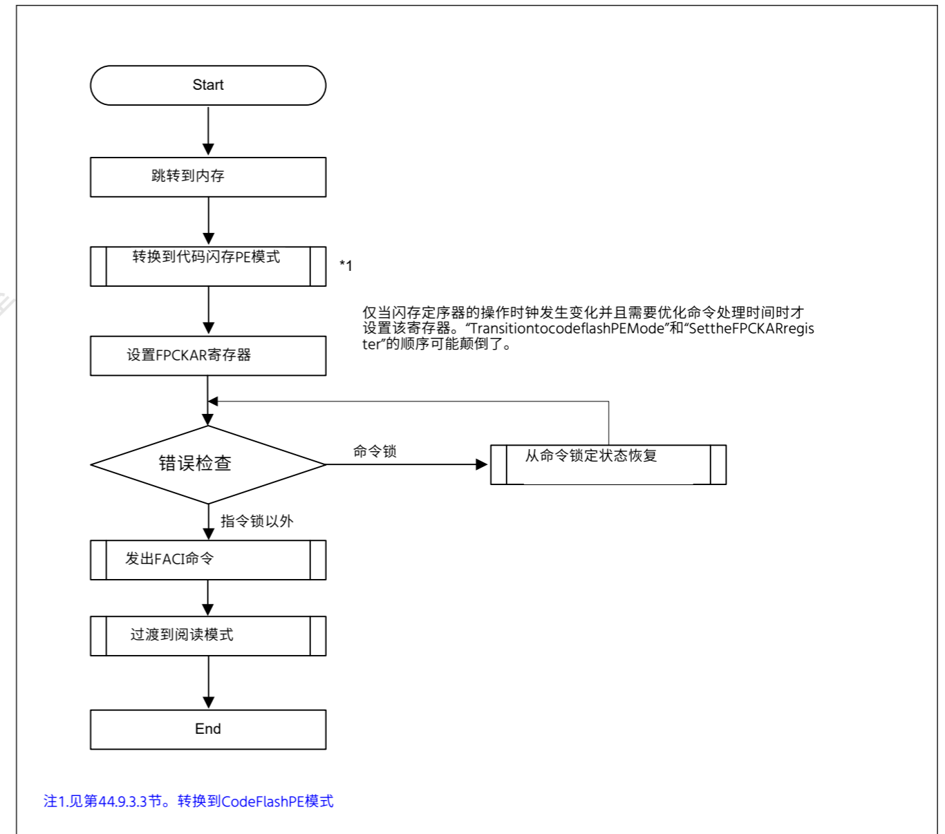
Figure 44.7 CodeflashPE模式下的命令使用概述
