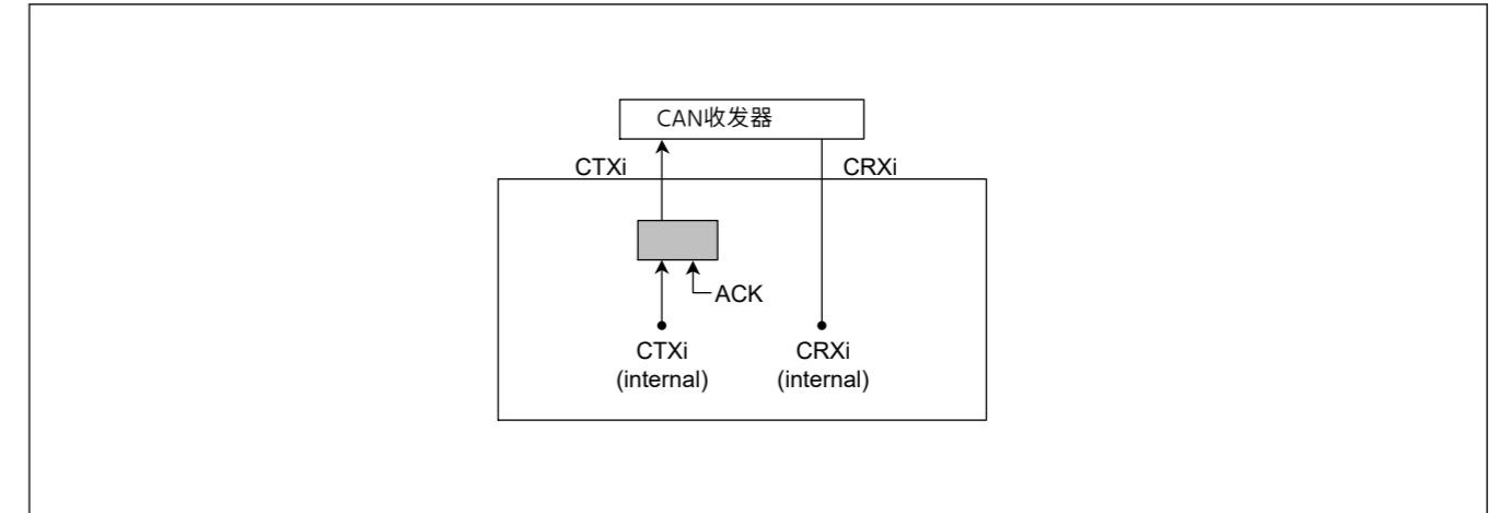
Figure 29.7 选择自检模式0时的连接(i=0 1)
