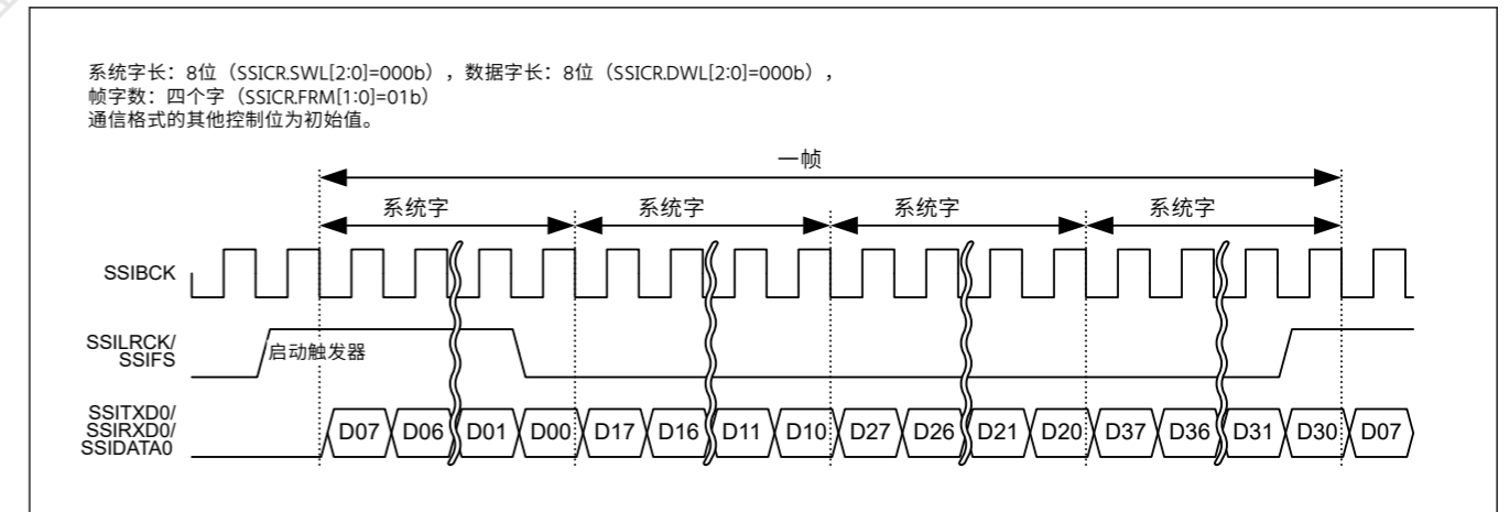
Figure 32.41 TDM格式 (无填充: 系统字长=数据字长)
