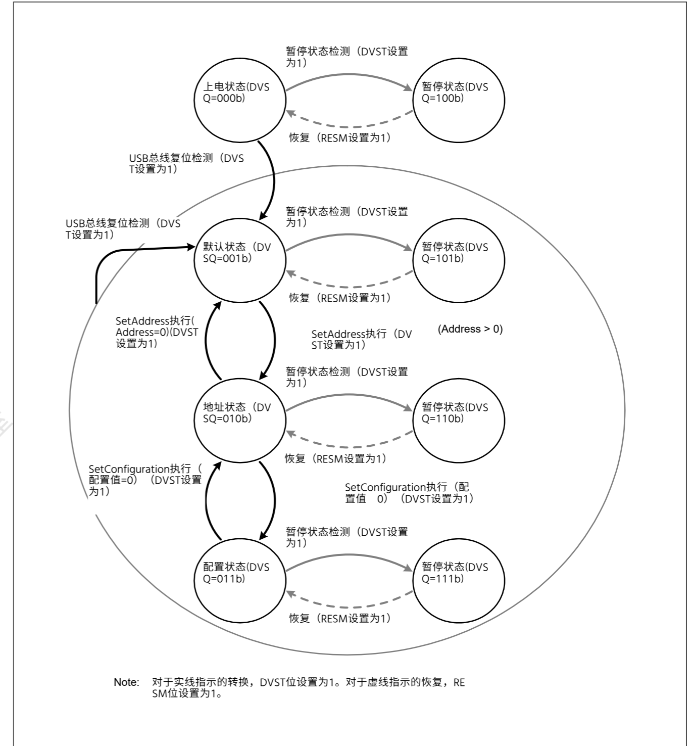
Figure 26.15 设备状态转换
