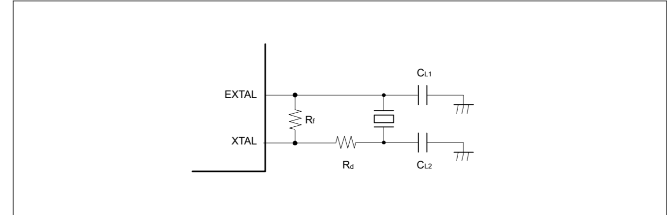
Figure 8.2 晶体谐振器连接示例
