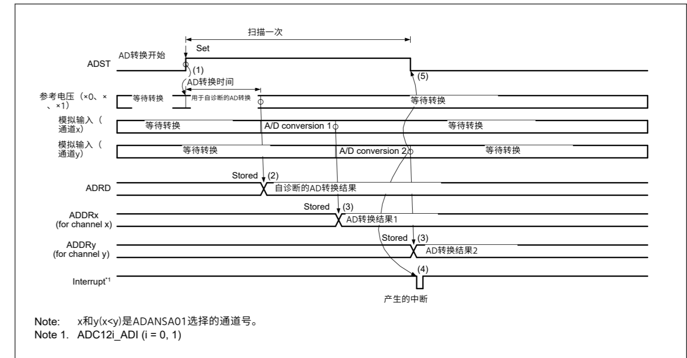
Figure 37.9 使用自诊断选择模拟输入（通道x和y）时单次扫描模式下的基本操作示例
