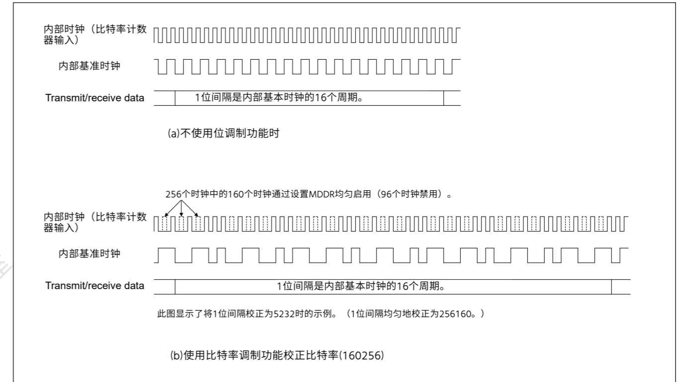
图27.100使用比特率调制功能时的内部基准时钟示例
