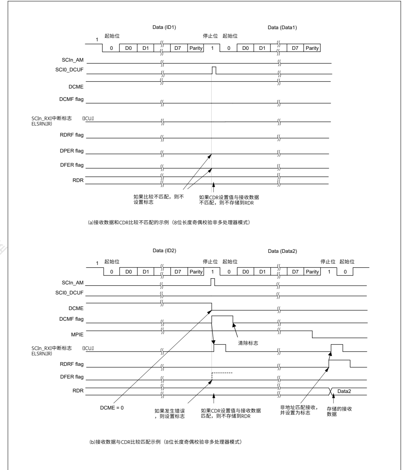
Figure 27.9 地址匹配示例 (一) 普通模式
