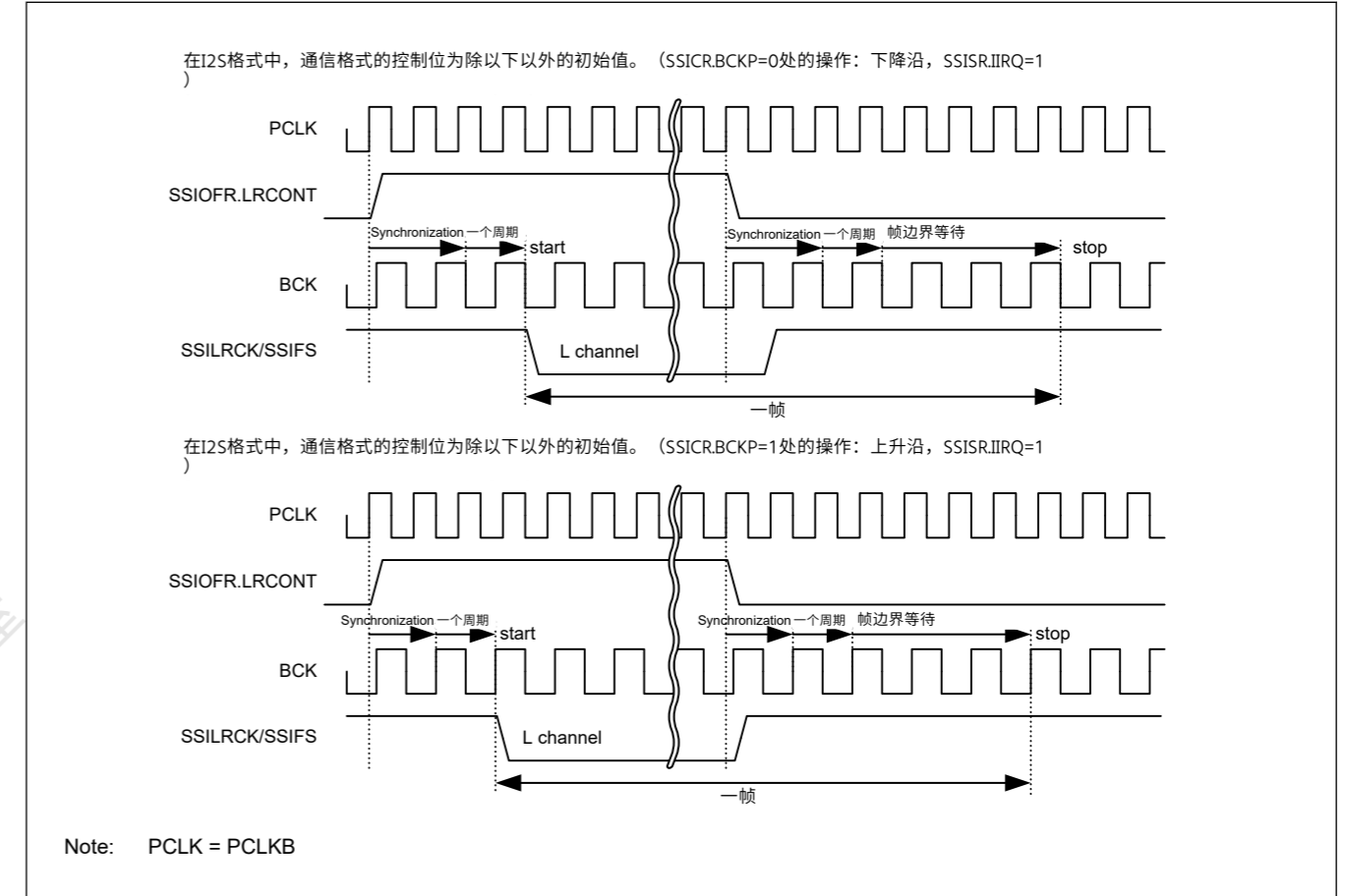
Figure 32.44 通过SSIOFR.LRCONT禁用LR时钟帧同步继续的示例
