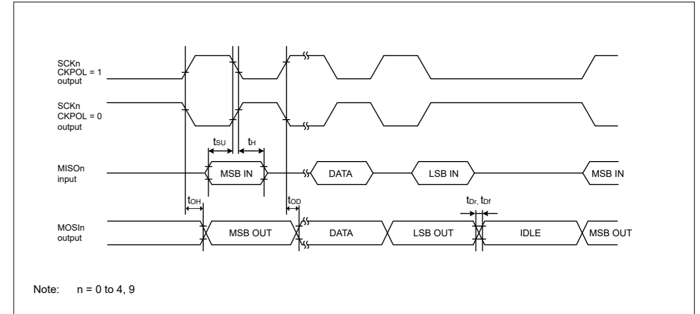
Figure 47.30 CKPH=0时主机的SCI简单SPI模式时序
