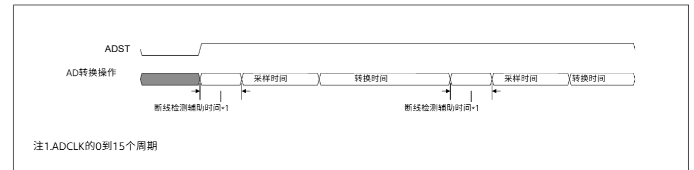
Figure 37.33 使用断线检测辅助功能时的AD转换动作
