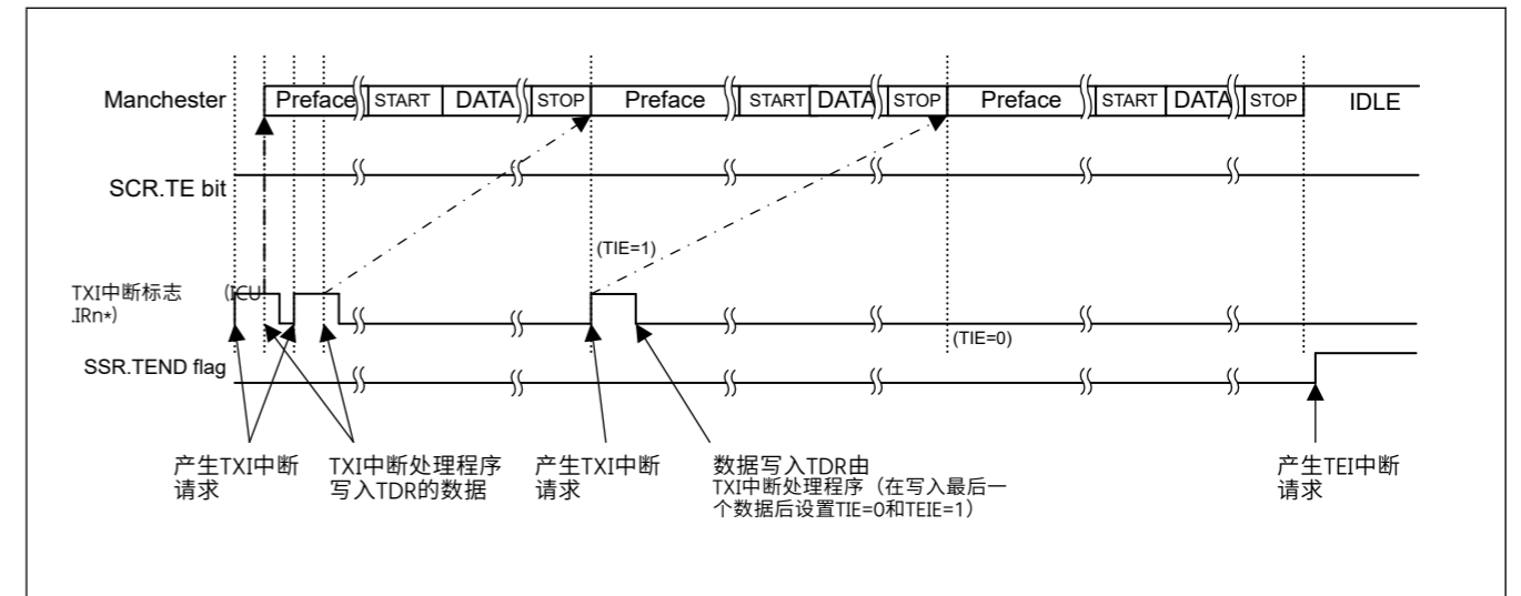
Figure 27.58 曼彻斯特模式下串行传输的传输结束操作示例 (使用前言但没有CTS功能)
