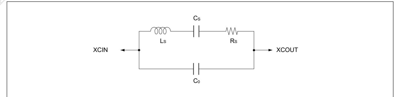
Figure 8.6 32.768kHz晶体谐振器的等效电路
