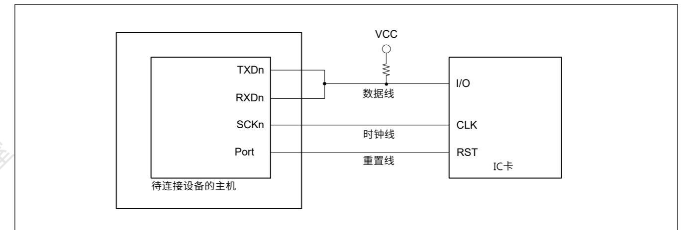
Figure 27.77 与智能卡（IC卡）的连接示例
