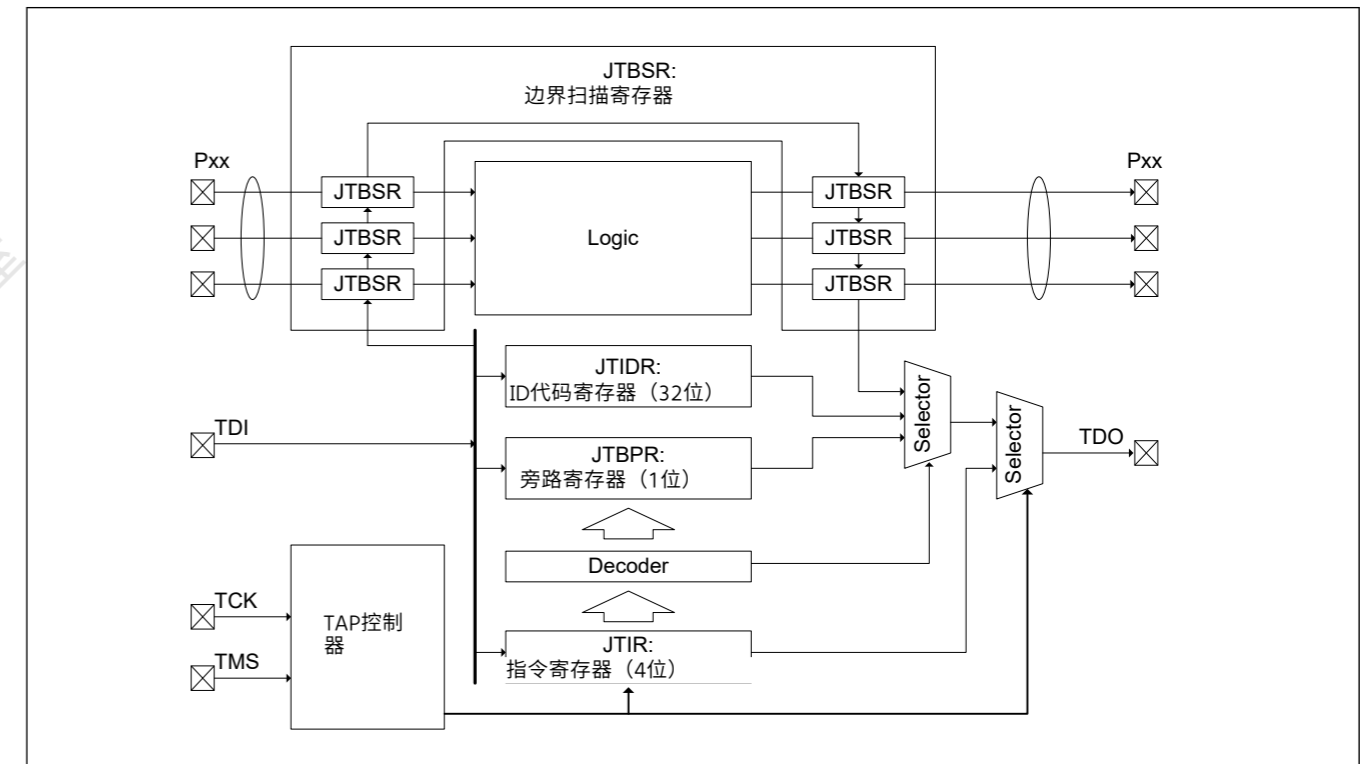
Figure 35.1 边界扫描功能框图
