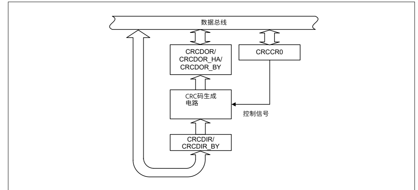
Figure 34.1 CRC计算器框图
