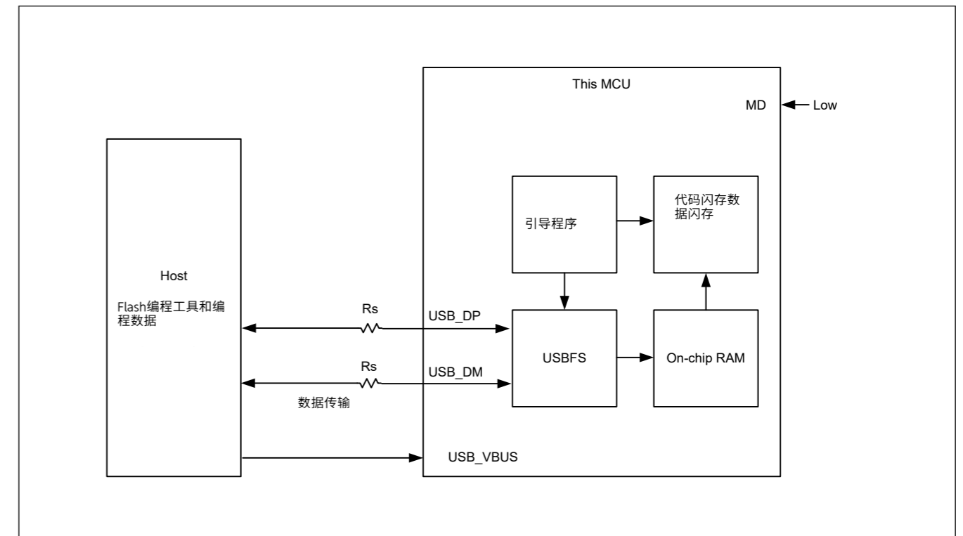
Figure 44.41 引导模式下的系统配置（用于USB接口）
