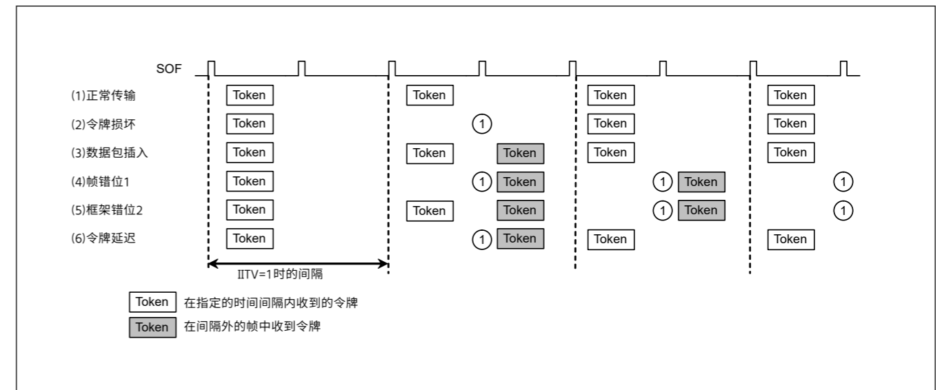
Figure 26.23 IITV=1时发生的示例间隔错误
