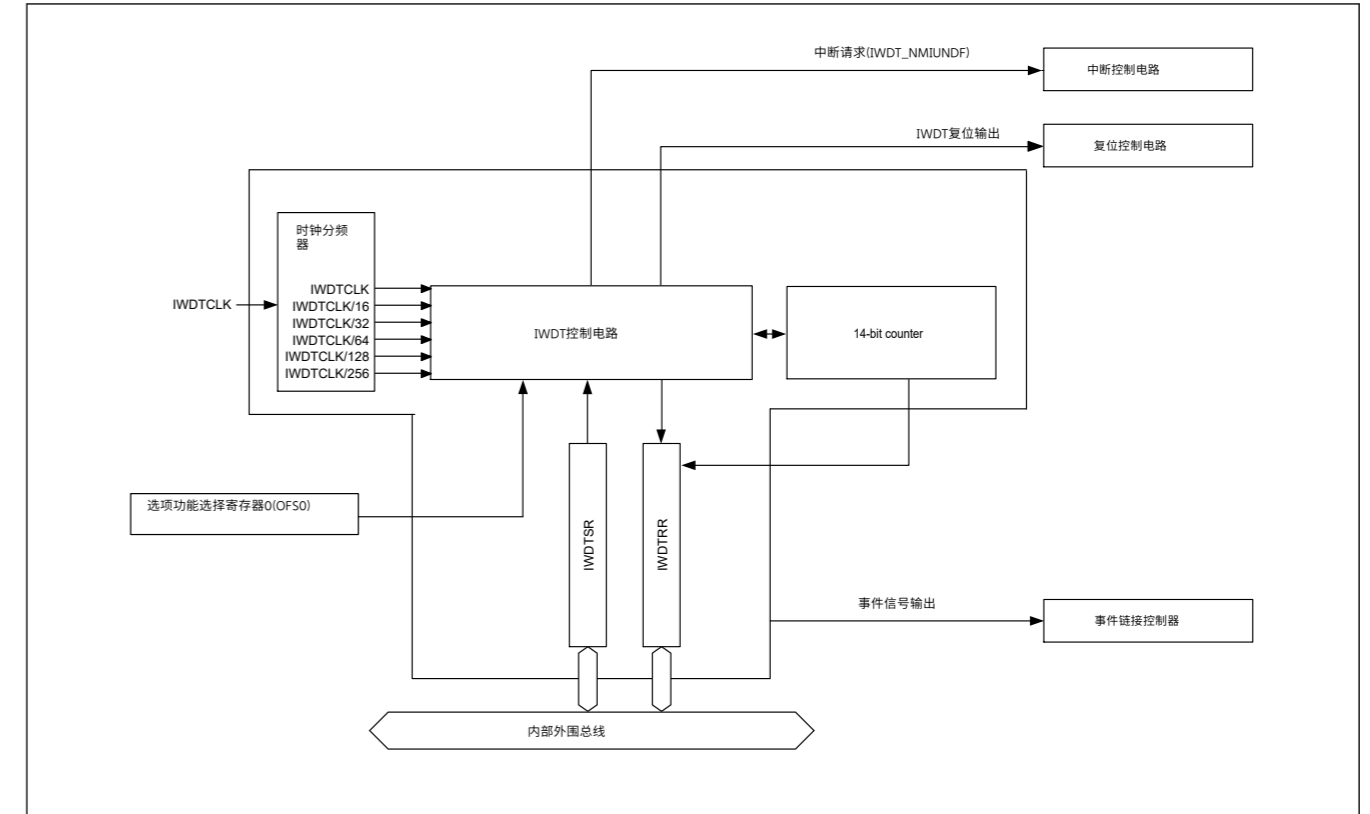
Figure 25.1 IWDT框图
