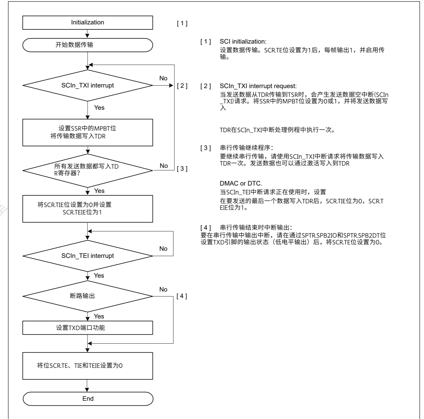
Figure 27.41 选择非FIFO的多处理器串行传输示例流程
