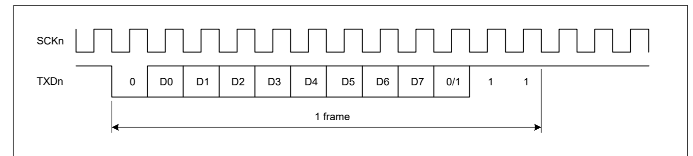
Figure 27.8 异步模式下输出时钟与传输数据的相位关系 SMR.CHR=0, PE=1, MP=0, STOP=1
