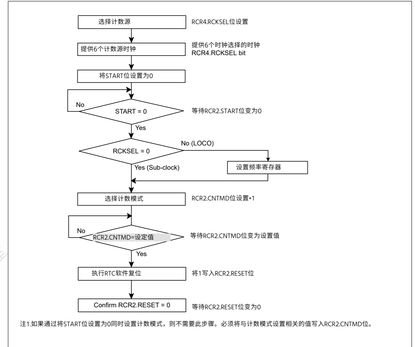
Figure 23.3 时钟和计数模式设置程序
