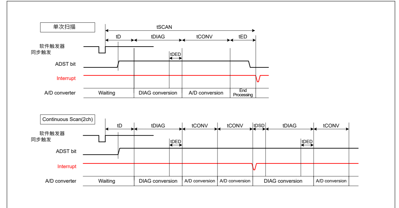
Figure 37.31 由软件或同步触发输入(ELC)激活时的扫描转换时序
