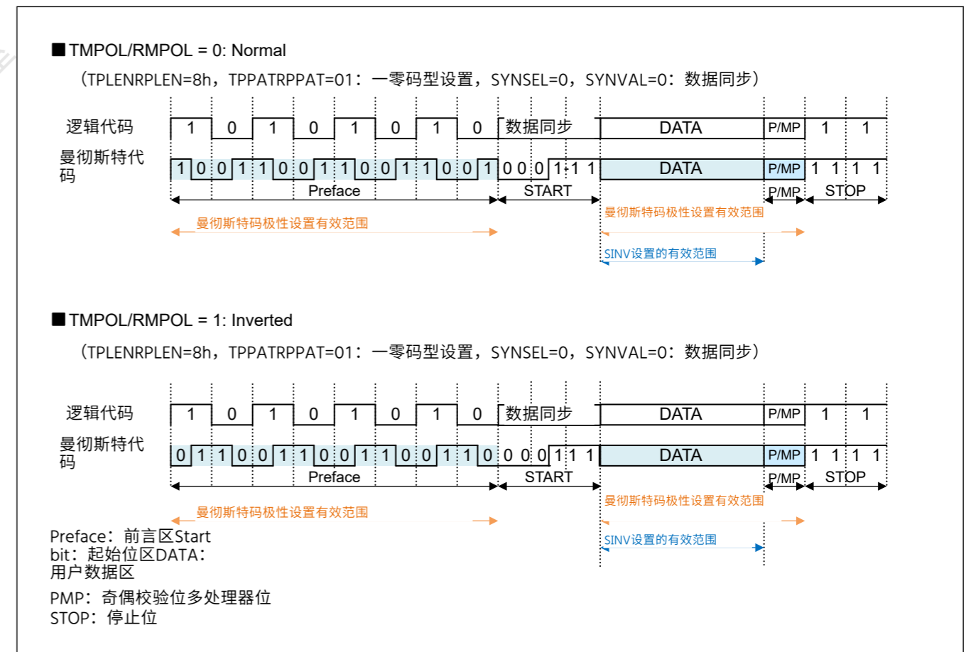
Figure 27.64 曼彻斯特码极性设置的有效范围
