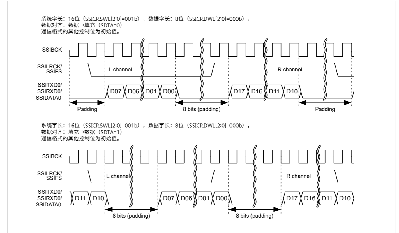
Figure 32.10 串行数据的对齐设置与填充位
