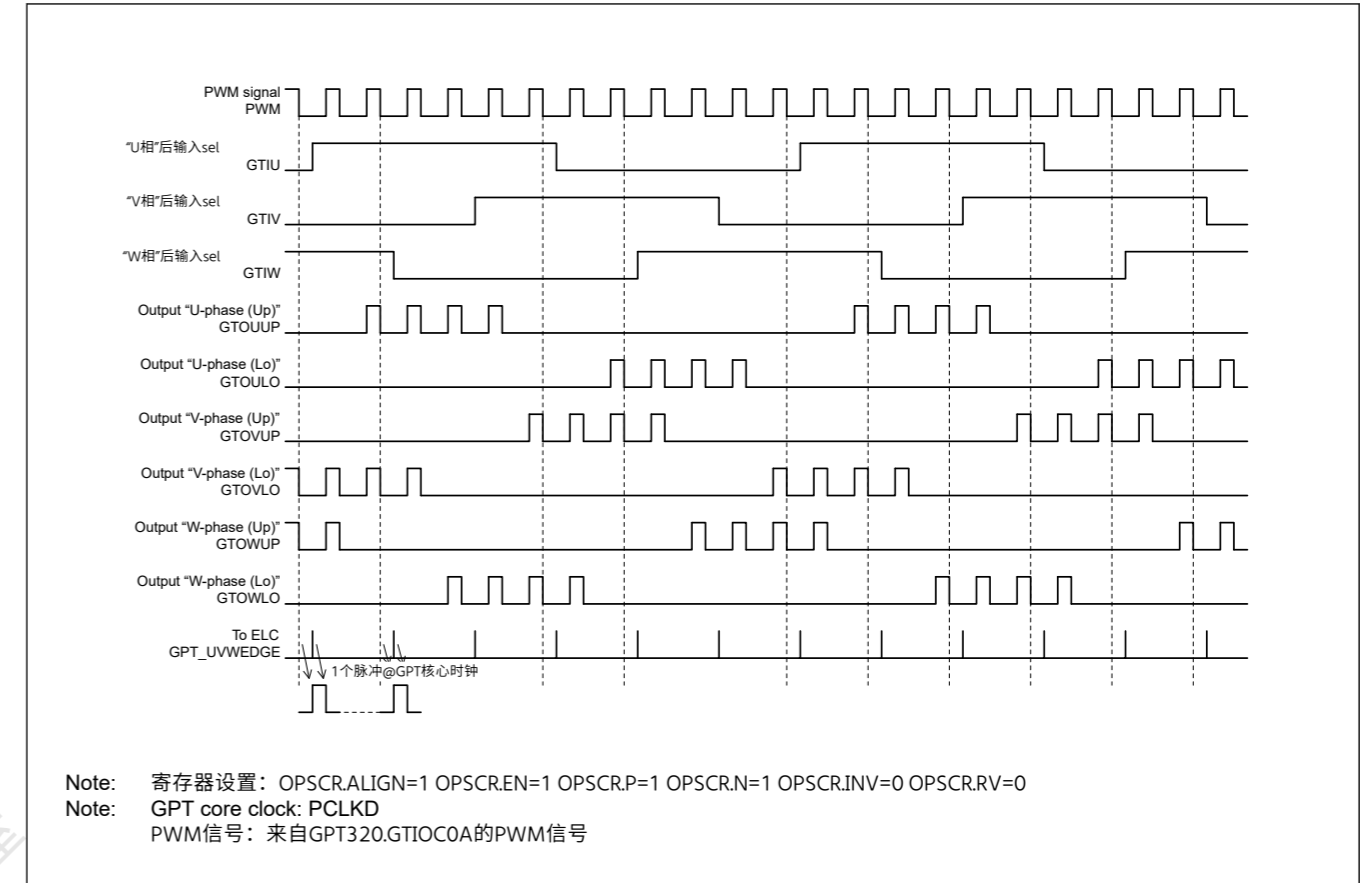
Figure 21.59 带斩波器控制的6相PWM输出操作示例
