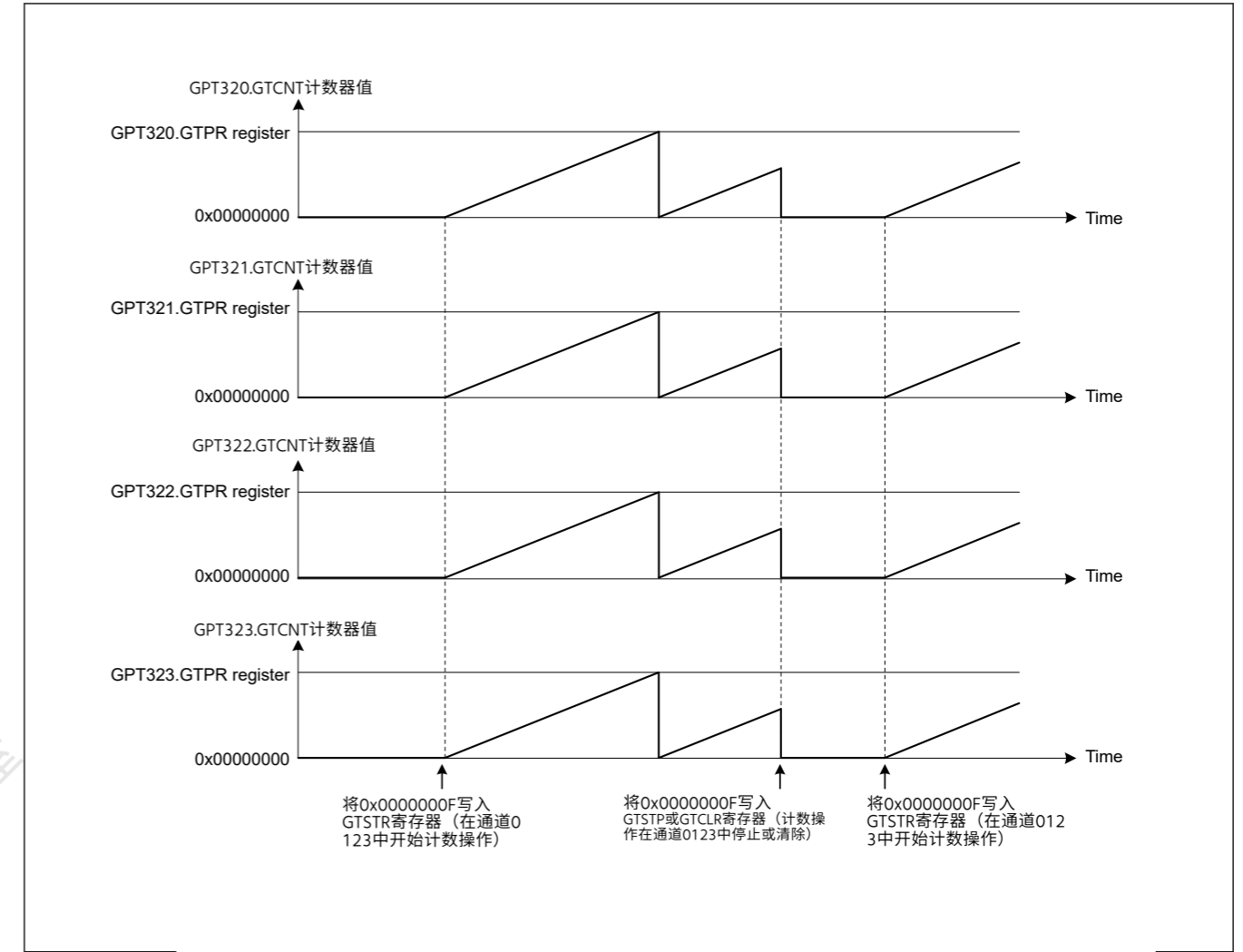
Figure 21.36 使用相同计数周期 (GTPR寄存器值) 的软件同时启动、停止和清除的示例
