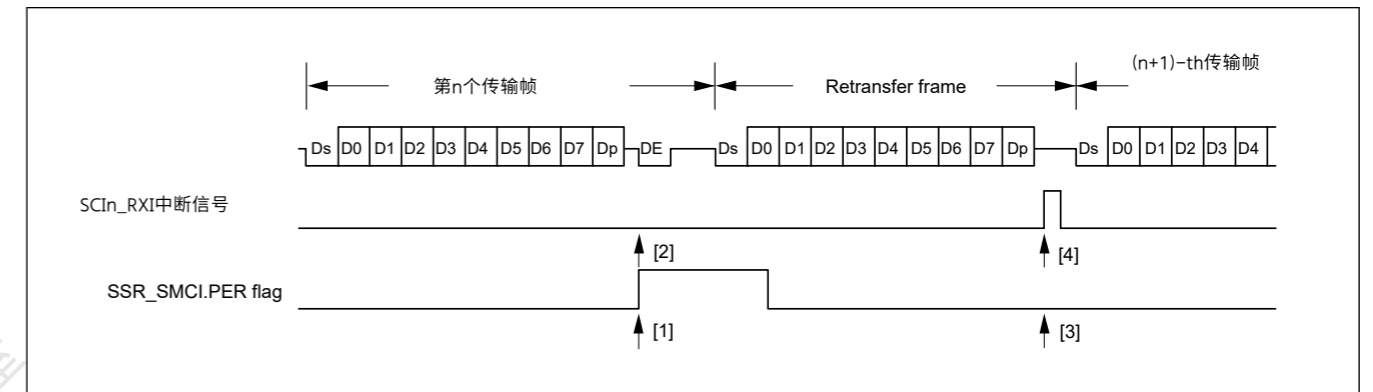
Figure 27.85 智能卡接口接收模式下的数据重传操作
