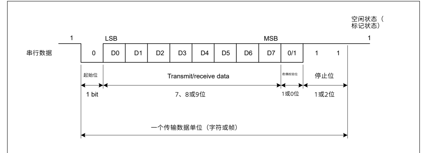
Figure 27.6 异步串行通信中的数据格式，包含8位数据、奇偶校验位和2个停止位
