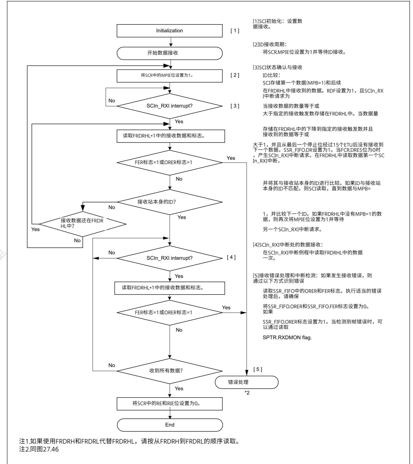
Figure 27.48 选择FIFO的多处理器模式下的串行接收示例流程
