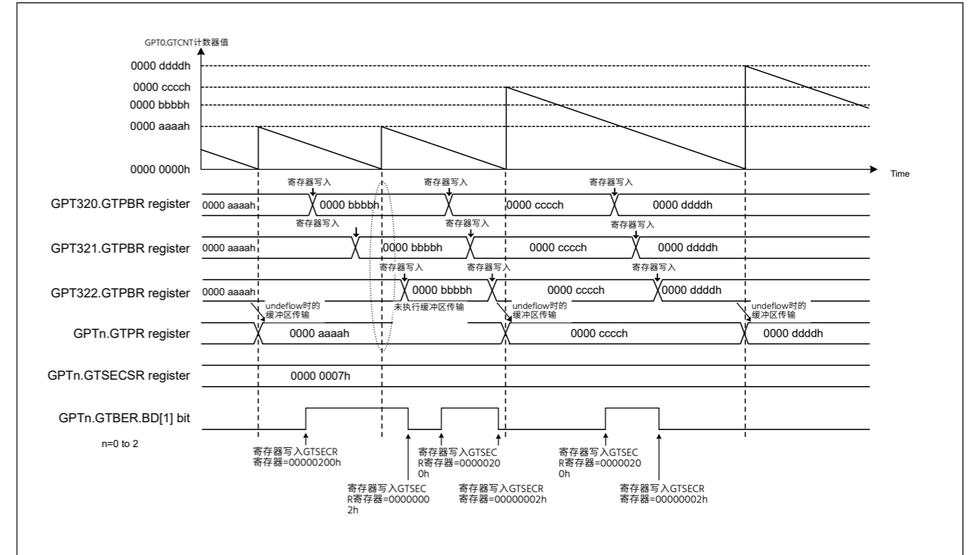
Figure 21.65 禁用缓冲区操作的多通道操作示例 (锯齿波, 单缓冲操作)
