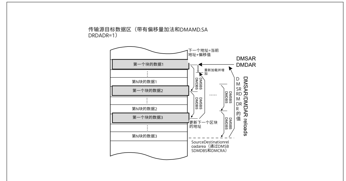
Figure 16.17 使用DMAMD.SADR和DMAMD.DADR=1进行偏移添加中的地址更新
