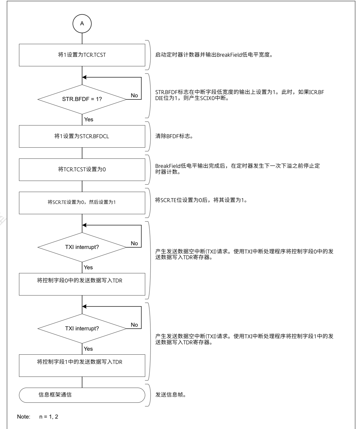
图27.104起始帧传输示例(2/2)
