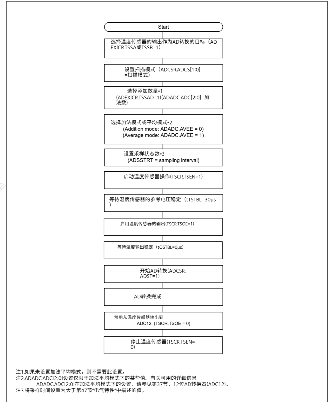
Figure 39.2 使用TSN的过程示例
