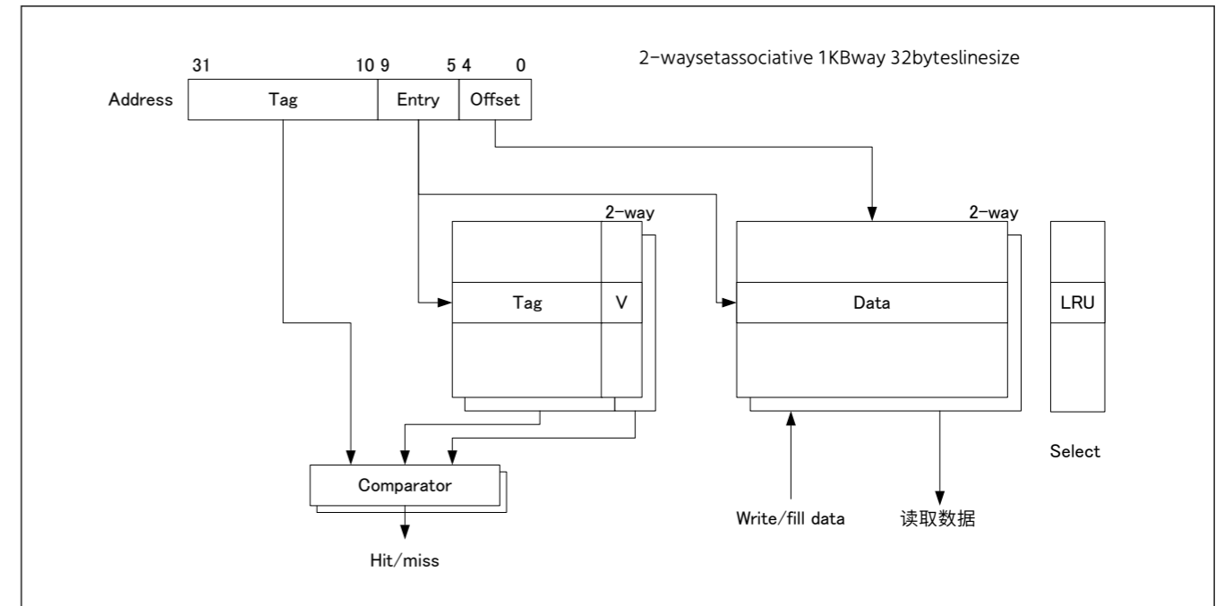
Figure 14.5 2KB容量和32字节行大小的2路组关联的缓存结构
