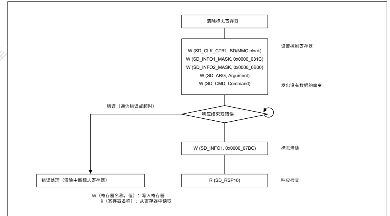
Figure 33.10 没有数据的命令流示例
