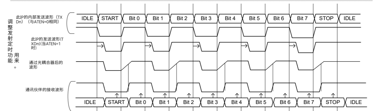
Figure 27.37 通过光电耦合器的发射波形的解释
