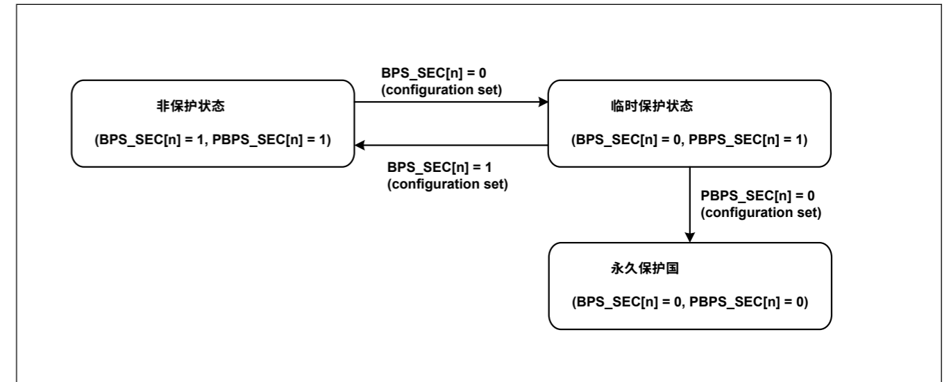
Figure 44.32 通过BPS_SEC[n]和PBPS_SEC[n]进行闪存定序器的状态转换
