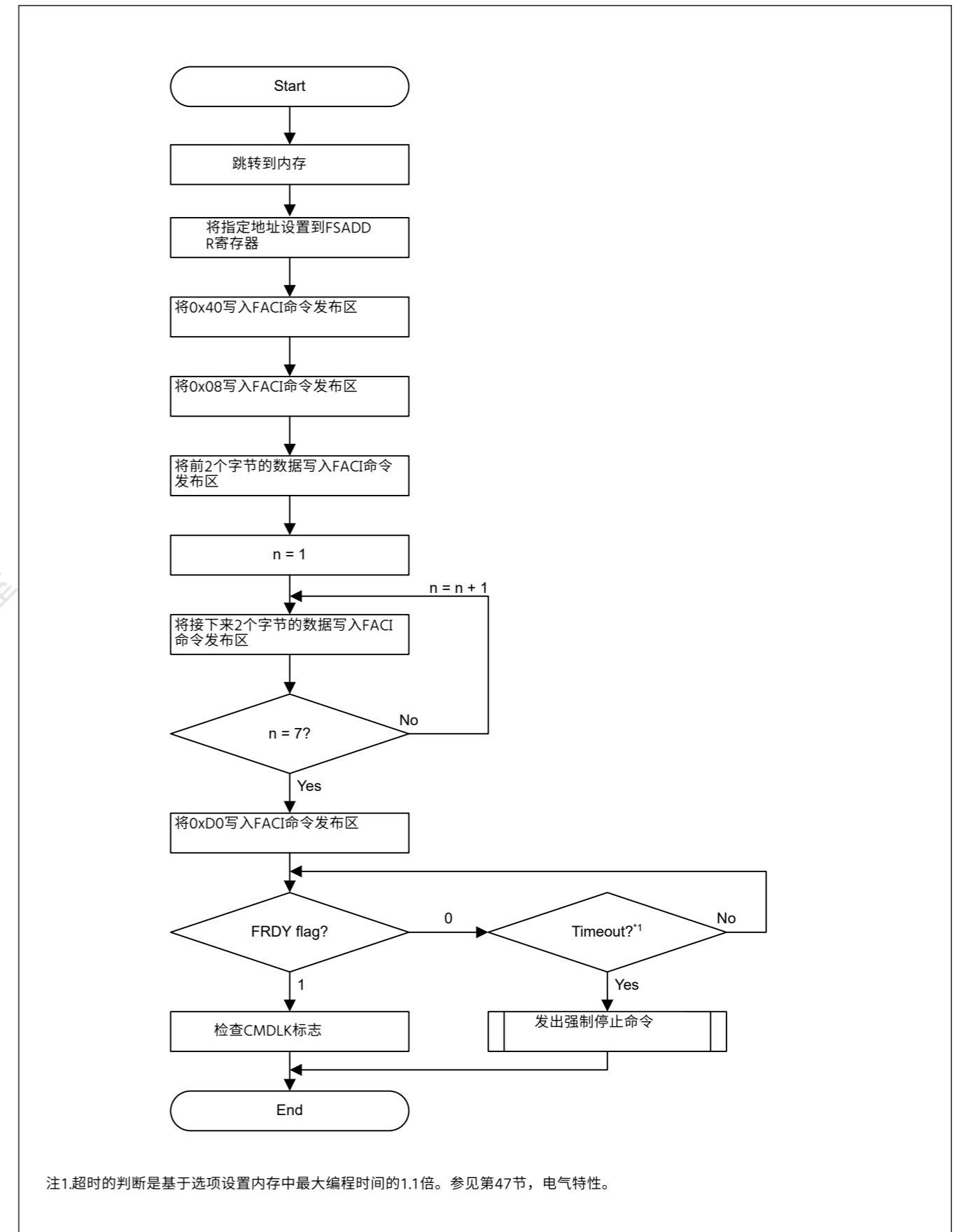
Figure 44.24 配置集命令使用流程
