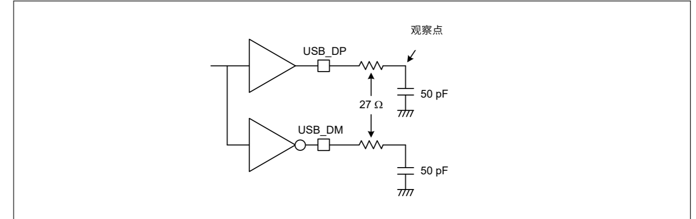
Figure 47.53 全速模式下的测试电路
