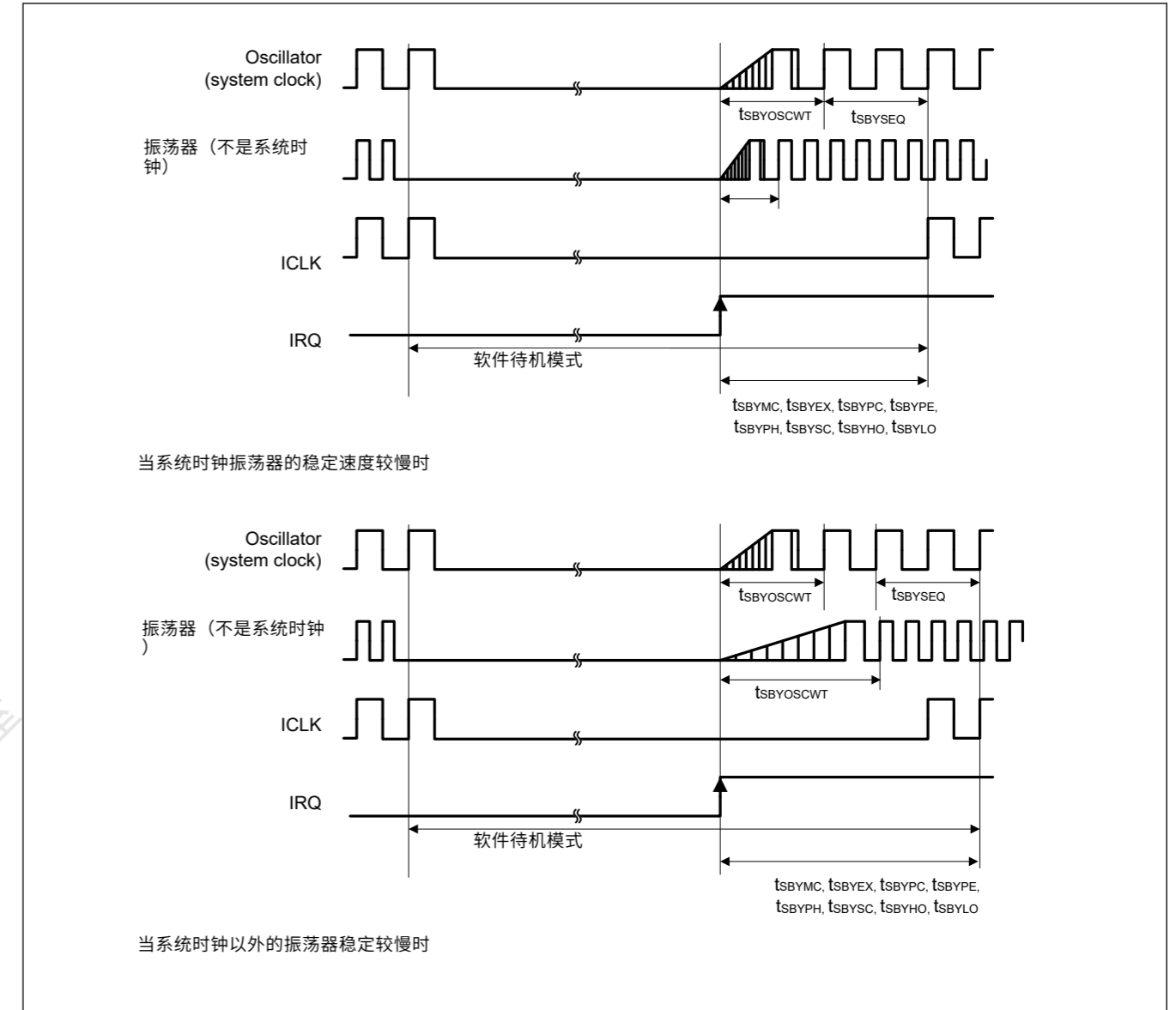
Figure 47.14 软件待机模式取消时序
