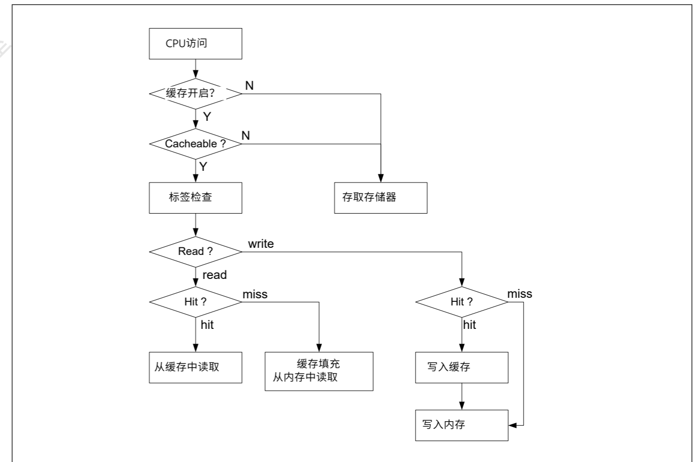
Figure 14.6 从CPU到S-cache的访问流程
