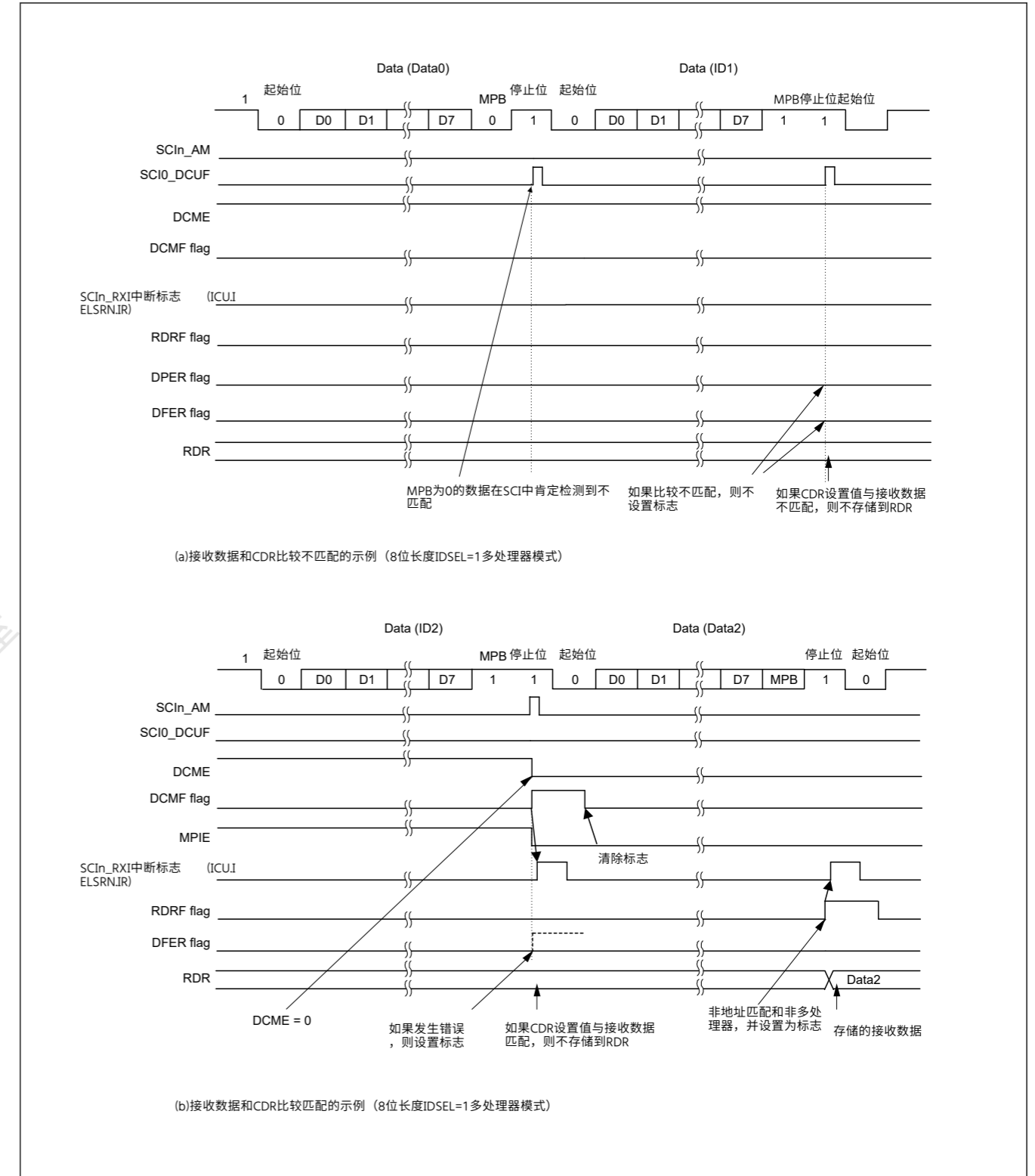
Figure 27.10 地址匹配示例 (二) 多处理器模式
