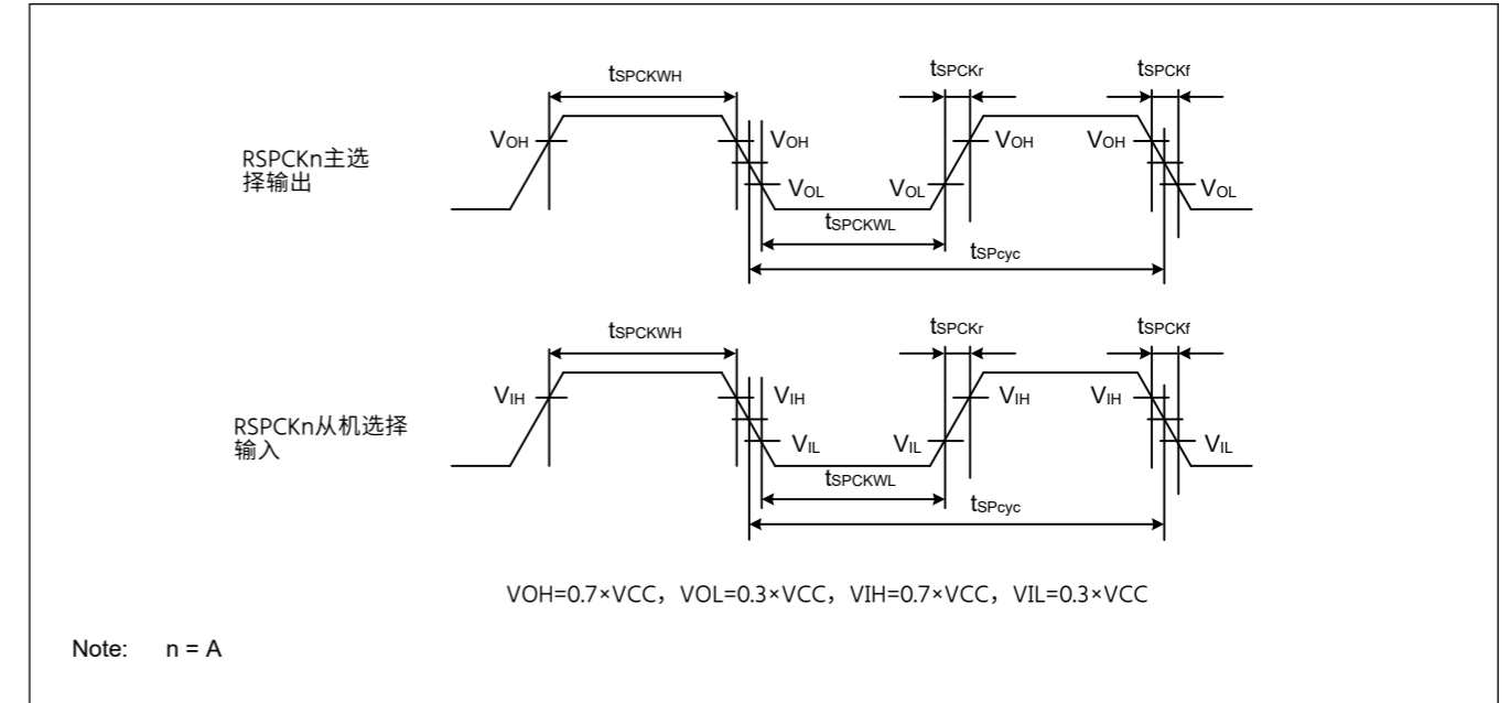
Figure 47.34 SPI时钟时序
