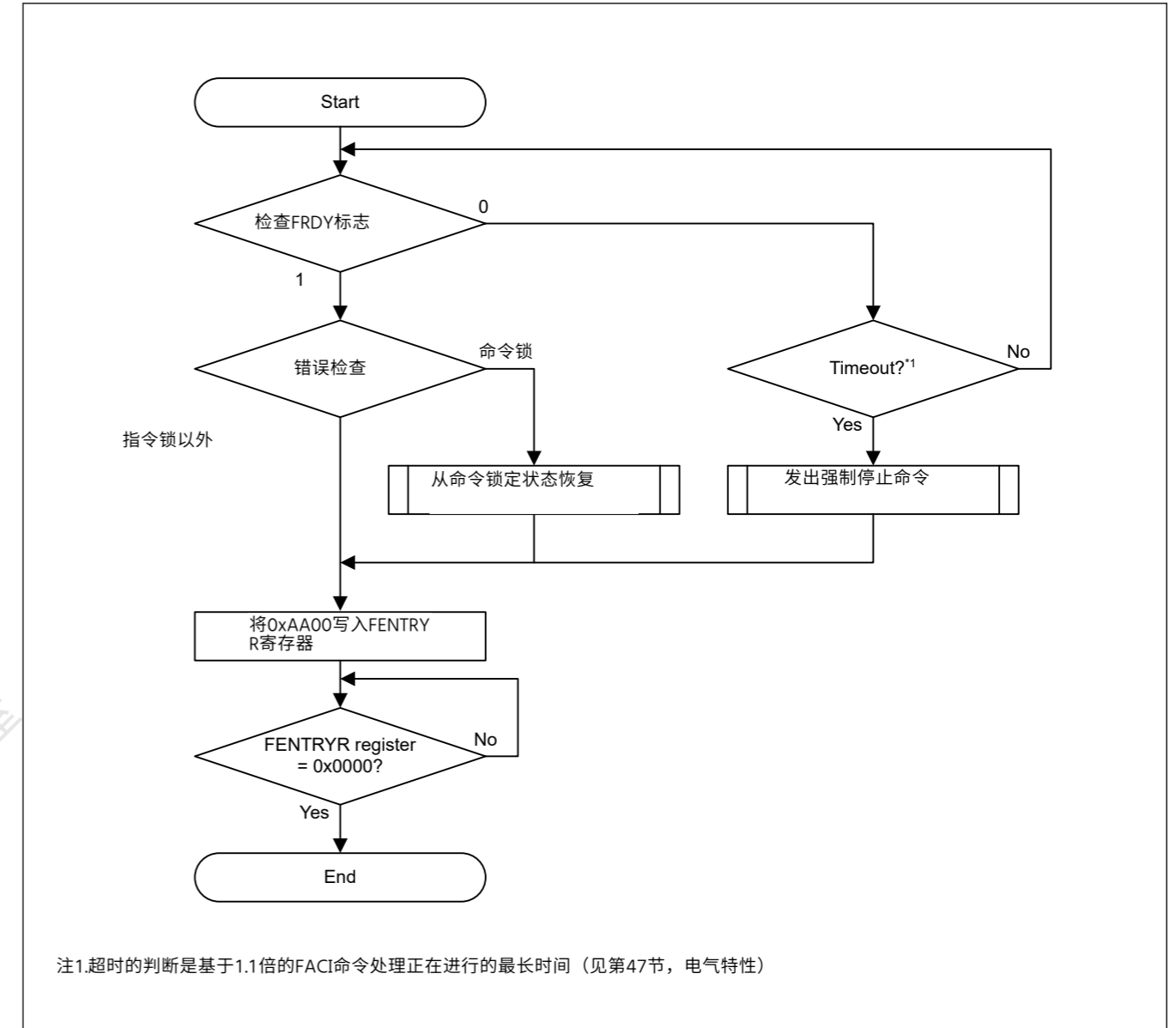
Figure 44.11 转换到阅读模式的过程
