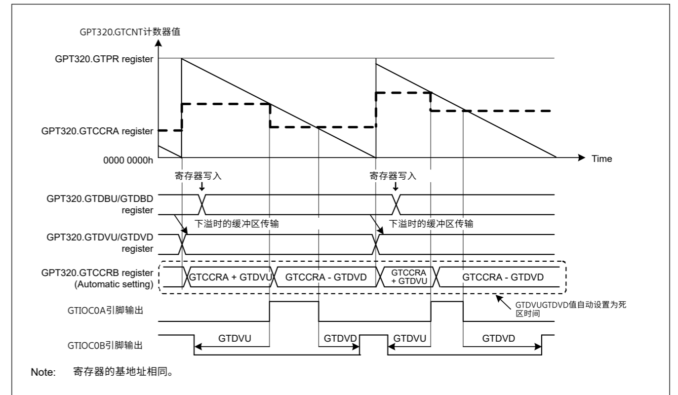
Figure 21.25 锯齿波单发脉冲模式、递减计数和高电平有效的自动死区时间设置功能操作示例
