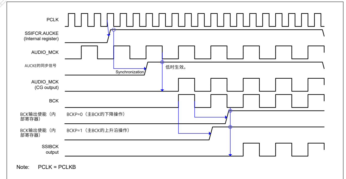
Figure 32.26 从系统复位到主模式通信开始的时序图
