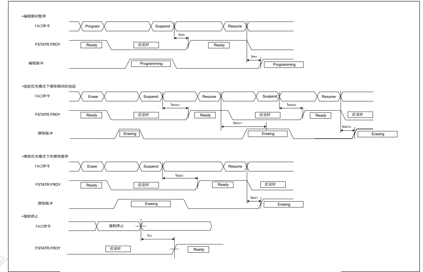
Figure 47.62 闪存编程和擦除的暂停和强制停止时序
