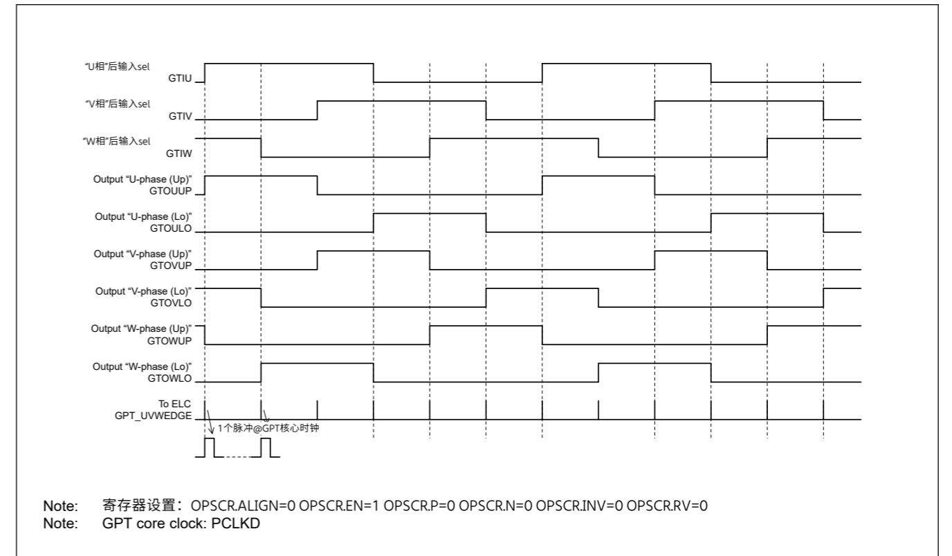
Figure 21.58 6相电平输出动作示例
