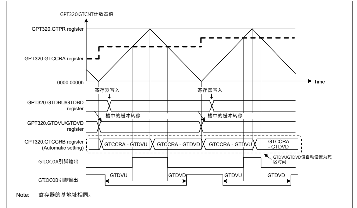
Figure 21.26 三角波中带死区时间的自动比较匹配值设置功能示例 PWM模式1, 高电平有效
