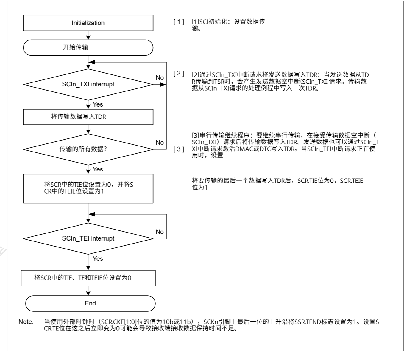
Figure 27.69 选择非FIFO的时钟同步模式下的串行传输示例流程
