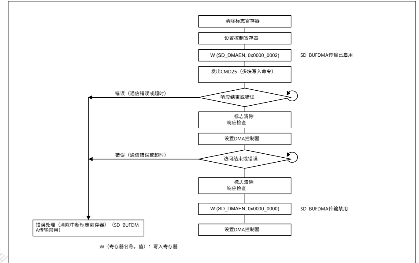
Figure 33.24 SD_BUF_DMA写操作示例
