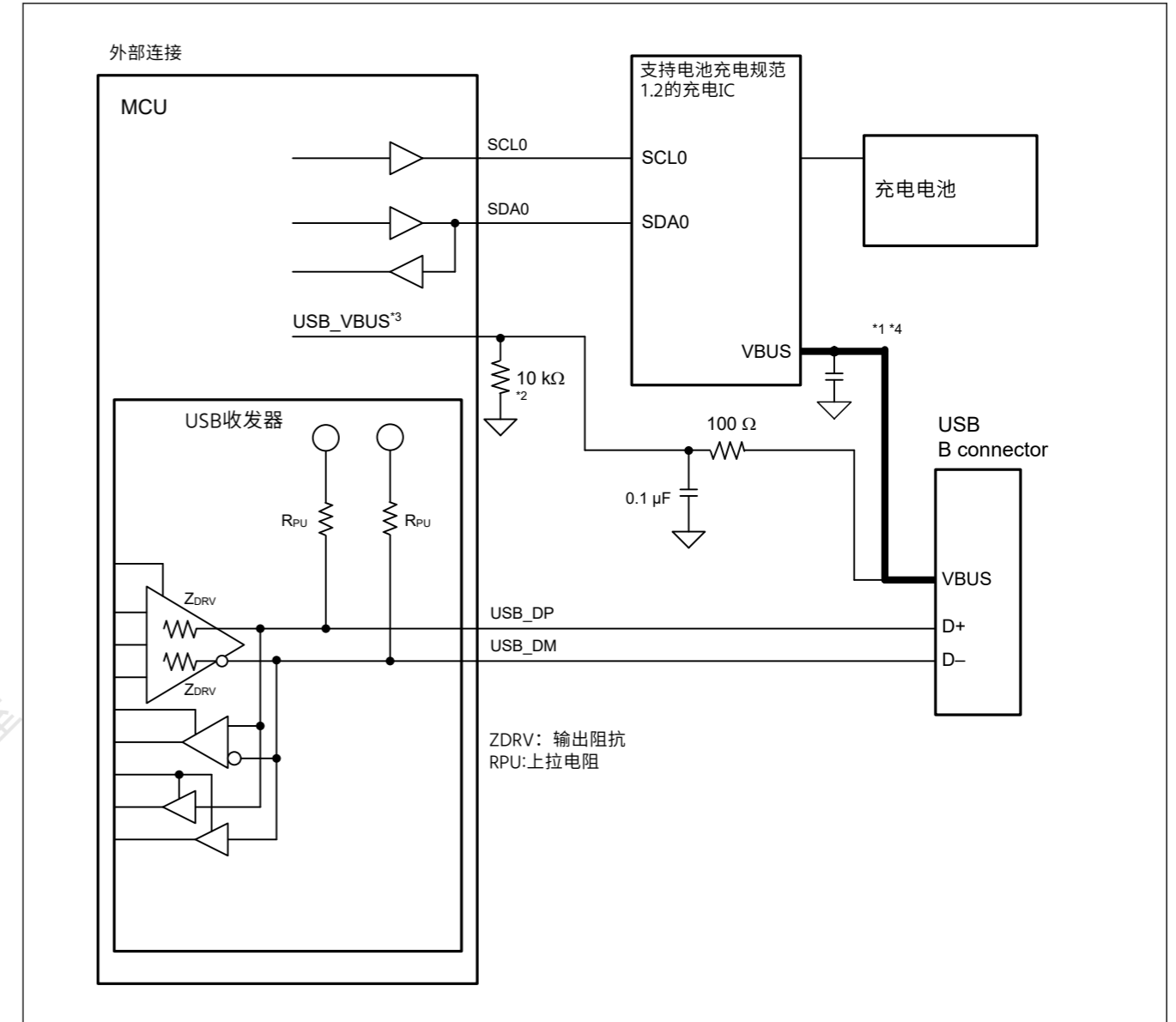
Figure 26.6 支持电池充电版本1.2的功能连接示例
