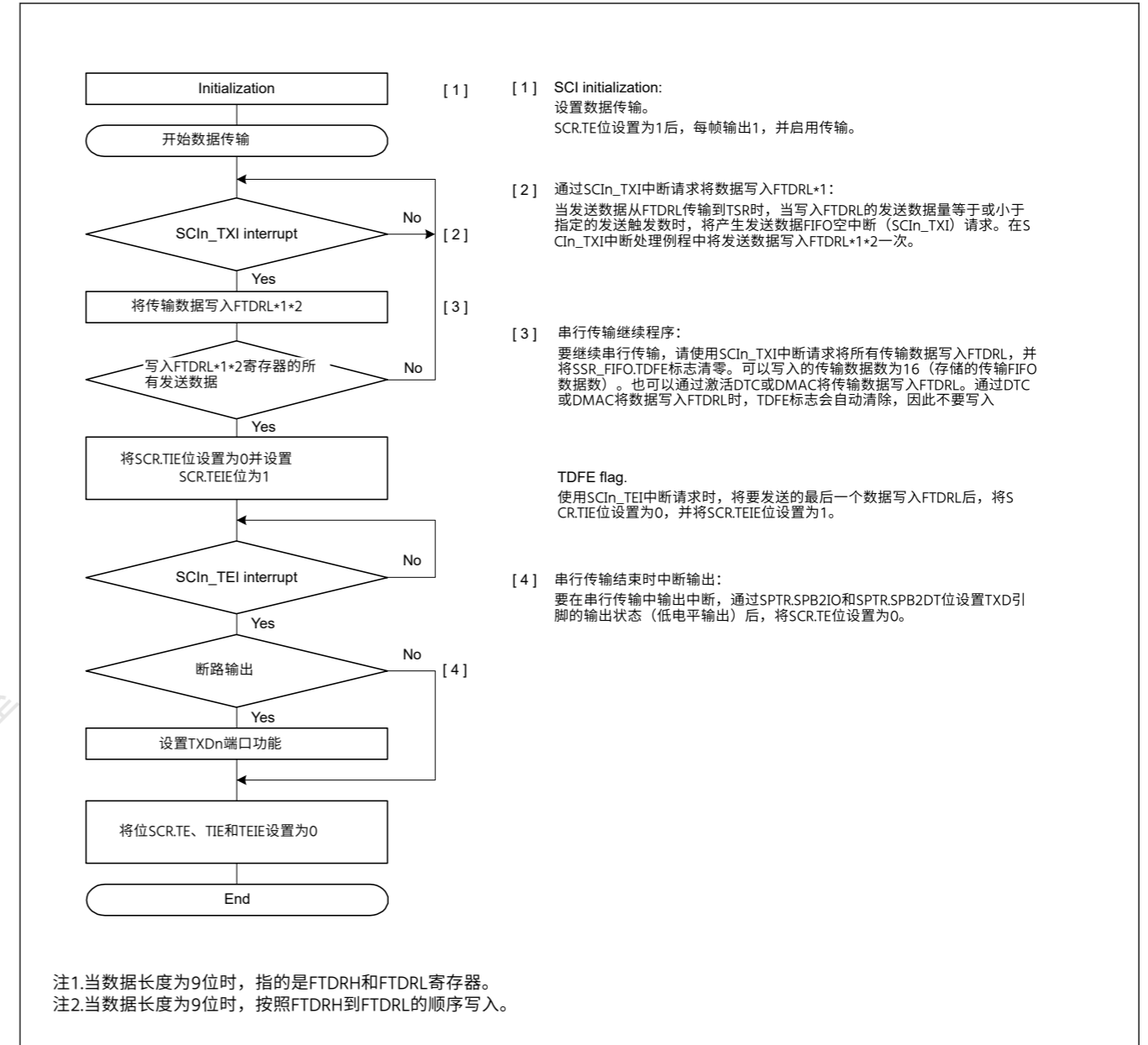
Figure 27.17 选择FIFO的异步模式下串行传输示例流程
