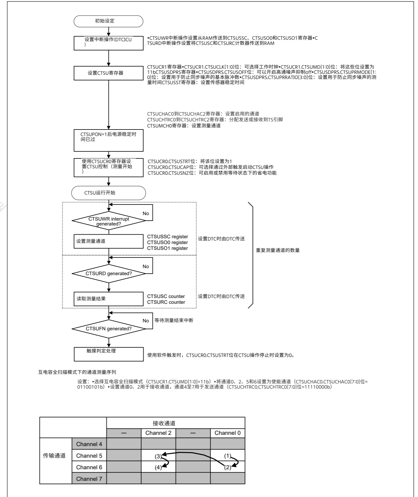
Figure 40.16 互电容全扫描模式的软件流程和示例操作
