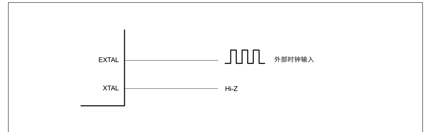
Figure 8.4 外部时钟等效电路
