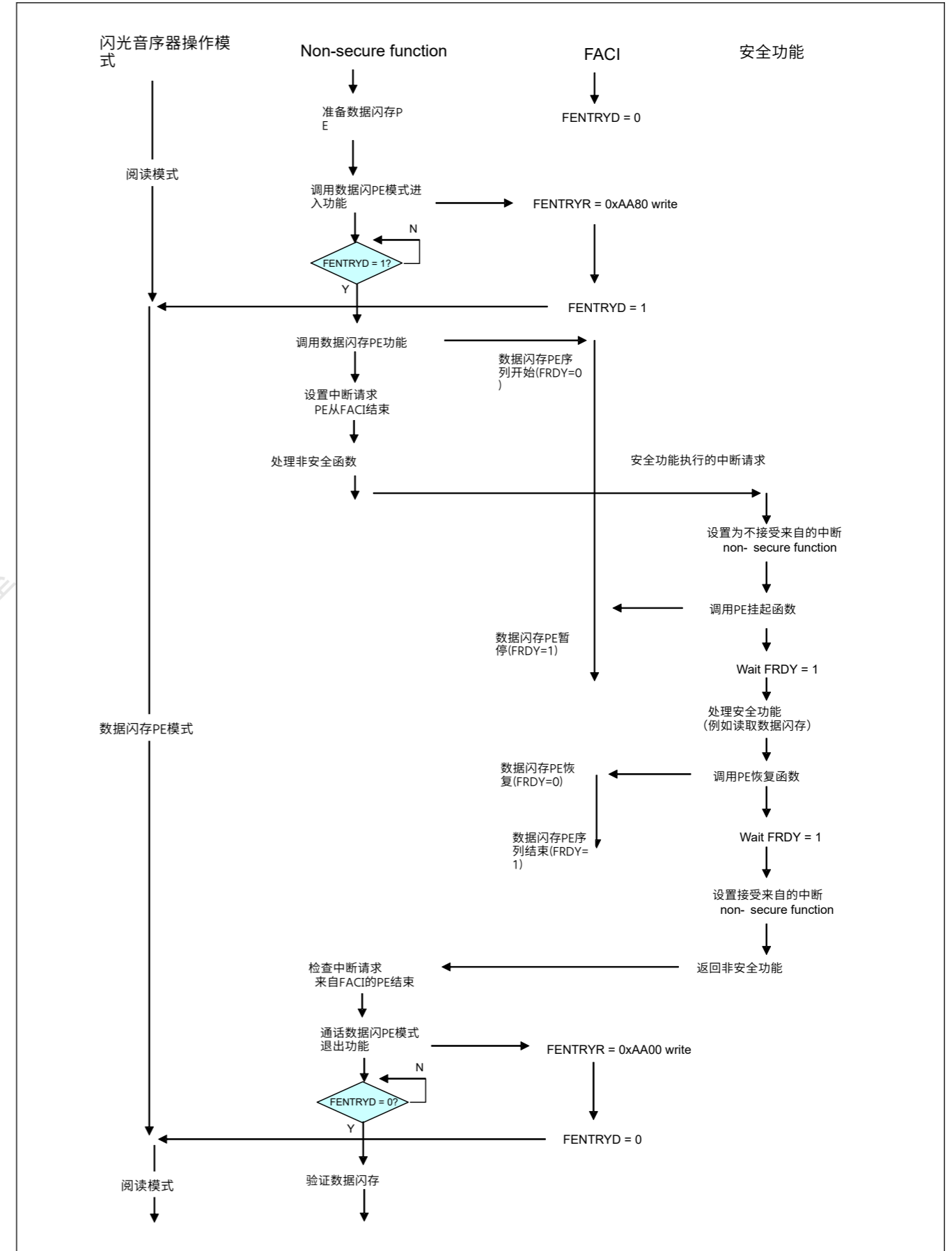
Figure 44.38 数据闪存PE安全功能暂停示例（检查中断请求以检测PE结束）
