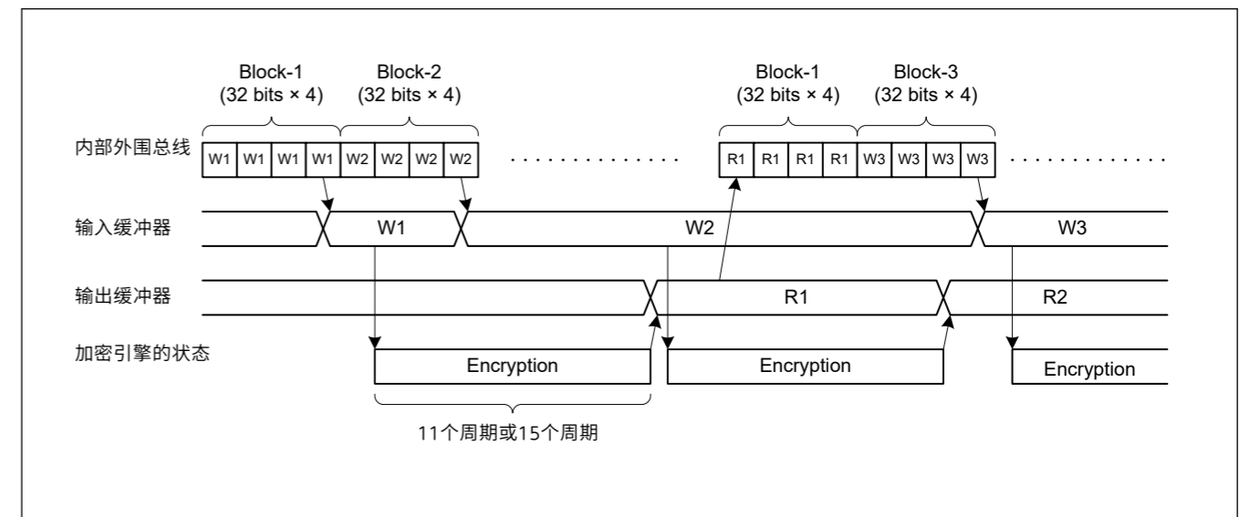
Figure 36.3 加密和解密时序 (AES)
