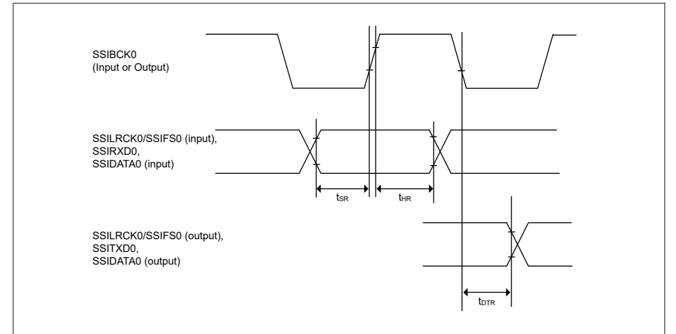
Figure 47.46 SSICR.BCKP=0时的SSIE数据发送和接收时序
