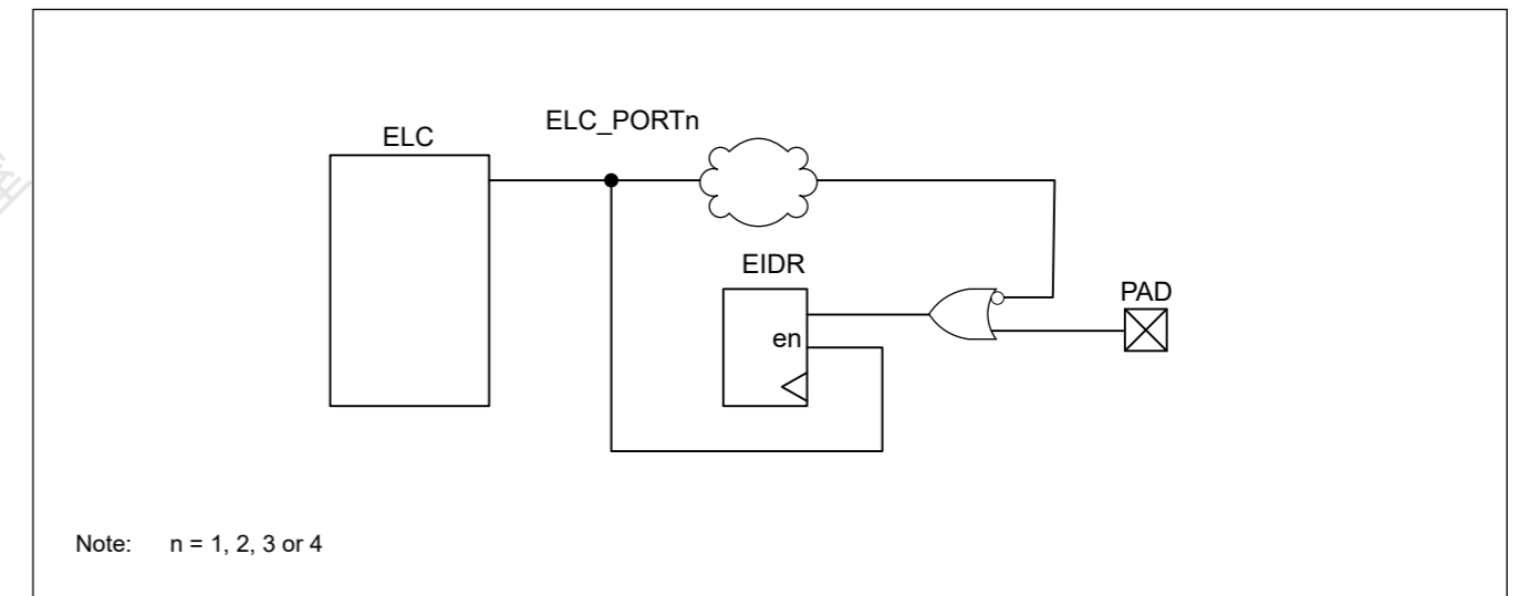
Figure 19.2 事件端口输入数据
