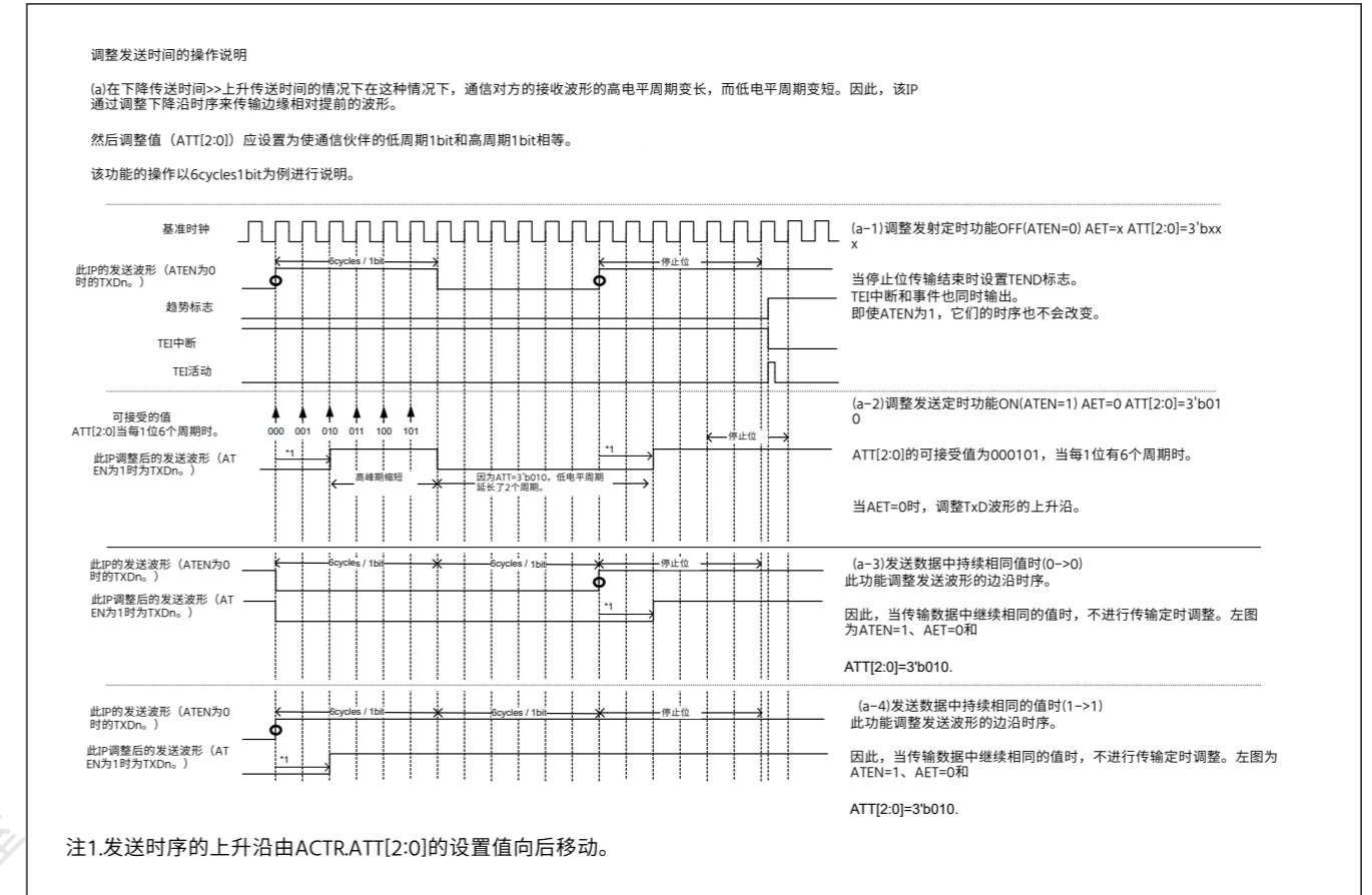
Figure 27.38 AET为0时发射时序调整操作说明
