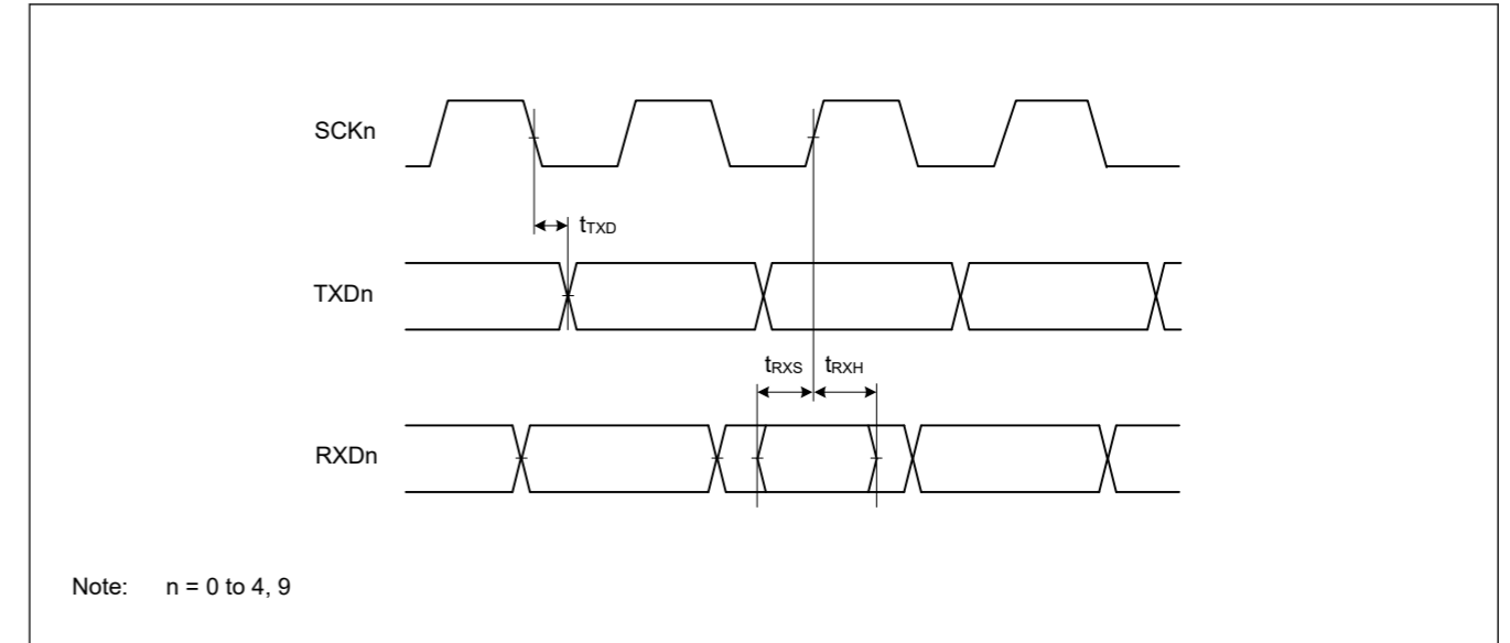
Figure 47.27 时钟同步模式下的SCI输入输出时序
