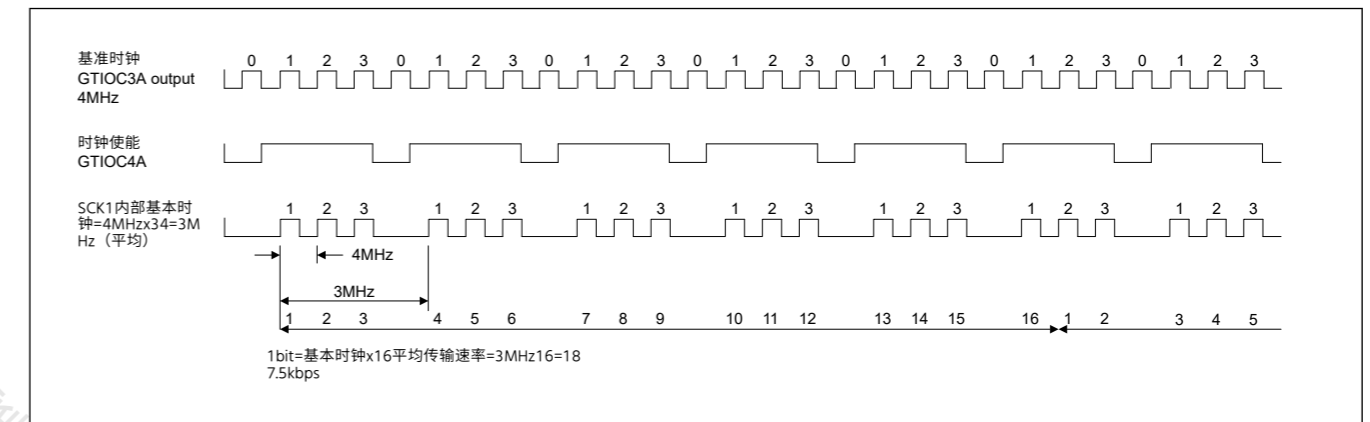
Figure 27.4 输入GPT时钟时的平均传输速率设置示例
