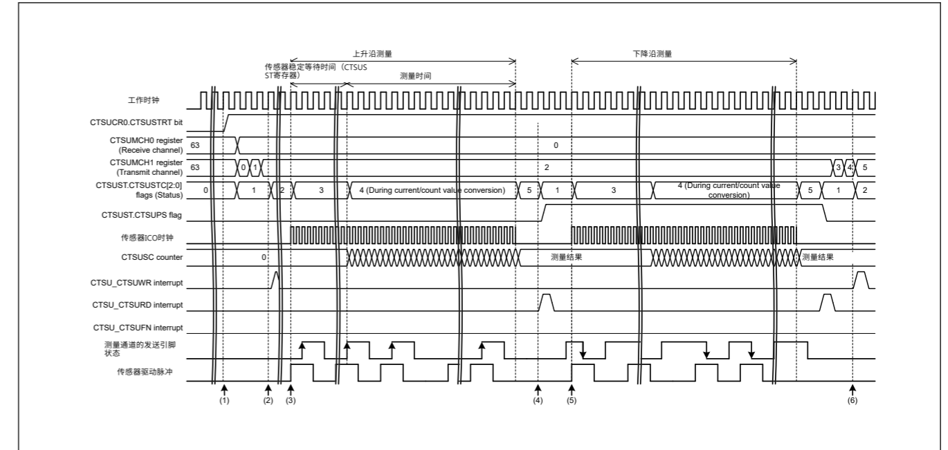
Figure 40.17 测量开始条件为软件触发时互电容全扫描模式的时序
