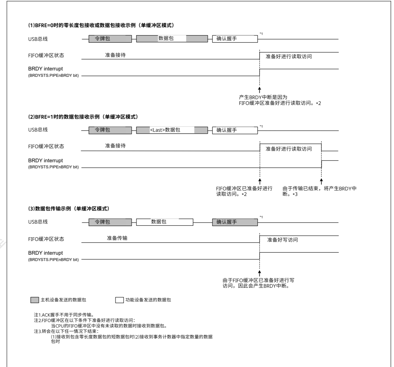
Figure 26.12 BRDY中断产生的时序
