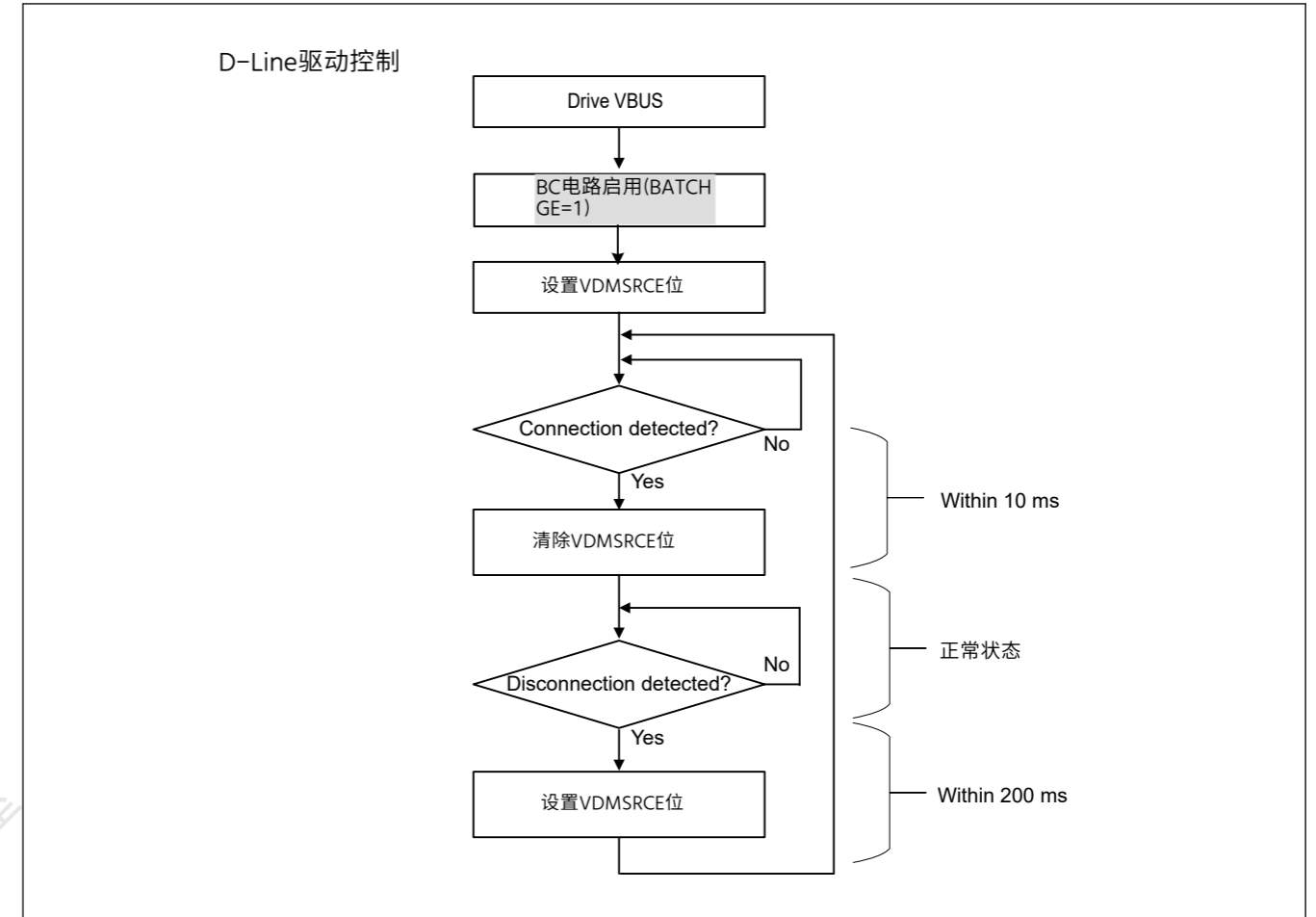
Figure 26.26 不使用便携设备检测功能时的处理流程 (步骤a.和b.)
