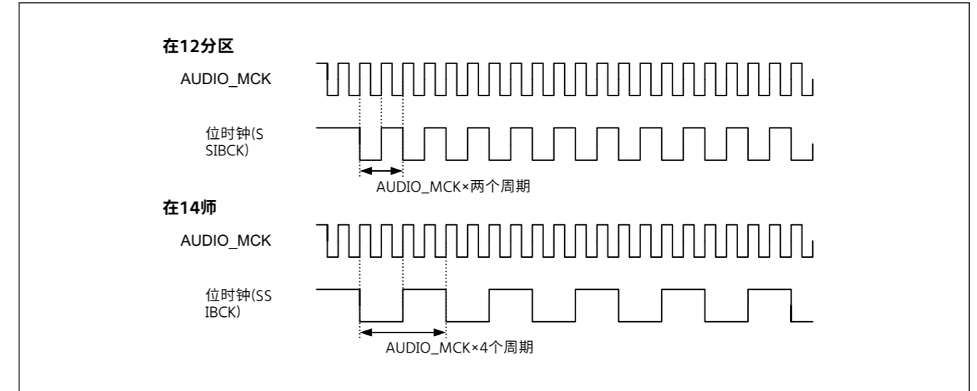
Figure 32.6 主模式通信中的采样频率
