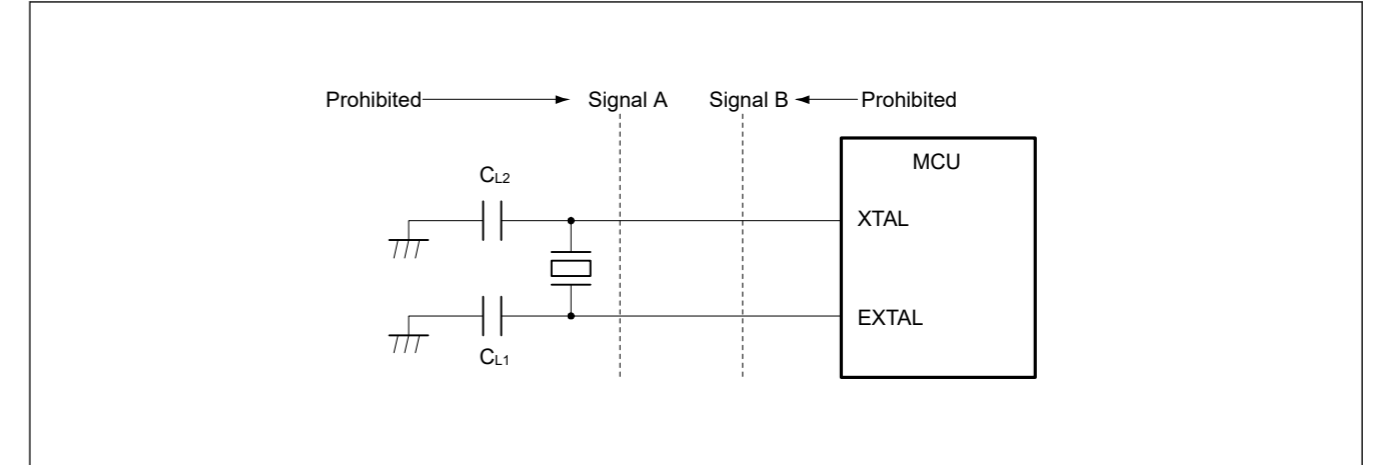
Figure 8.11 振荡电路板设计中的信号路由
