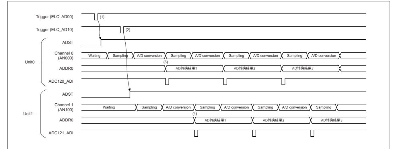
Figure 37.25 在交错操作中选择AN000和AN100时连续扫描模式下的示例操作
