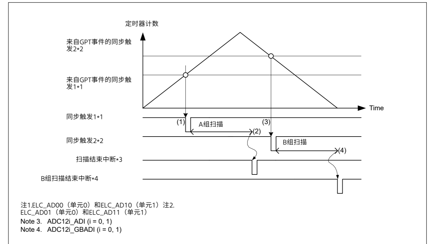
Figure 37.16 使用来自ELC的同步触发时组扫描模式下的基本操作示例
