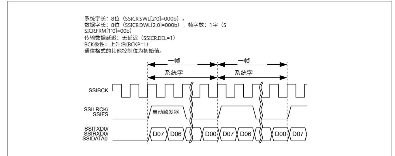
Figure 32.40 单声道格式的长帧 (无填充)
