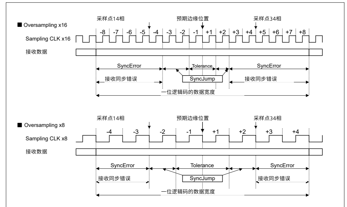
Figure 27.63 接收重定时范围的概念图
