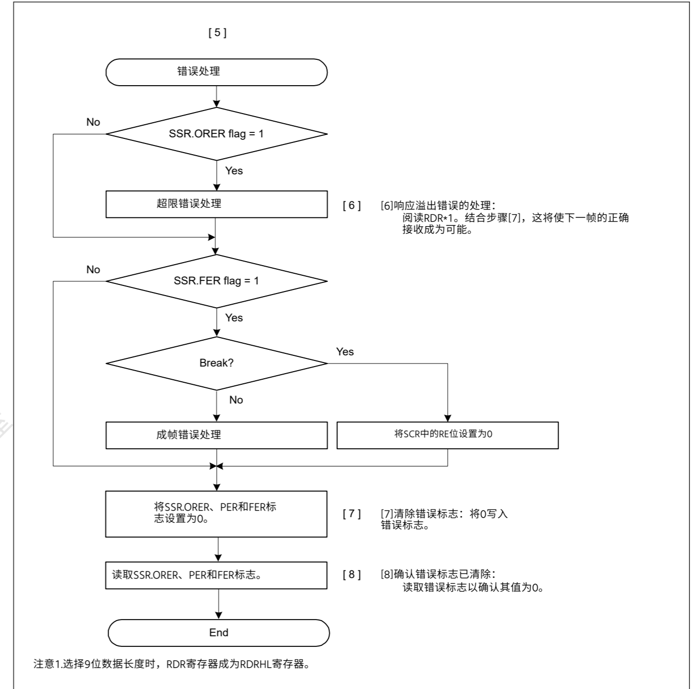
Figure 27.46 选择非FIFO的多处理器串行接收示例流程(2)
