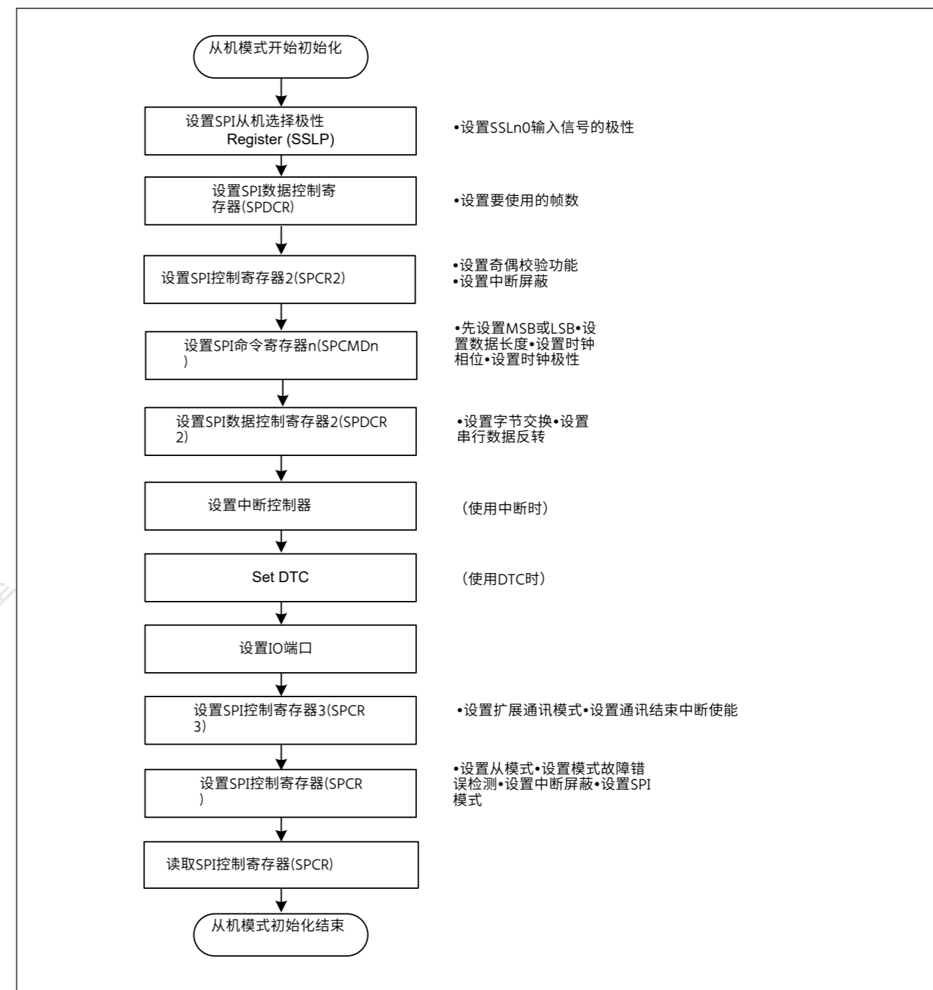
Figure 30.52 SPI操作的从模式初始化流程示例
