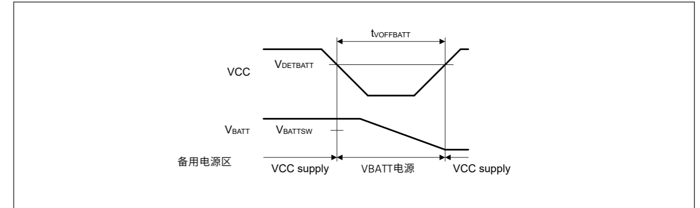
Figure 47.60 电池备份功能特点
