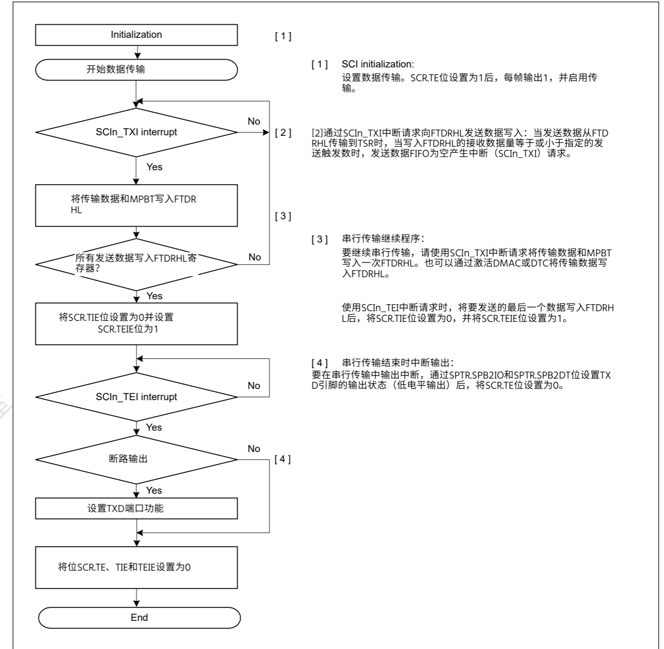
Figure 27.43 选择FIFO的多处理器模式下的串行传输示例流程
