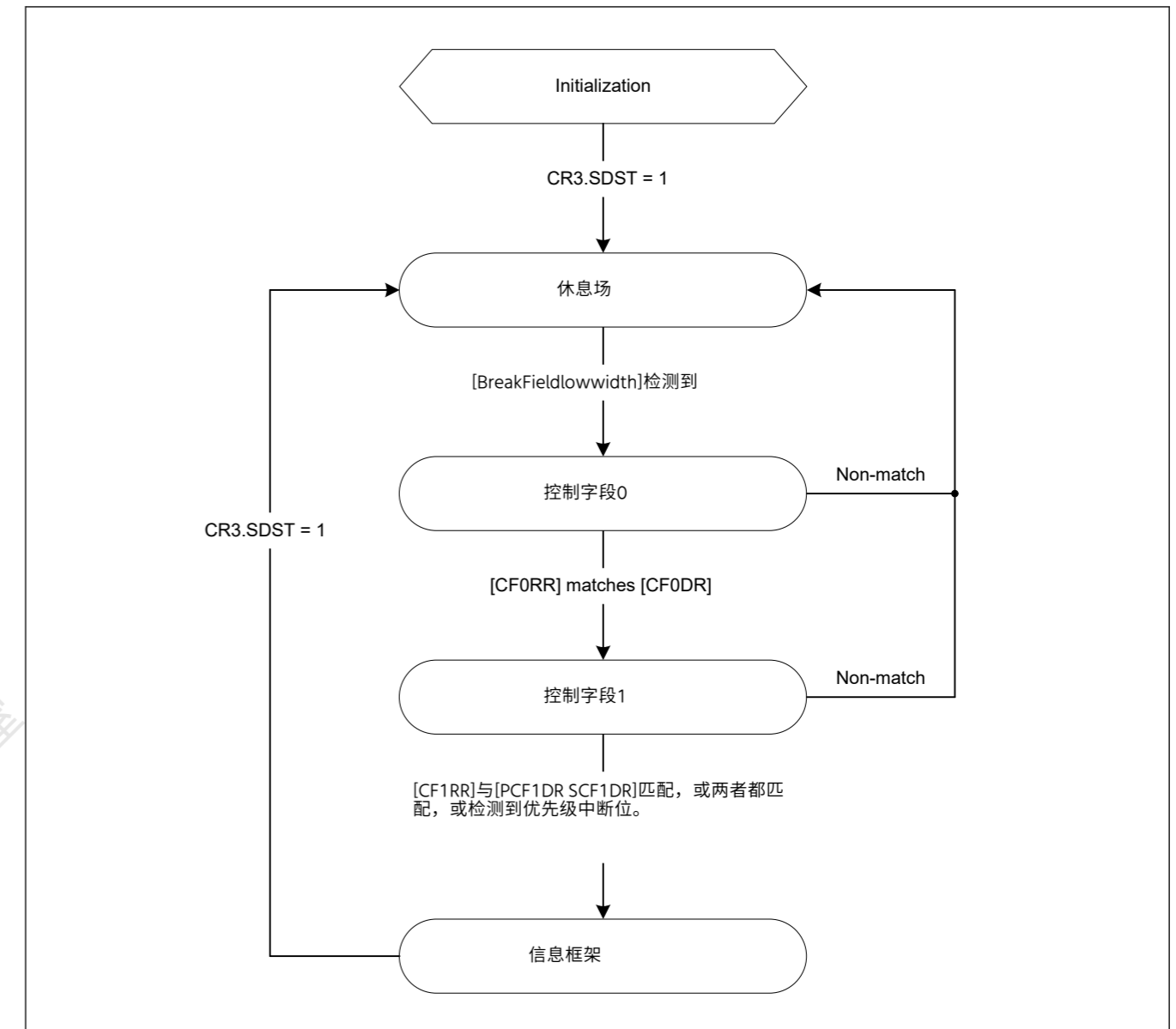
图27.109接收起始帧时的状态转换
