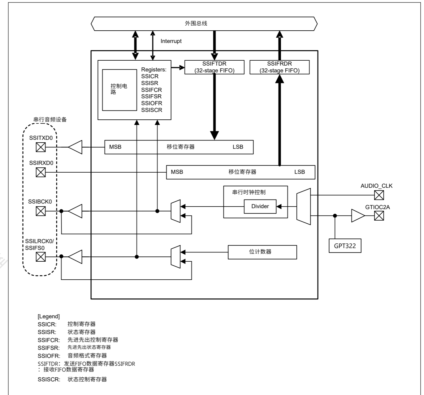
Figure 32.2 全双工通信的SSIE框图
