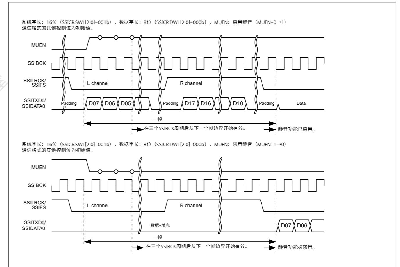
Figure 32.5 设置静音功能传输数据
