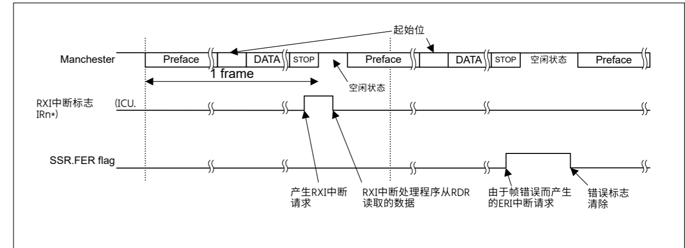
Figure 27.60 曼彻斯特模式下串行数据接收操作示例（附前言）
