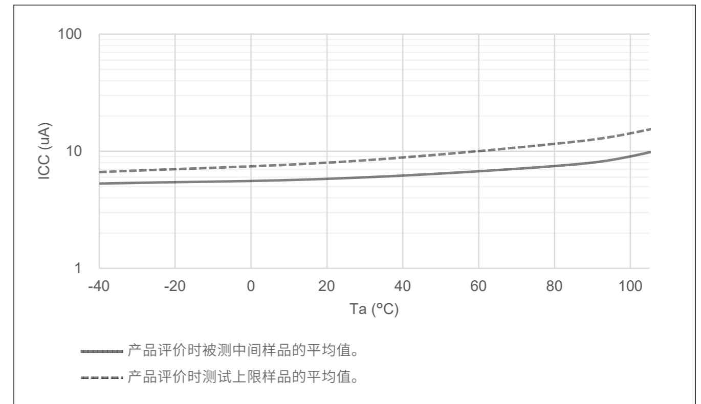
Figure 47.5 深度软件待机模式下的温度依赖性，未向SRAM供电或USB恢复检测单元，上电复位电路低功耗功能启用（参考数据）
