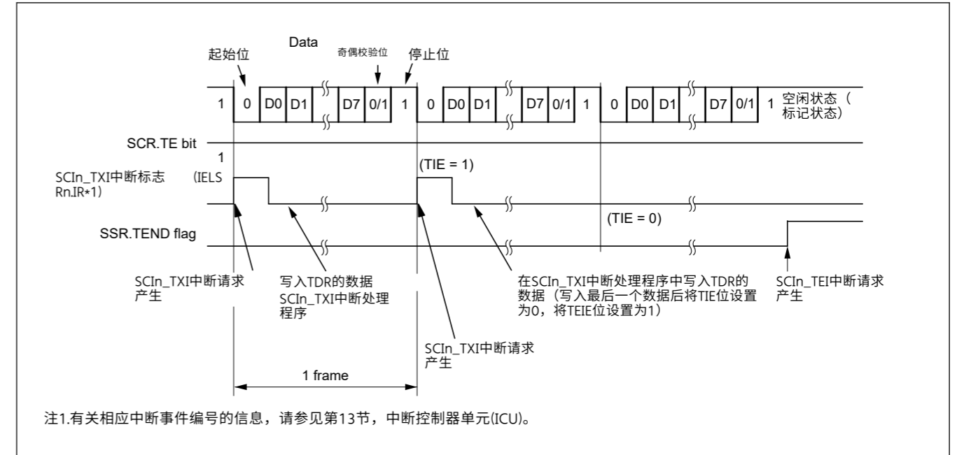
Figure 27.13 异步模式下串行传输的示例操作(3)使用8位数据、奇偶校验位、一个停止位、未使用CTS功能,以及从传输中间到传输完成
