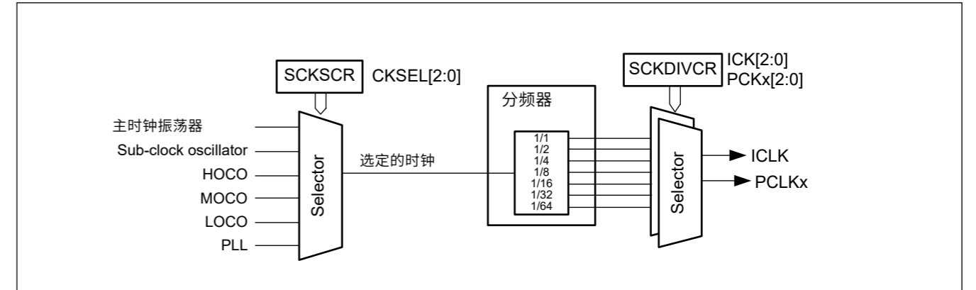
Figure 8.9 时钟源选择器框图
