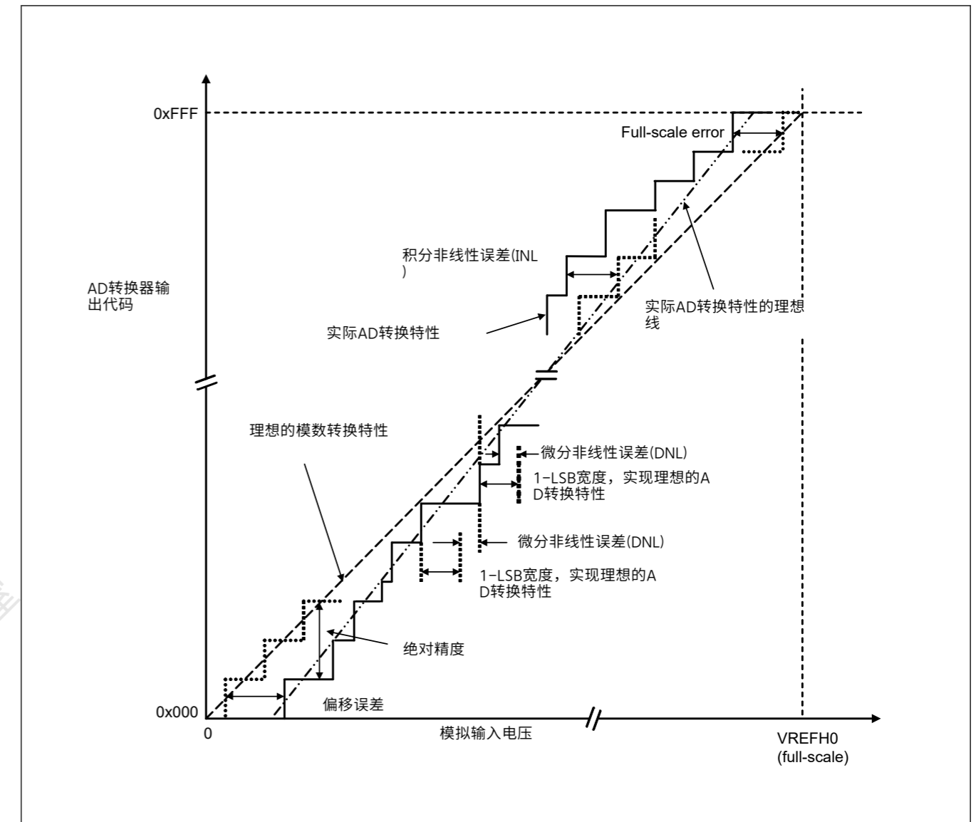
Figure 47.54 ADC12特征项说明
