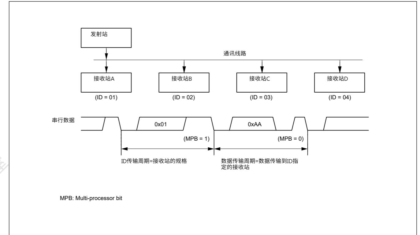
Figure 27.40 使用多处理器格式的通信示例，将数据0xAA传输到接收站A
