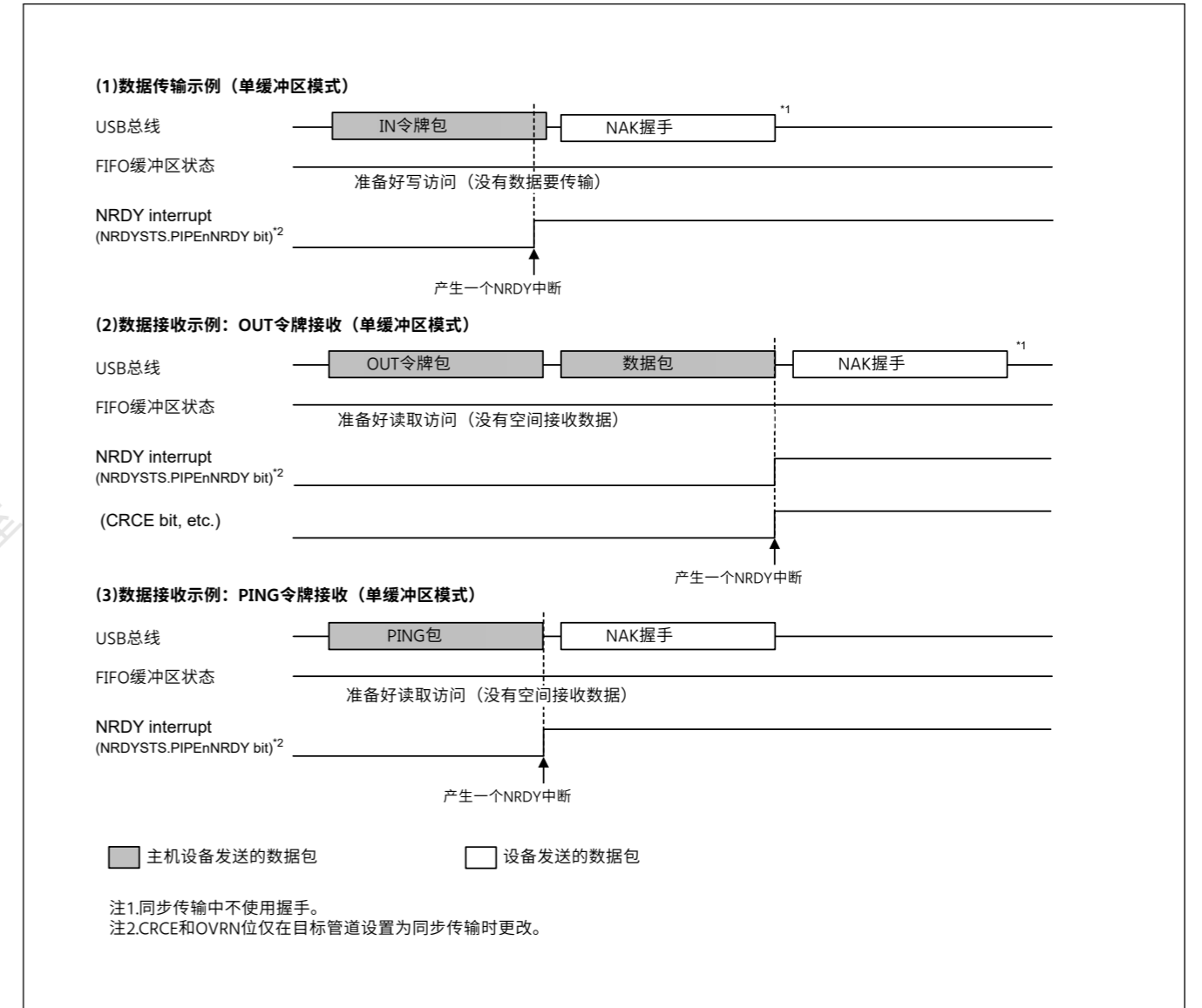
Figure 26.13 设备控制器模式下NRDY中断产生的时序
