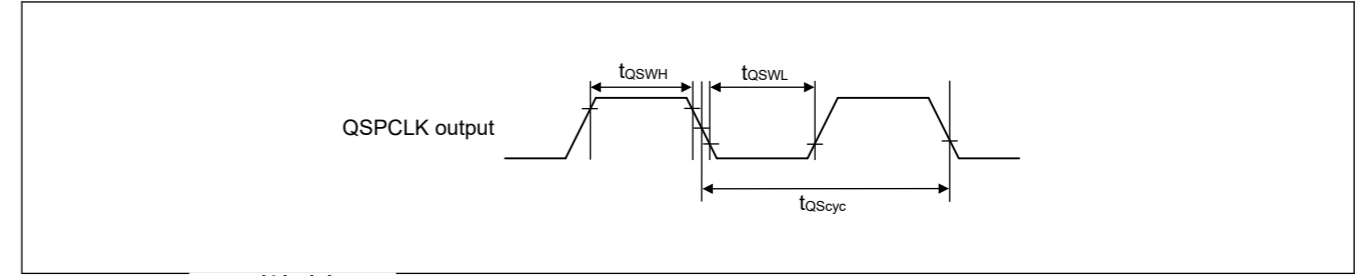
Figure 47.41 QSPI时钟时序
