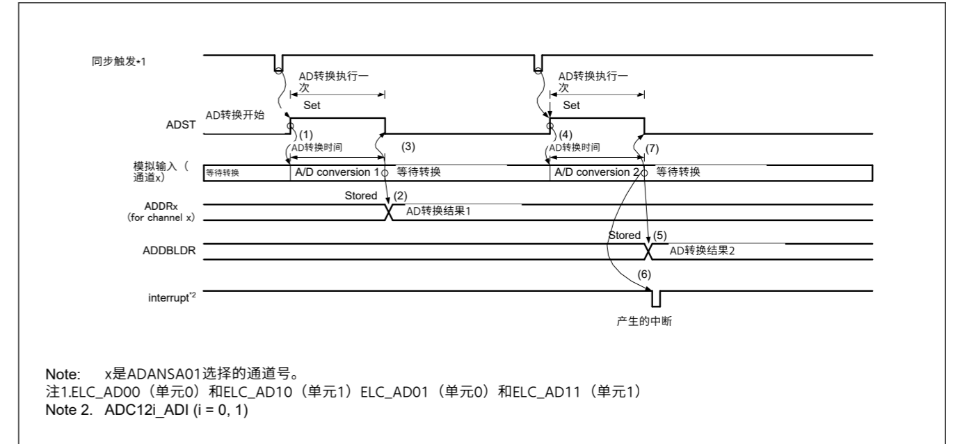
Figure 37.11 选择双触发模式并复制模拟输入 (通道x) 时的单扫描模式操作示例
