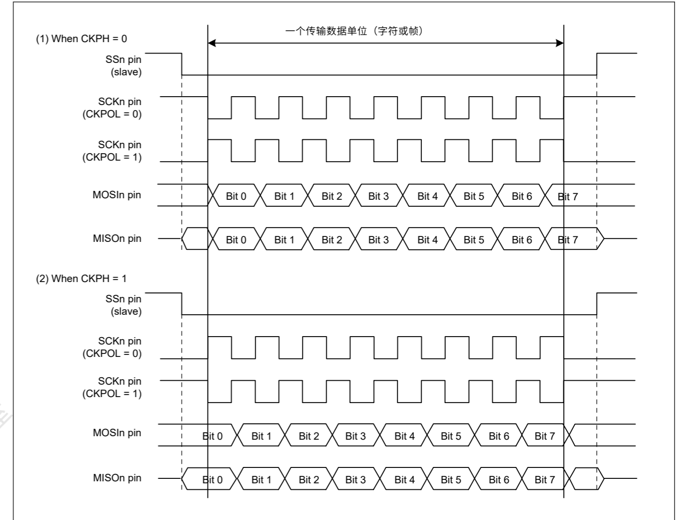
Figure 27.99 简单SPI模式下时钟信号与发送或接收数据的关系
