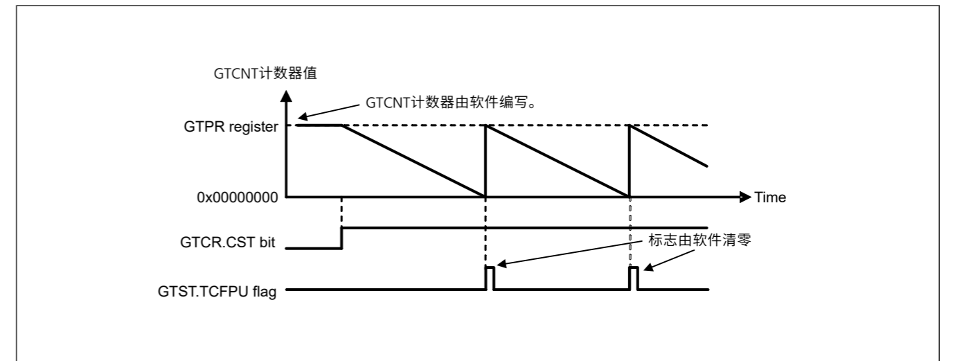
Figure 21.4 计数时钟递减计数中的周期计数操作示例
