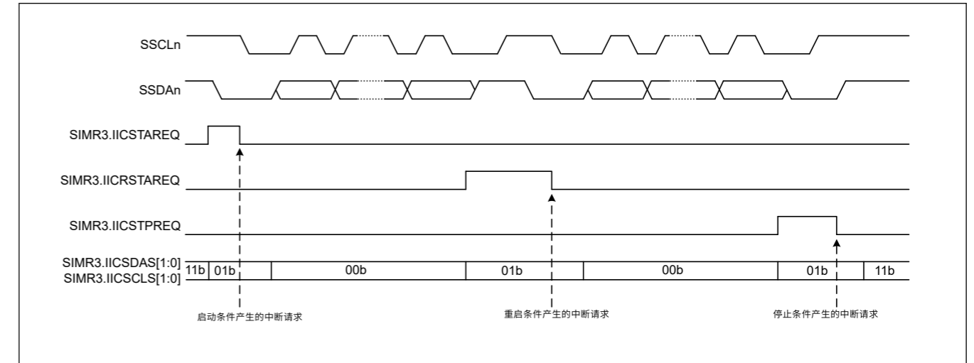
Figure 27.90 生成启动、重启和停止条件时的操作时序
