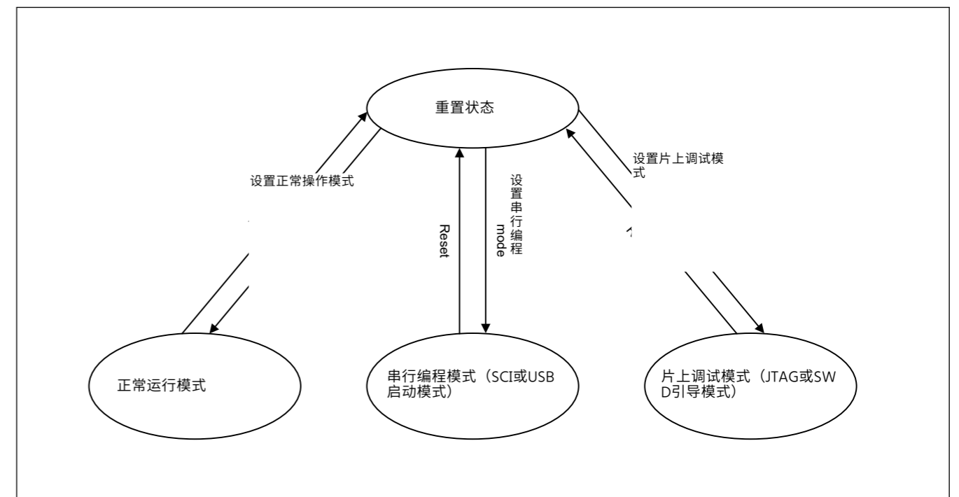
Figure 44.5 与闪存相关的模式转换
