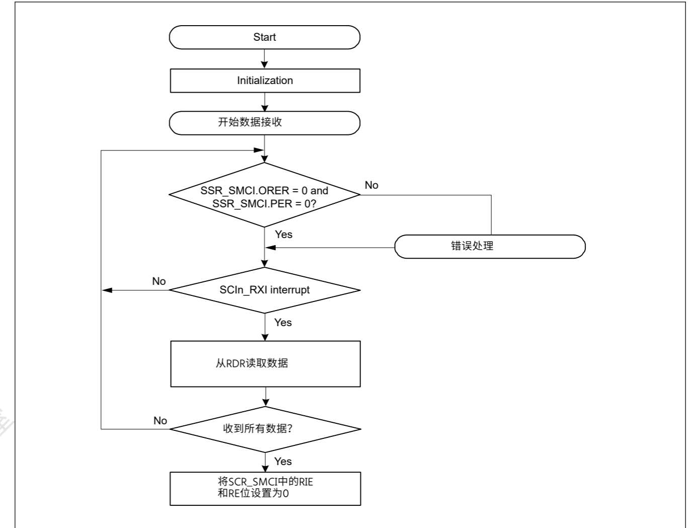
Figure 27.86 智能卡接口接收示例流程
