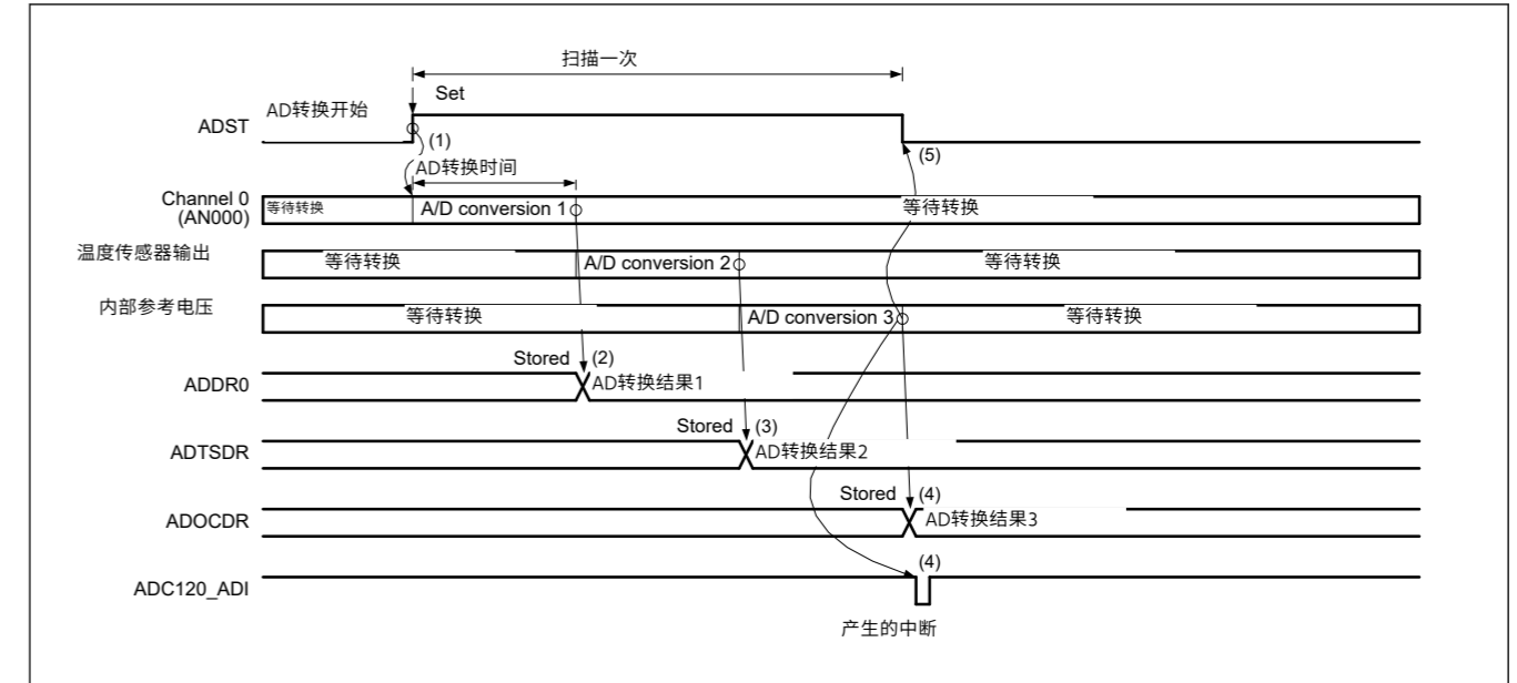
Figure 37.10 选择AN000和温度传感器输出或内部参考电压时单次扫描模式下的基本操作示例
