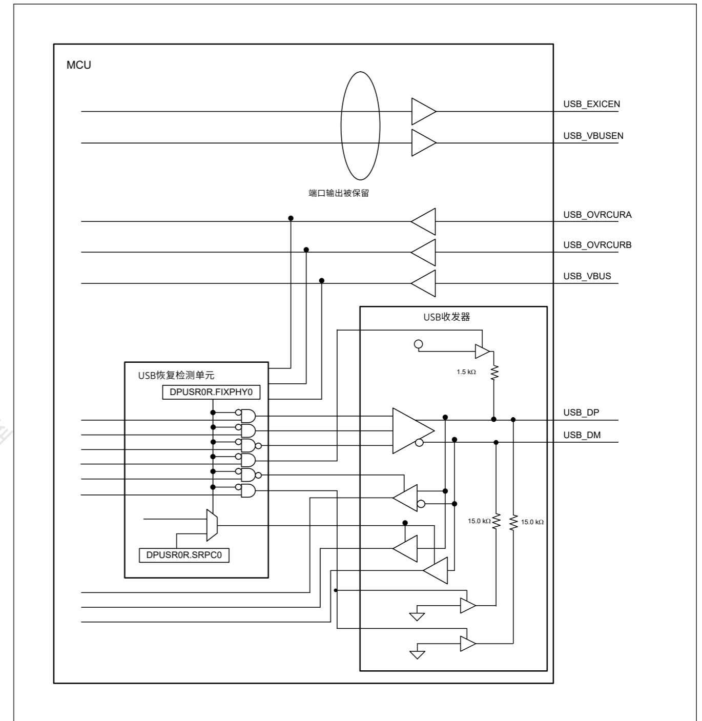
Figure 26.7 USB恢复检测单元与USBIO管脚的连接
