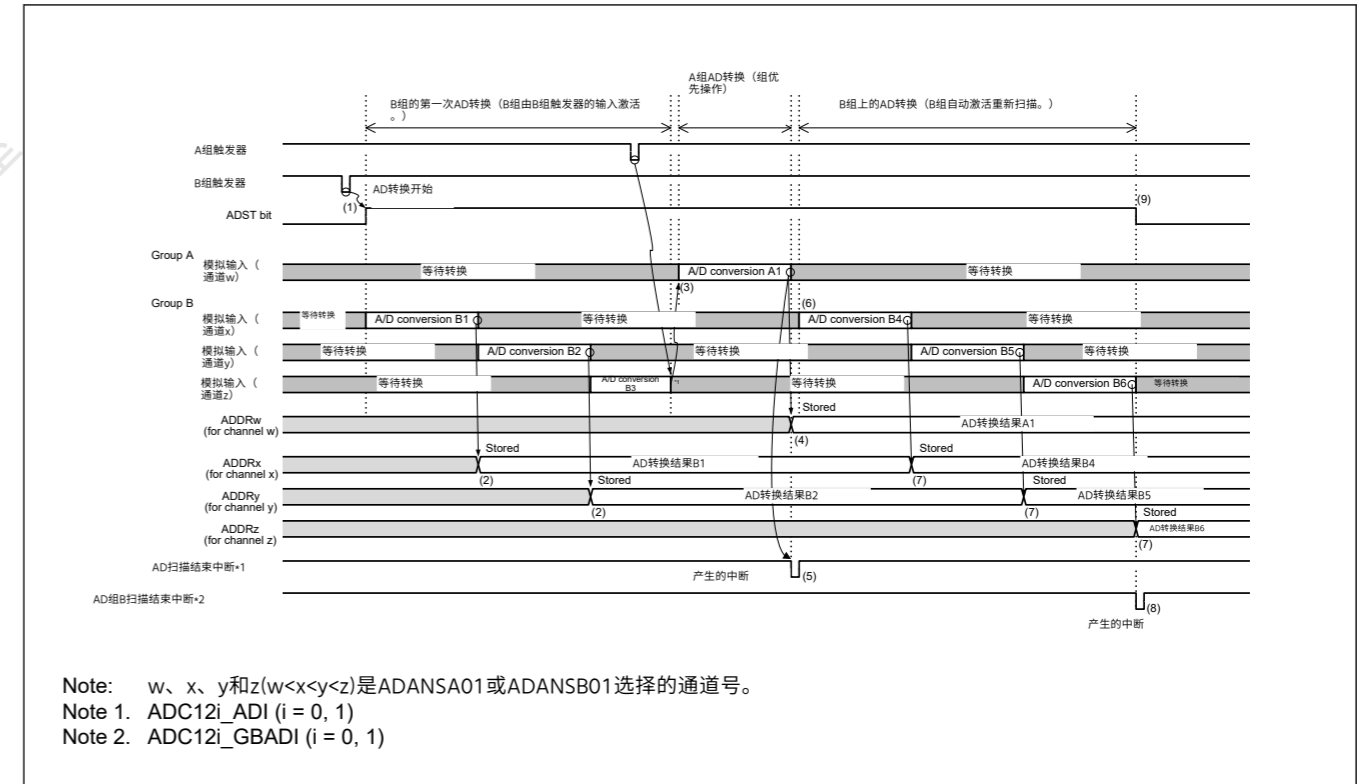
Figure 37.19 组优先操作1-1示例：启用重新扫描时，在B组扫描期间A组触发输入（当ADGSPCR.GBRSCN=1、ADGSPCR.GBRP=0和ADGSPCR.LGRRS=0时）
