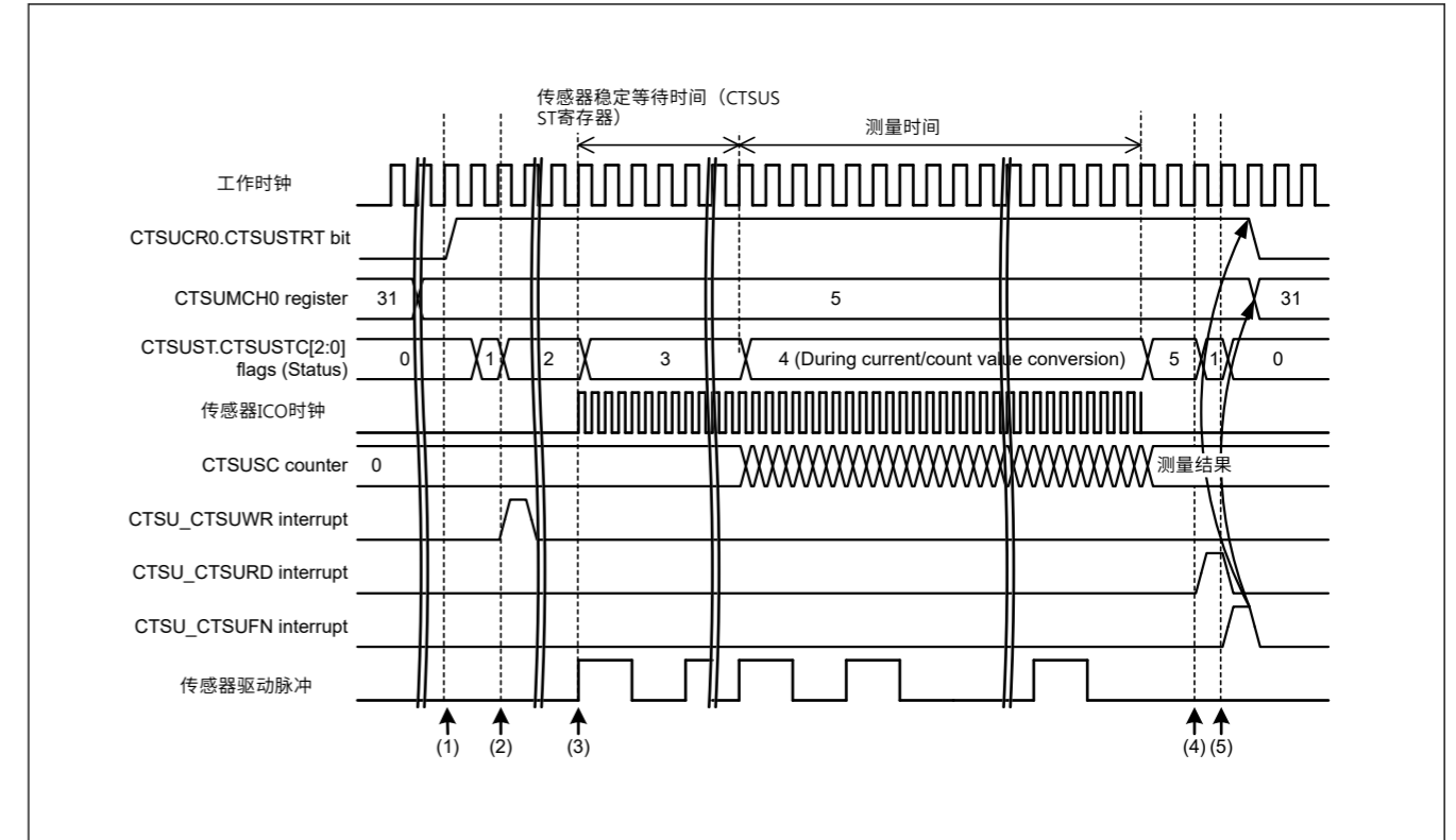
Figure 40.13 测量开始条件为软件触发时的自电容单次扫描模式时序
