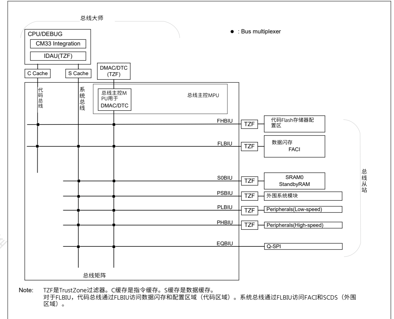
Figure 14.1 巴士连接
