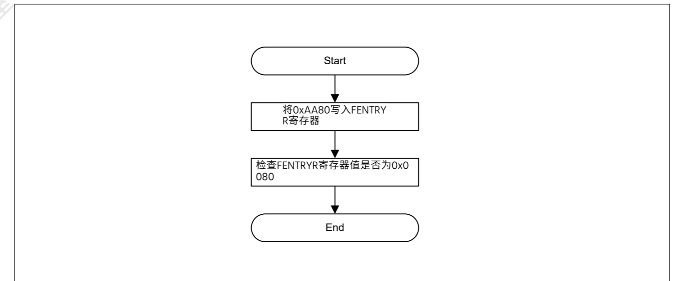
Figure 44.10 转换到数据闪存PE模式的步骤
