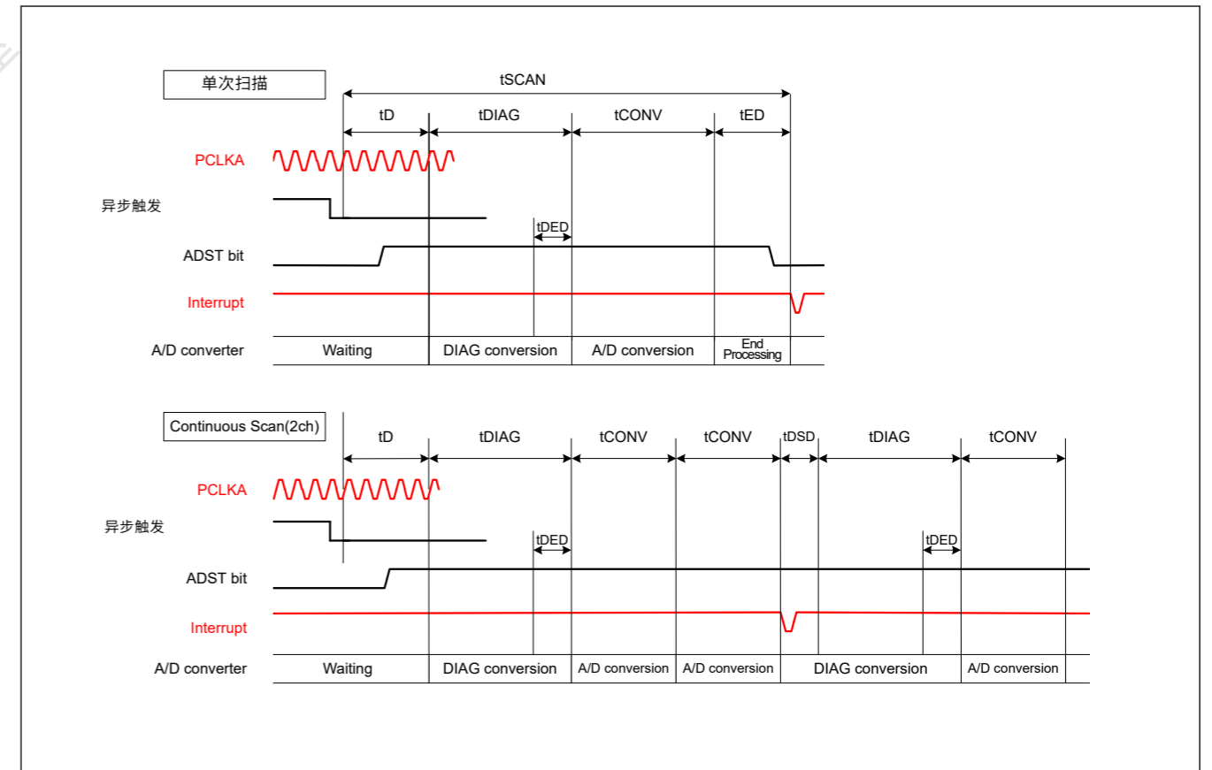
Figure 37.32 由异步触发输入(ADTRG0)激活时的扫描转换时序
