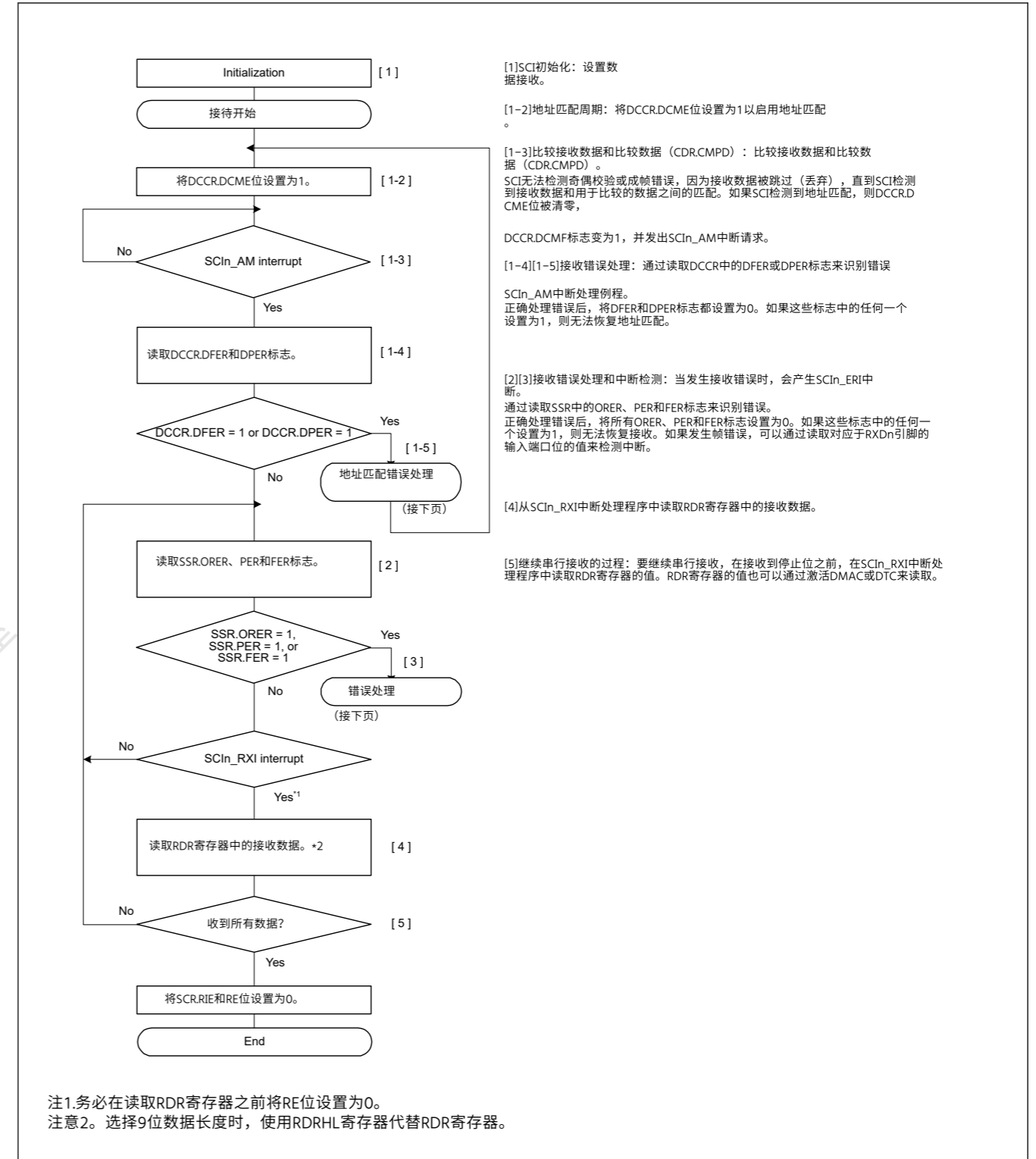
Figure 27.22 异步模式下串行接收的示例流程图 (未选择FIFO和地址匹配启用) (1)
