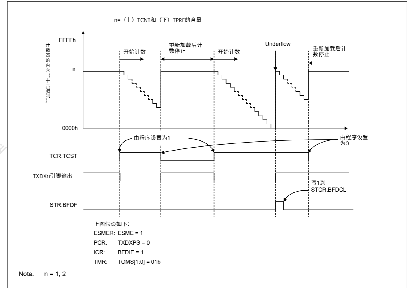
图27.115中断场低宽度输出模式下的操作示例
