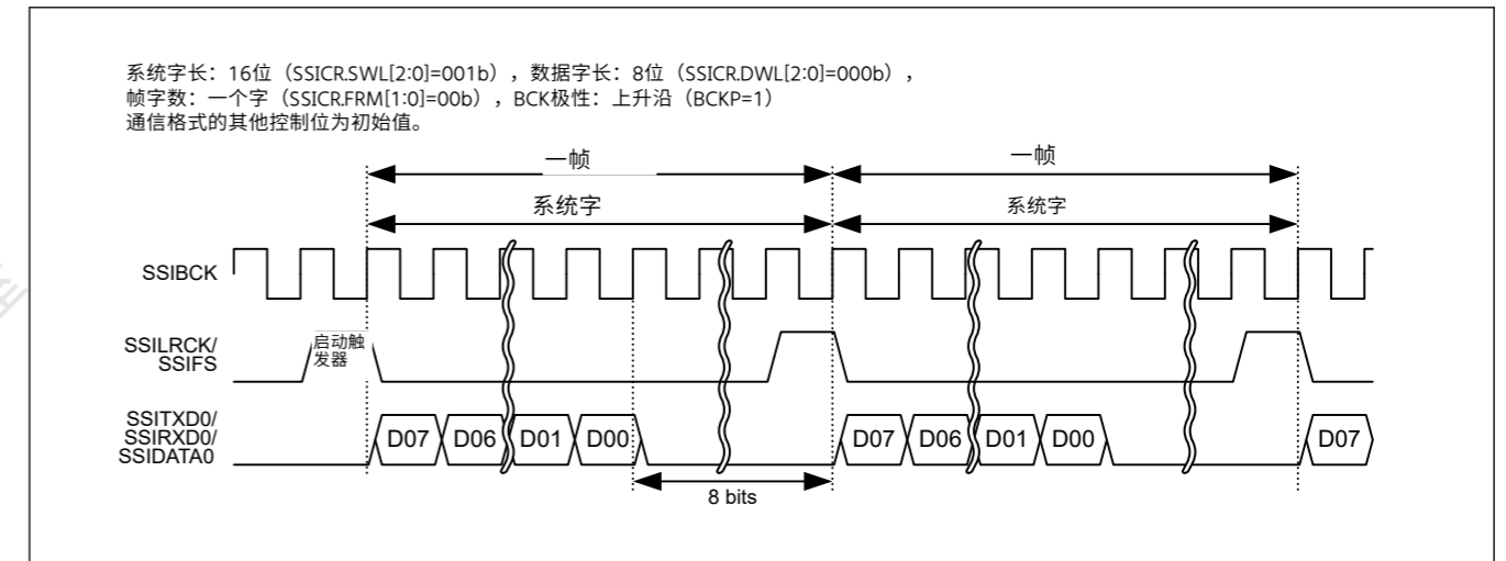
Figure 32.39 单声道格式的短帧 (带填充: 系统字长>数据字长)
