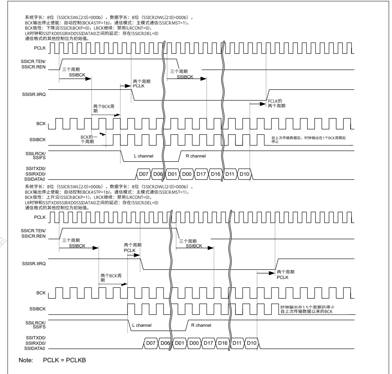
Figure 32.35 BCKASTP位的示例操作 (BCKASTP=1的通信操作)
