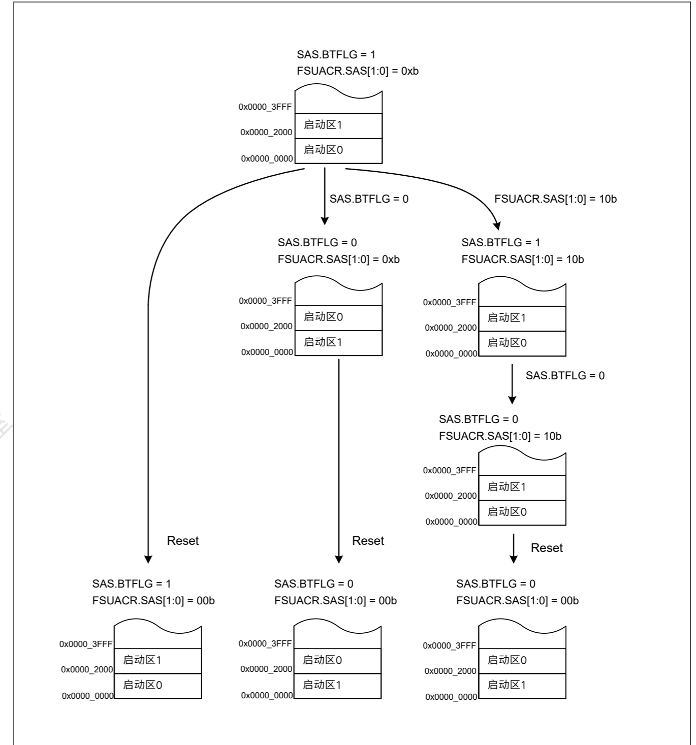
Figure 44.26 启动程序保护设置的转换示例1
