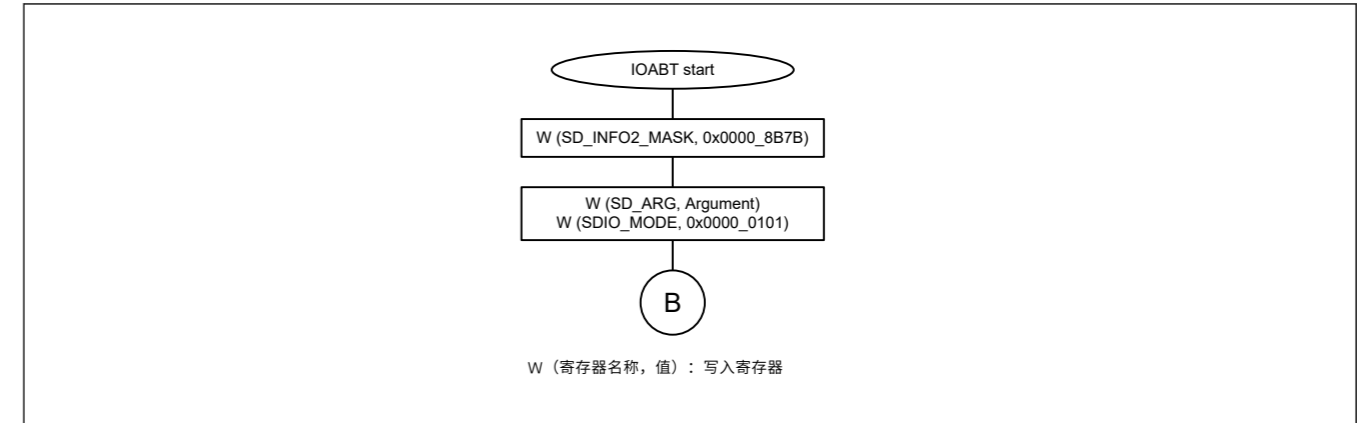
Figure 33.18 在CMD53多块读取期间发出CMD52 (SDIO中止) 时的流程
