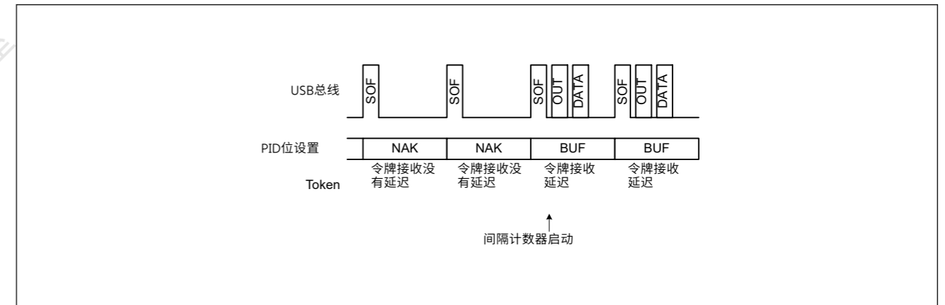
Figure 26.19 IITV[2:0]=0时帧与预期令牌接收之间的关系
