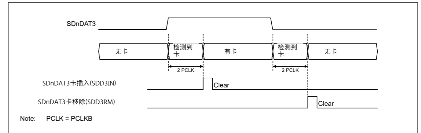
Figure 33.8 使用SDnDAT3检测SD卡
