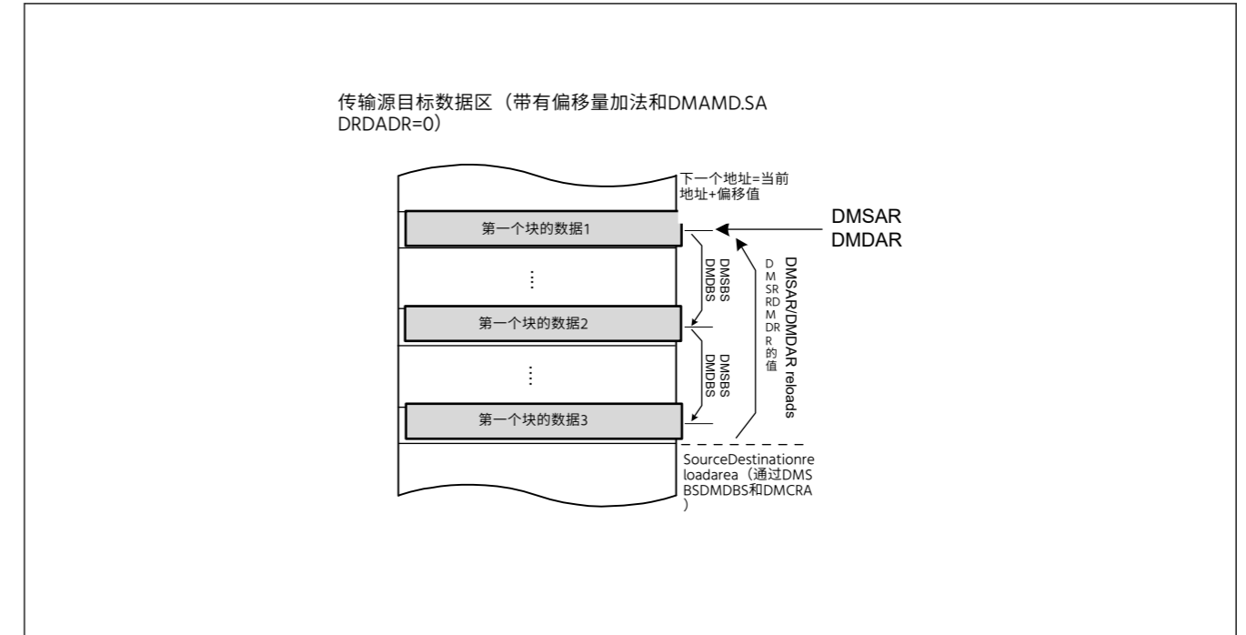
Figure 16.16 使用DMAMD.SADR和DMAMD.DADR=0进行偏移加法中的地址更新
