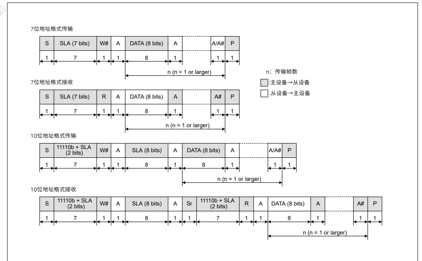
Figure 27.88 I 2 C总线格式
