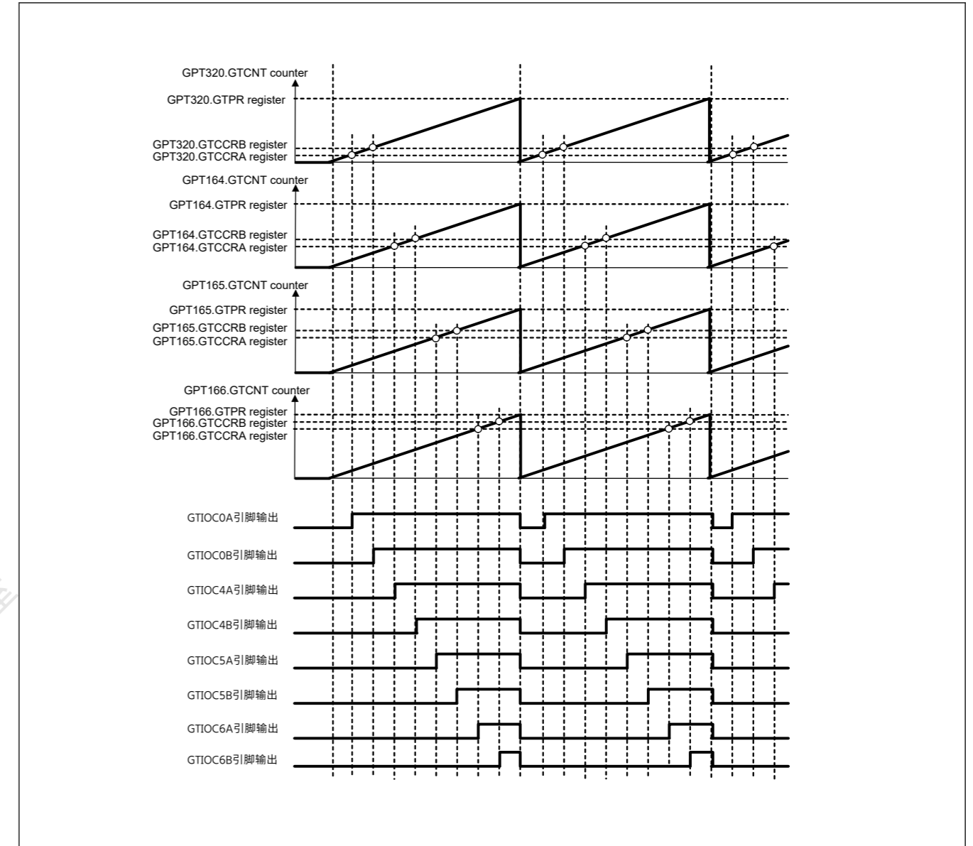
Figure 21.39 同步PWM输出示例
