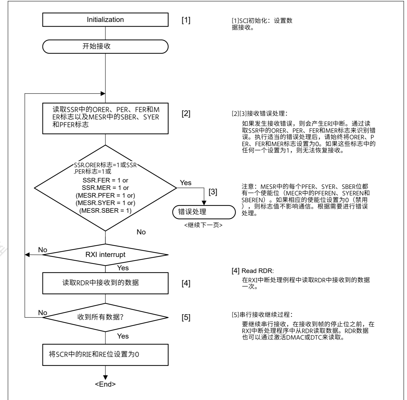
Figure 27.61 曼彻斯特模式下的串行数据接收流程图示例 (正常接收)
