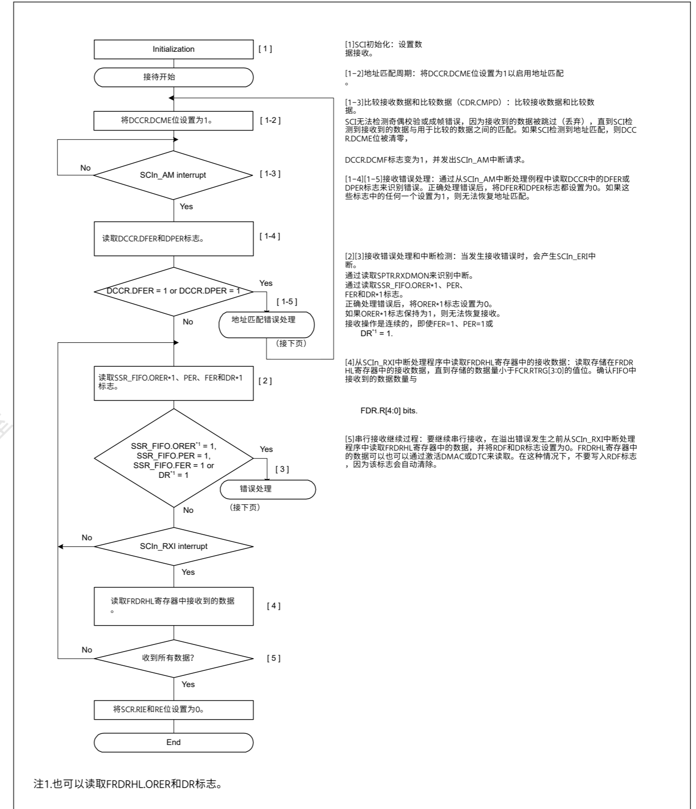
Figure 27.28 异步模式下串行接收的示例流程图（FIFO选择和地址 Matching Enabled）(1)
