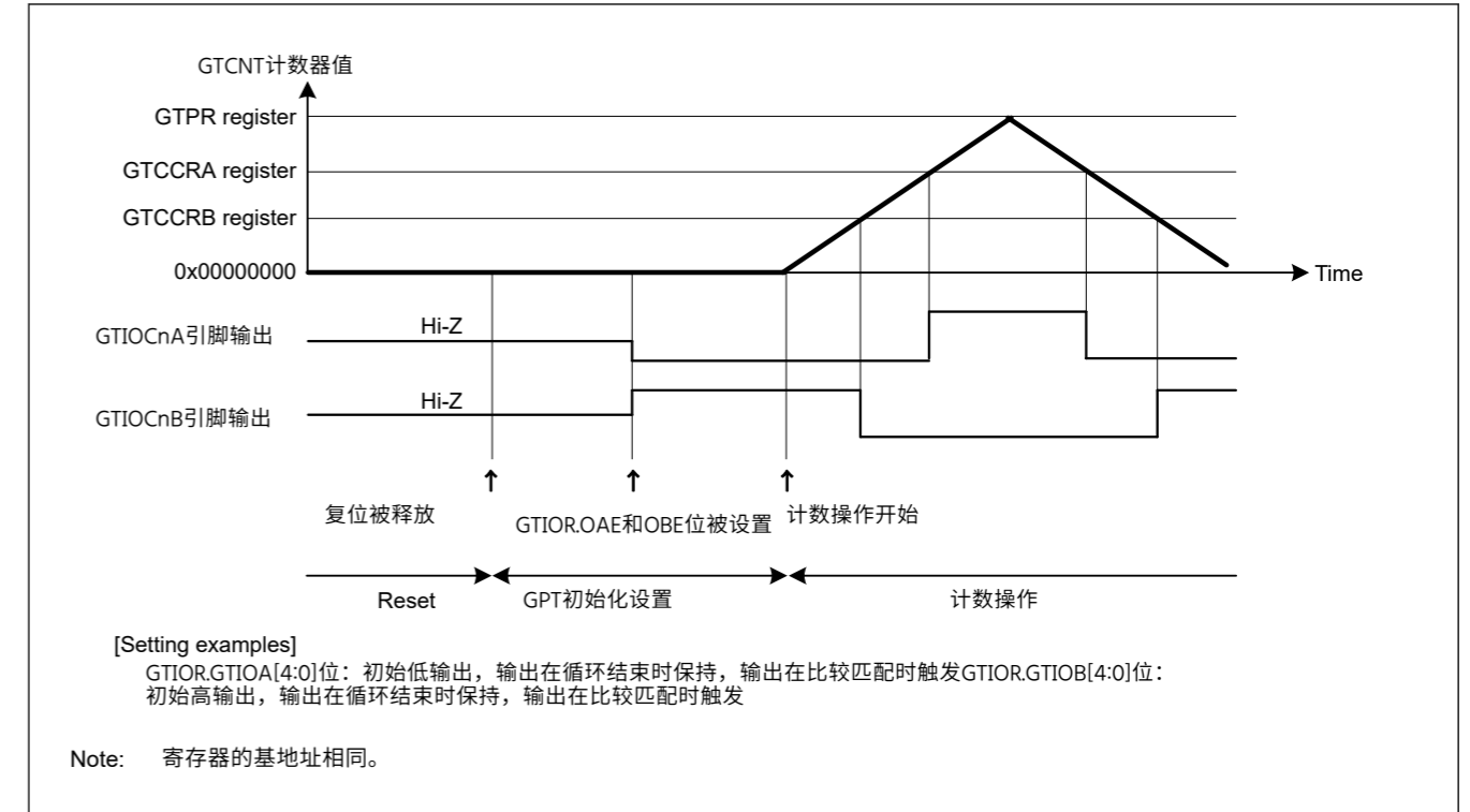
Figure 21.67 复位后的引脚设置示例
