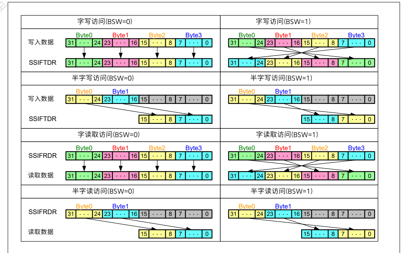
Figure 32.24 字节交换操作示例
