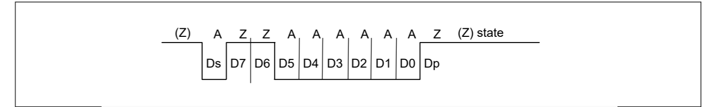
Figure 27.80 SCMR=1中的SDIR、SCMR=1中的SINV和SMR_SMCI=1中的PM的逆约定
