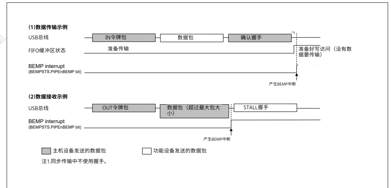
Figure 26.14 设备控制器模式下BEMP中断产生的时序
