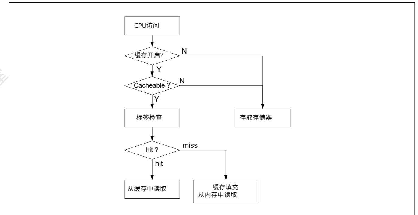
Figure 14.7 从CPU到C-cache的访问流程
