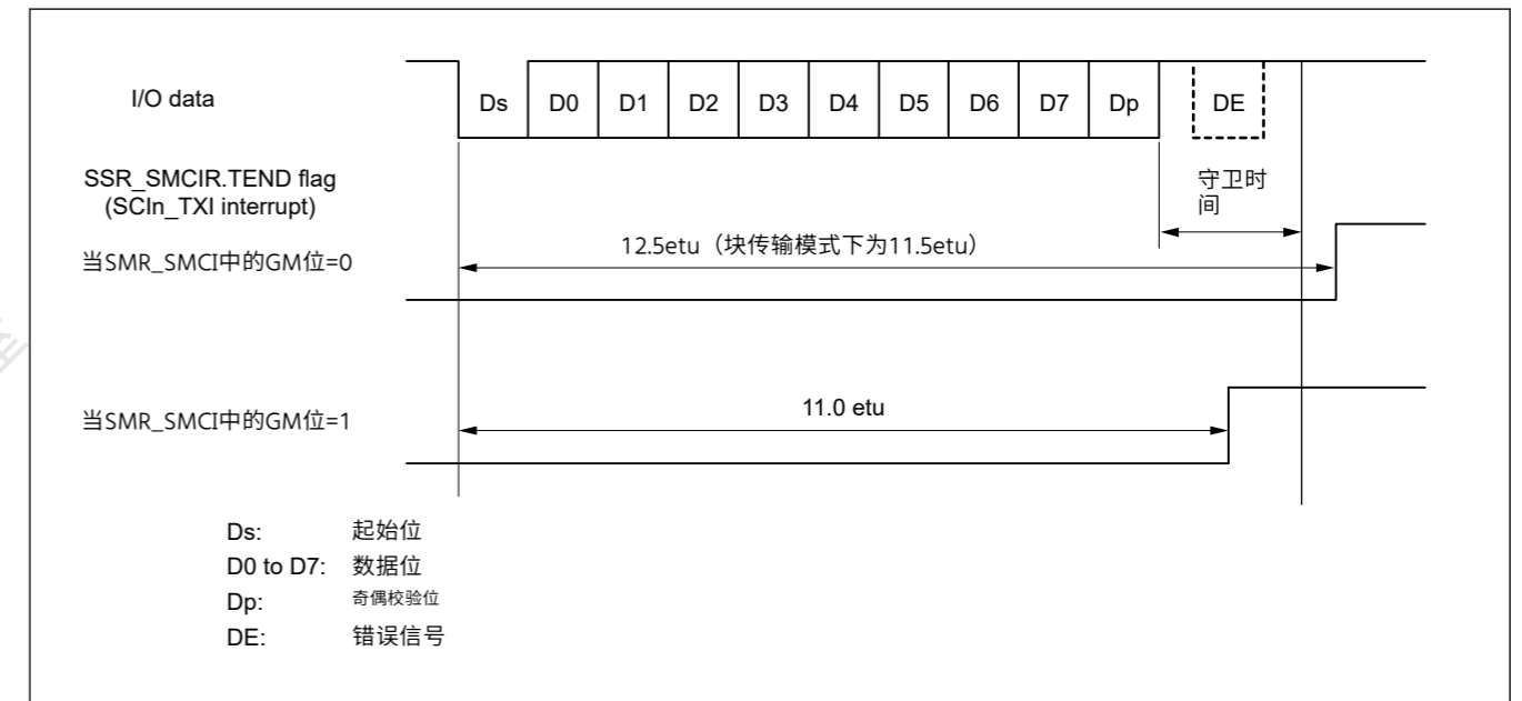
Figure 27.83 发送期间的SSR.TEND标志生成时序
