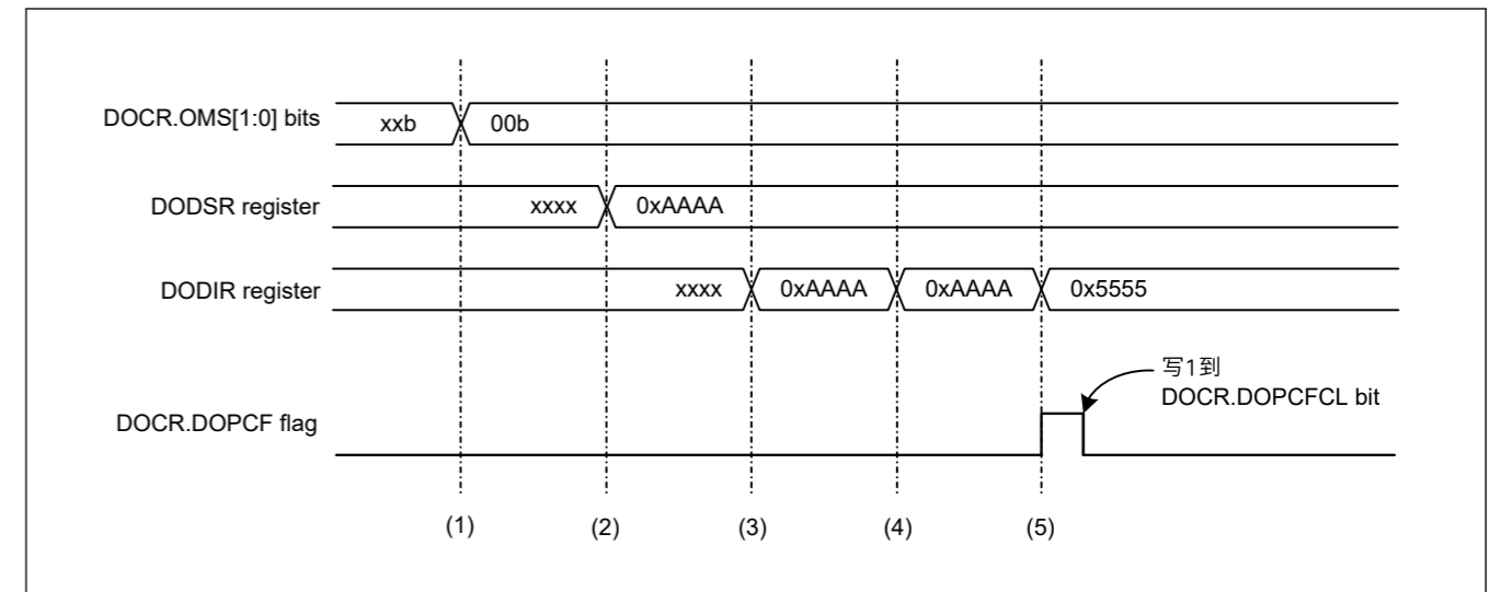
Figure 41.2 数据比较模式的操作示例
