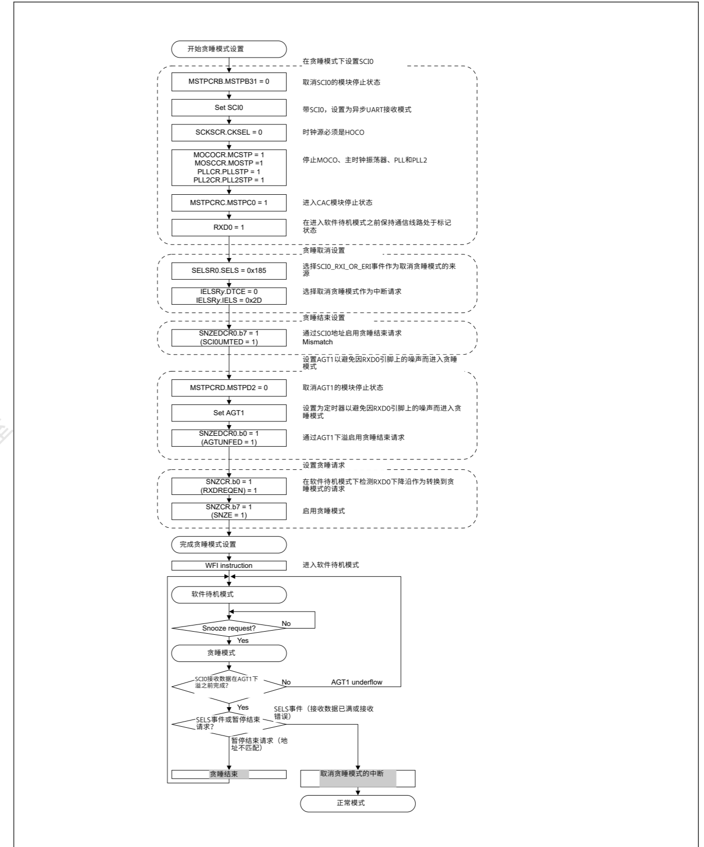
Figure 10.7 在Snooze模式进入使用SCI0的设置示例
