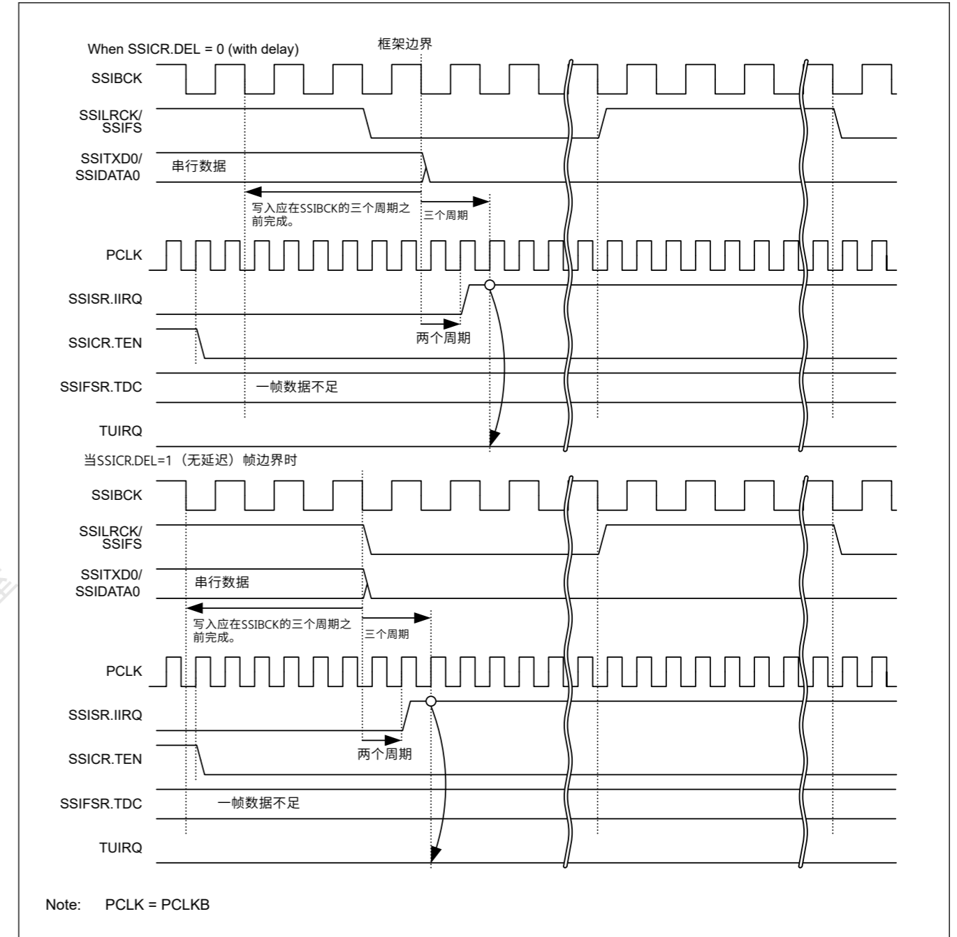
Figure 32.21 TUIRQ设置时间 (通信停止时)
