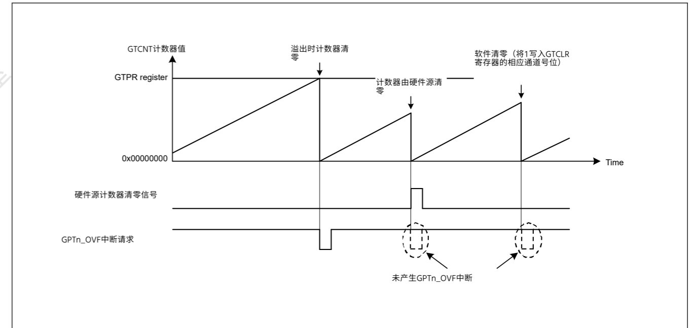
Figure 21.35 硬件源计数器清零与GPTn_OVF(n=0to7)中断的关系
