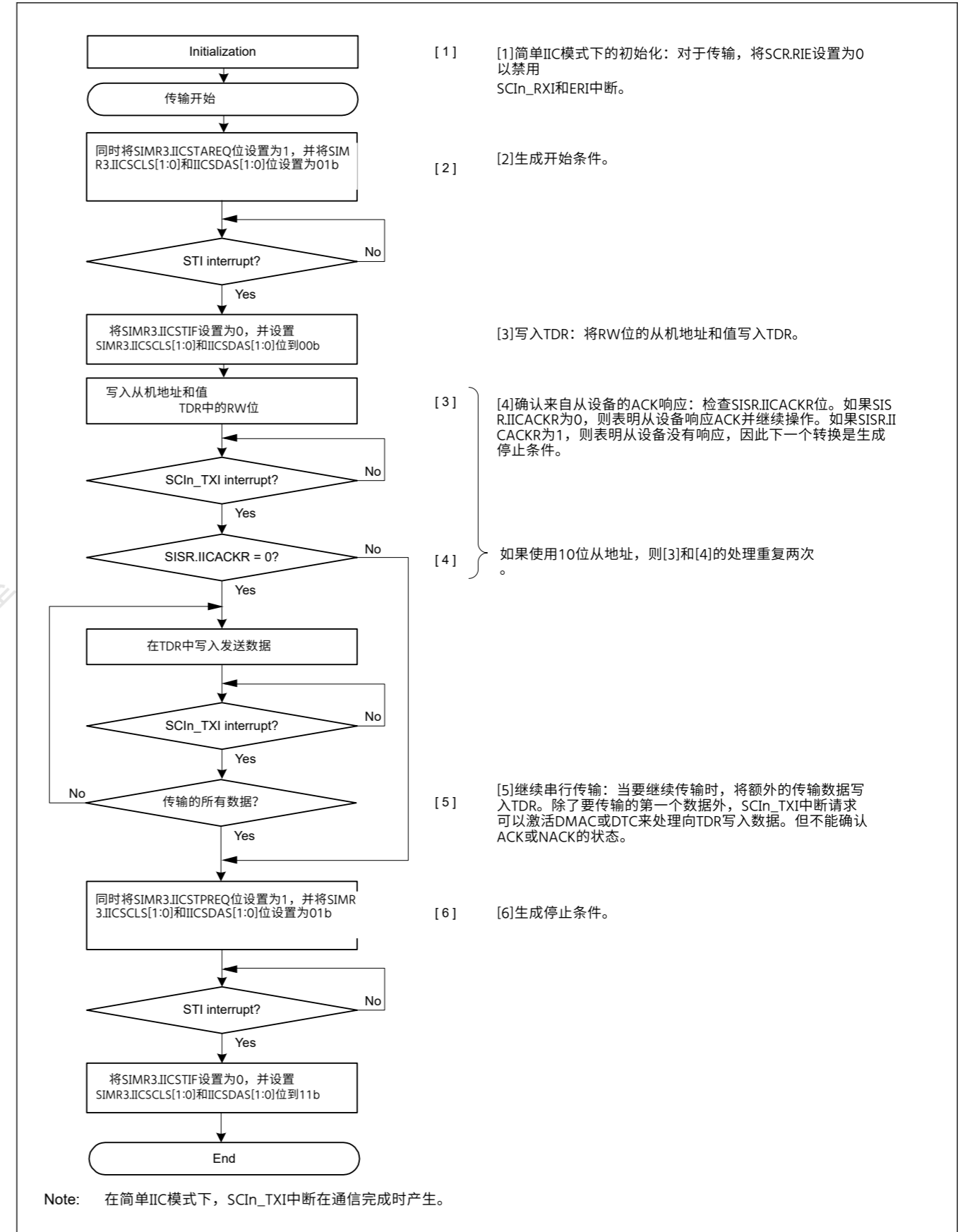
Figure 27.95 带有发送中断和接收中断的简单IIC模式下的主机发送示例流程
