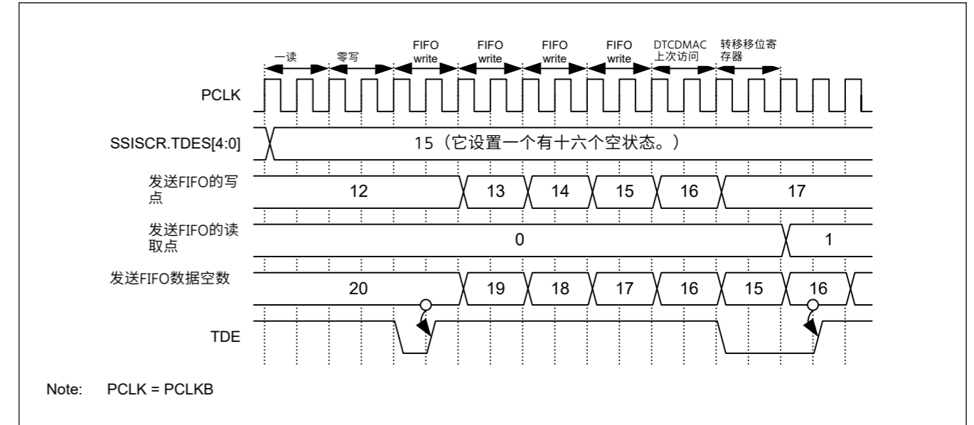
Figure 32.29 设置和清除TDE的时序图
