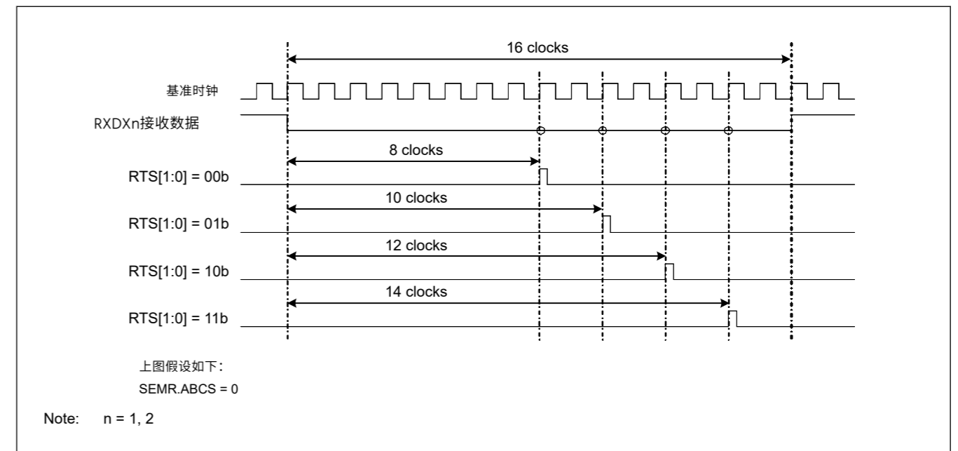
图27.114对通过RXDXn接收的数据进行采样的时序
