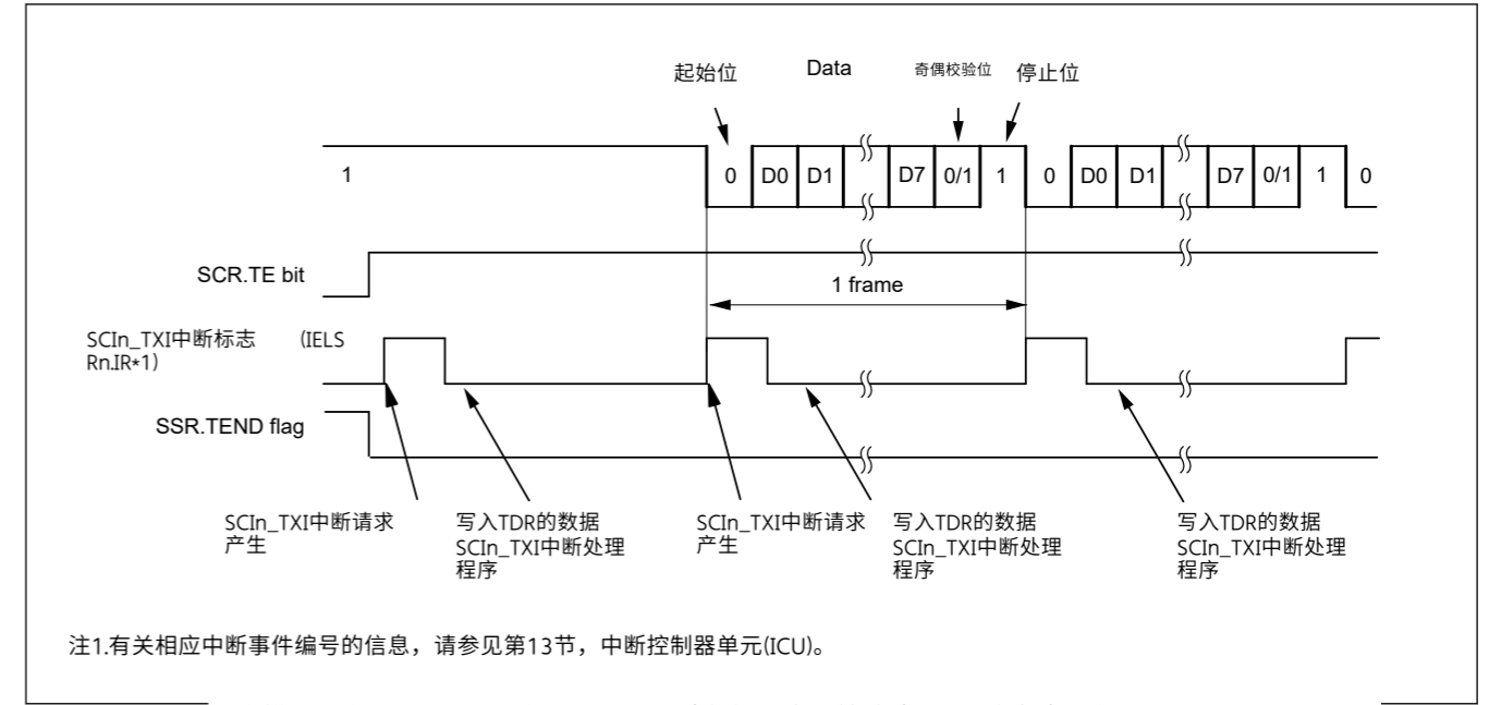
Figure 27.11 异步模式下串行传输的示例操作(1)使用8位数据、奇偶校验位、1个停止位、未使用CTS功能以及传输开始时
