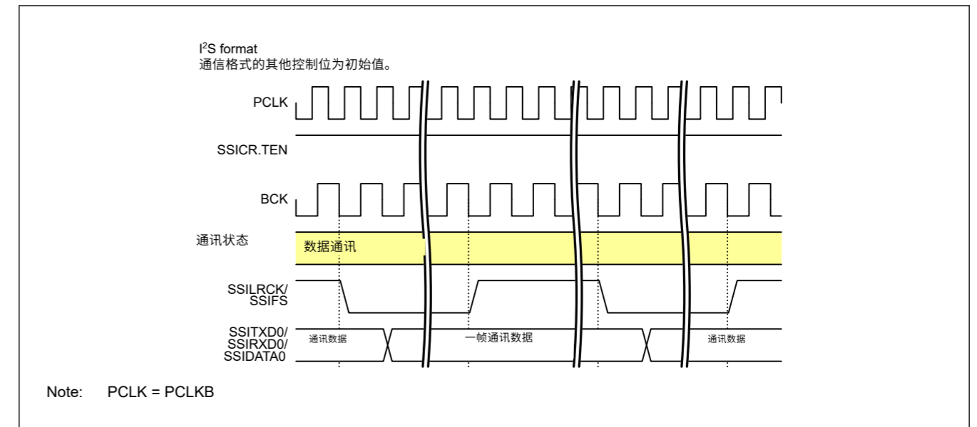
Figure 32.47 继续数据通信
