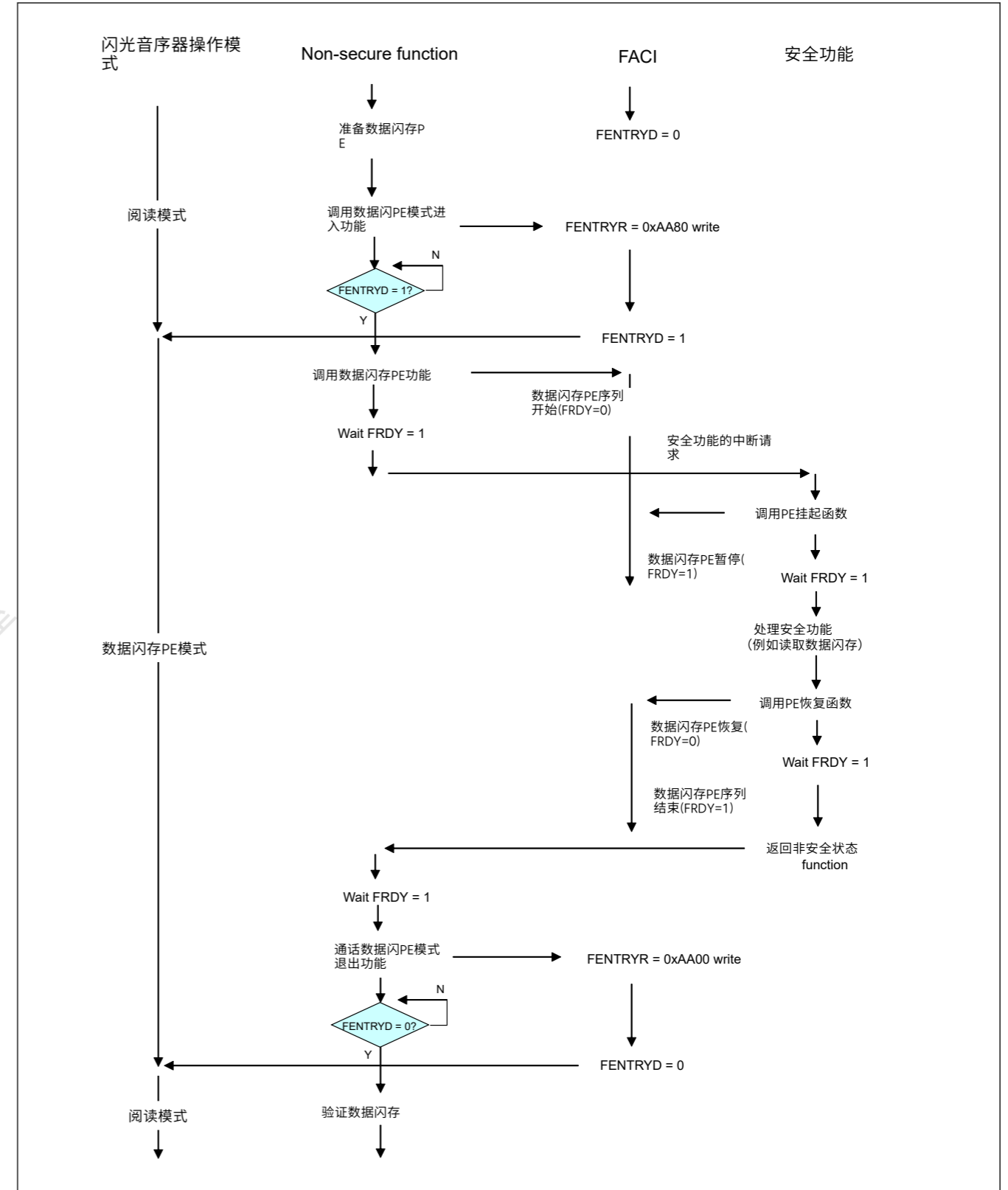
Figure 44.37 数据闪存PE安全功能暂停示例 (检查FRDY位以检测PE结束)
