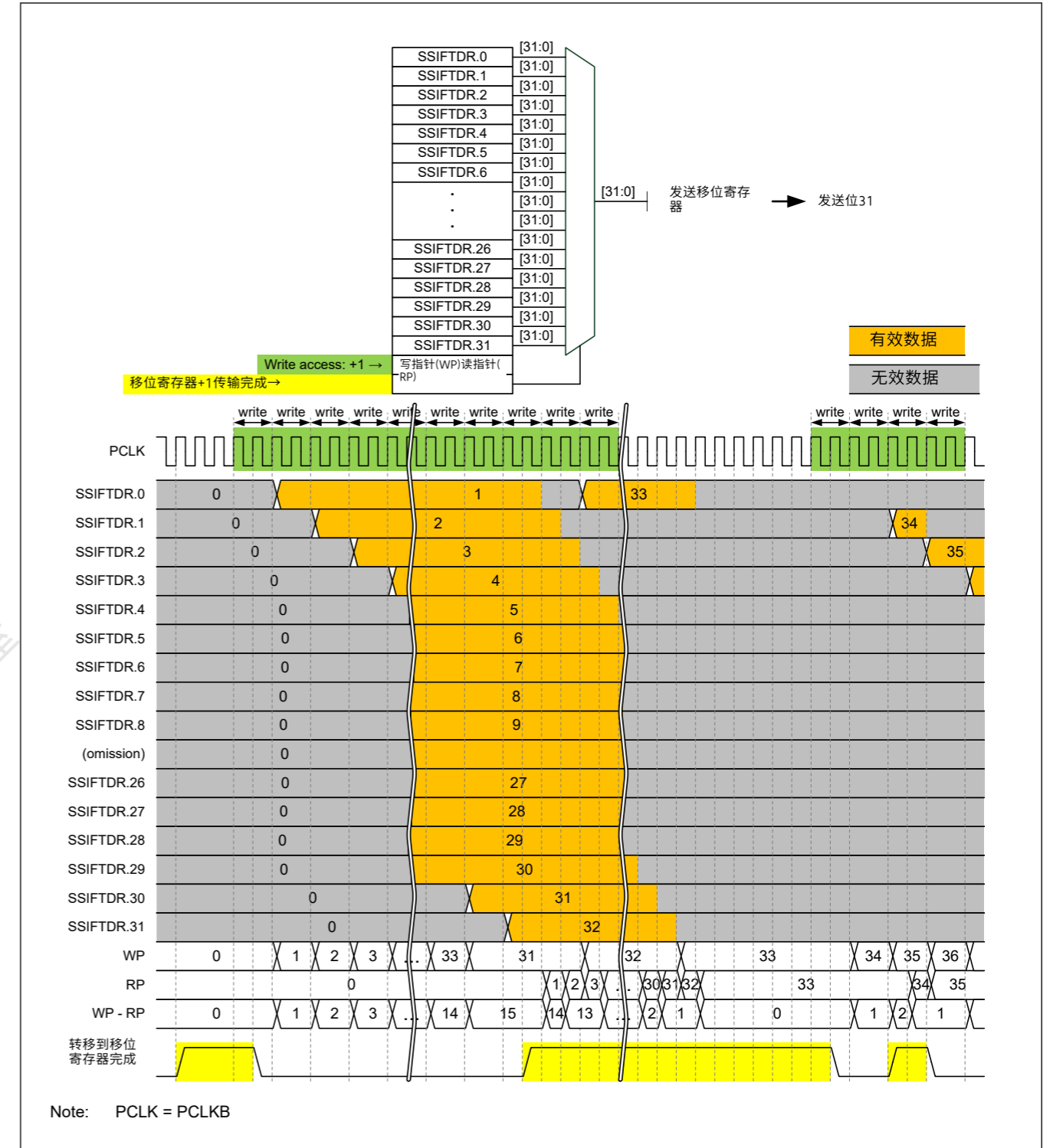
Figure 32.31 发送FIFO数据寄存器和发送移位寄存器的配置，以及FIFO操作示例
