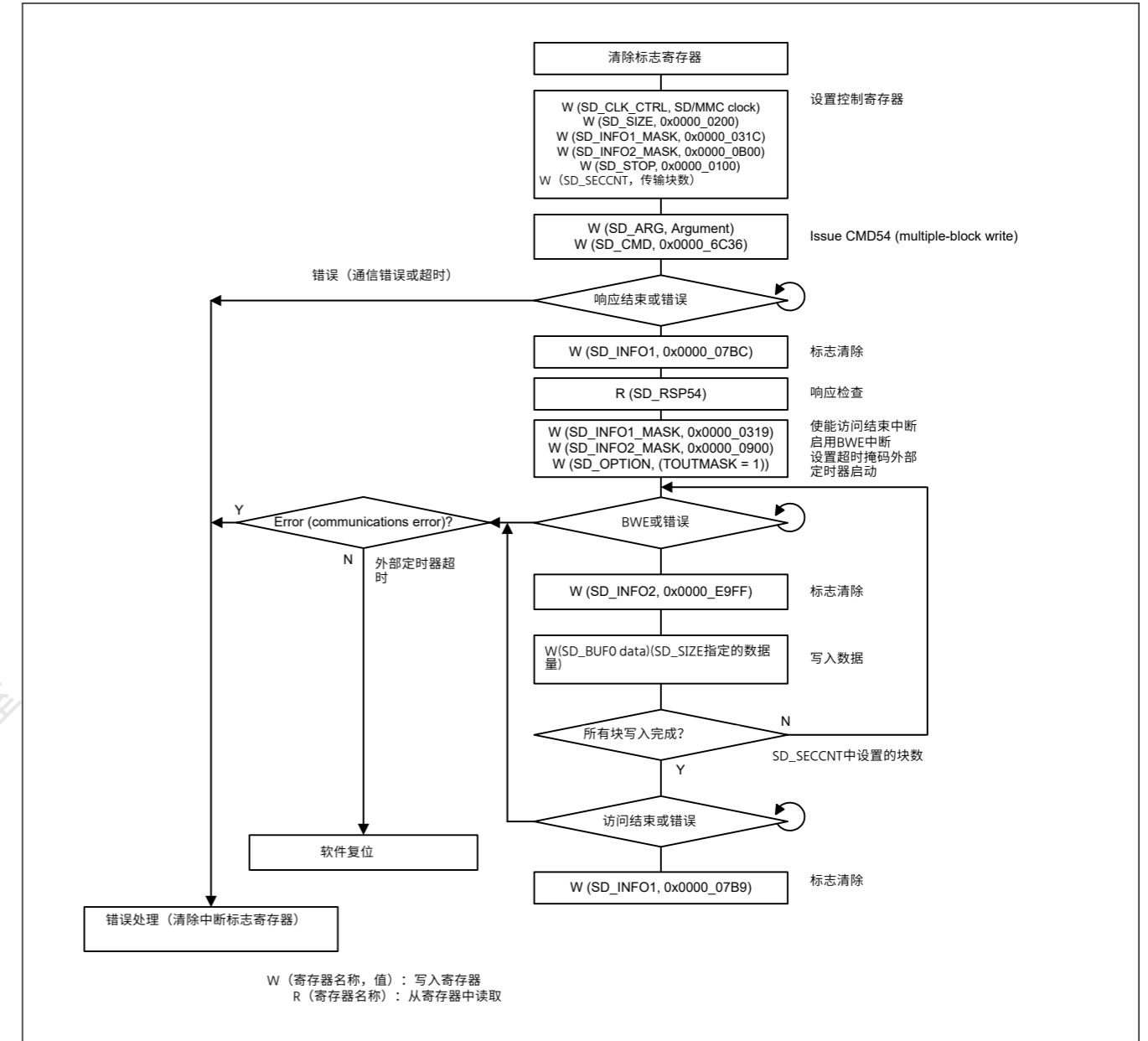
Figure 33.15 使用外部定时器的多块写入操作示例
