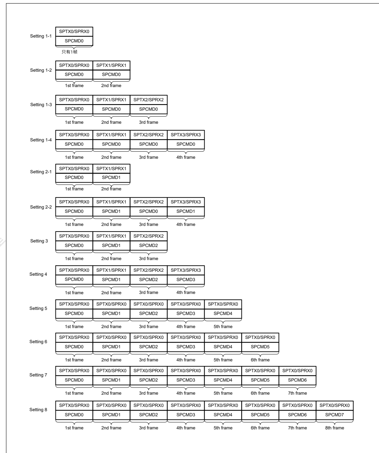
Figure 30.58 顺序操作中SPI命令寄存器与发送接收缓冲区的对应关系
