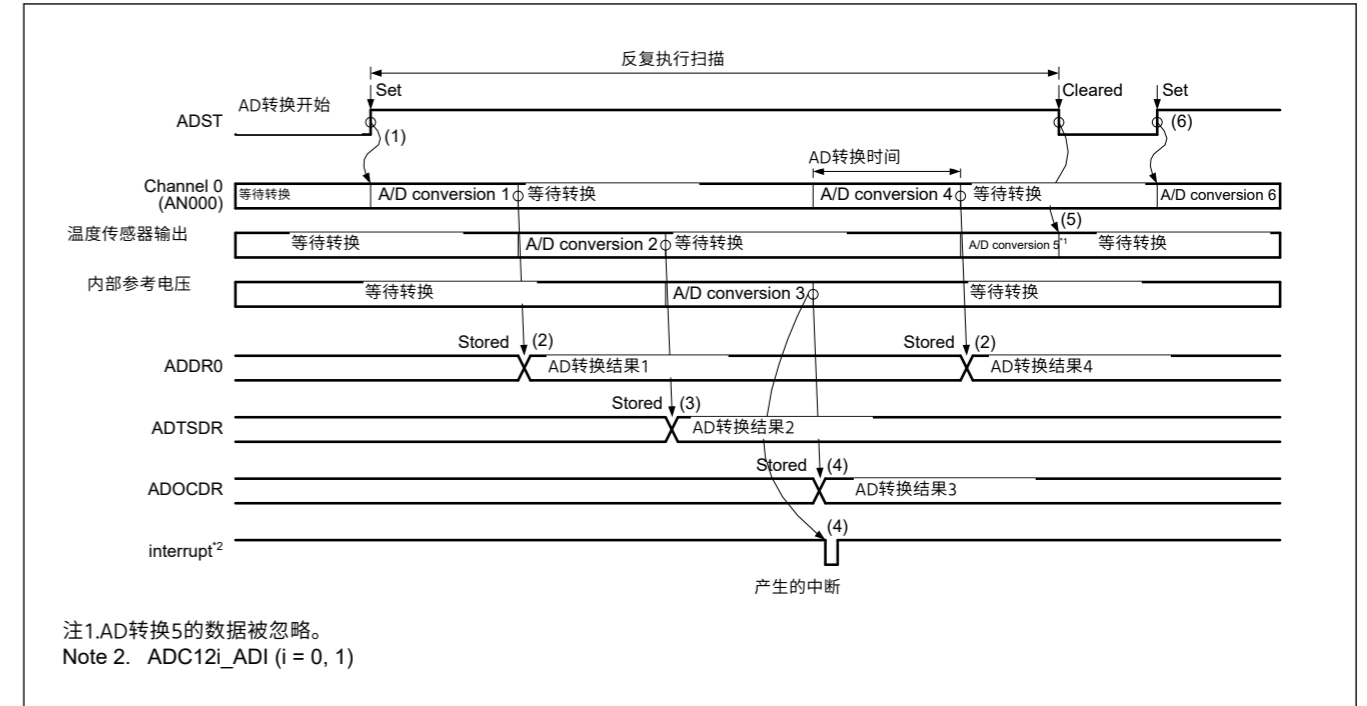
Figure 37.15 选择AN000和温度传感器输出或内部参考电压时连续扫描模式下的基本操作示例
