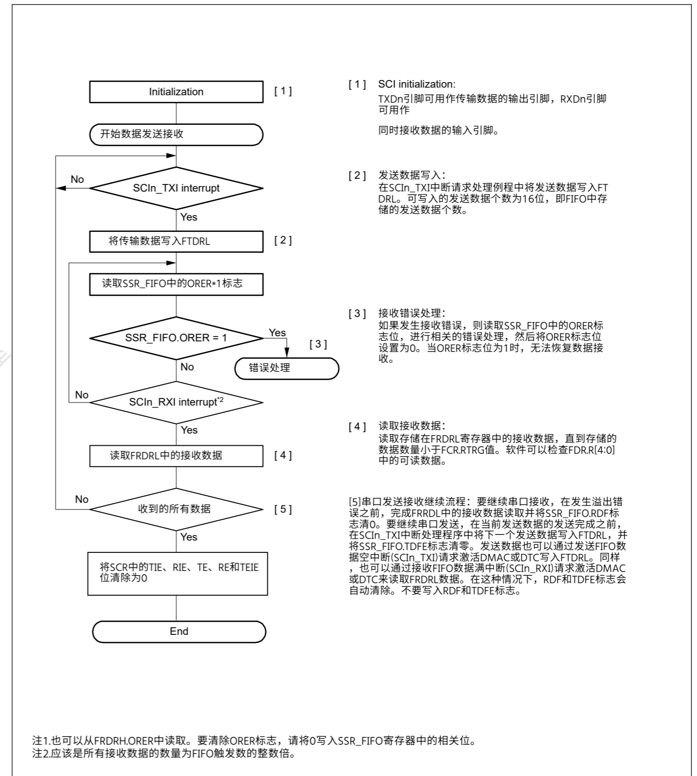
Figure 27.76 选择FIFO的时钟同步模式下同时串行发送和接收的示例流程
