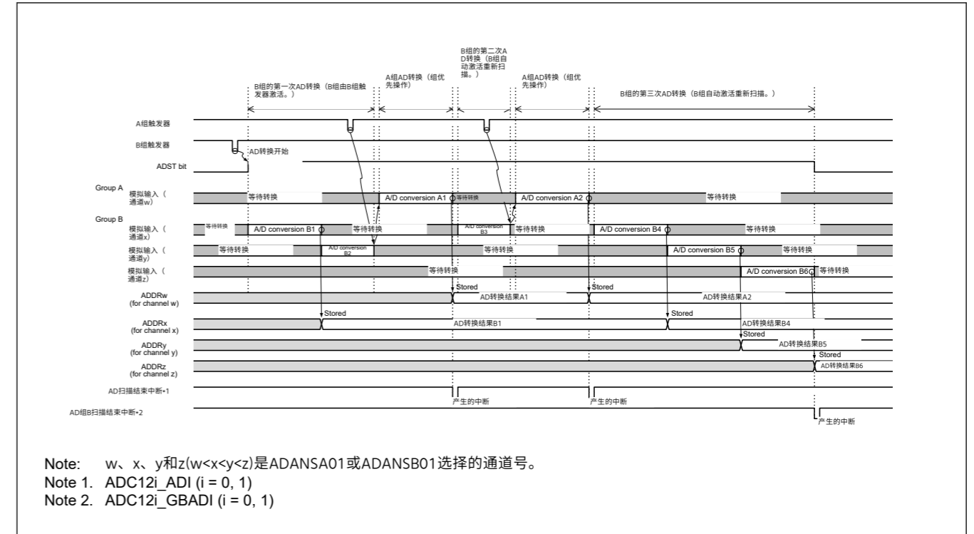
Figure 37.20 组优先操作1-2示例：启用重新扫描时（当ADGSPCR.GBRSCN=1、ADGSPCR.GBRP=0和ADGSPCR.LGRRS=0时）在B组重新扫描期间A组触发输入
