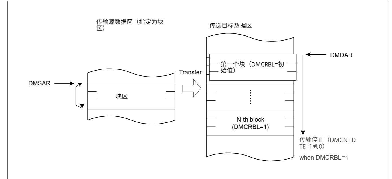
Figure 16.9 DMTMD.TKP位设置为0时块传输模式下的操作
