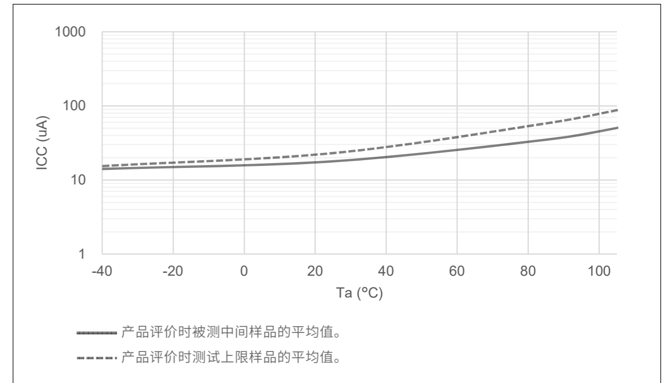
Figure 47.3 深度软件待机模式下的温度依赖性、为待机SRAM和USB恢复检测单元供电 (参考数据)
