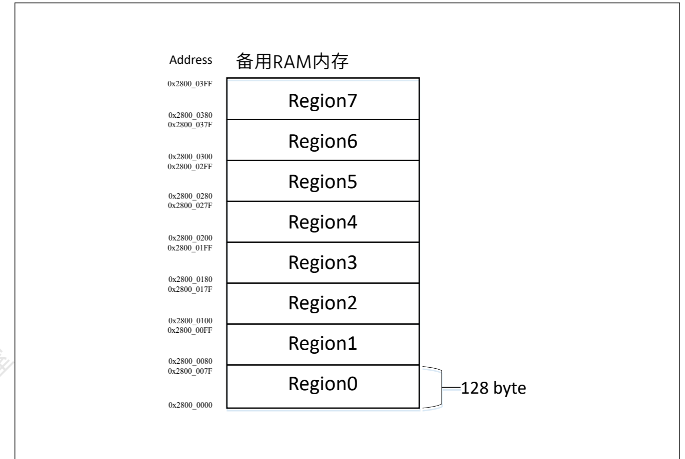
Figure 43.1 备用RAM区域
