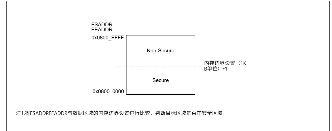
Figure 44.34 数据区域中的安全非安全区域
