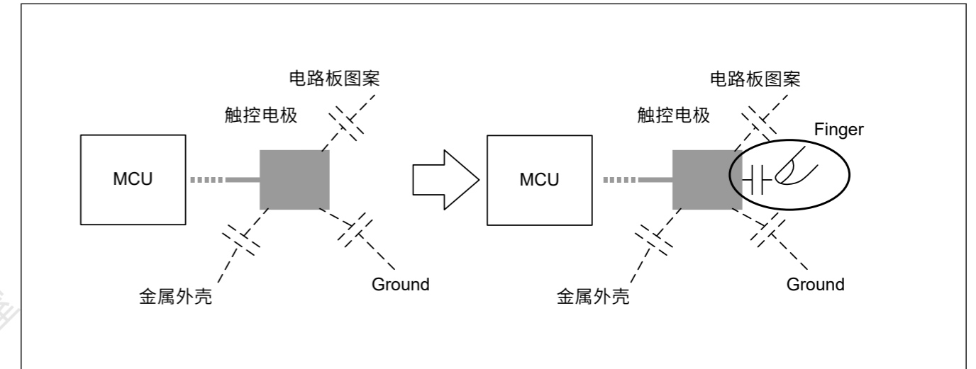
Figure 40.1 由于手指的存在而增加了静电电容
