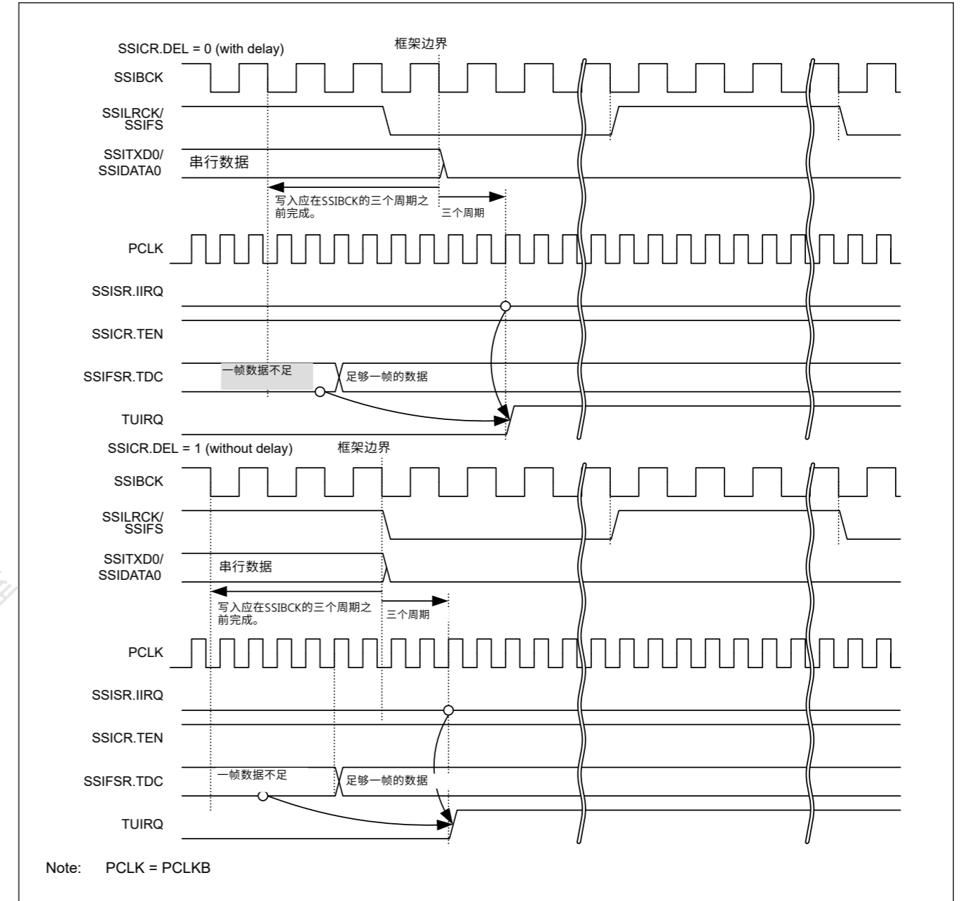
Figure 32.20 TUIRQ设置时间 (通信继续时)
