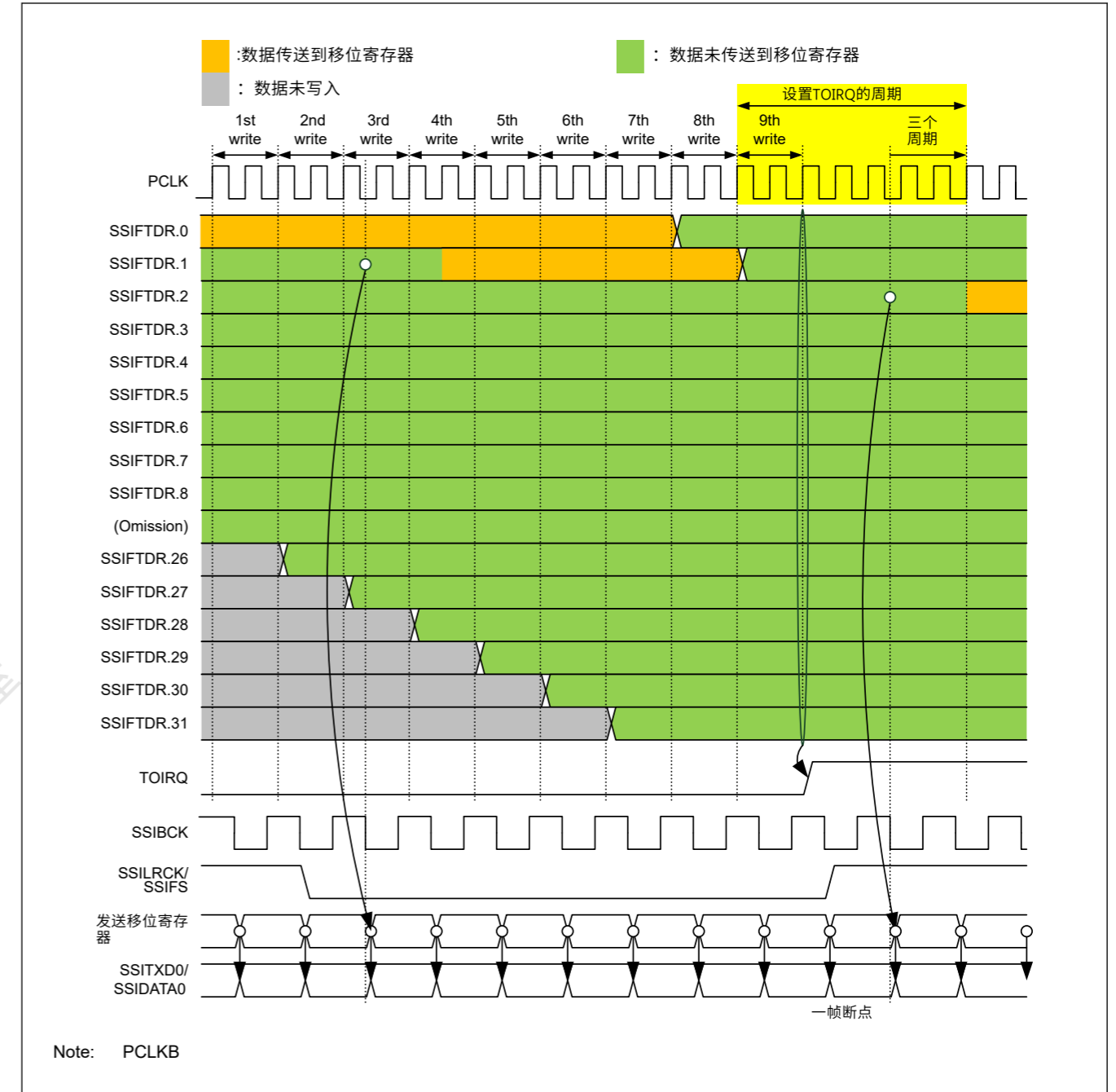
Figure 32.18 TOIRQ设置时序
