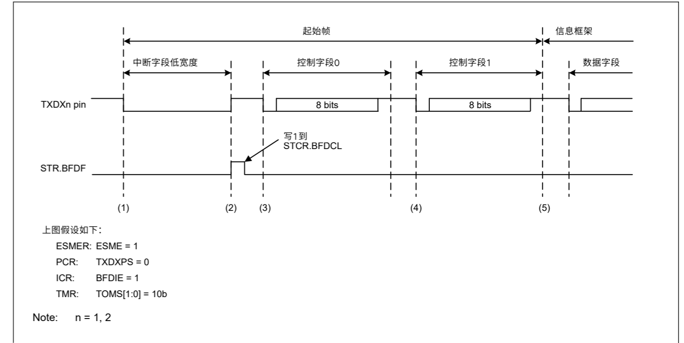
图27.102发送起始帧时的操作示例
