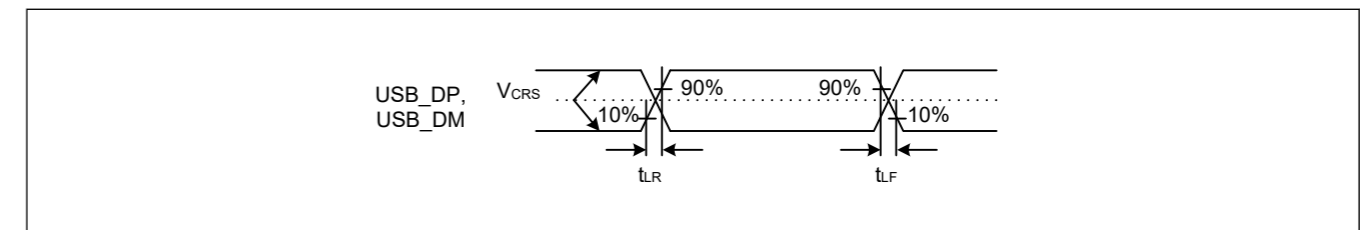
Figure 47.50 低速模式下的USB_DP和USB_DM输出时序
