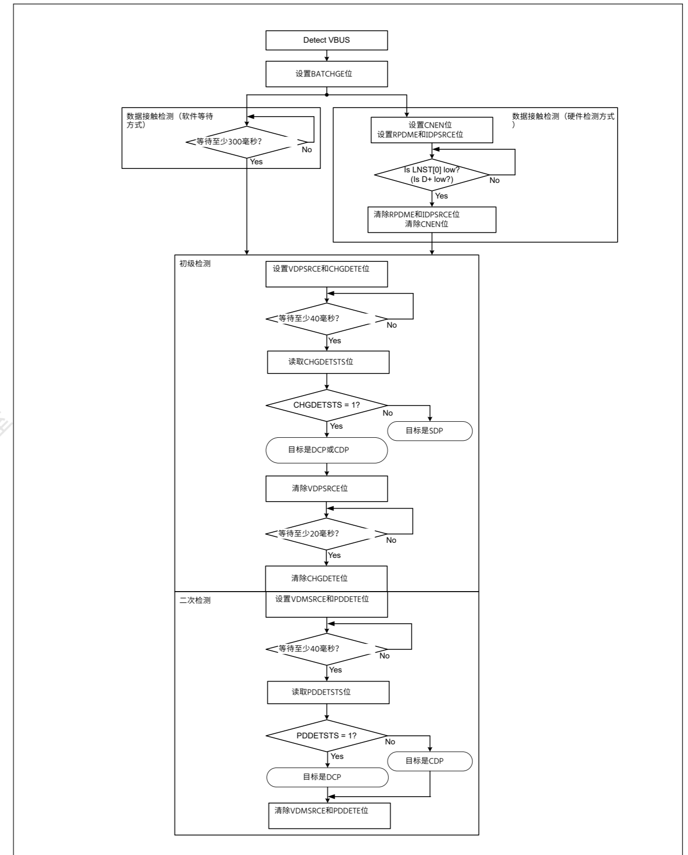
Figure 26.24 作为便携式设备的处理流程
