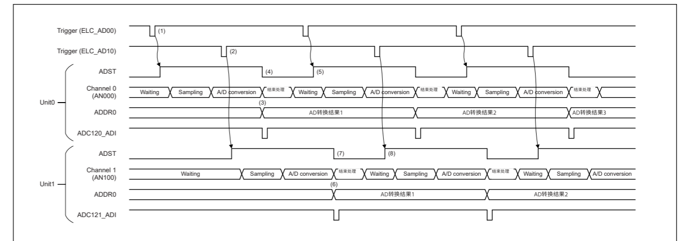
Figure 37.26 在交错操作中选择AN000和AN100时单扫描模式下的示例操作
