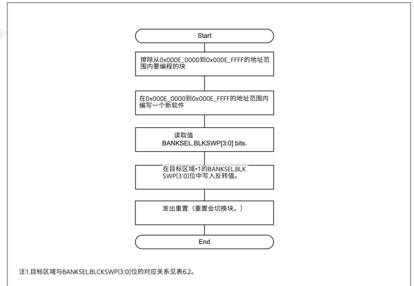
Figure 44.30 块交换选择流程示例 (适用于具有1MB代码闪存的产品)
