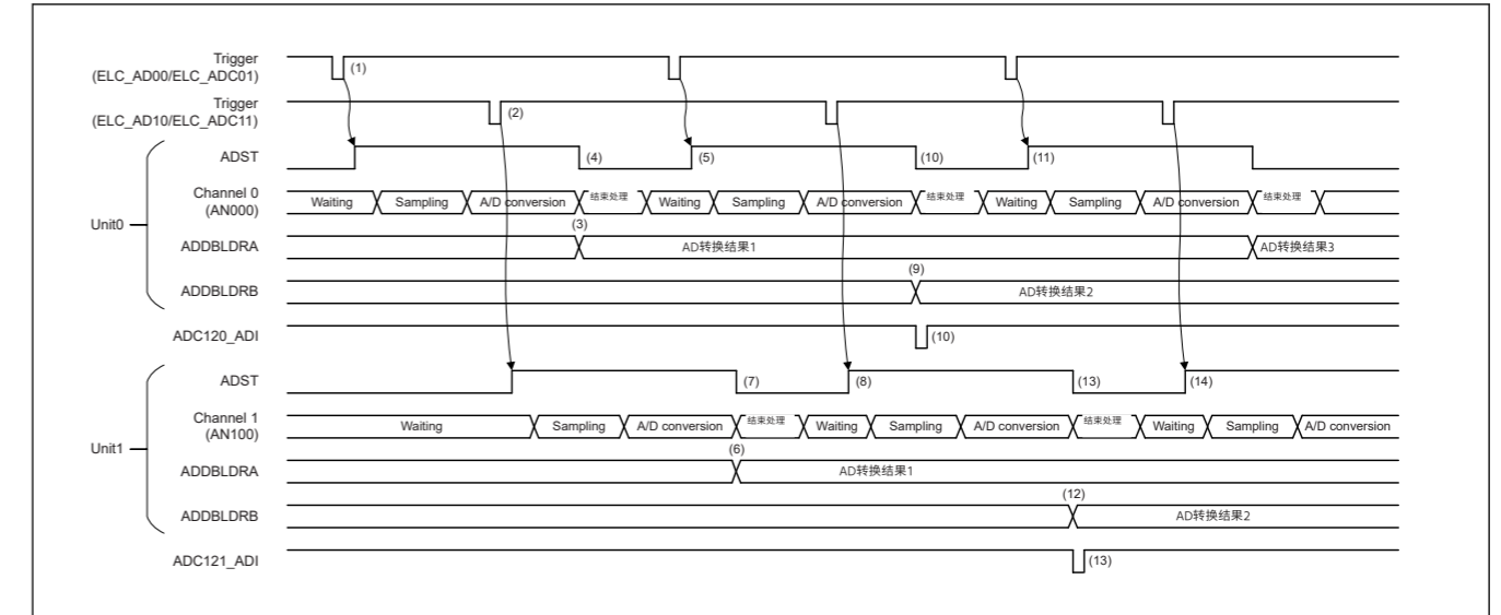
Figure 37.27 当AN000和扩展双触发模式时，单扫描模式下的示例操作 AN100在交错操作中选择
