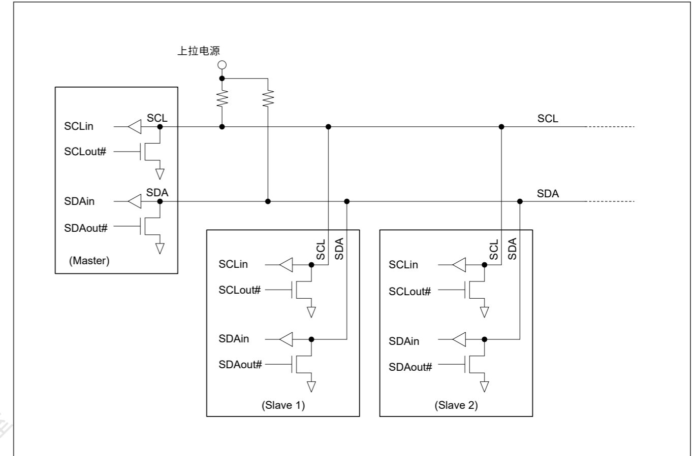
Figure 28.2 IO引脚连接到外部电路 (I2C总线配置示例)
