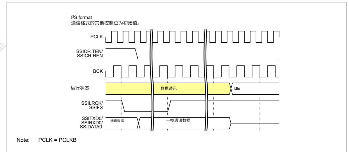
Figure 32.48 停止数据通信（无填充位）
