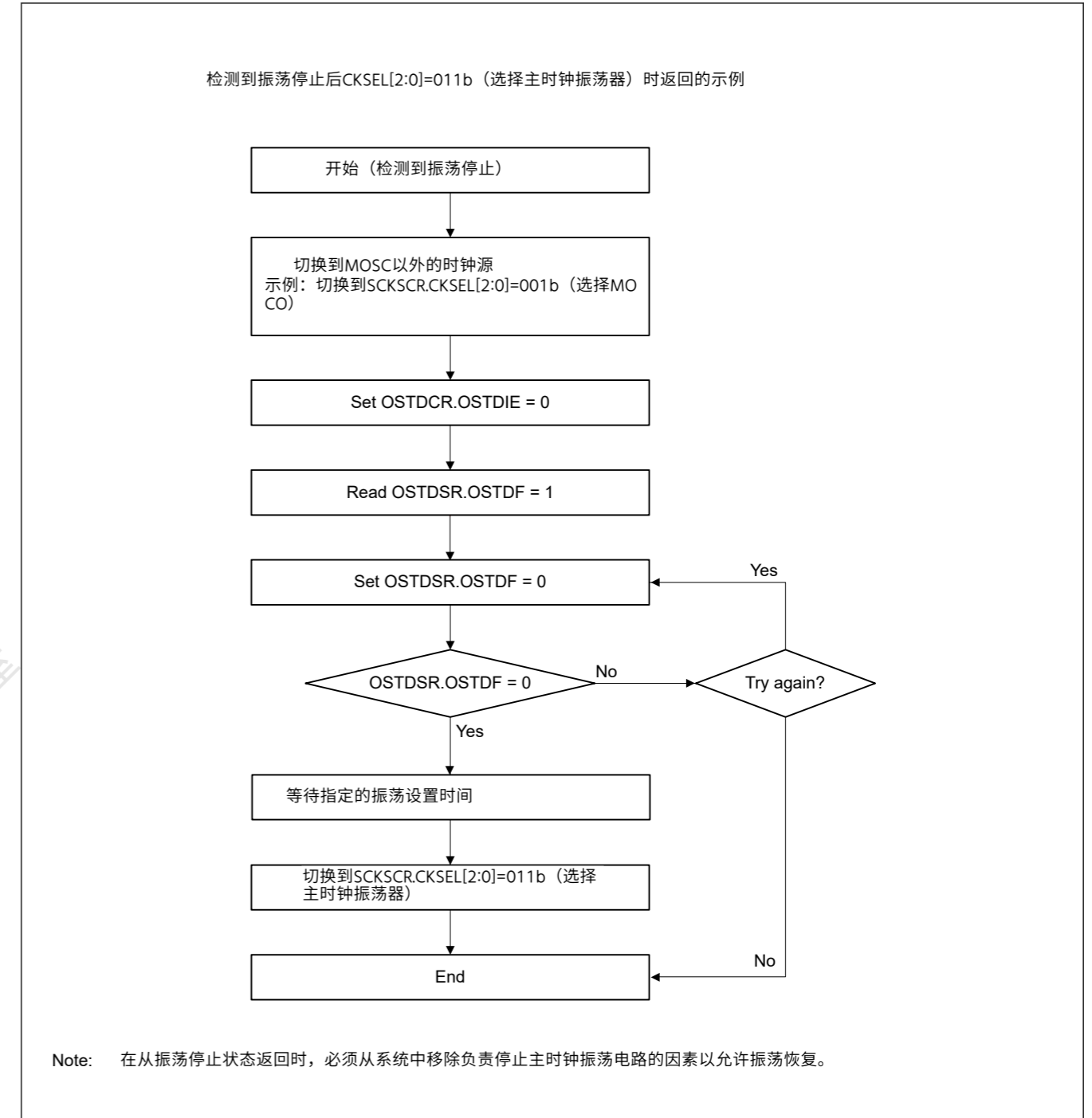
Figure 8.8 检测到振荡器停止时的恢复流程
