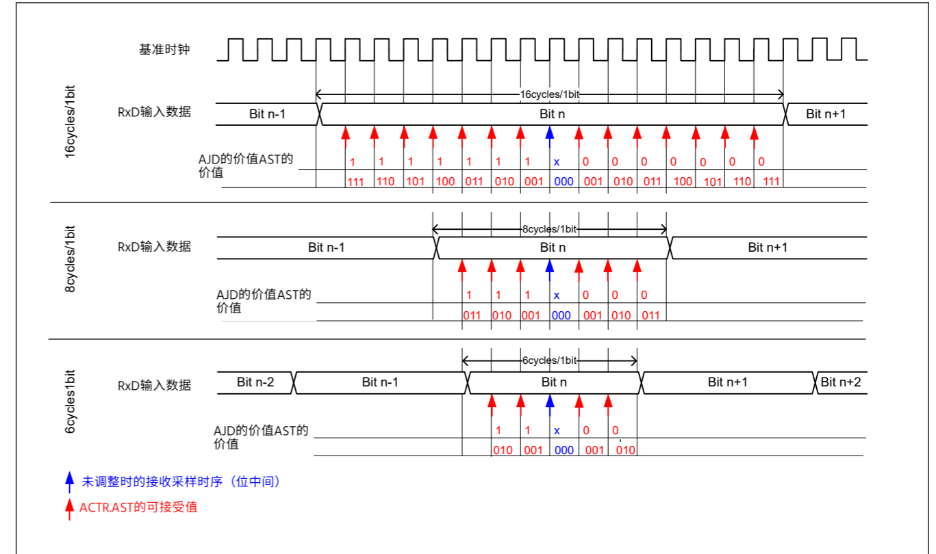
Figure 27.34 接收采样时序调整操作说明 (使用内部时钟的异步模式)
