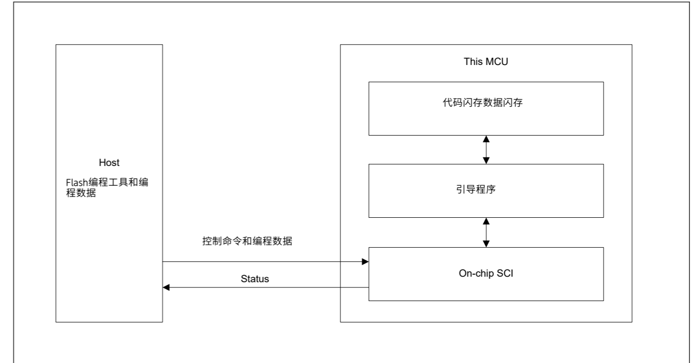
Figure 44.40 引导模式下操作的系统配置（用于SCI接口）
