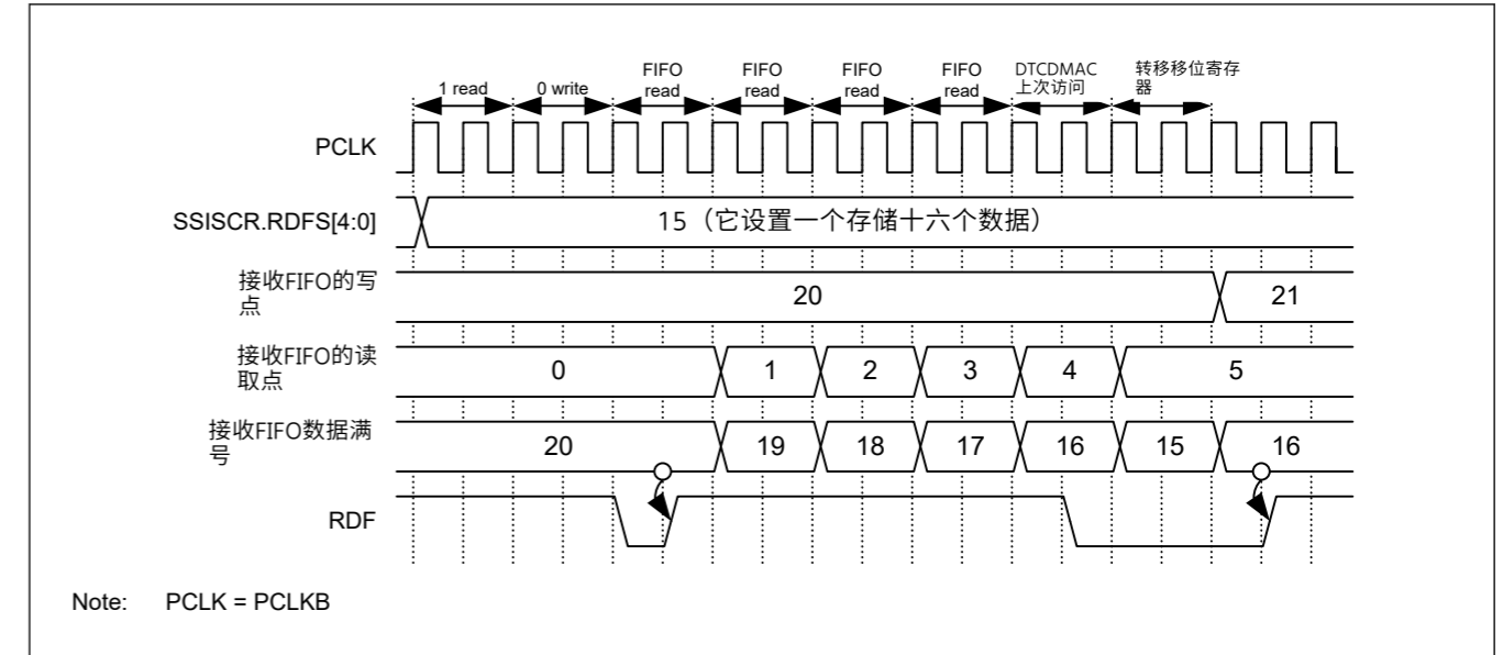
Figure 32.28 设置和清除RDF的时序图
