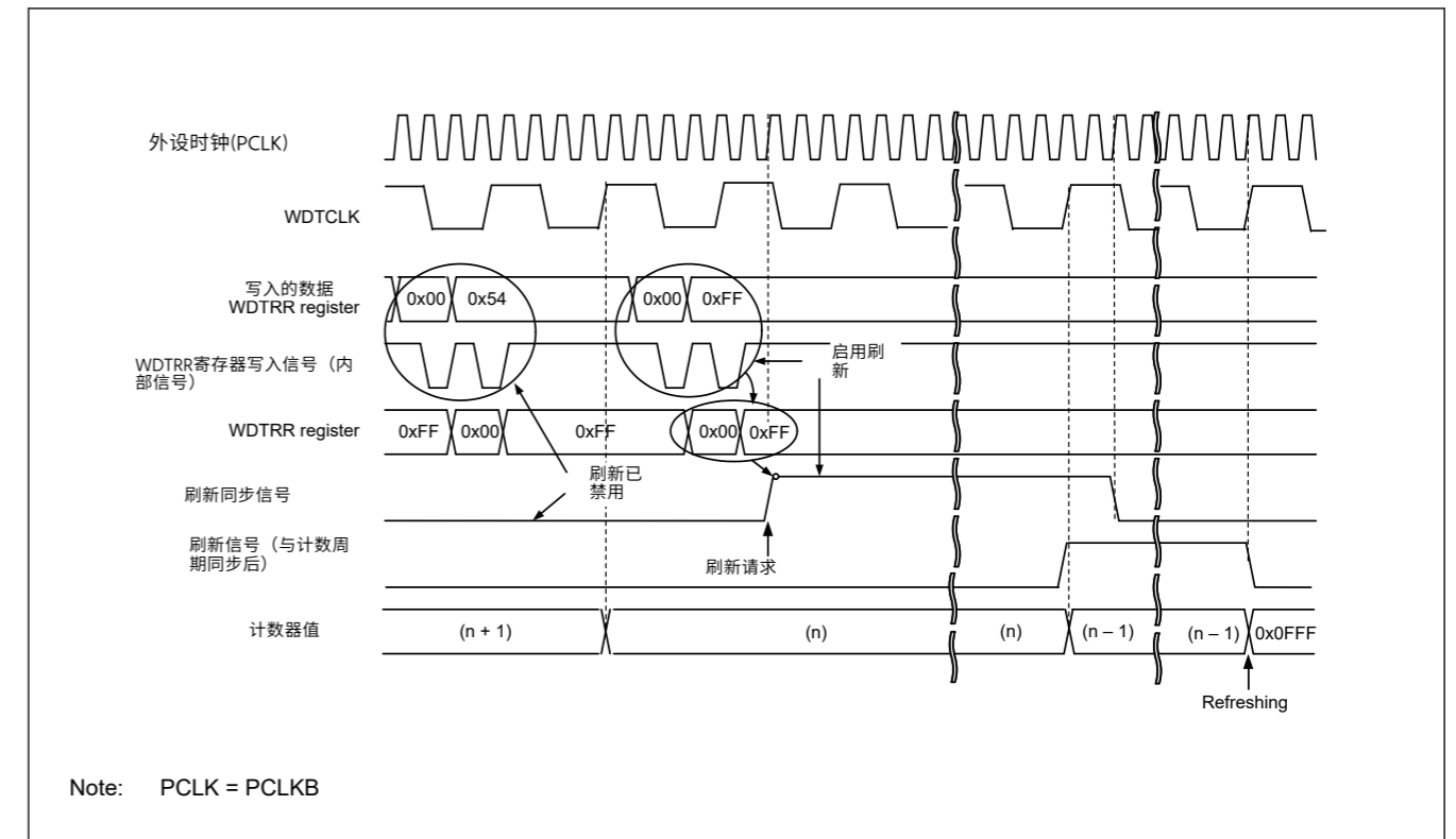
Figure 24.6 WDTCSR.CKS[3:0]=0x4和WDTCSR.TOPS[1:0]=01b时的WDT刷新操作波形
