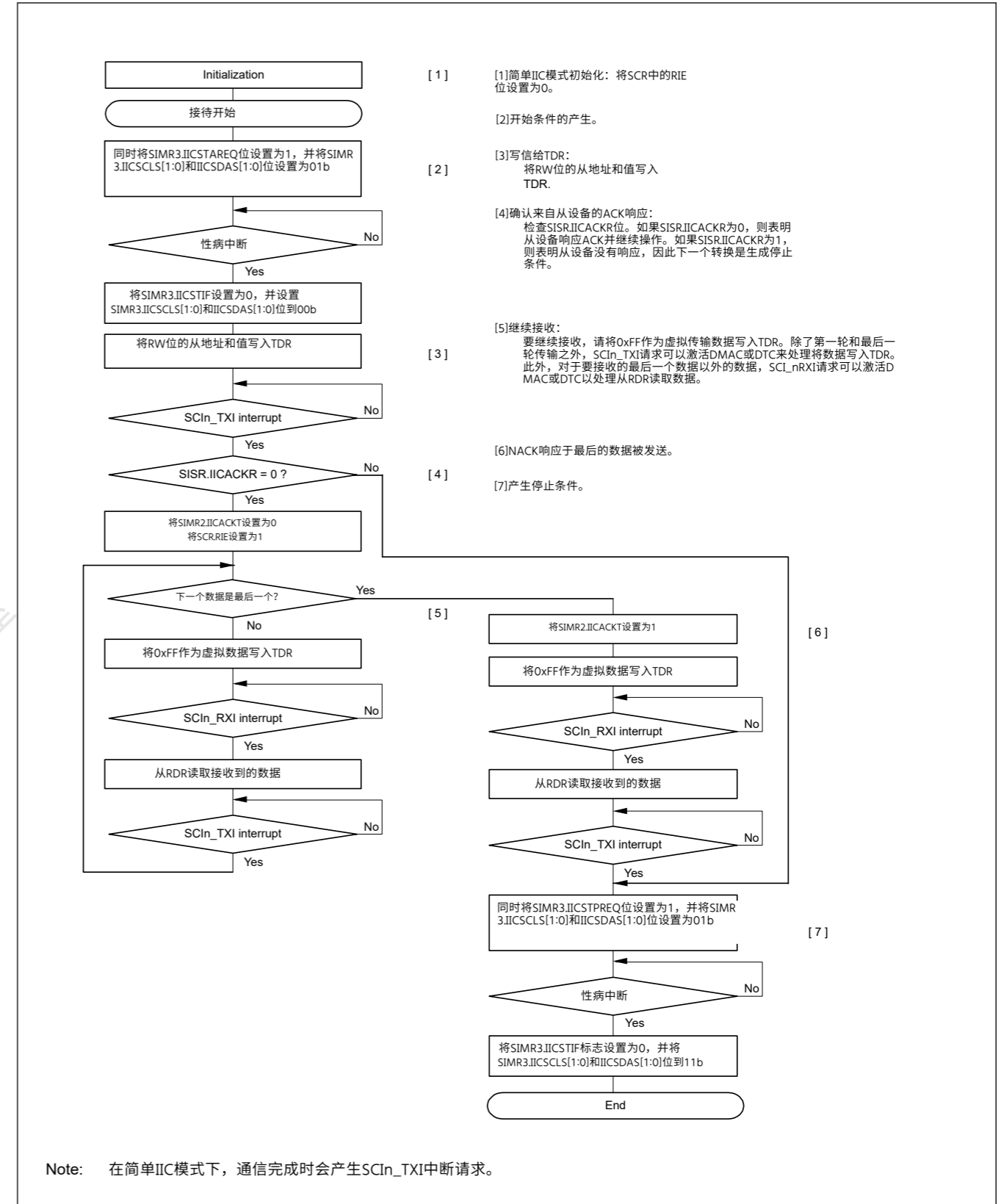
Figure 27.97 带有发送中断和接收中断的简单IIC模式下的主机接收示例流程
