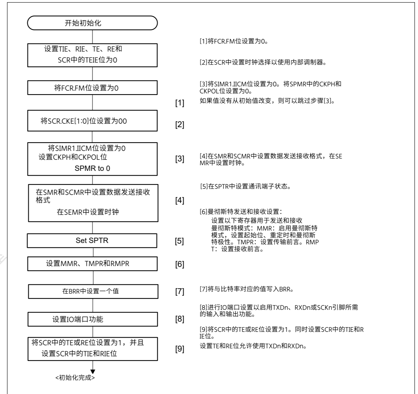
Figure 27.54 曼彻斯特模式下的SCI初始化流程
