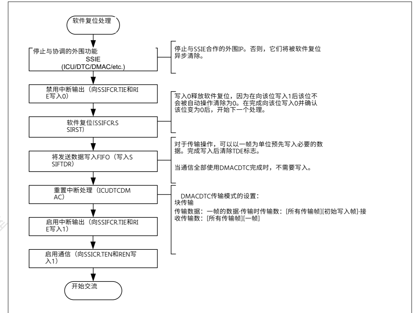
Figure 32.61 软件复位程序 (CPU操作程序)
