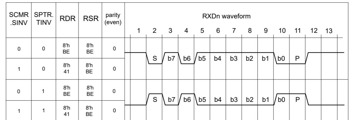
Figure 27.5 接收发送数据控制示例
