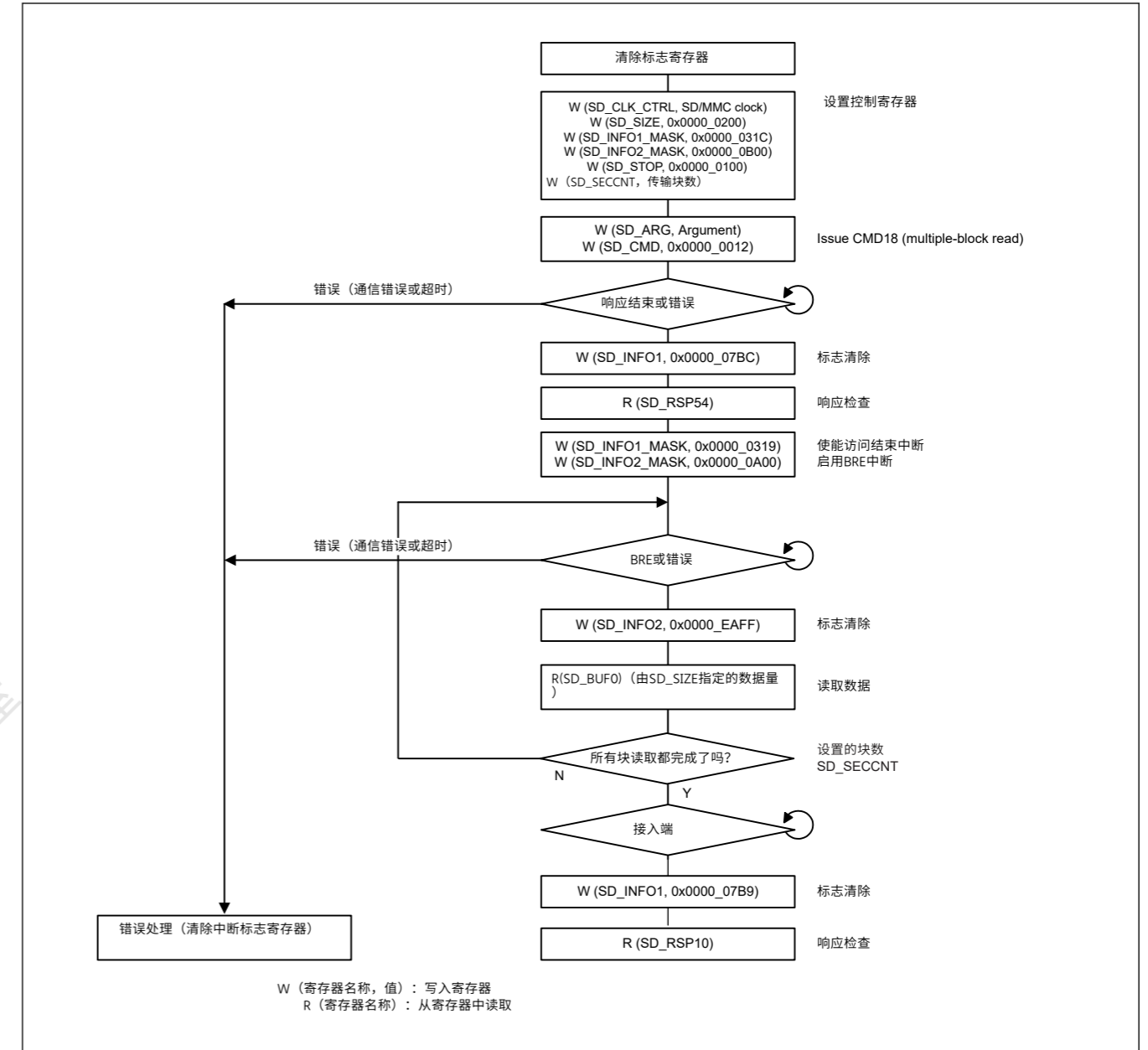
Figure 33.13 多块读取操作示例
