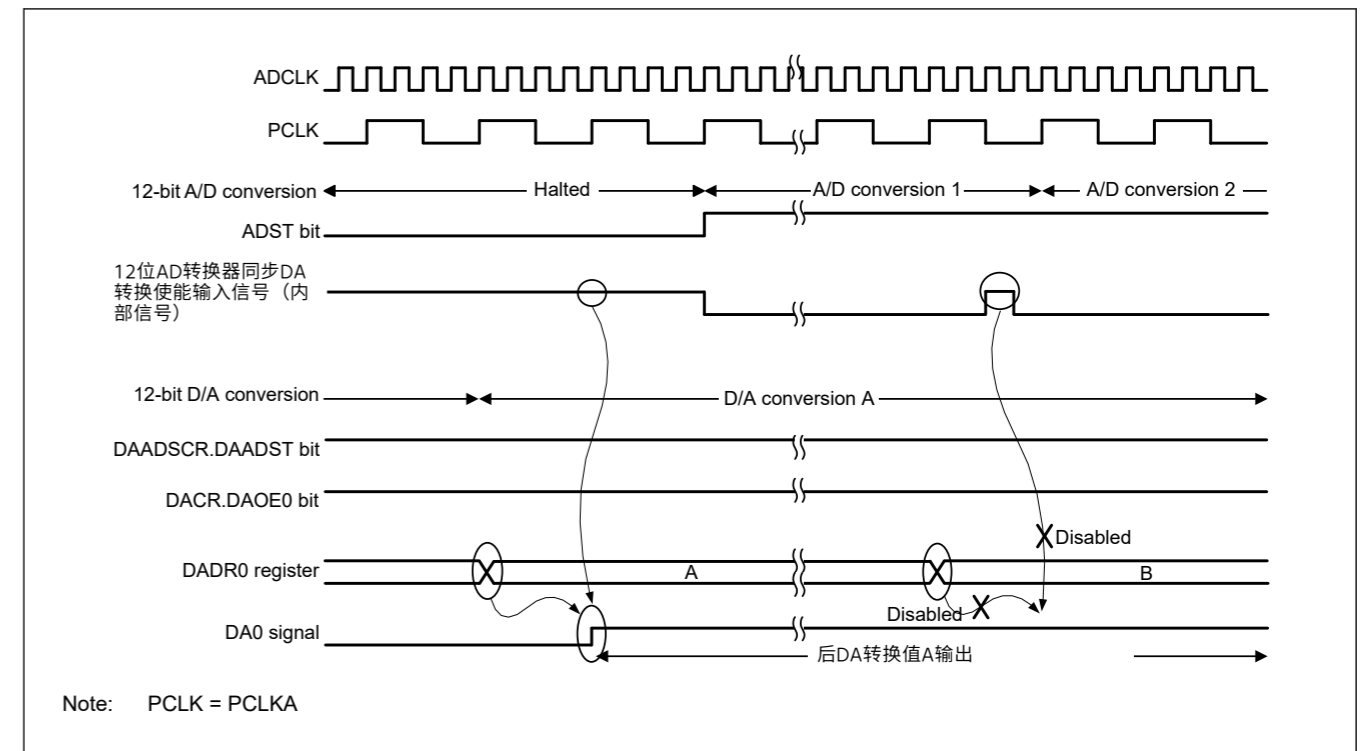
Figure 38.4 DAC12无法捕获来自ADC12 (单元1) 的同步DA转换使能输入信号时的示例
