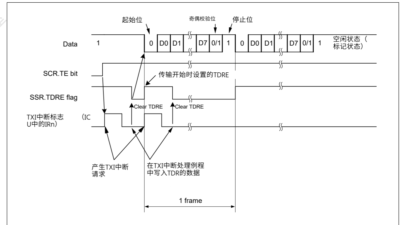
Figure 27.14 异步模式下串行传输的操作示例(4) (使用8位数据,奇偶校验,1个停止位,未使用CTS功能,从传输中间到传输完成,停止序言)
