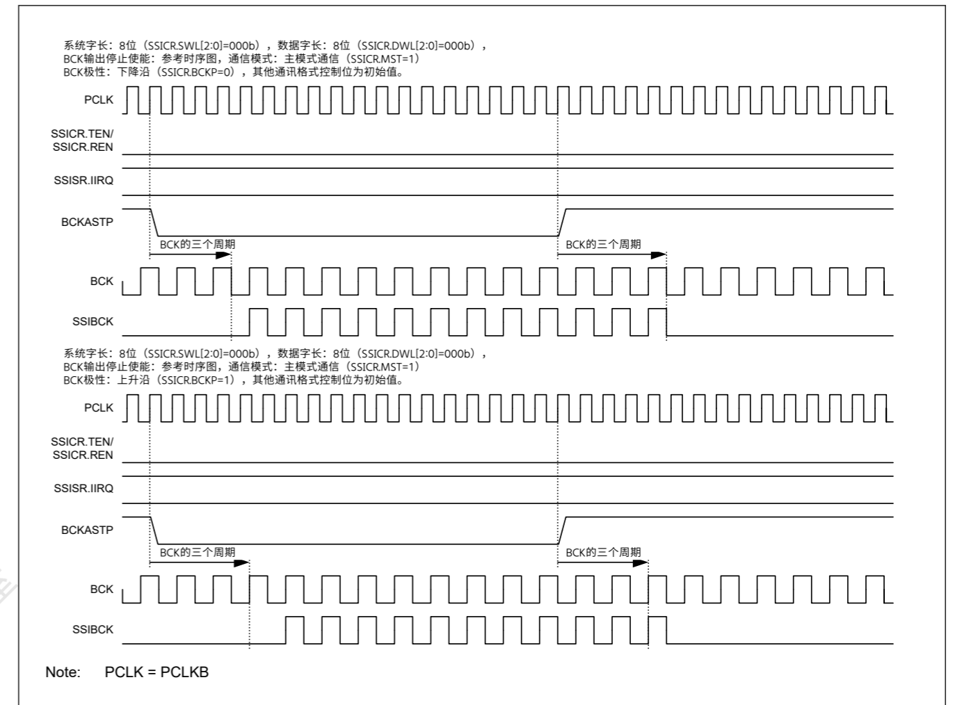
Figure 32.34 BCKASTP位的示例操作 (空闲状态)
