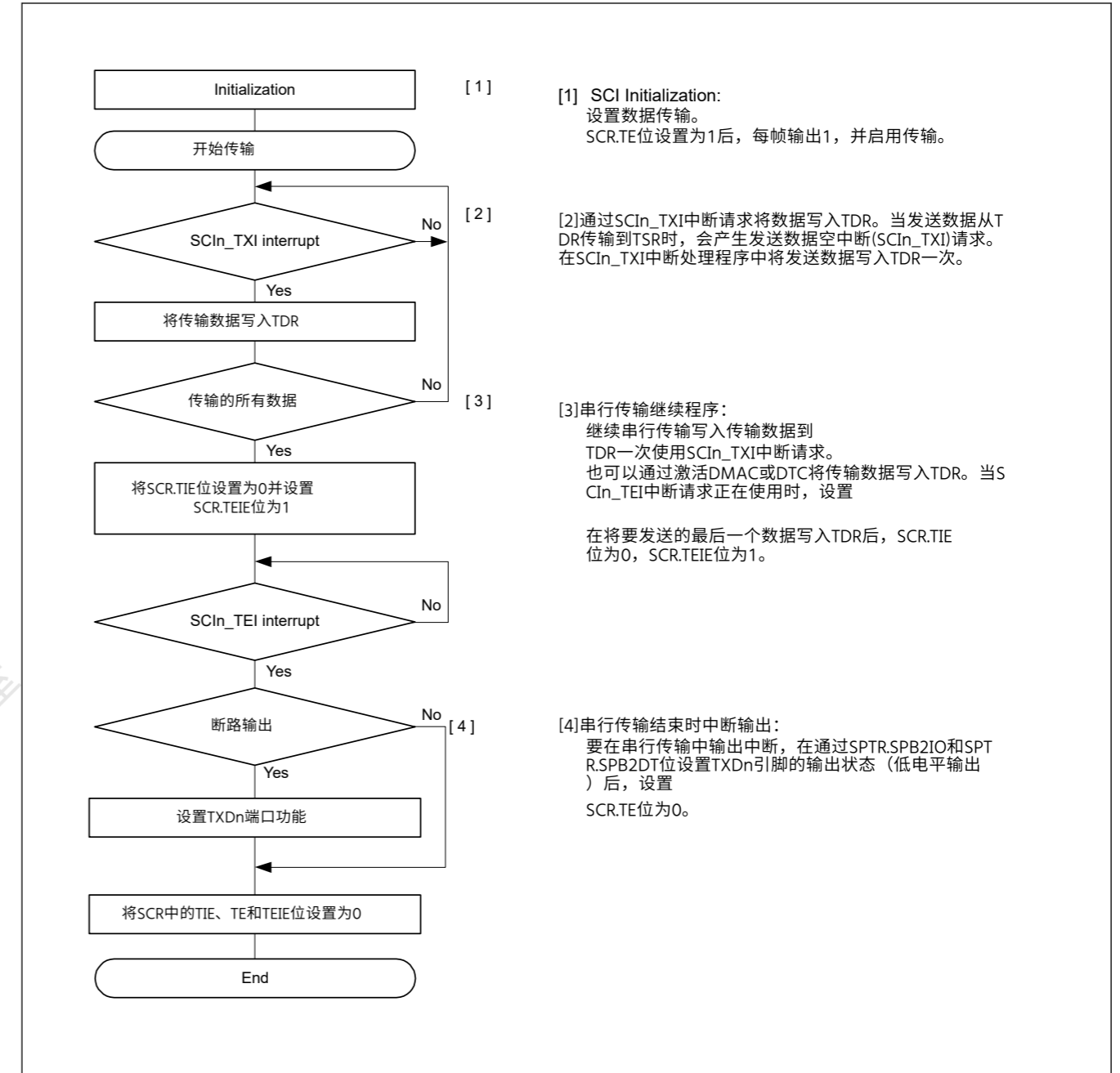
Figure 27.15 选择非FIFO的异步模式下串行传输示例流程
