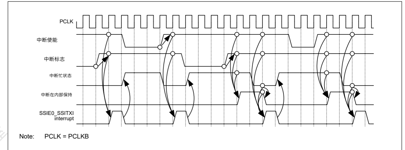
Figure 32.60 SSIE0_SSITXI中断时序图
