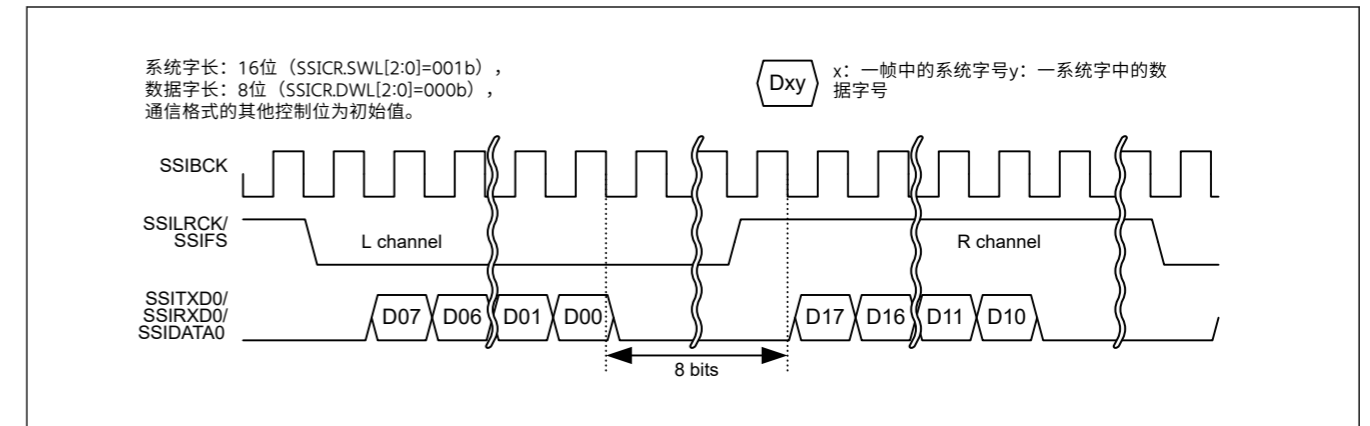
Figure 32.36 填充位传输示例 (I 2 S格式: 系统字长>数据字长)
