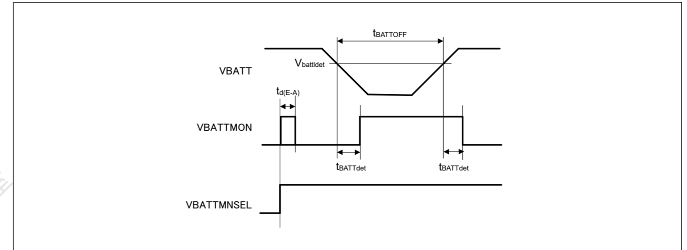
Figure 47.61 电池备份功能特点
