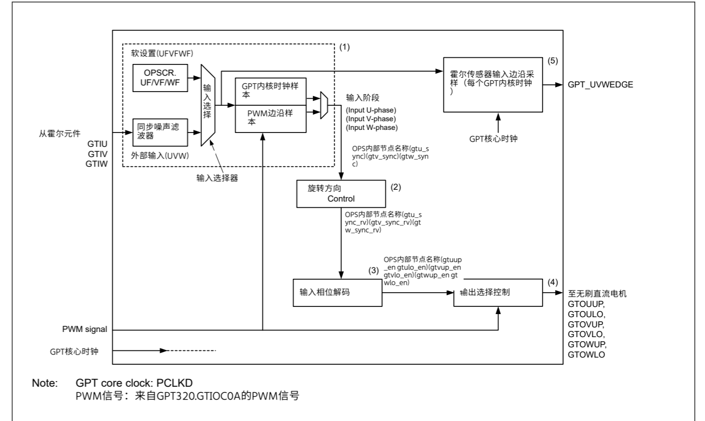
Figure 21.57 GPT_OPS控制流程概念图
