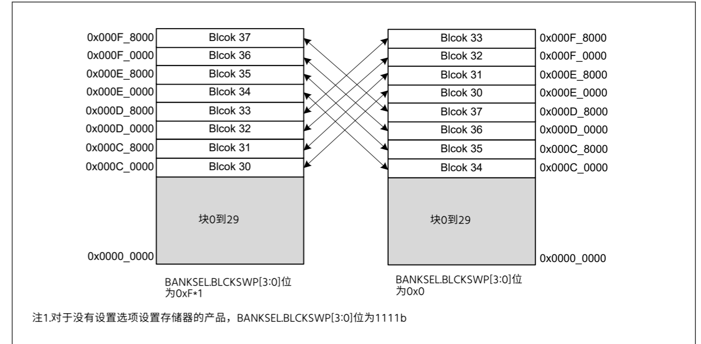
Figure 44.29 块交换选择示例 (适用于具有1MB代码闪存的产品)
