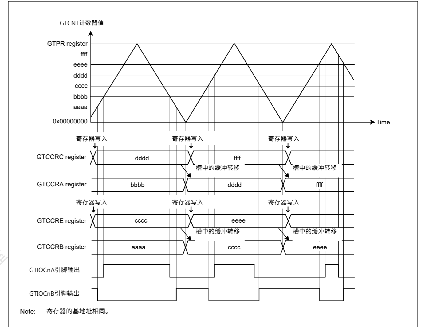
Figure 21.21 带缓冲操作的三角波PWM模式1操作示例，从GTIOCnA引脚和GTIOCnB引脚在计数开始时的高电平输出，输出在GTCCRA/GTCCRB寄存器比较匹配，并在循环结束时保留输出
