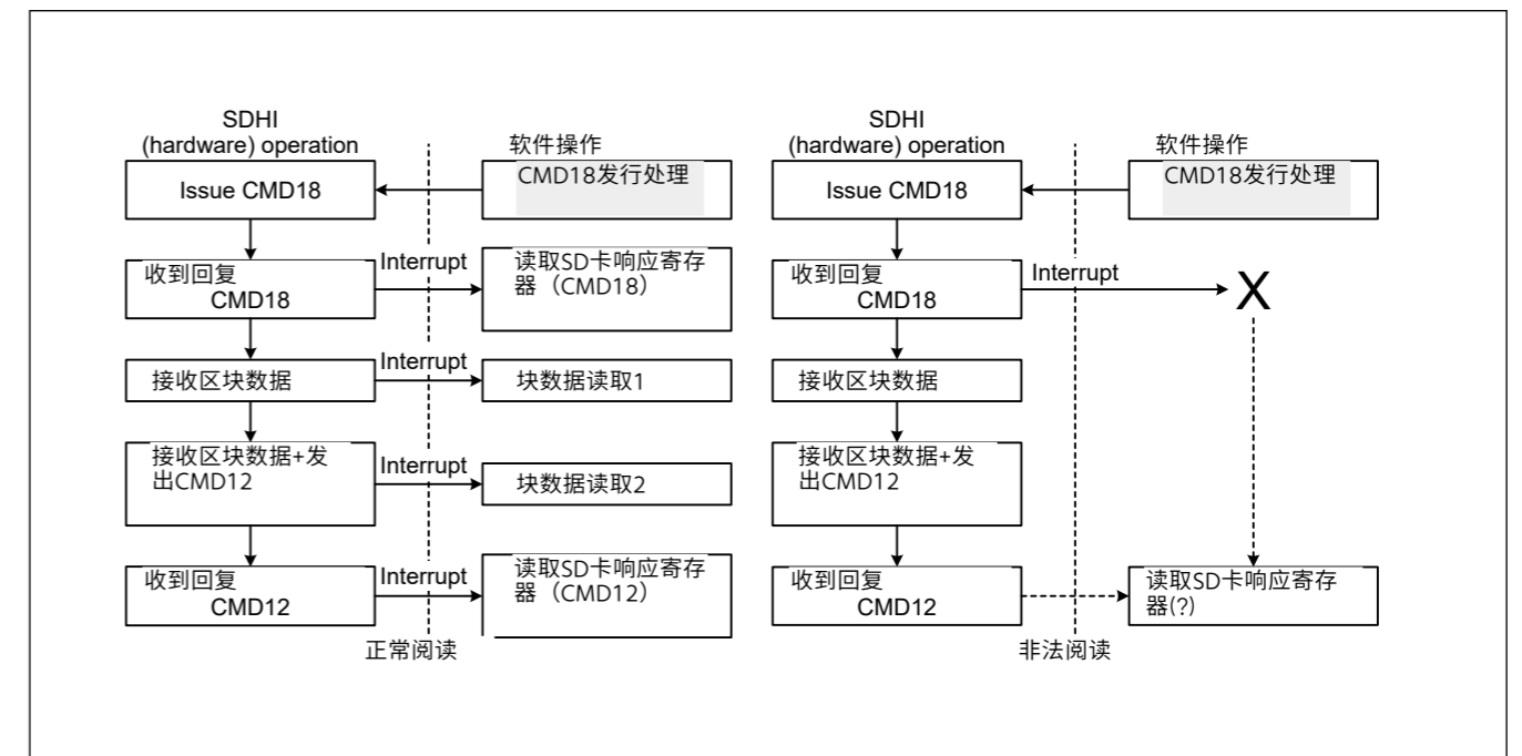
Figure 33.25 多块读取操作流程图 (两个块)
