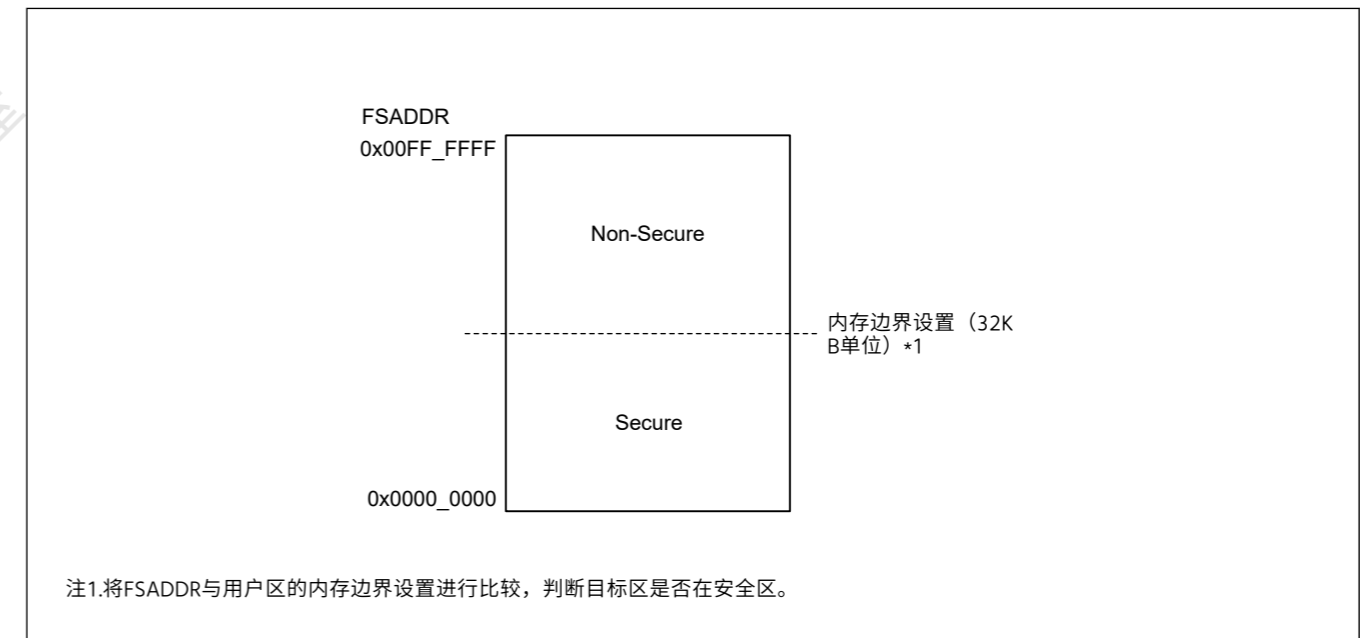
Figure 44.33 用户区域中的安全非安全区域
