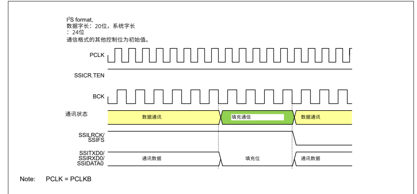
Figure 32.49 从数据通经过渡到填充通信
