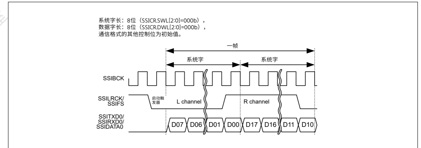
Figure 32.37 I 2 S格式 (无填充: 系统字长=数据字长)
