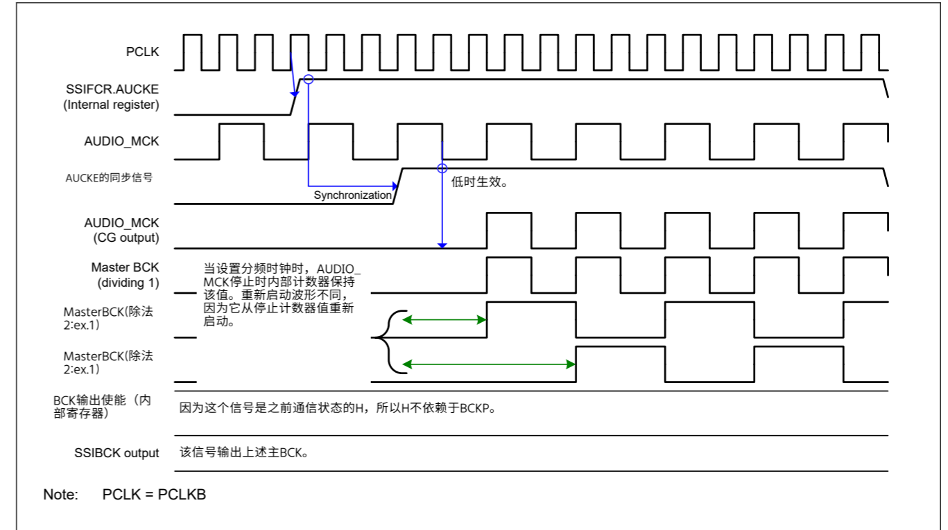
Figure 32.27 从停止通信到开始主模式通信的操作时序图
