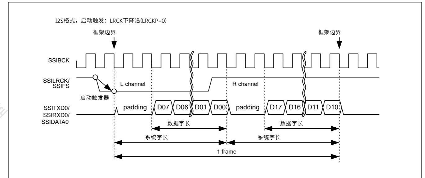
Figure 32.1 通讯格式的定义
