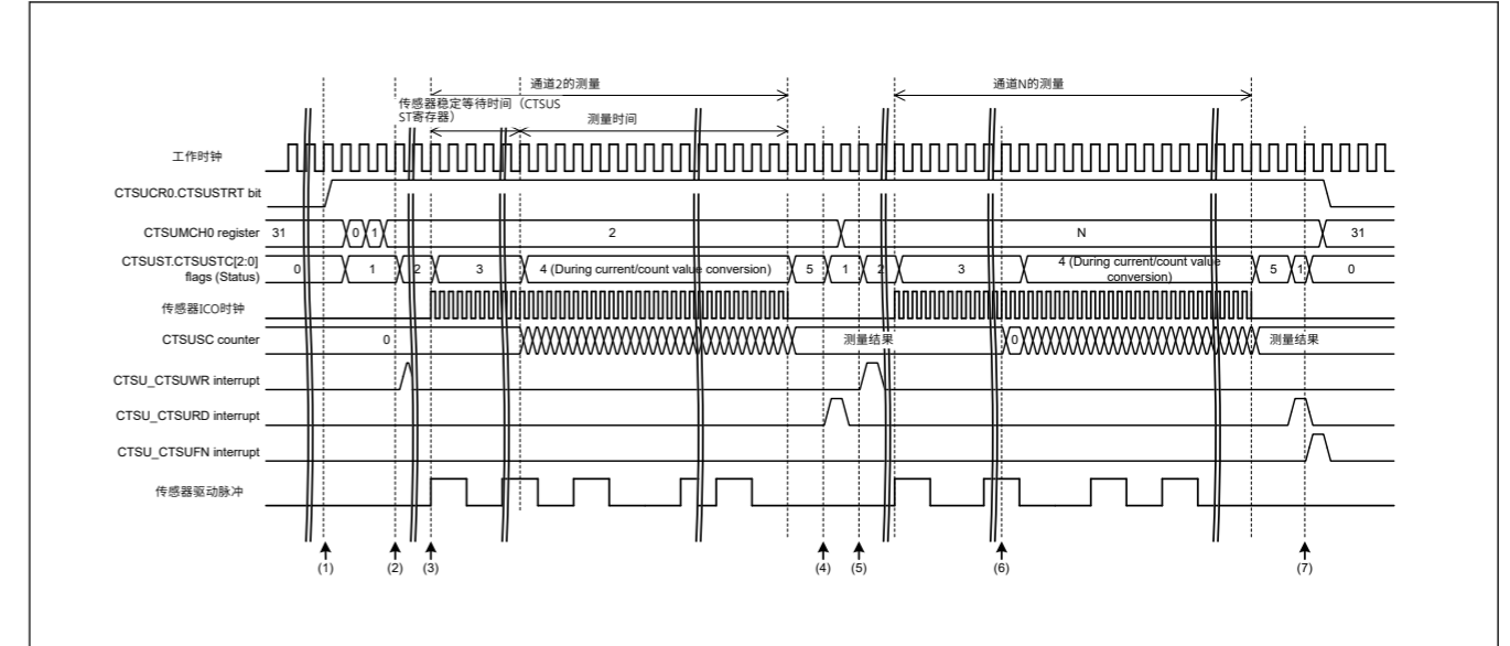
Figure 40.15 测量开始条件为软件触发时的自电容多次扫描模式时序
