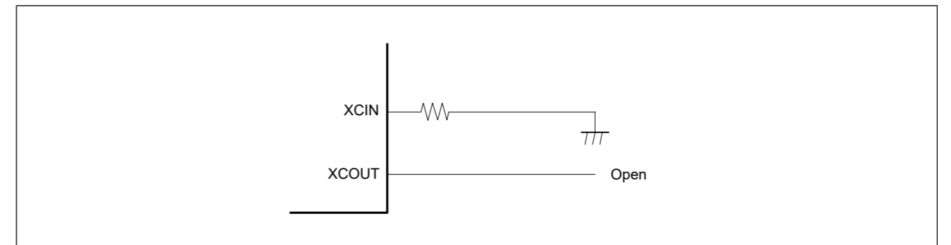
Figure 8.7 不使用副时钟振荡器时的引脚处理
