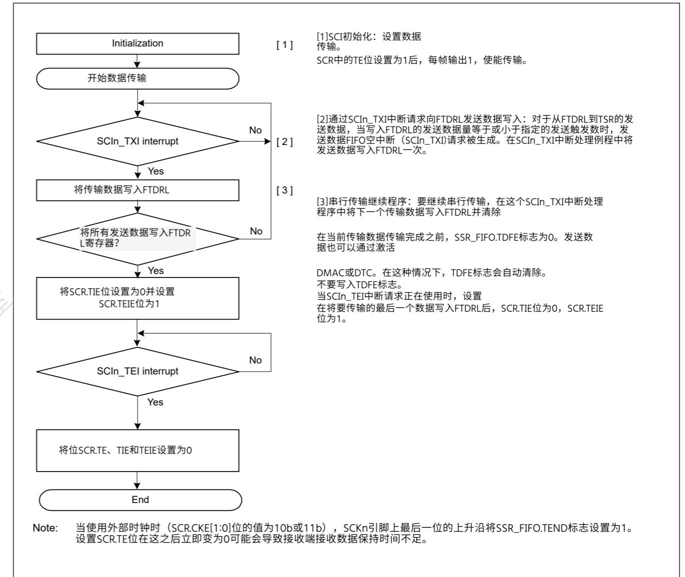
Figure 27.70 选择FIFO的时钟同步模式下的串行传输示例流程
