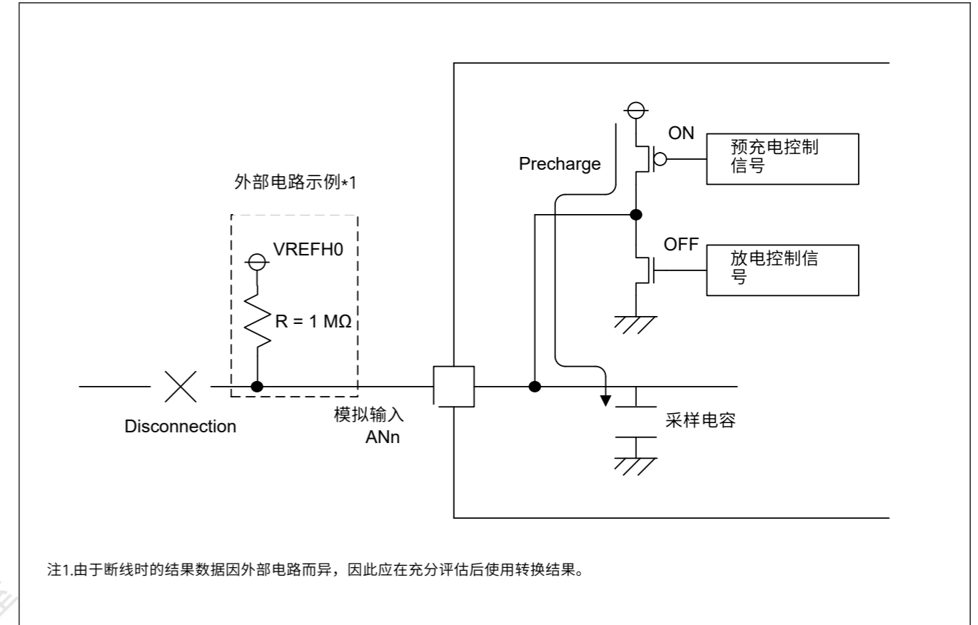
Figure 37.34 选择预充电时的断线检测示例
