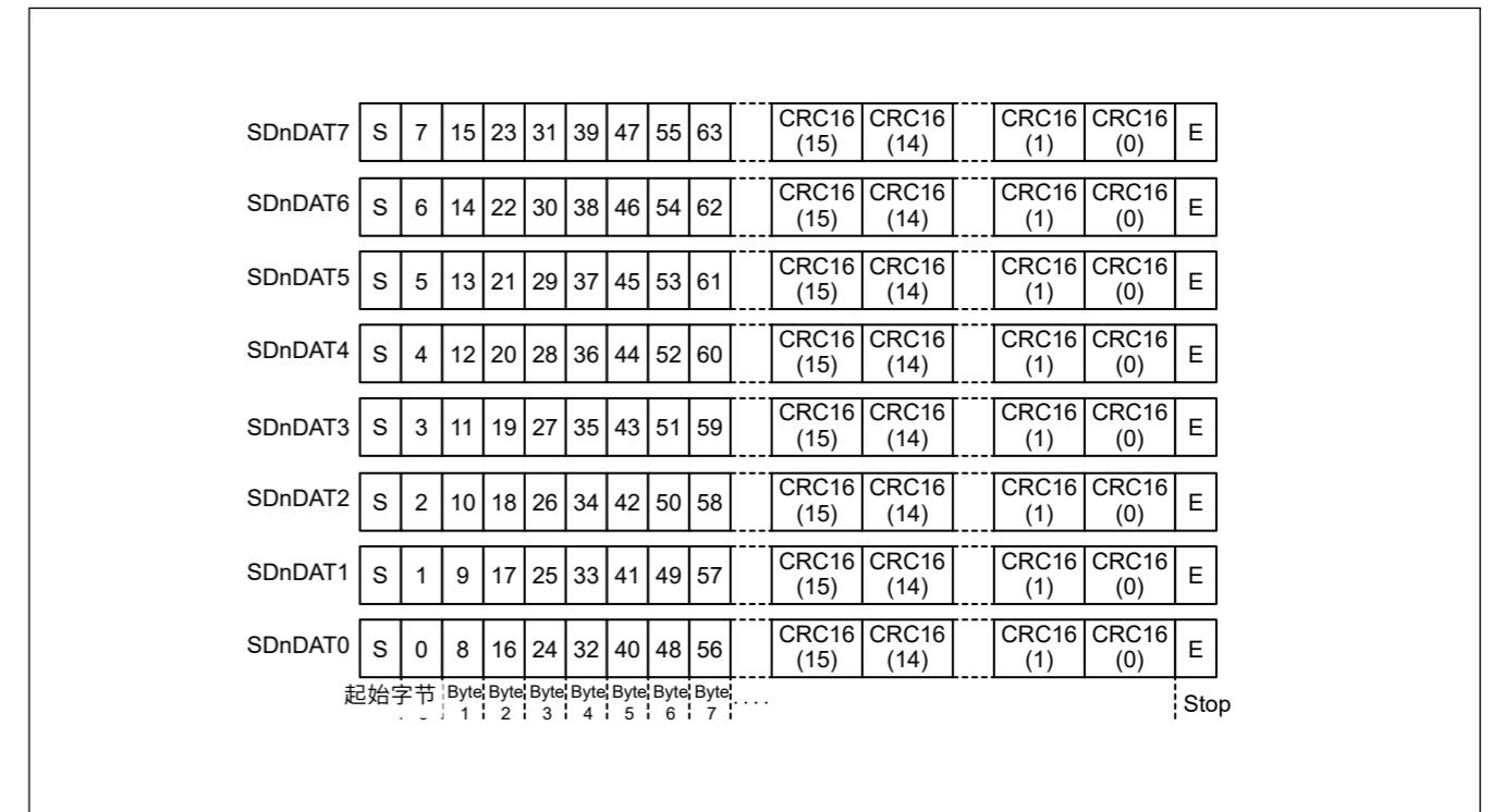
Figure 33.4 SDnDAT在8位宽度模式下
