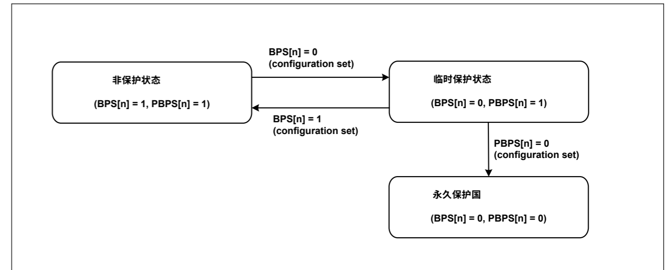
Figure 44.31 通过BPS[n]和PBPS[n]进行闪存定序器的状态转换
