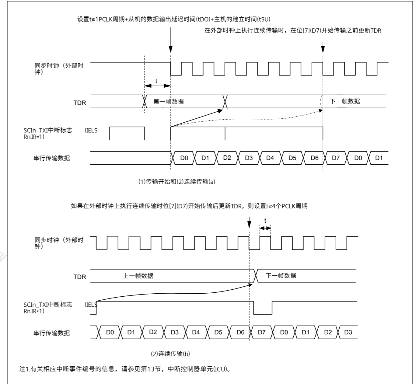
图27.123时钟同步传输中使用外部时钟的限制
