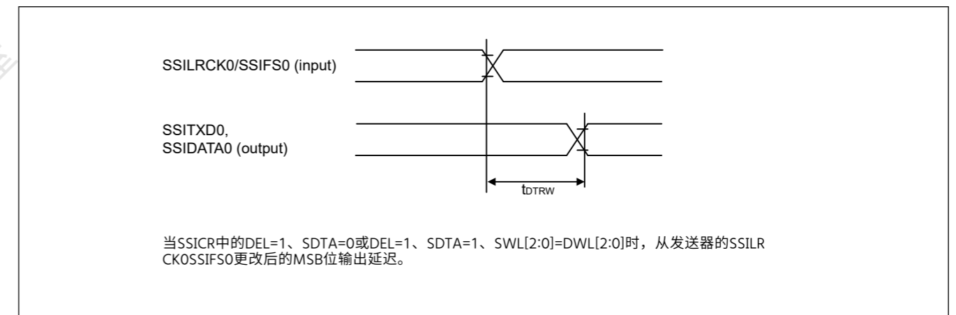
Figure 47.48 SSILRCKOSSIFS0更改后的SSIE数据输出延迟
