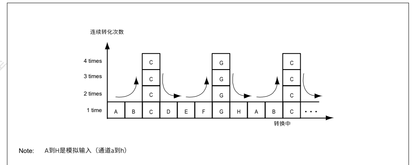
Figure 37.3 使用ADADC.ADC[2:0]=011b扫描转换序列，将模拟输入C和G设置为1 ADADS0/1
