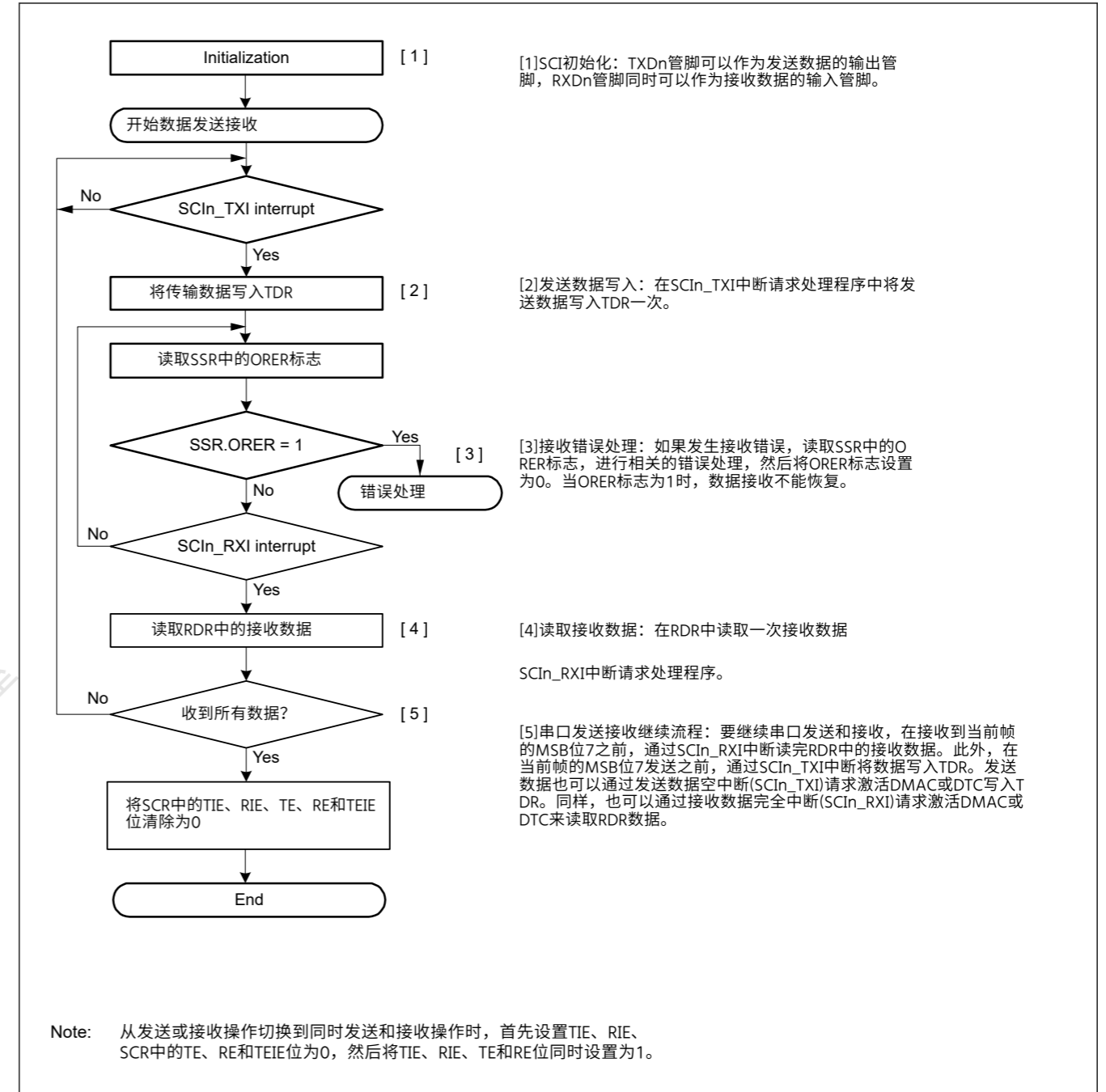
Figure 27.75 选择非FIFO的时钟同步模式下同时串行发送和接收的示例流程
