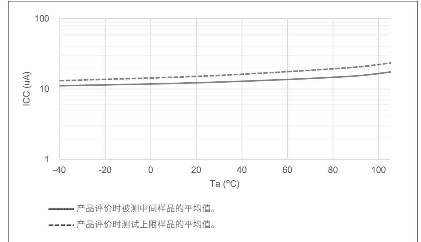
Figure 47.4 深度软件待机模式下的温度依赖性、未向SRAM或USB恢复检测单元供电、上电复位电路低功耗功能禁用（参考数据）
