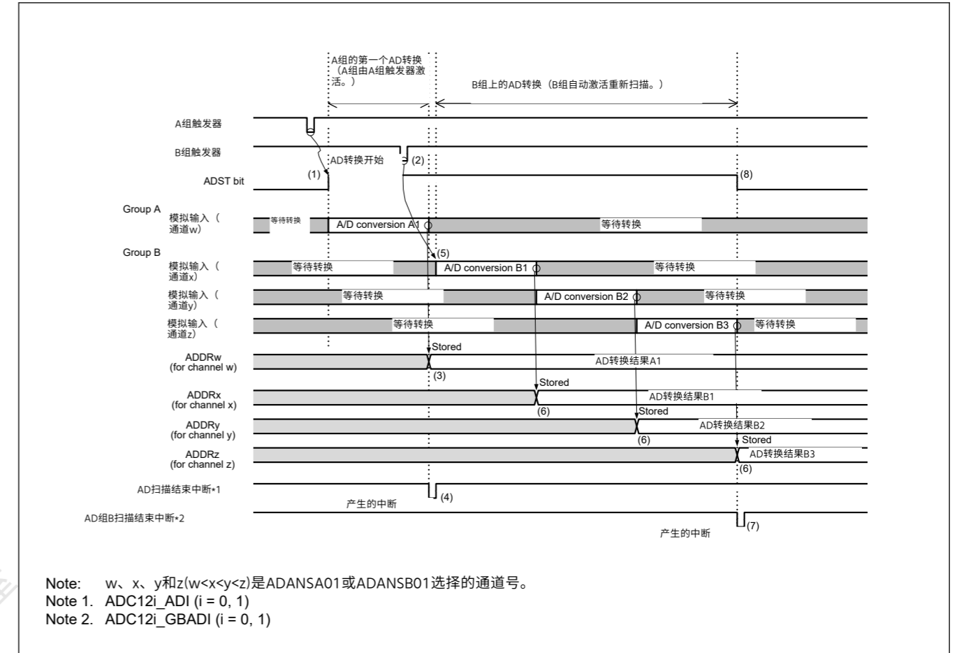
Figure 37.21 组优先操作1-3示例：启用重新扫描时A组扫描期间的B组触发输入（当ADGSPCR.GBRSCN=1、ADGSPCR.GBRP=0和ADGSPCR.LGRRS=0时）
