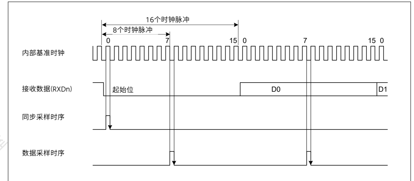
Figure 27.7 异步模式下接收数据采样时序
