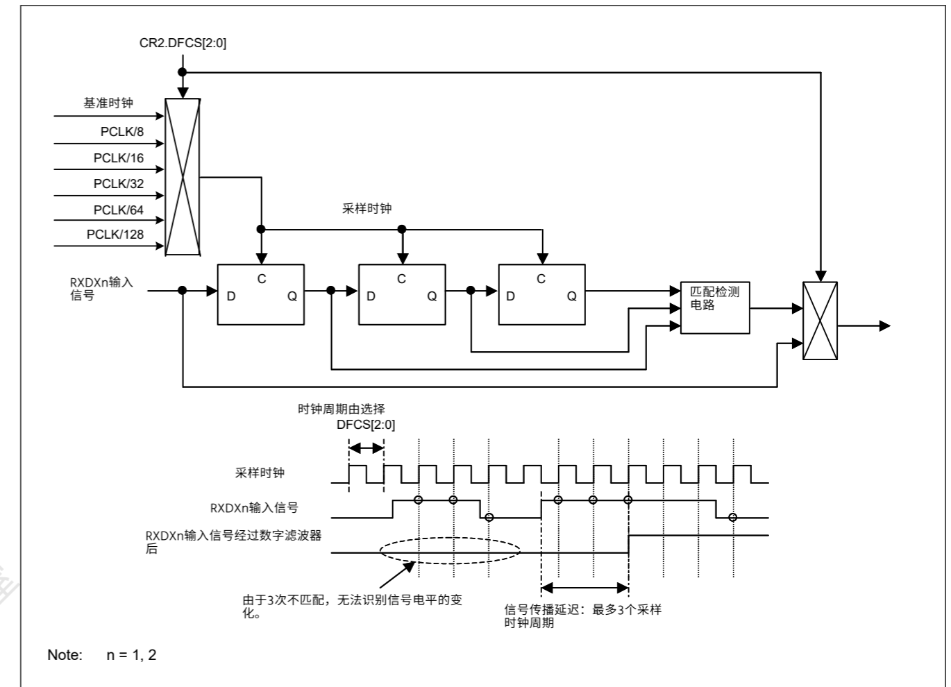
图27.112使用数字滤波器的操作示例
