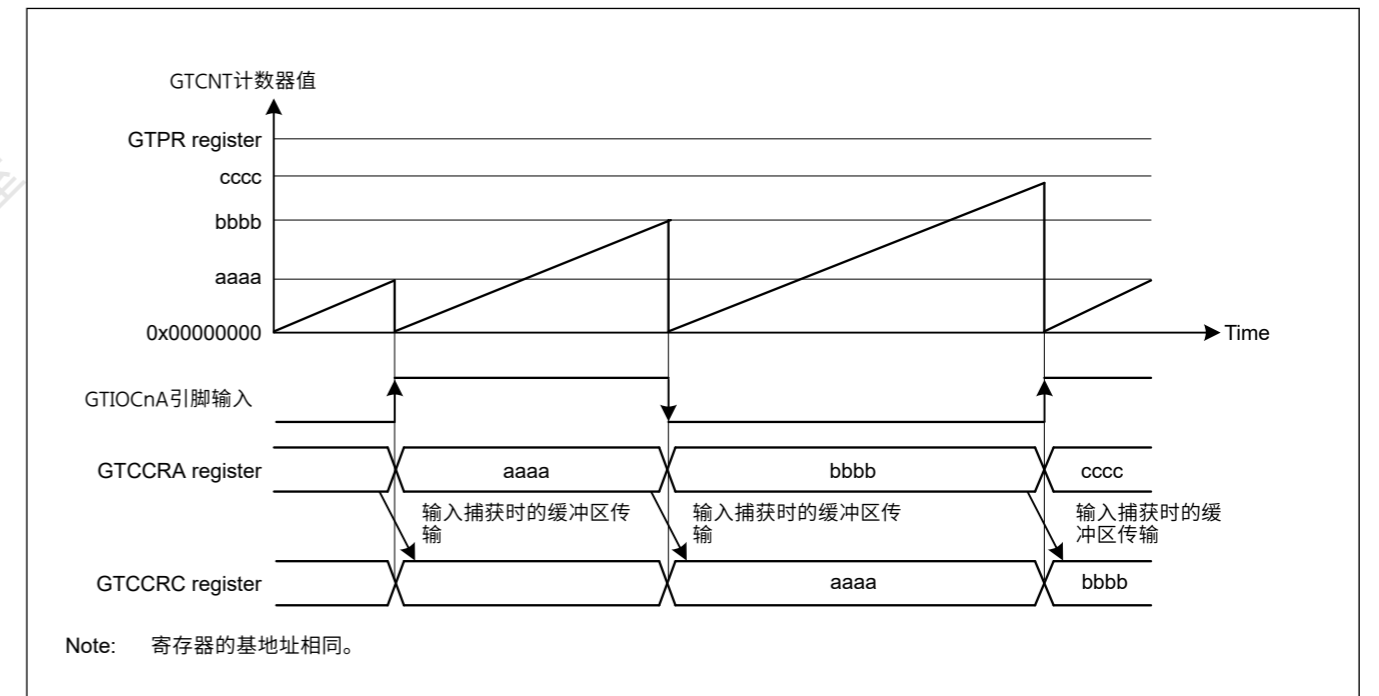
Figure 21.17 GTCCRA和GTCCRB缓冲区操作的示例，在两个边沿都有输入捕捉GTIOCnA输入，递增计数中的锯齿波，并且GTCNT计数器在GTIOCnA输入
