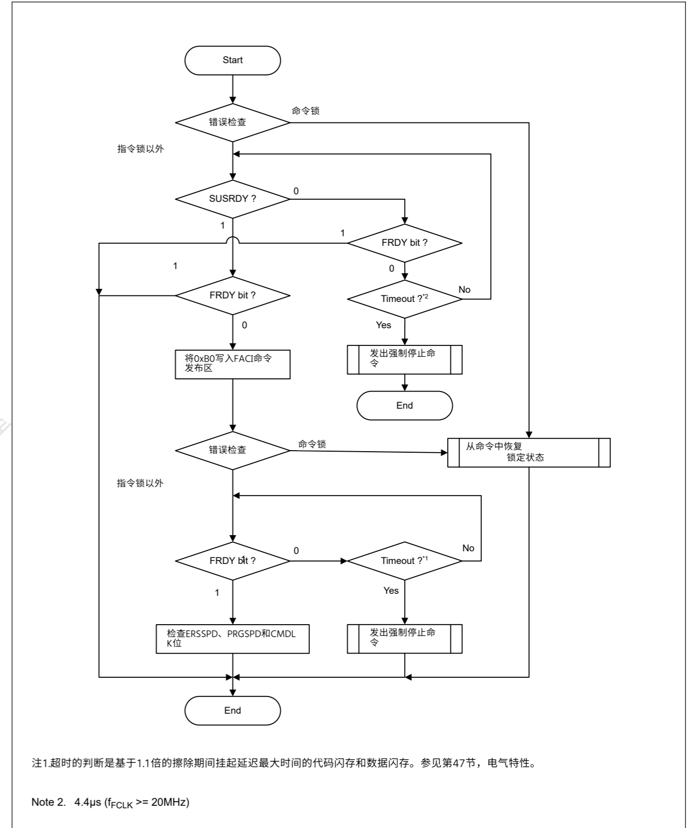
Figure 44.16 PE挂起命令的使用流程
