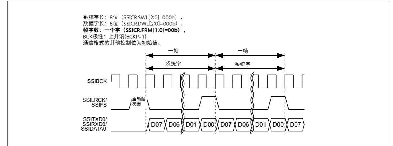
Figure 32.38 单声道格式的短帧 (无填充: 系统字长=数据字长)
