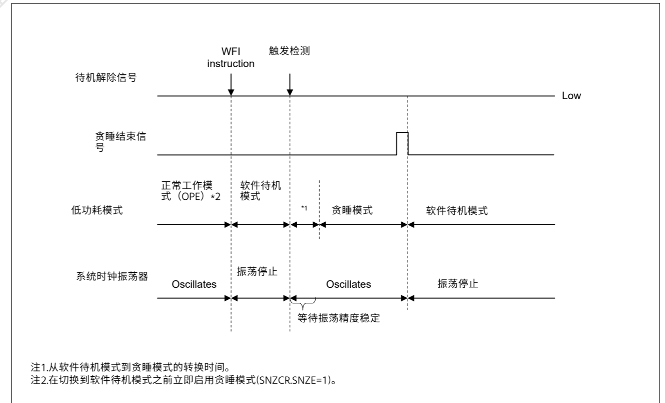
Figure 10.5 未产生中断请求信号时取消贪睡模式
