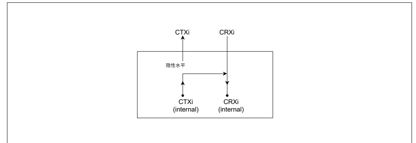
Figure 29.6 选择只听模式时的连接(i=0 1)
