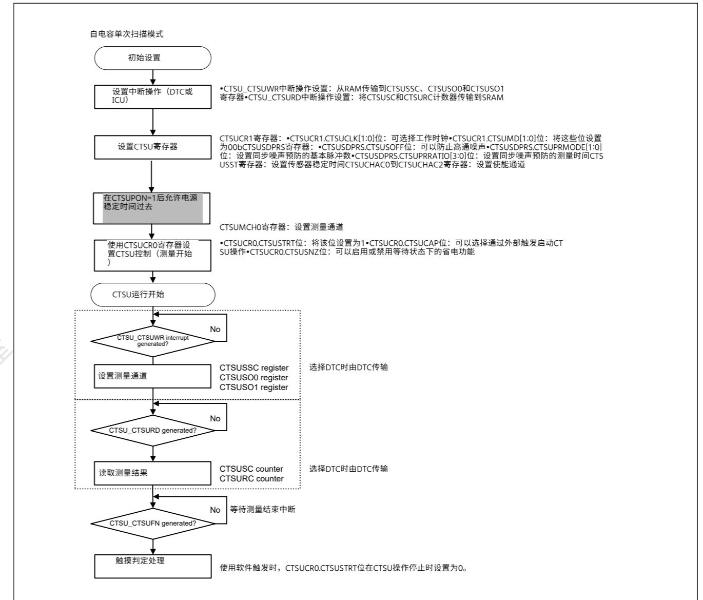
Figure 40.12 自电容单次扫描模式的软件流程和示例操作
