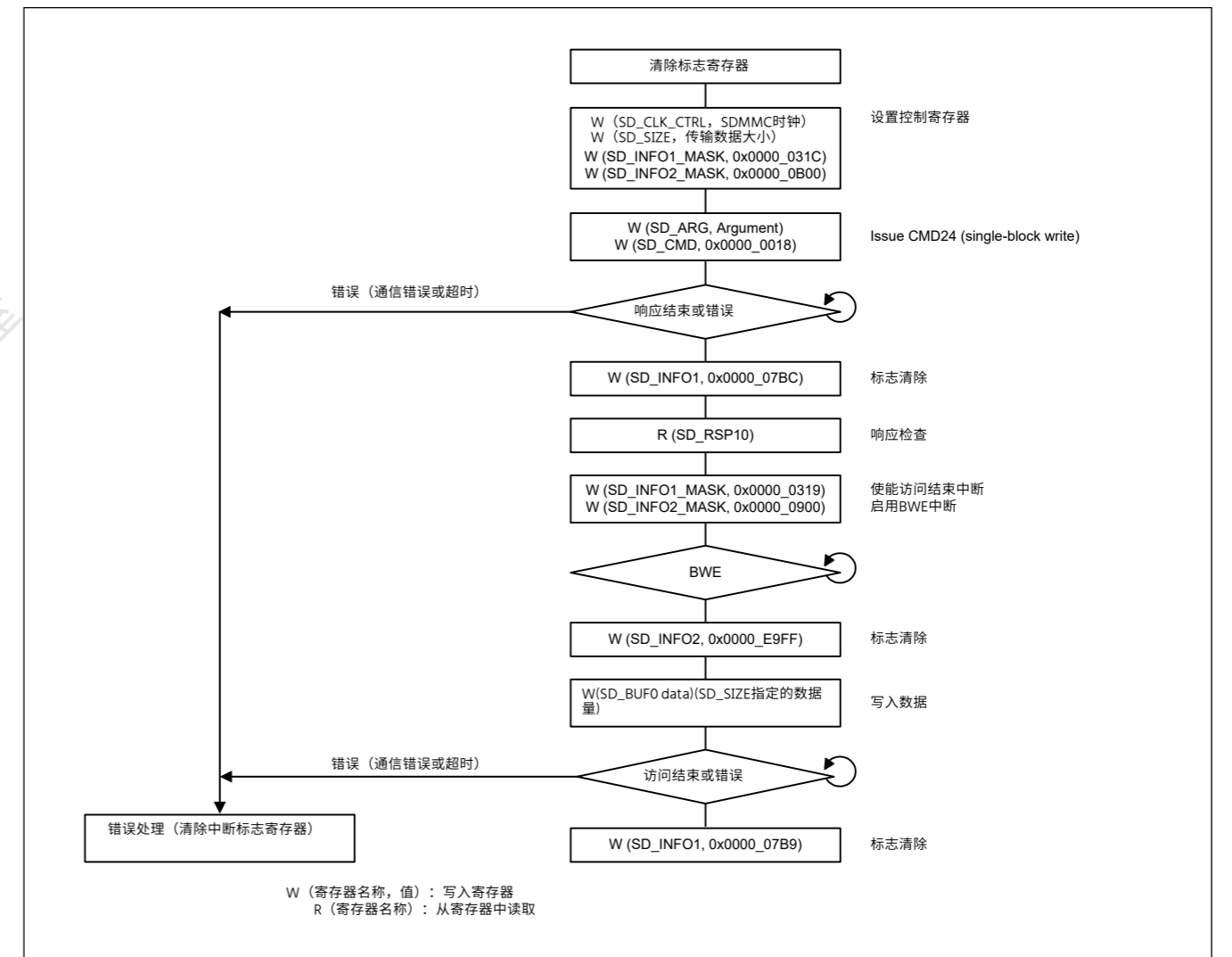
Figure 33.12 单块写操作示例
