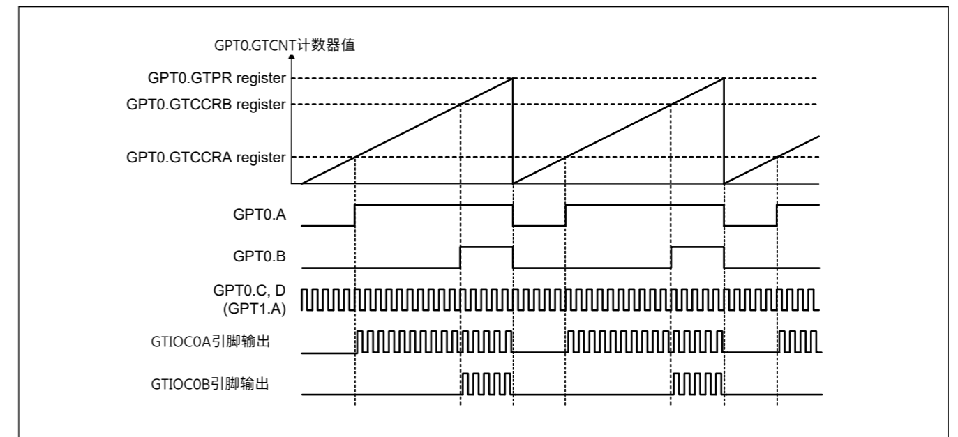
Figure 21.62 通道间逻辑运算示例
