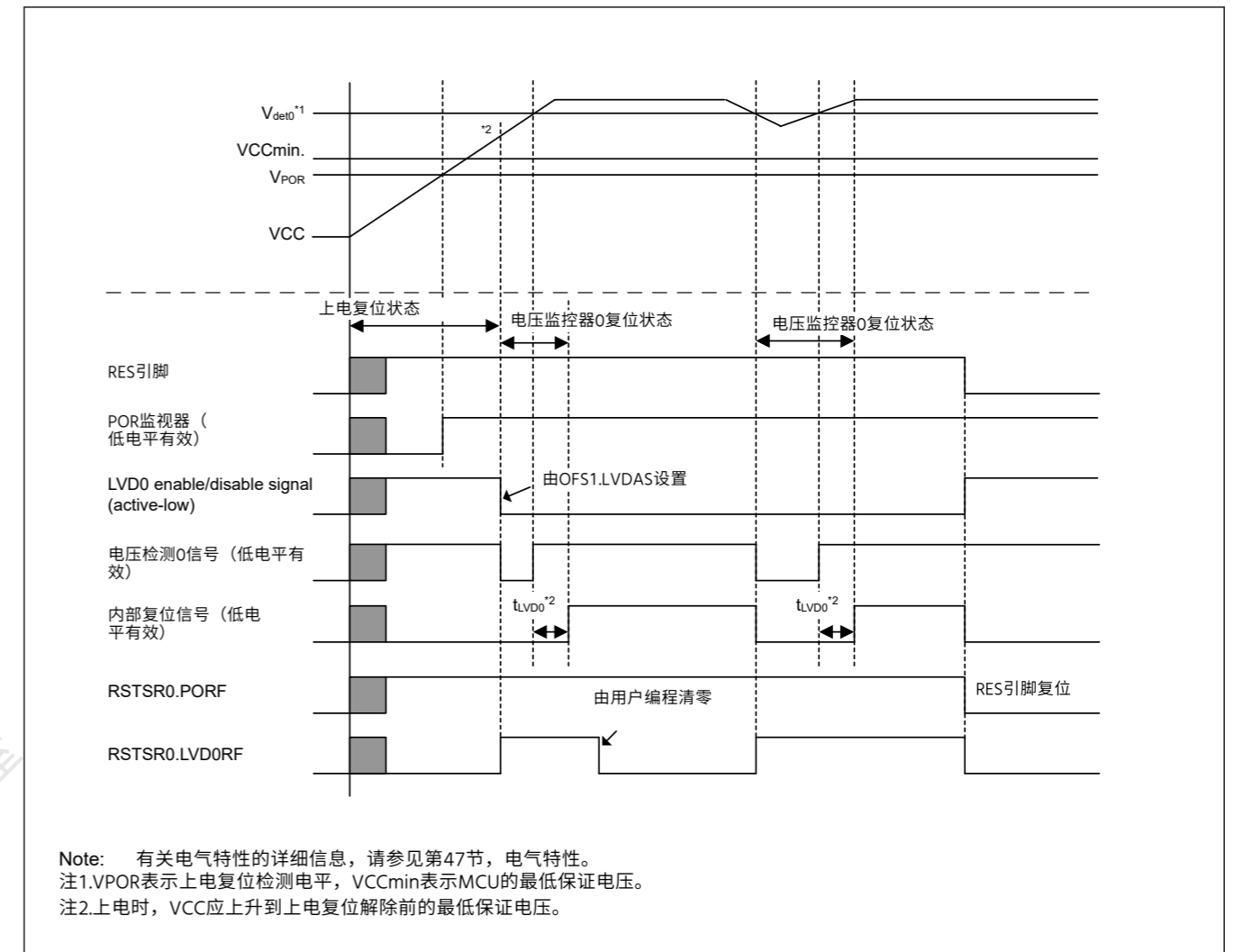
Figure 5.1 上电复位时的动作示例
