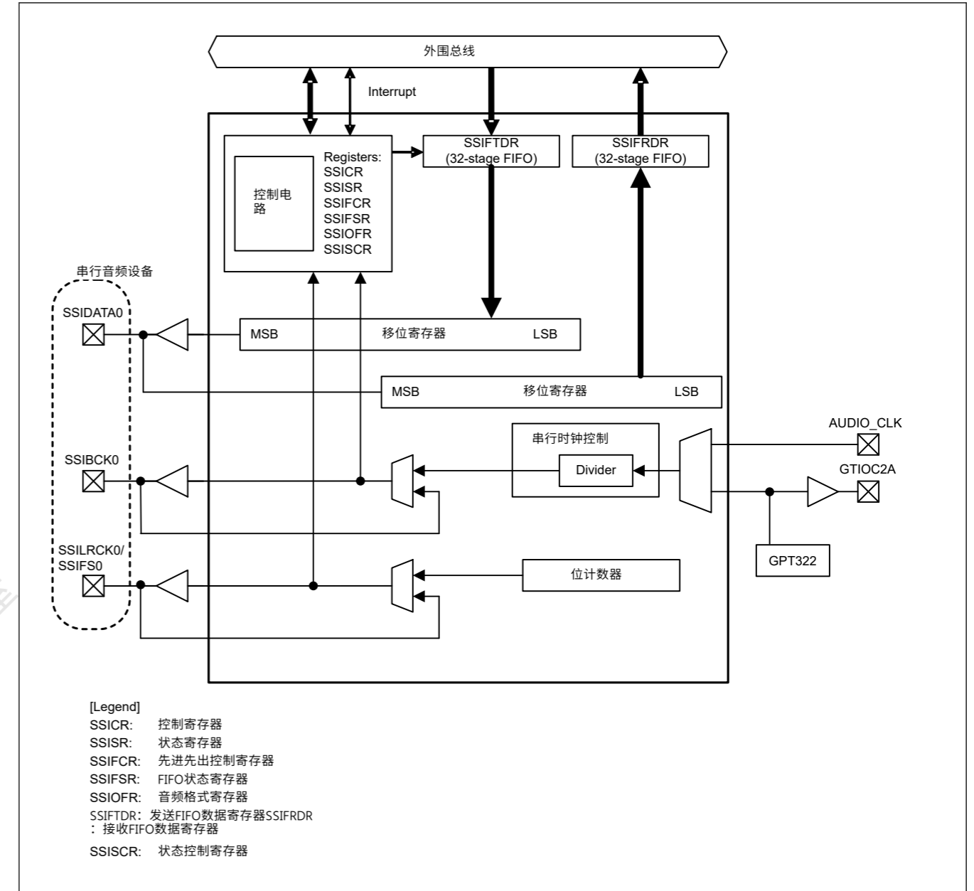
Figure 32.3 半双工通信的SSIE框图
