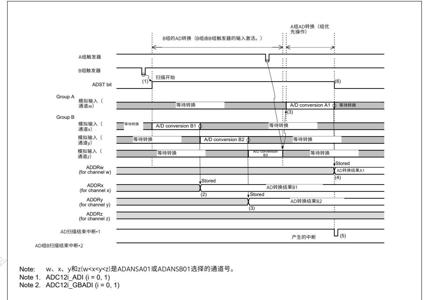
Figure 37.22 组优先操作示例1-4: “在B组扫描期间输入A组触发”当禁用重新扫描时 (当ADGSPCR.GBRSCN=0、ADGSPCR.GBRP=0和ADGSPCR.LGRRS=0时)
