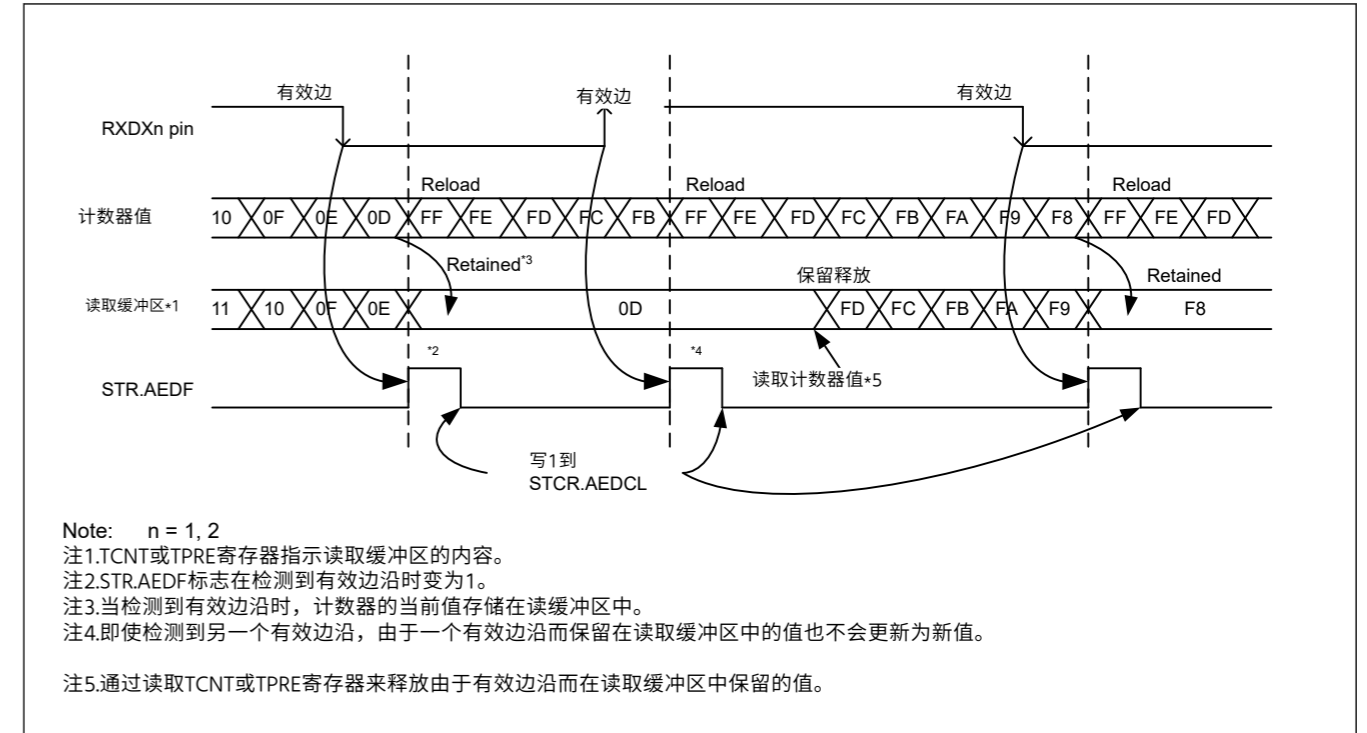
图27.113比特率测量操作示例
