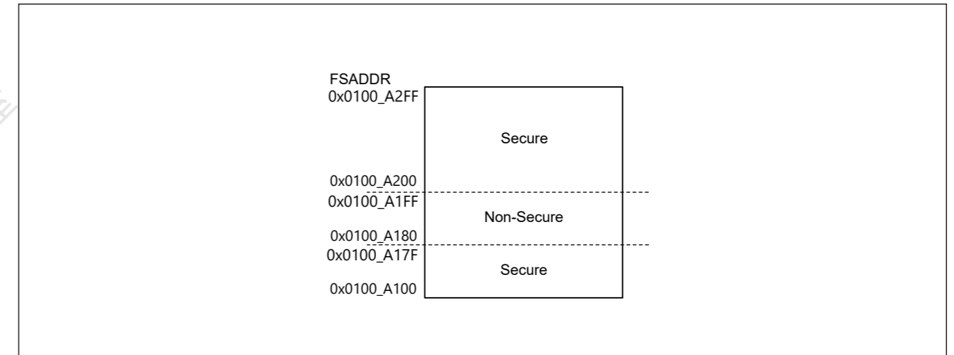
Figure 44.35 选项设置内存中的安全非安全区域
