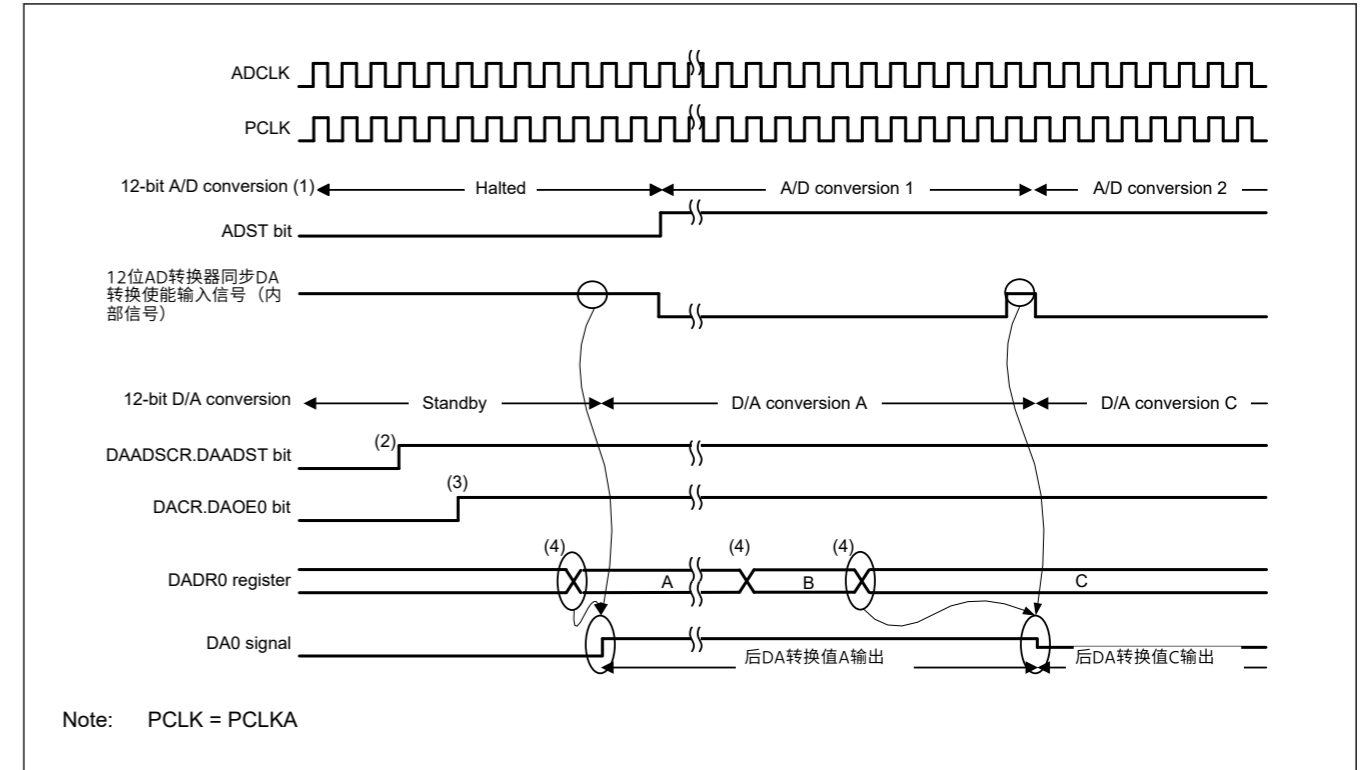
Figure 38.3 DAC12与ADC12同步时的转换示例 (单元1)
