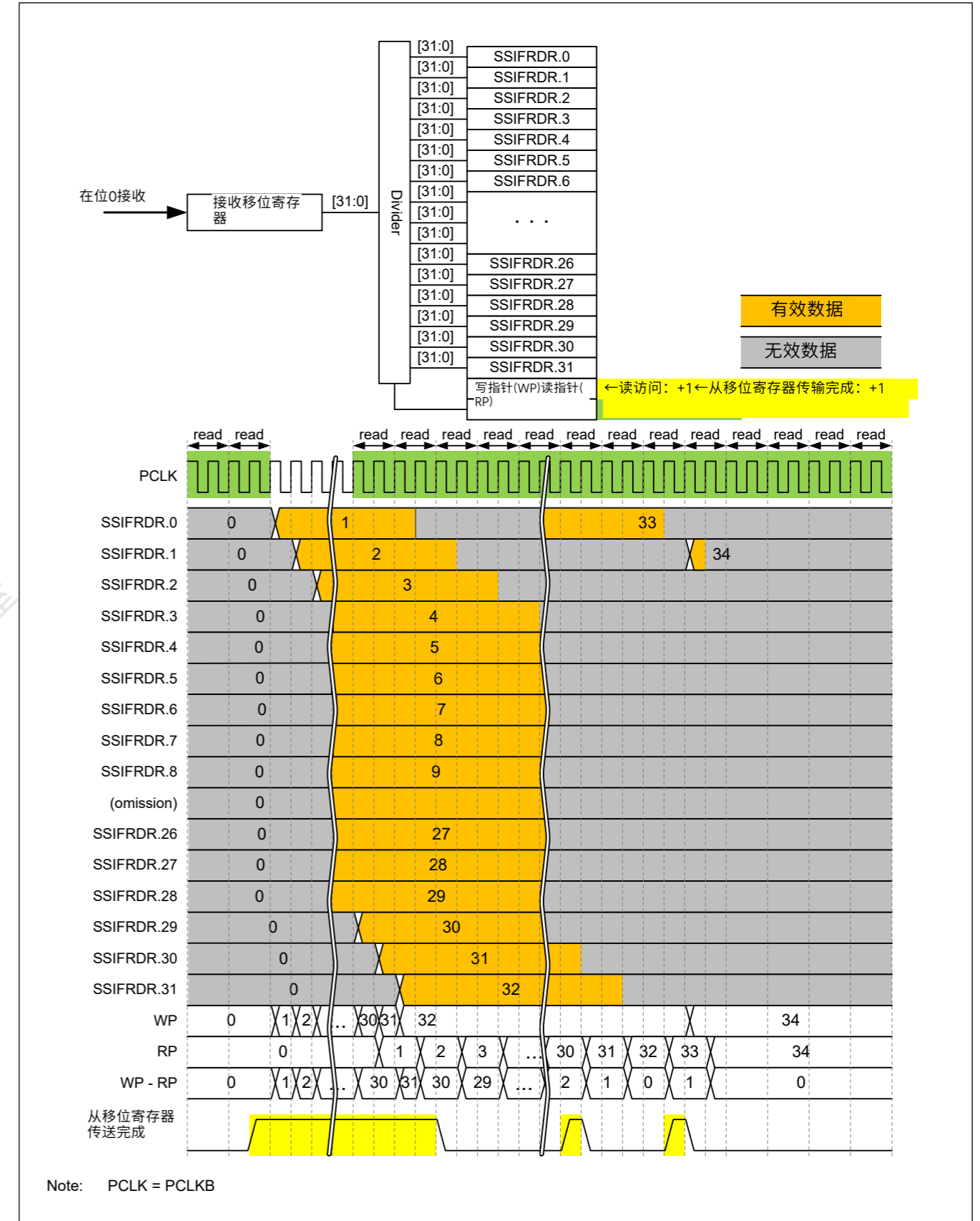
Figure 32.32 发送FIFO数据寄存器和发送移位寄存器的配置，以及FIFO操作示例
