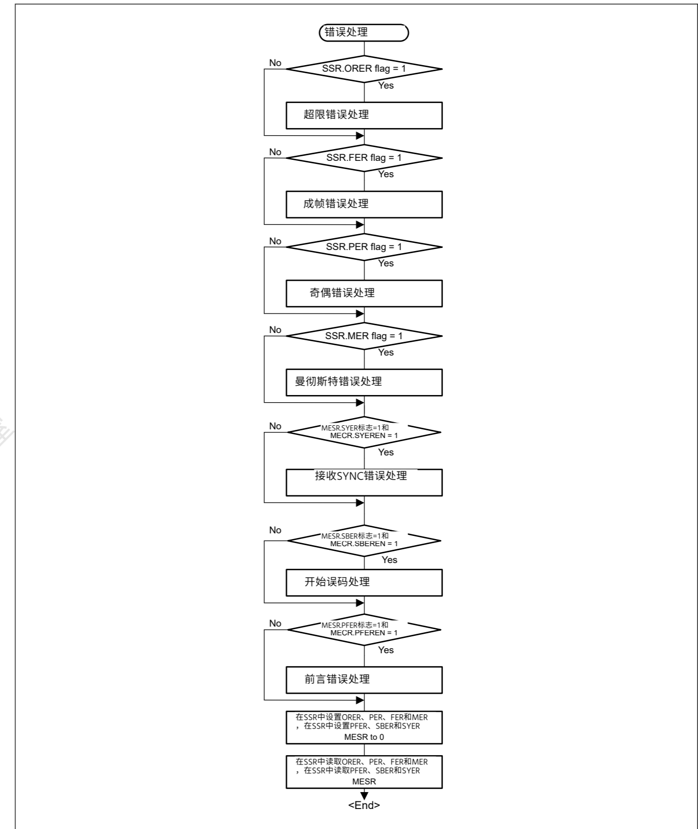
Figure 27.62 曼彻斯特模式下的串行接收流程图示例 (错误处理)
