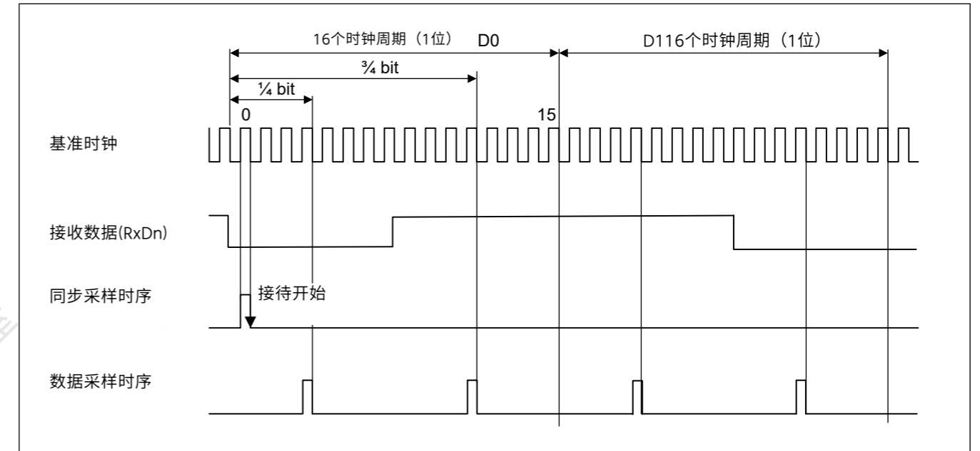
Figure 27.59 曼彻斯特模式下的数据接收采样时序
