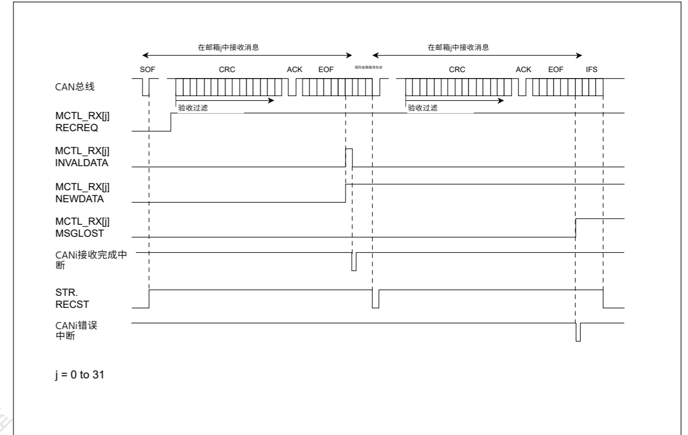
Figure 29.19 溢出模式下数据帧接收的操作示例
