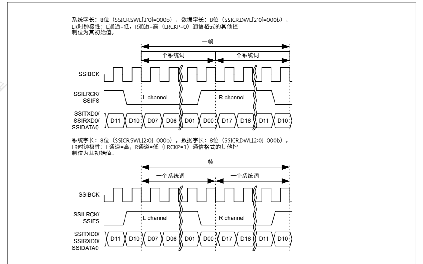
Figure 32.12 LR时钟帧同步极性设置
