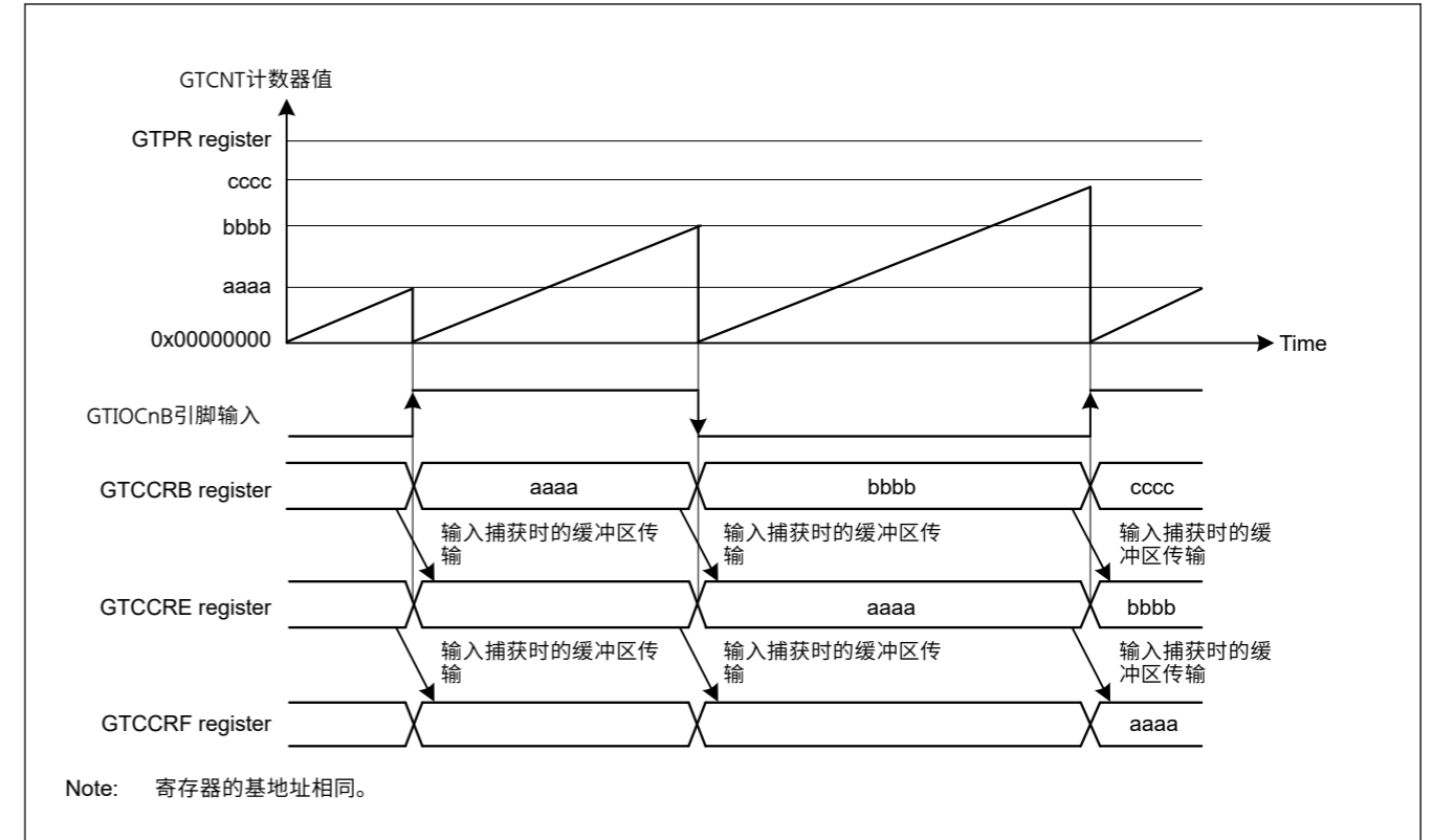
Figure 21.18 GTCCRA和GTCCRB双缓冲操作示例，在两个边沿进行输入捕获 GTIOcNB输入，递增计数中的锯齿波，GTCNT计数器在两个边缘清零 GTIOcNB input
