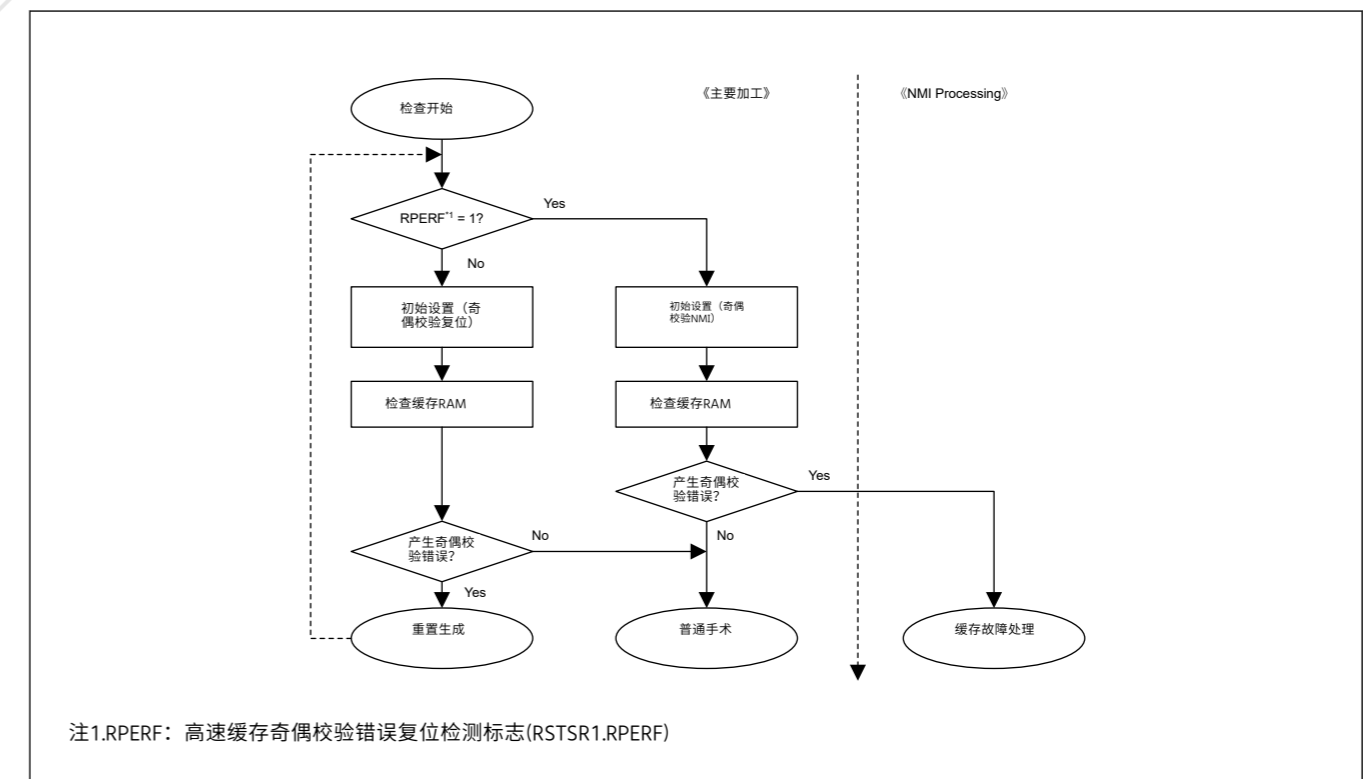
Figure 14.8 启用奇偶校验时的缓存奇偶校验流程
