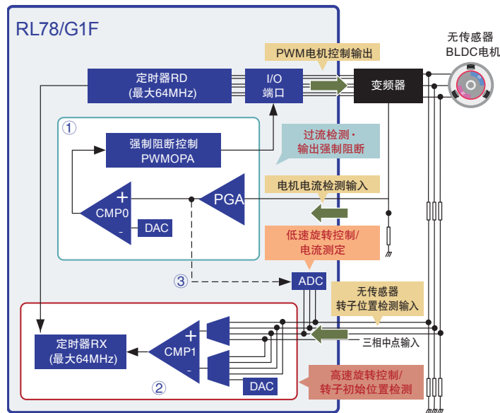
RL78的无传感器BLDC电机控制示例
